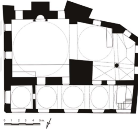
Şekil 7: Hatuniye Cami rölovesi (Ürer, 2017:231).
