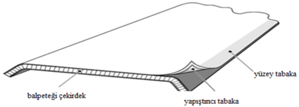
Şekil 5.16 Kalıplama yöntemiyle imal edilmiş örnek bir kompozit yapı [69]
