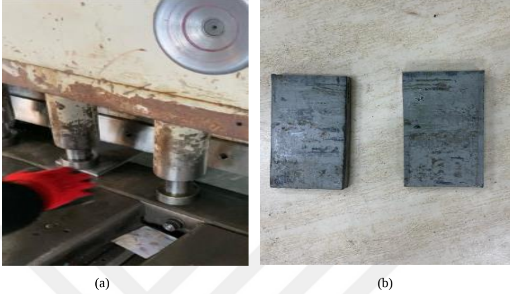
Şekil 7.19 (a) Metal levhanın basma deneyi için giyotin makasında kesilme işlemi (b) Kesim sonrası hali
