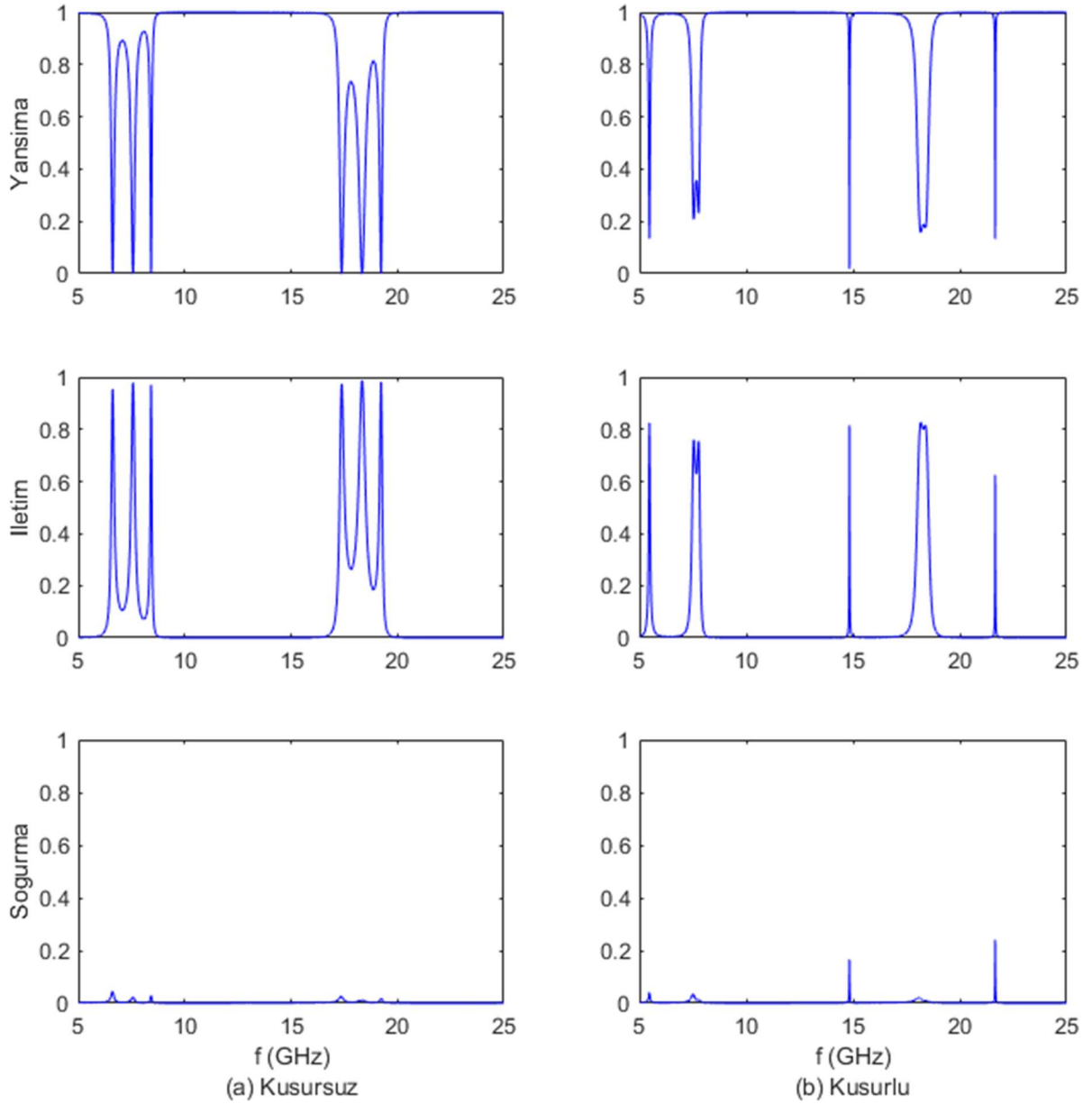
Şekil 4.1. Periyodik dizilime göre tasarlanan kusursuz ve kusurlu PFK yapısı için yansım, iletim ve soğurma katsayısı
