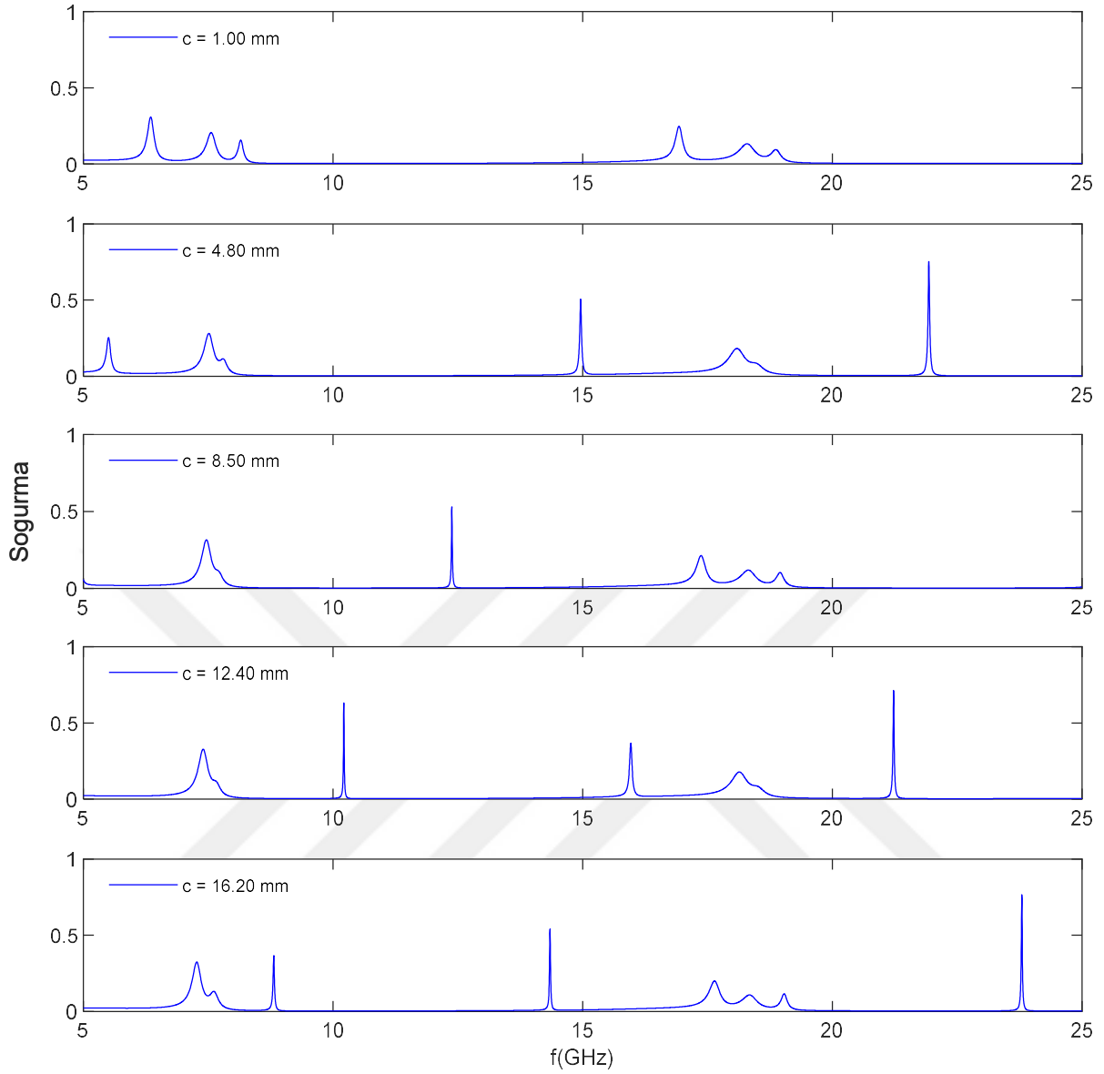
Şekil 4.4. Periyodik dizilimin c = 1 \text{ mm} , 4.8 \text{ mm} , 8.6 \text{ mm} , 12.4 \text{ mm} , 16.2 \text{ mm} kusur katmanı kalınlığı değerleri için soğurma katsayısı
