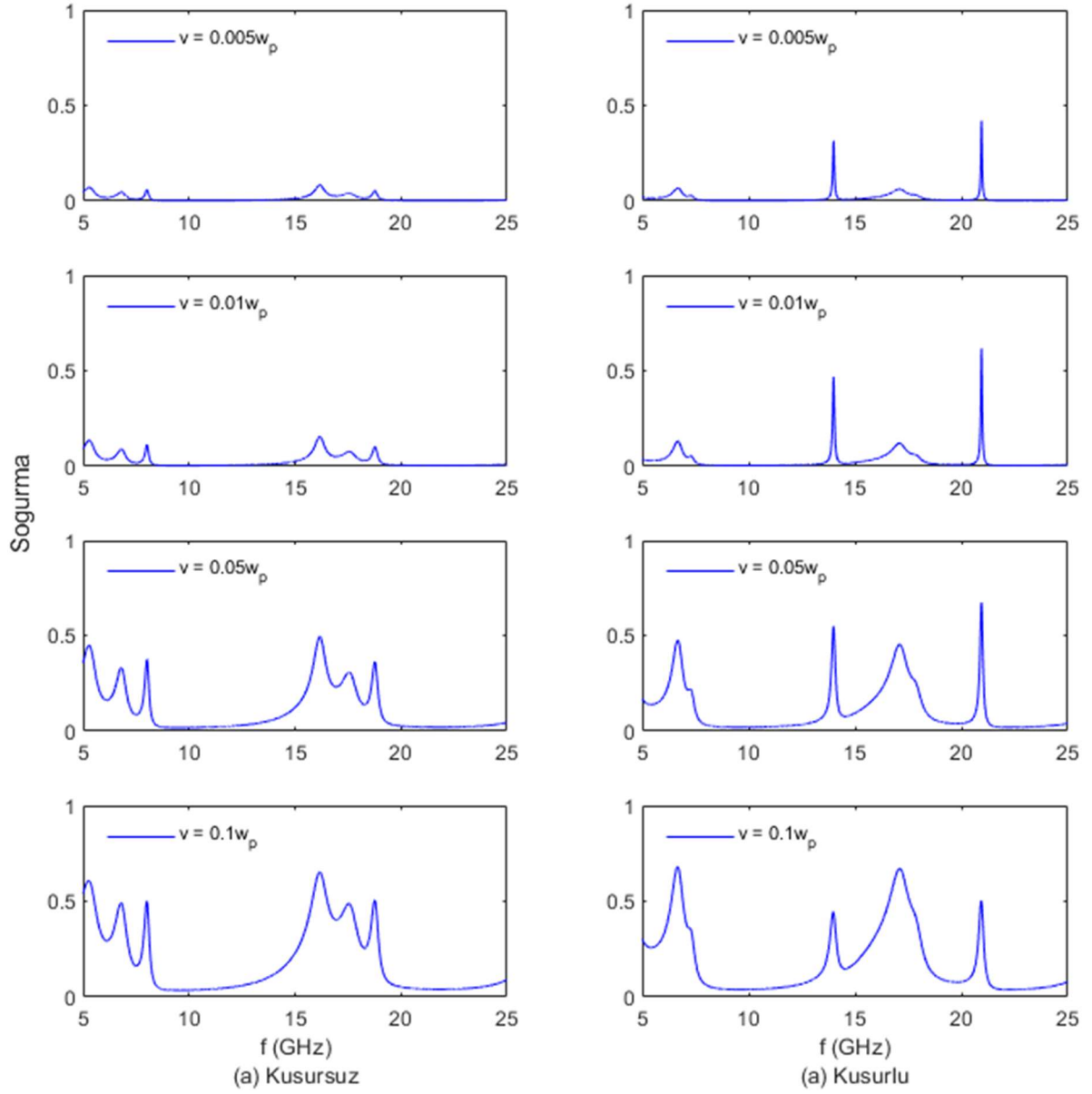
Şekil 4.16. Periyodik dizilimin çarpışma frekansı \nu = 0.005\omega_p, 0.01\omega_p, 0.05\omega_p, 0.1\omega_p değerleri için soğurma katsayısı
