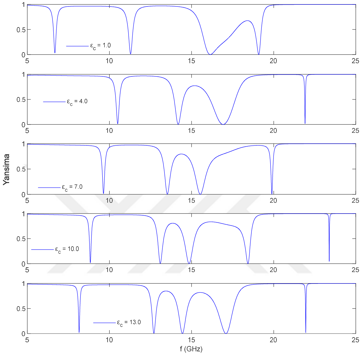
Şekil 4.21. Cantor dizilimin kusur katmanı \epsilon_c = 1, 4, 7, 10, 13 dielektrik sabiti değerleri için yansımaya katsayısı
