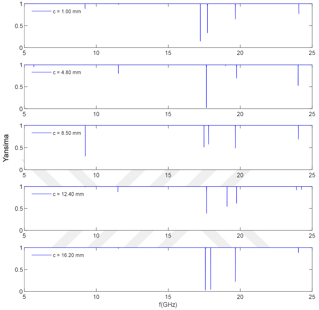
Şekil 3.16. Fibonacci dizilimin c = 1 \text{ mm} , 4.8 \text{ mm} , 8.6 \text{ mm} , 12.4 \text{ mm} , 16.2 \text{ mm} kusur katmanı kalınlığı değerleri için yansima katsayısı
