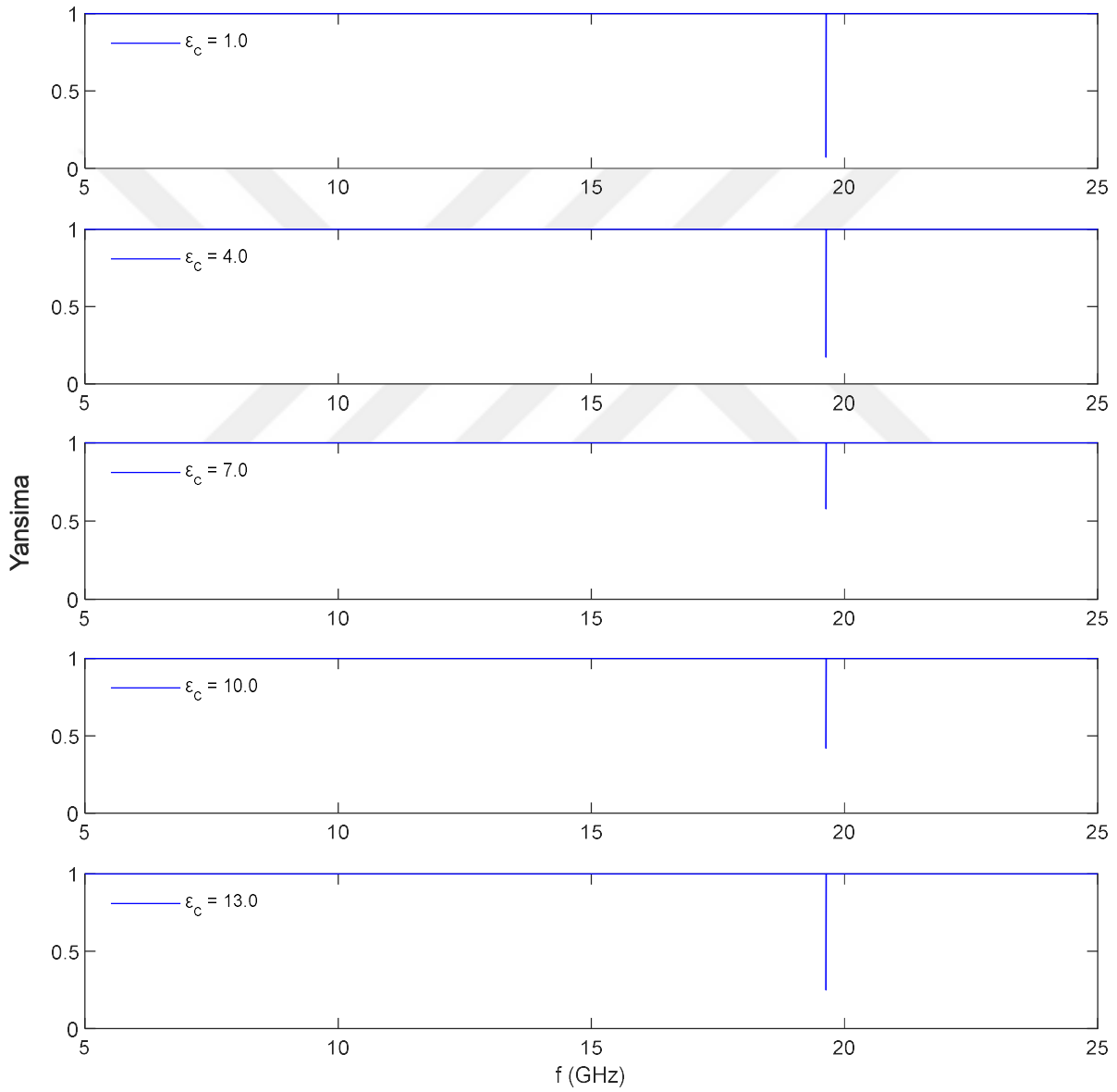
Şekil 3.26. Thue-morse dizilimin kusur katmanı \epsilon_c = 1, 4, 7, 10, 13 dielektrik sabiti değerleri için yansımaya katsayısı
