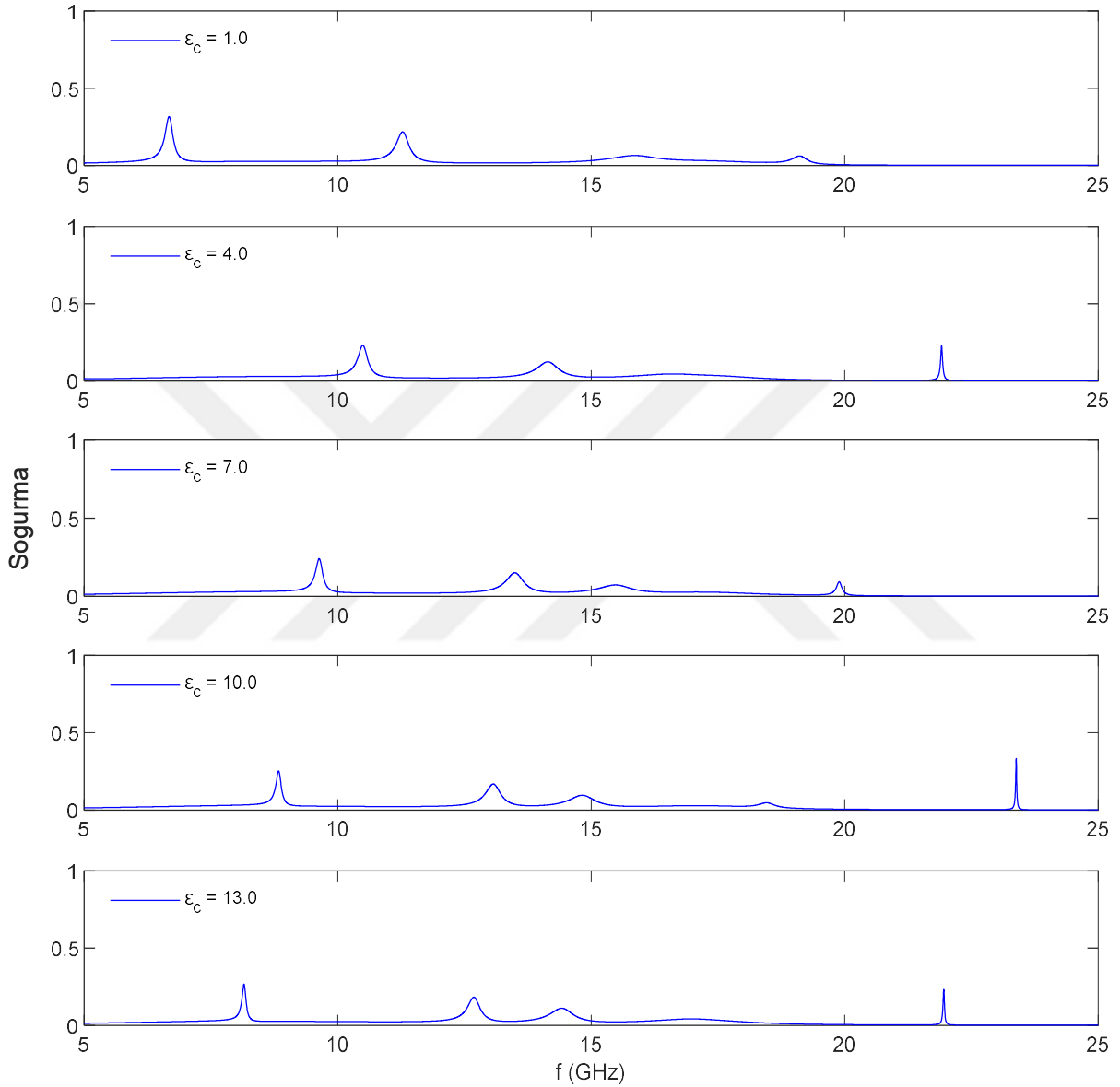
Şekil 4.23. Cantor dizilimin kusur katmanı \varepsilon_c = 1, 4, 7, 10, 13 dielektrik sabiti değeriileri için soğurma katsayısı
