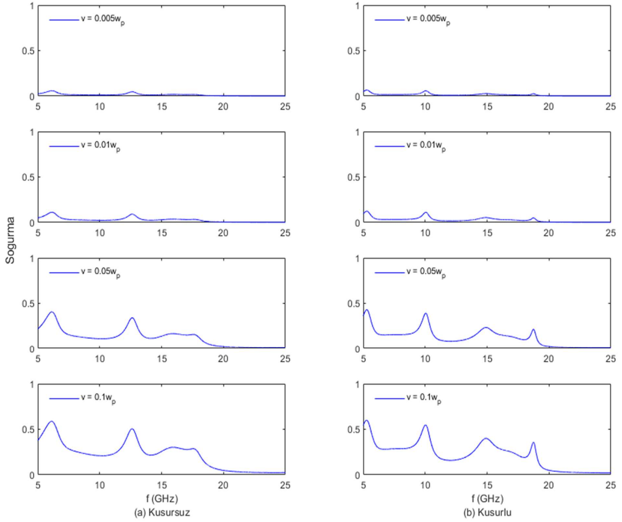
Şekil 4.32. Cantor dizilimin çarpışma frekansı \nu = 0.005\omega_p, 0.01\omega_p, 0.05\omega_p, 0.1\omega_p değerleri için soğurma katsayısı
