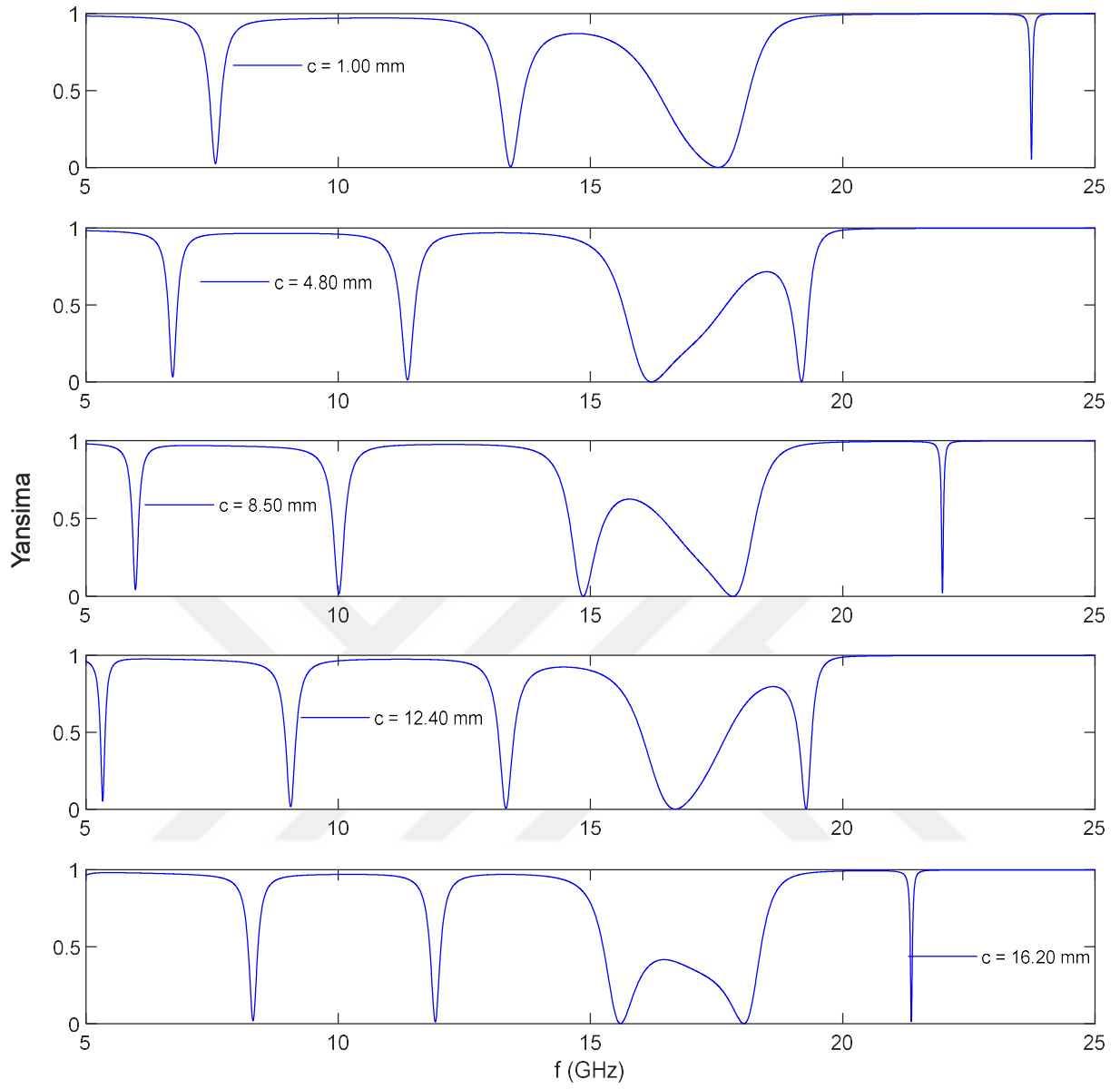
Şekil 4.18. Cantor dizilimin c = 1 \text{ mm} , 4.8 \text{ mm} , 8.6 \text{ mm} , 12.4 \text{ mm} , 16.2 \text{ mm} kusur katmanı kalınlığı değerleri için yansima katsayısı
