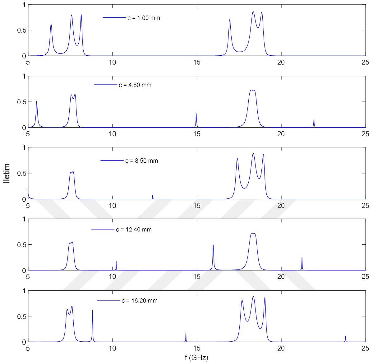
Şekil 4.3. Periyodik dizilimin c = 1 mm, 4.8 mm, 8.6 mm, 12.4 mm, 16.2 mm kusur katman kalınlığı değerleri için iletim katsayısı
