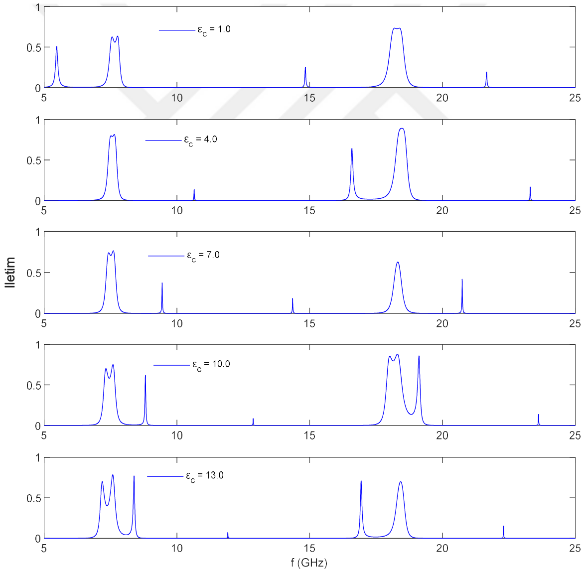
Şekil 4.6. Periyodik dizilimin kusur katmanı \epsilon_c = 1, 4, 7, 10, 13 dielektrik sabiti değerleri için iletim katsayısı
