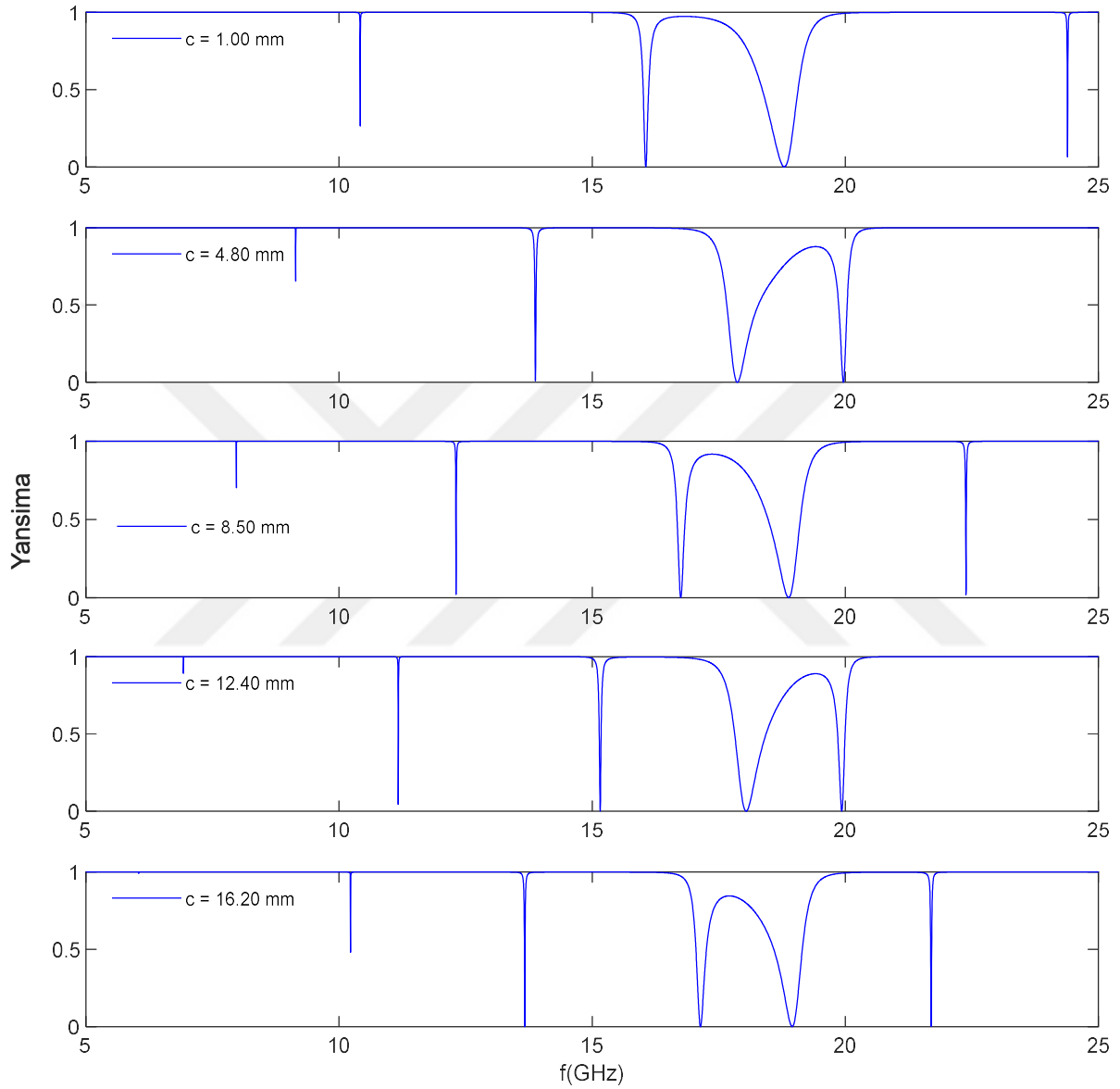
Şekil 3.32. Cantor dizilimin c = 1 \text{ mm} , 4.8 \text{ mm} , 8.6 \text{ mm} , 12.4 \text{ mm} , 16.2 \text{ mm} kusur katmanı kalınlığı değerleri için yansımaya katsayısı
