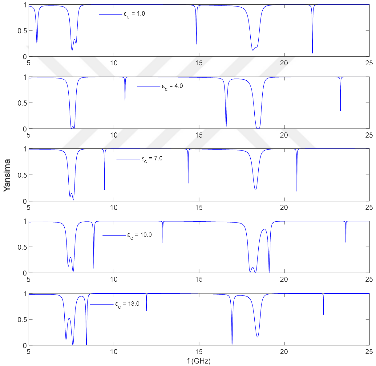
Şekil 4.5. Periyodik dizilimin kusur katmanı \epsilon_c = 1, 4, 7, 10, 13 dielektrik sabiti değerleri için yansıma katsayısı
