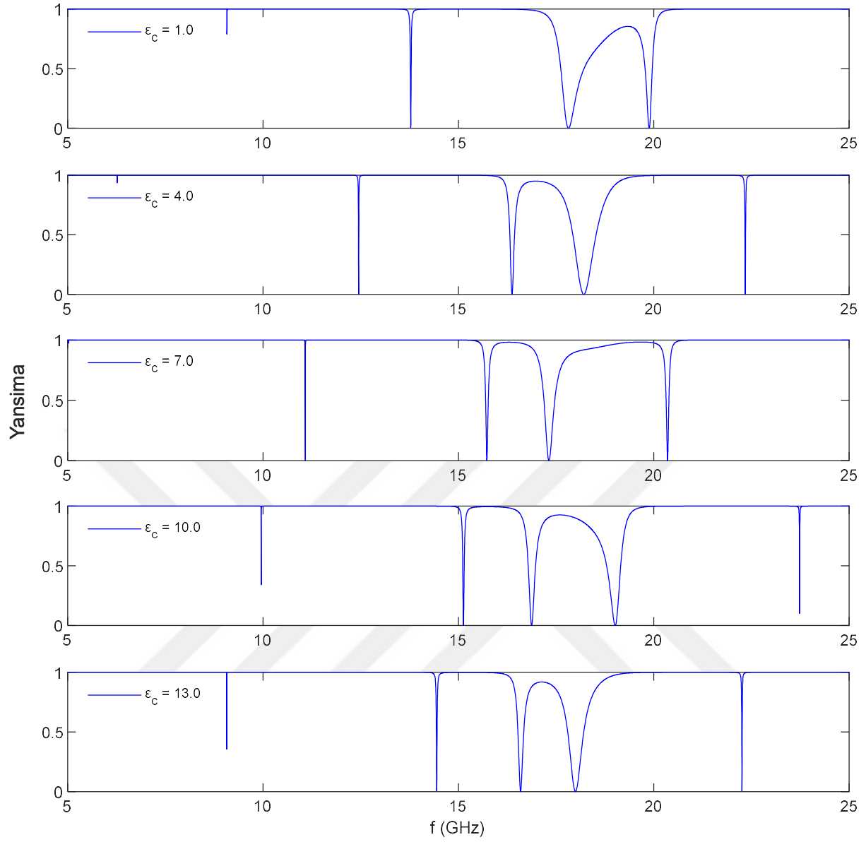
Şekil 3.34. Cantor dizilimin kusur katmanı \epsilon_c = 1, 4, 7, 10, 13 dielektrik sabiti değerleri için yansima katsayısı
