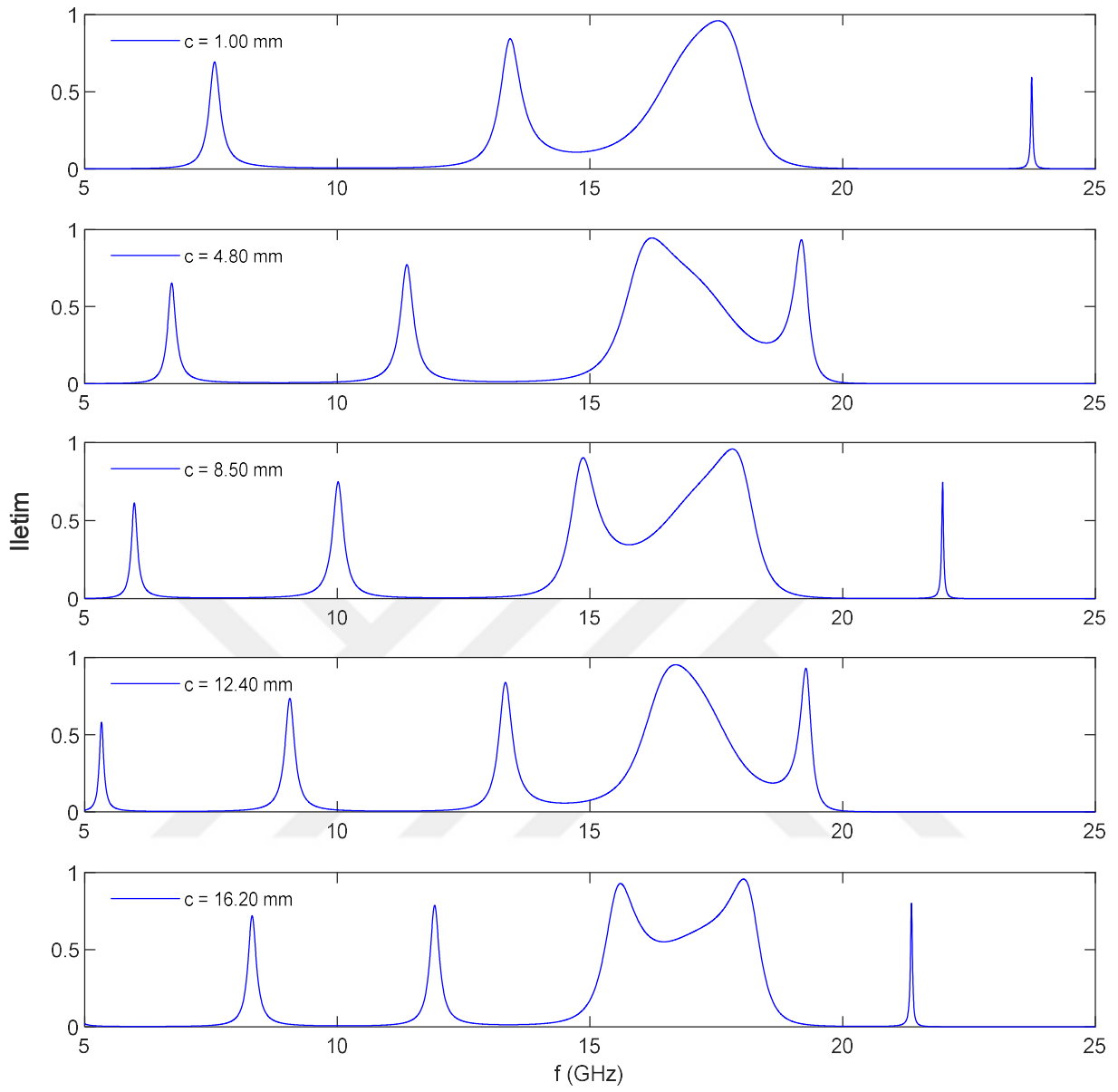
Şekil 4.19. Cantor dizilimin c = 1 \text{ mm} , 4.8 \text{ mm} , 8.6 \text{ mm} , 12.4 \text{ mm} , 16.2 \text{ mm} kusur katmanı kalınlığı değerleri için iletim katsayısı
