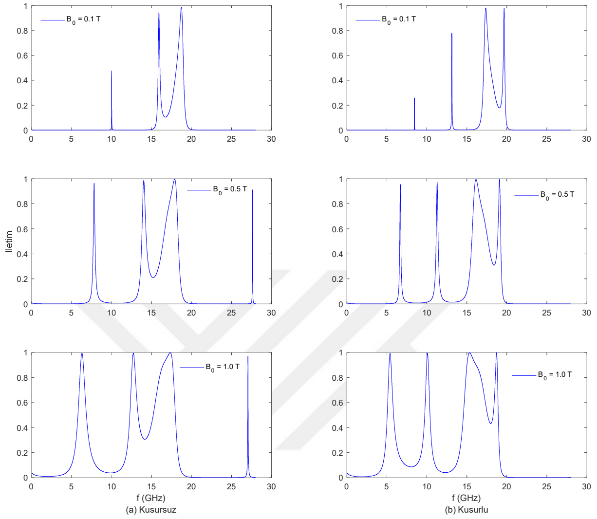
Şekil 4.28. Cantor dizilimin B_0 = 0.1 \text{ T} , 0.5 \text{ T} , 1 \text{ T} dış manyetik alan değerleri için iletim katsayısı
