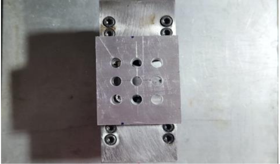
Şekil 4.5. Hava soğutma yöntemi ile delinen numune.
