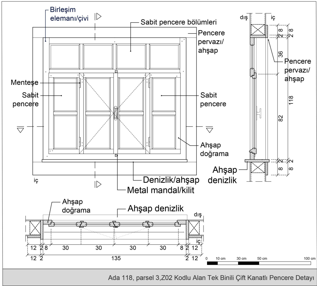
Şekil 5.44 Ada 118, parsel 3'teki konutun çift kanatlı pencere detayı (2023)
