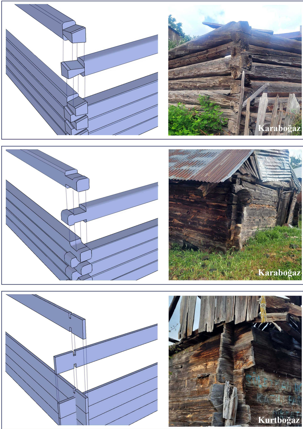
Şekil 5.20 Deveören Köyü'ndeki ambar yapılarında karaboğaz ve kurtboğaz birleşim detayları (Ç:V. O., 2022)
