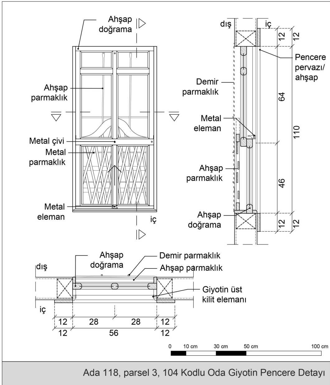
Şekil 5.45 Ada 118, parsel 3'teki konutun giyotin pencere ve parmaklık detayı (2023)
