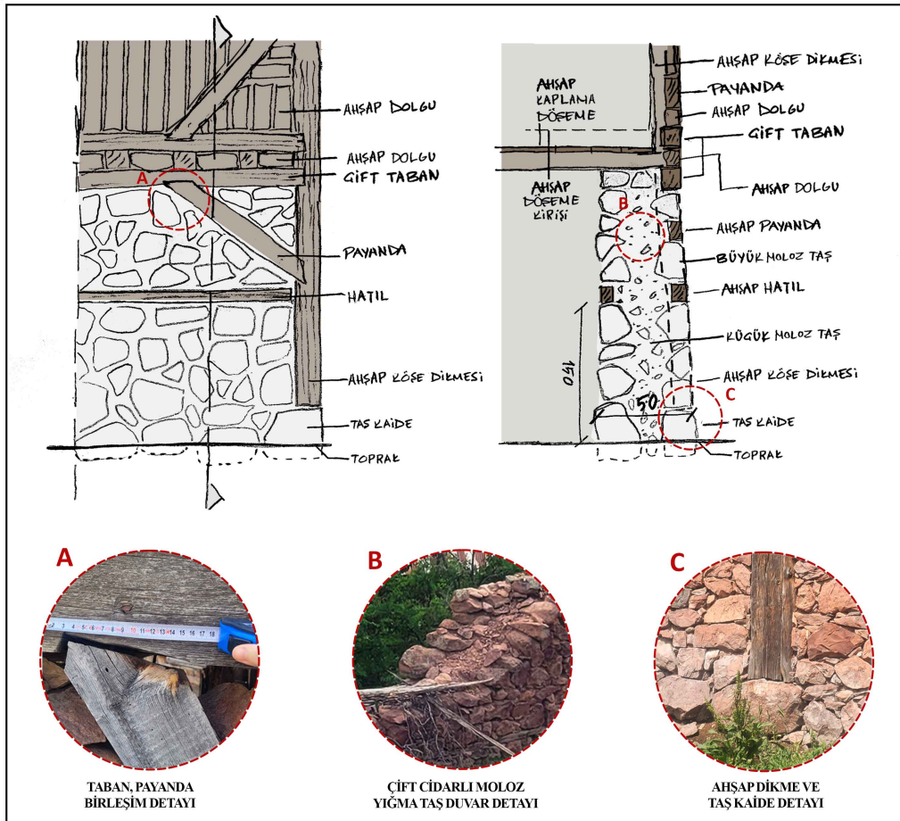
Şekil 5.57 Zemin katta ahır olan mekânların ahşap taşıyıcılı moloz taş duvar teknikleri (Ç:V.O., 2023)
