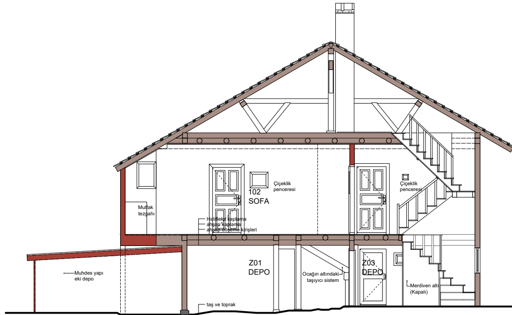
A-A KESİTİ
