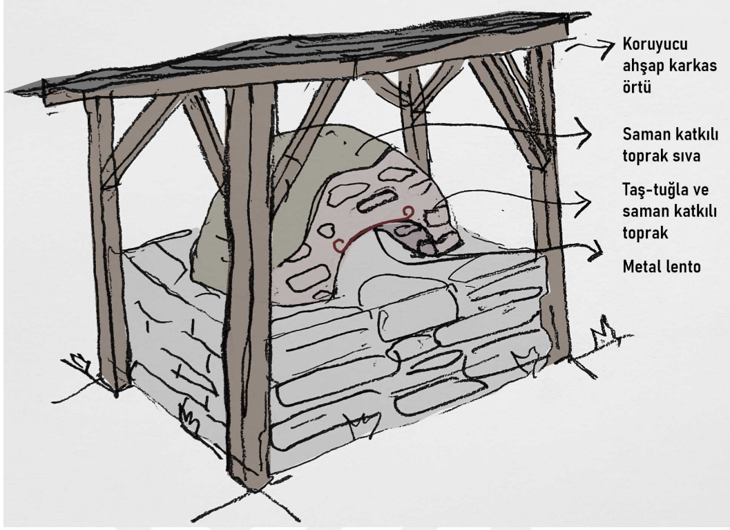
Şekil 5.7 Köydeki ortak fırınların yapım tekniği, yapı malzemeleri ve muhdes ahşap taşıyıcıyı sistem örtü (Ç:V.O.2024)
