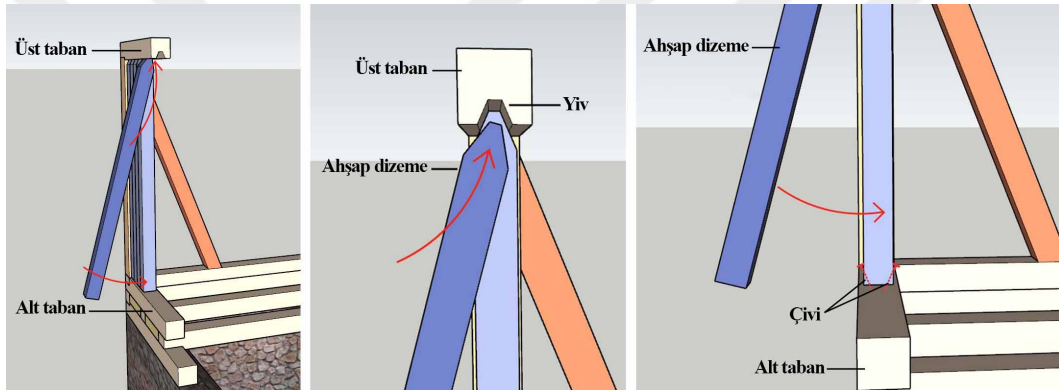
Şekil 5.59 Ahşap dizemenin yapılışı (Ç:V.O., 2023)
