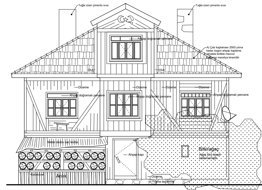
GÜNEYBATI GÖRÜNÜŞÜ
