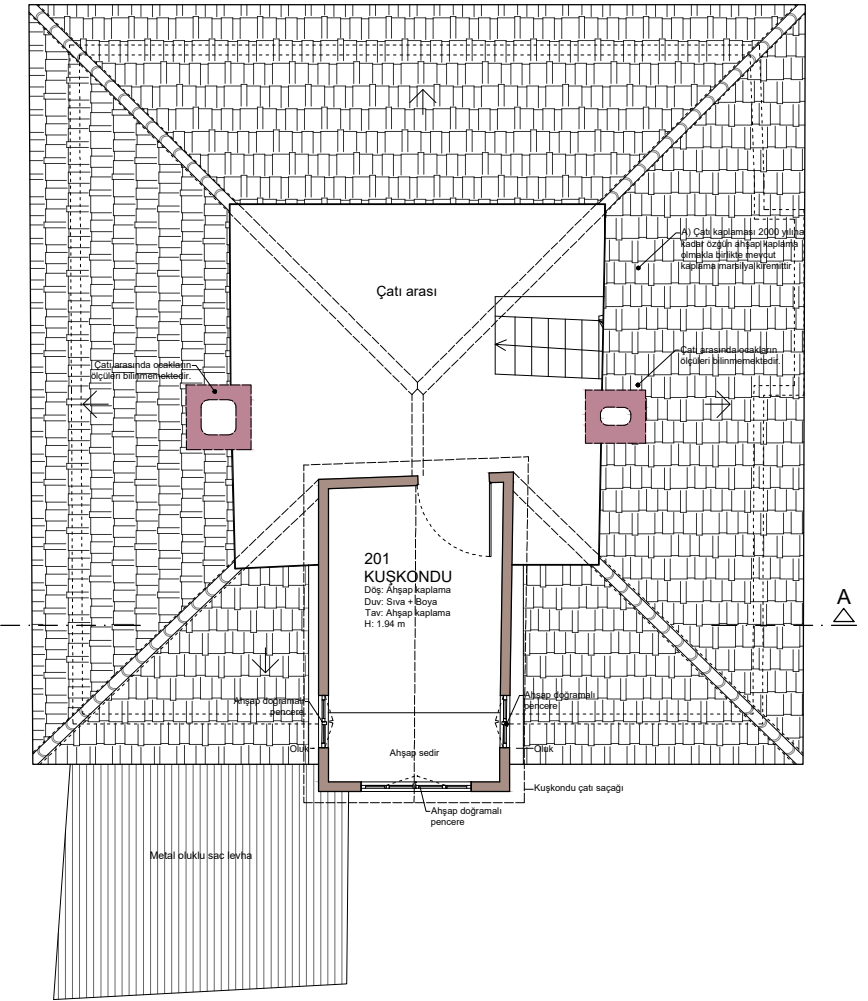
2. KAT(KUŞKONDU) PLANI
