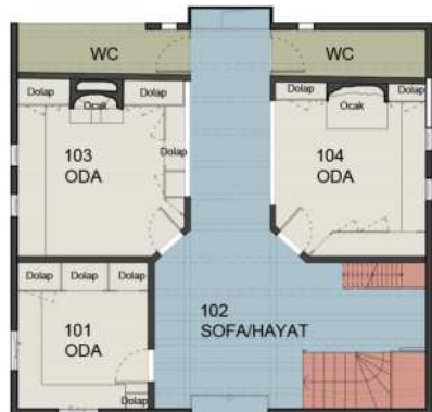
1. KAT PLANI ADA/PARSEL:118/15
