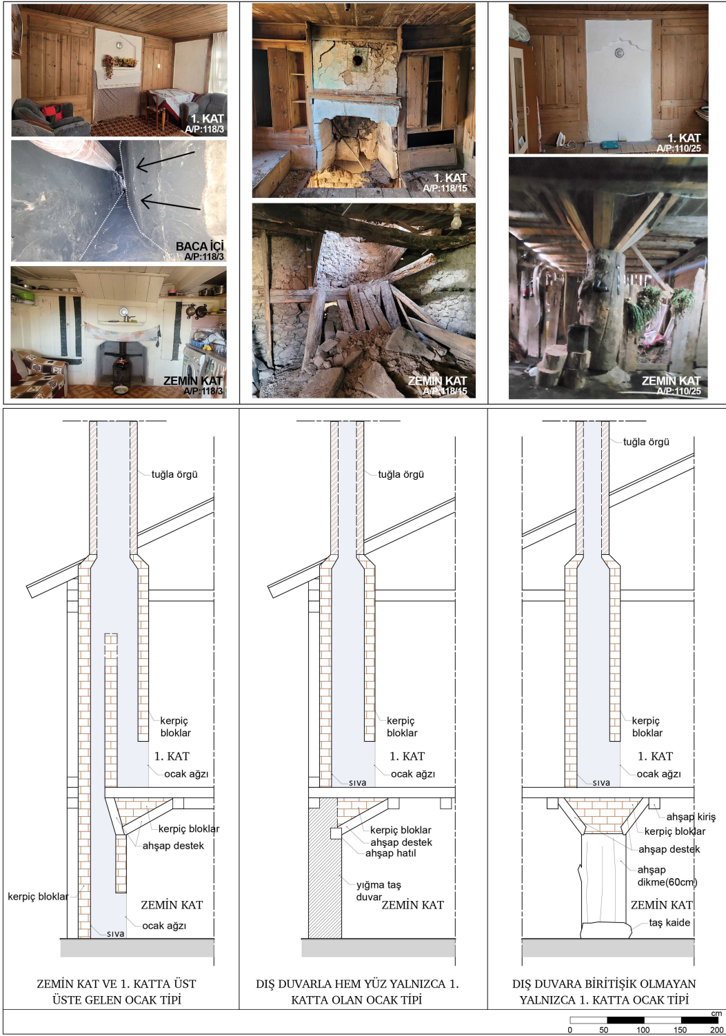
Şekil 5.28 Devecören Köyü’nde üç farklı taşıma sistemi uygulanan ocaklar tipleri (Ç:V.O., 2023)
