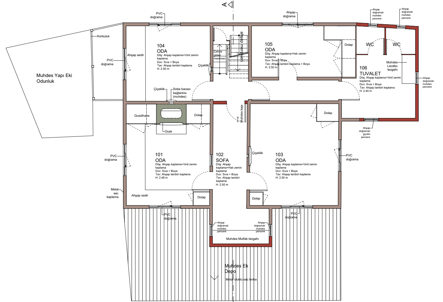
1. KAT PLANI
