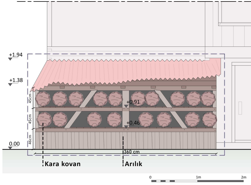
Şekil 5.24 Parsel 118, ada 16'daki arılık yapısı ve kara kovanlar (Ç:V.O., 2022)
