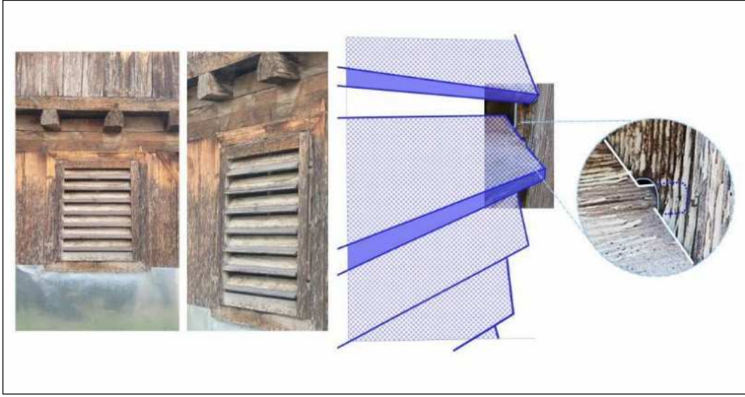
Şekil 5.46 Yapı Ustası M. E.'in evinde kendi yaptığı ahşap hareketli panjur (Ç:V.O, 2022)
