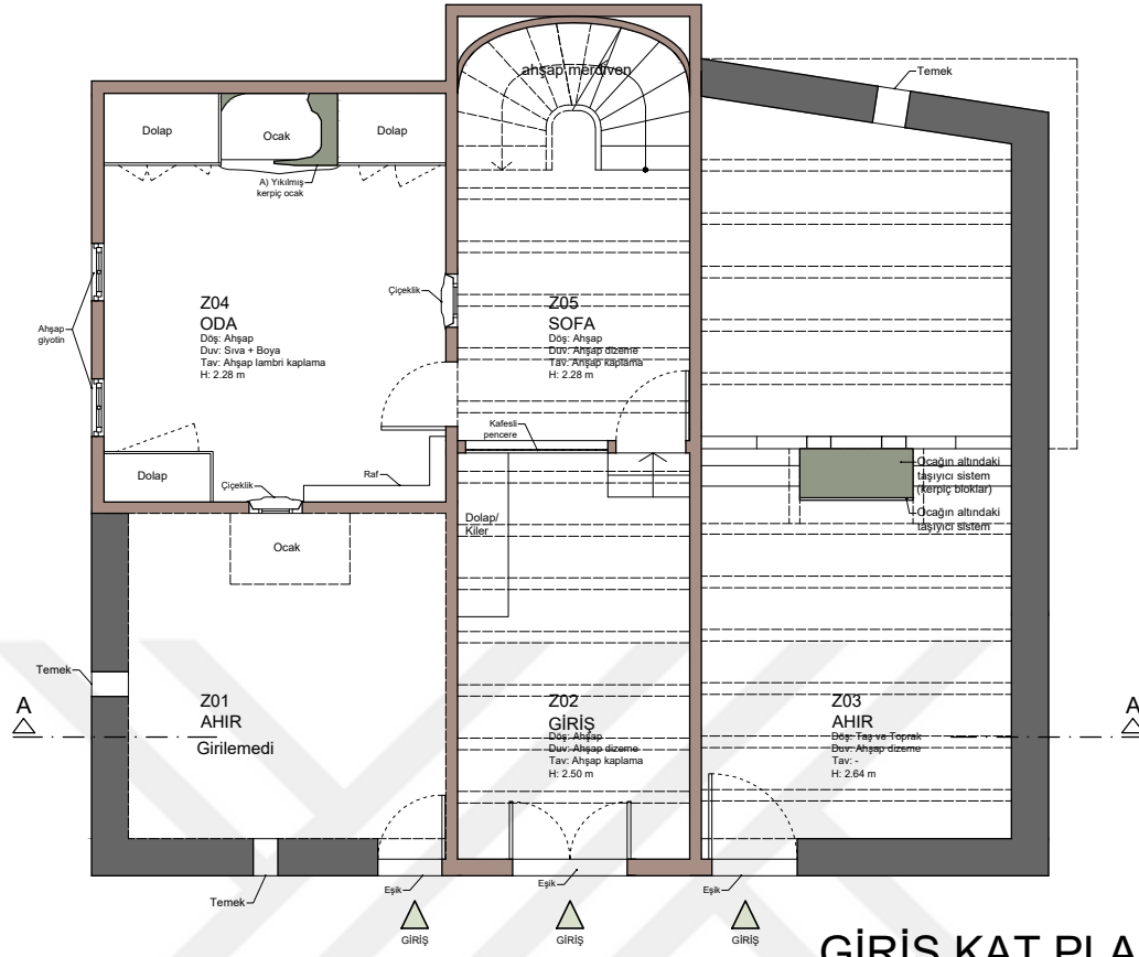
GİRİŞ KAT PLANI
