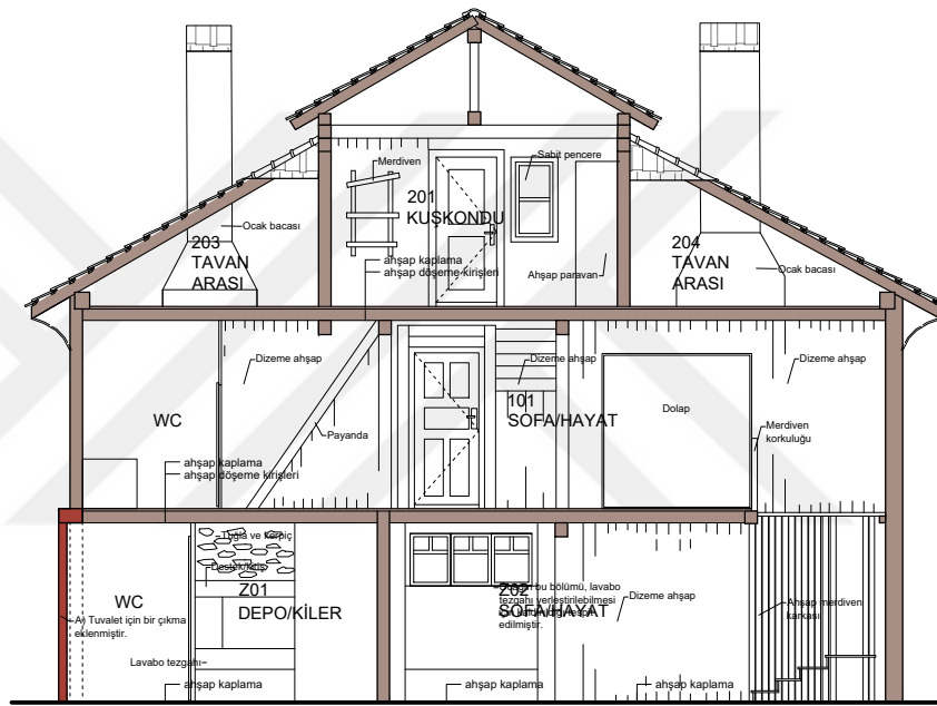
A-A KESİTİ
