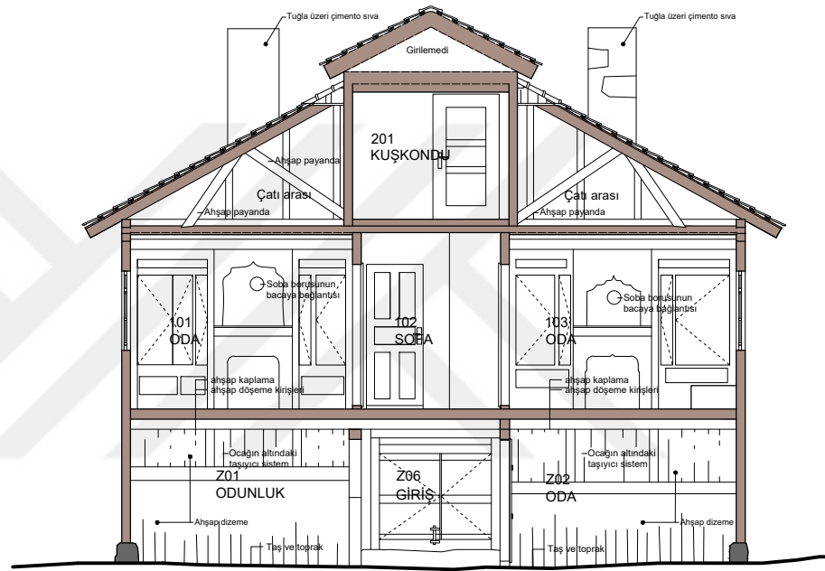
A-A KESİTİ
