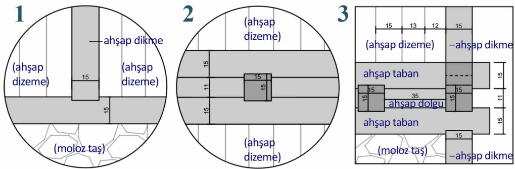
Şekil 5.64 Deveören Köyü geleneksel konutunda yapım tekniği sistemi (Ç:V.O., 2023)
