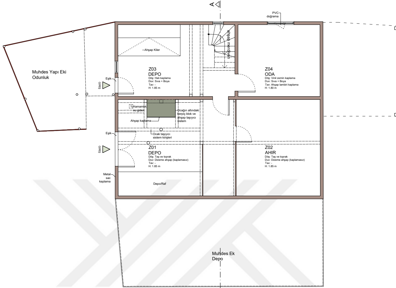
GİRİŞ KAT PLANI
