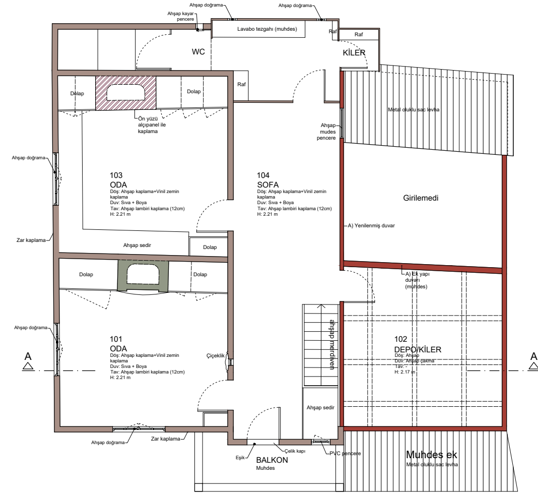
1. KAT PLANI
