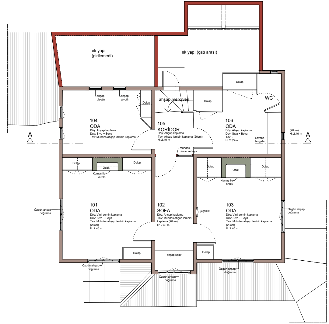
1. KAT PLANI
