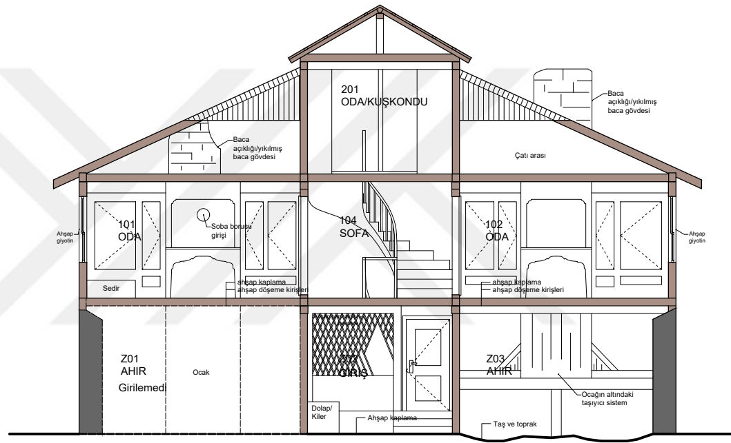
A-A KESİTİ
