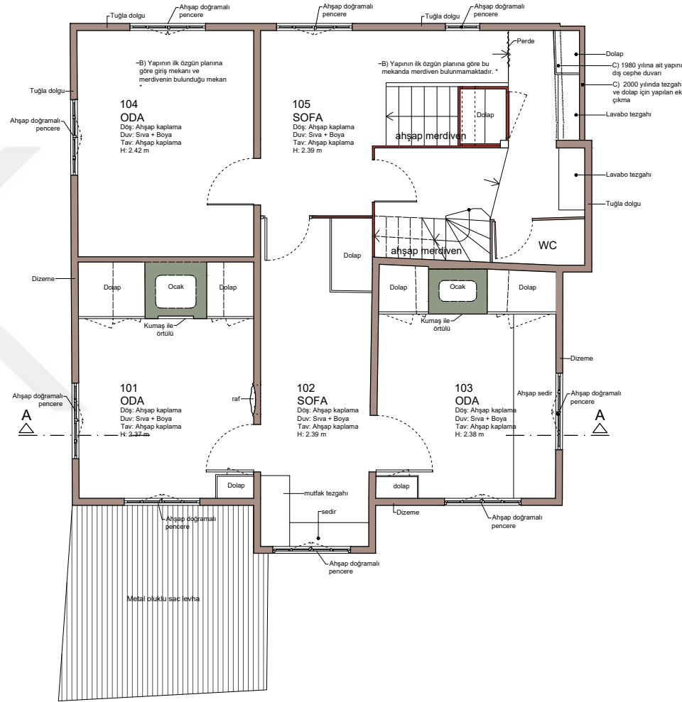
1. KAT PLANI
