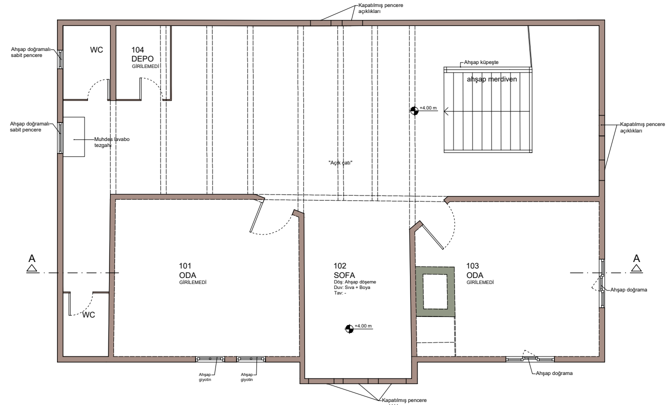
1. KAT PLANI
