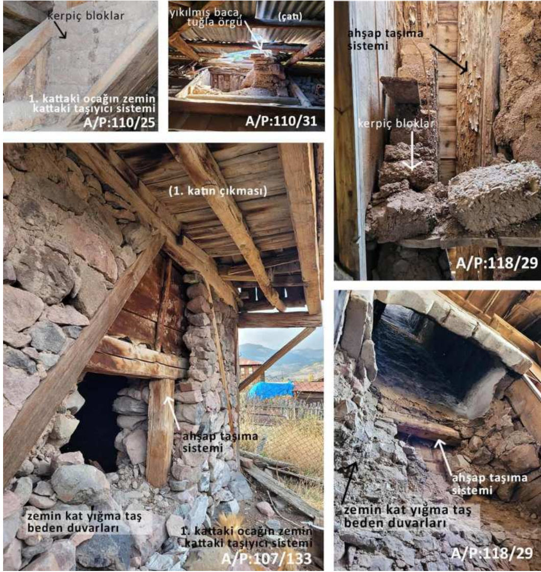
Şekil 5.27 Ocaklarda kullanılan yapı malzemeleri (2023)
