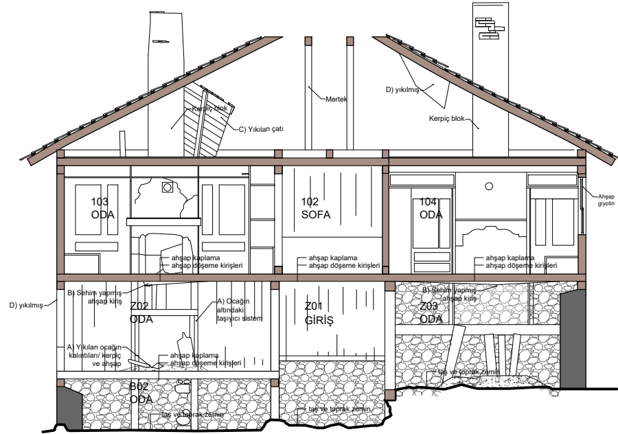
A-A KESİTİ
