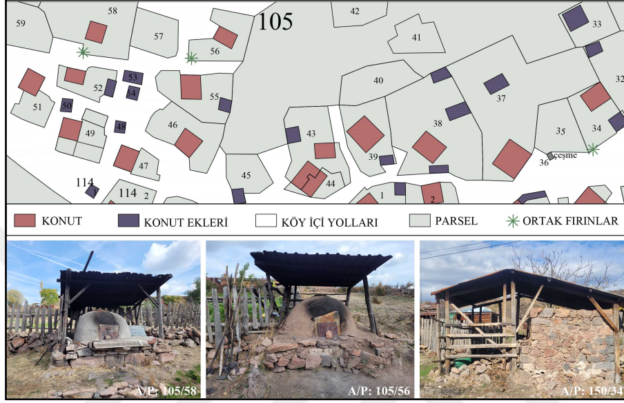
Şekil 5.6 Köyde bulunan ortak fırın krokisi ve örnekleri. Ada/Parsel sırasıyla: 105/58, 105/56, 105/34 (Ç:V.O., 2022)
