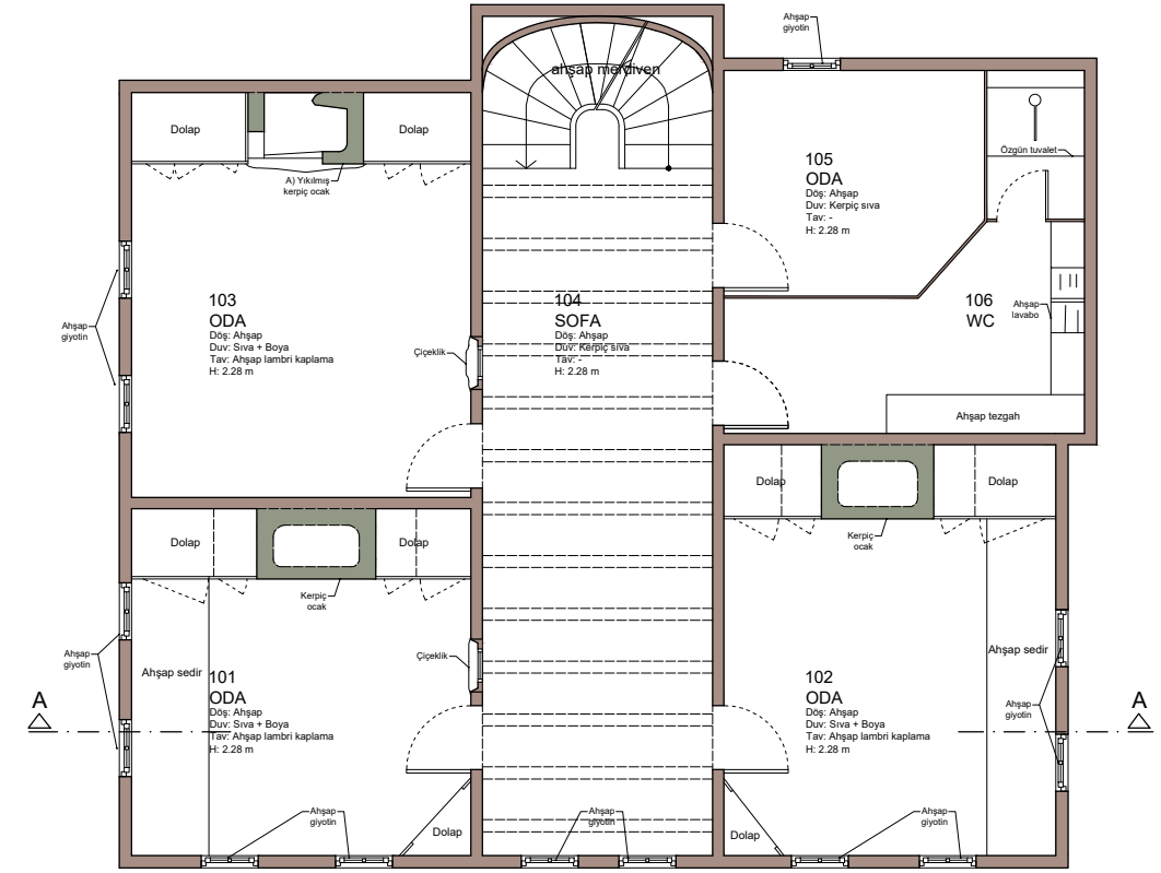
1. KAT PLANI
