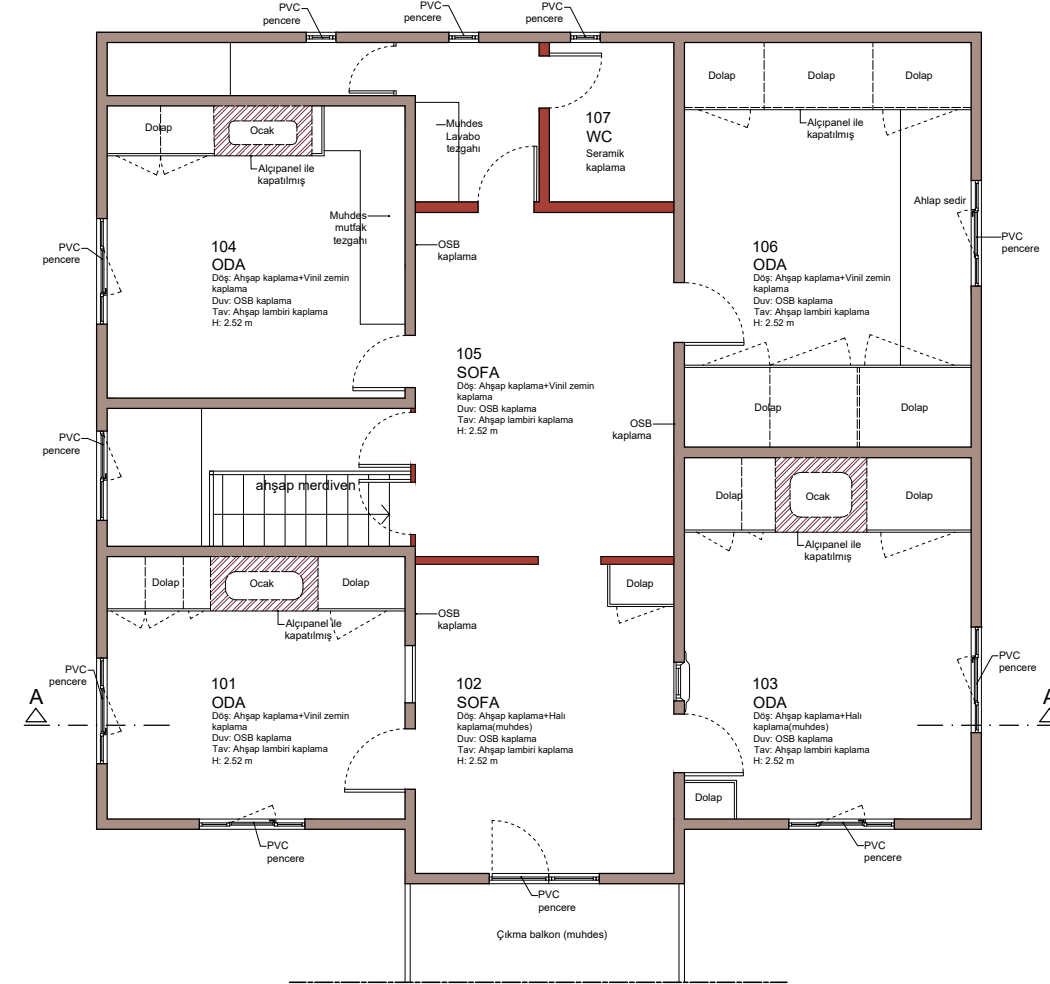
1. KAT PLANI
