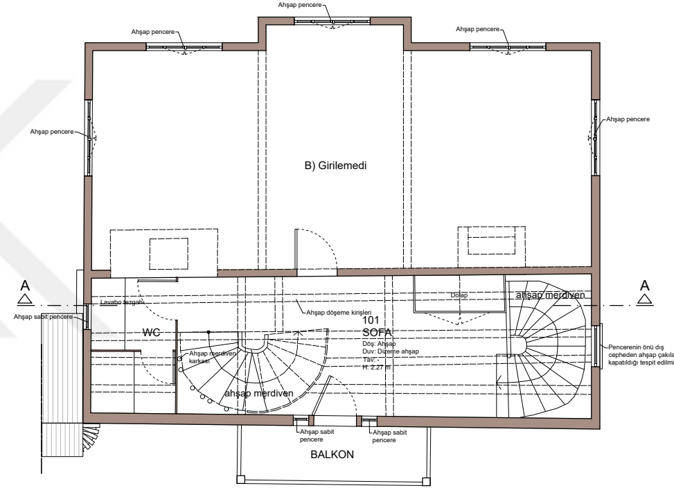
1. KAT PLANI
