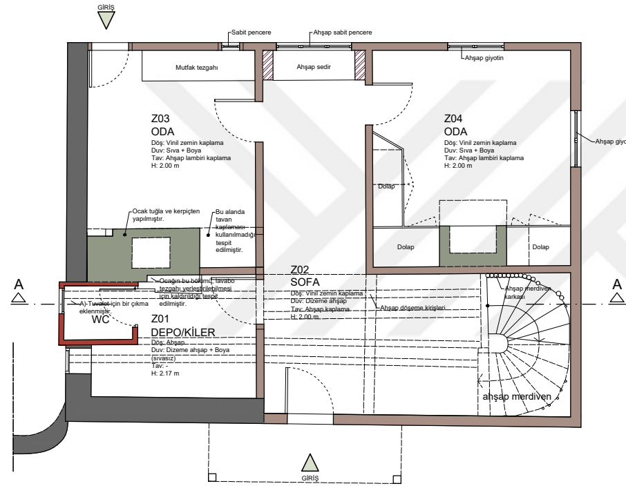
GİRİŞ KAT PLANI
