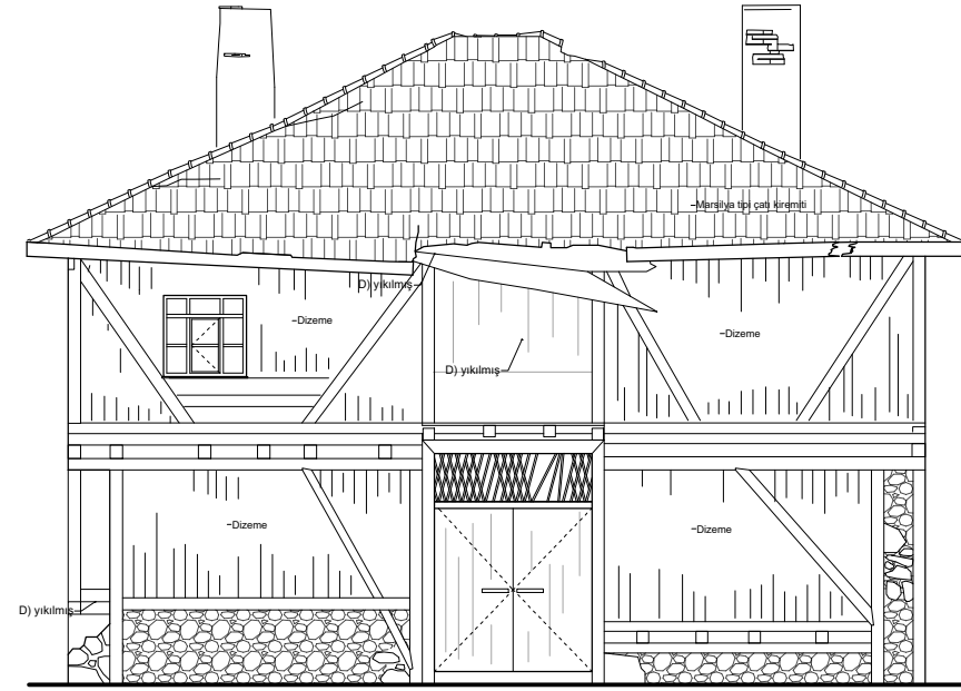
DOĞU CEPHESİ
