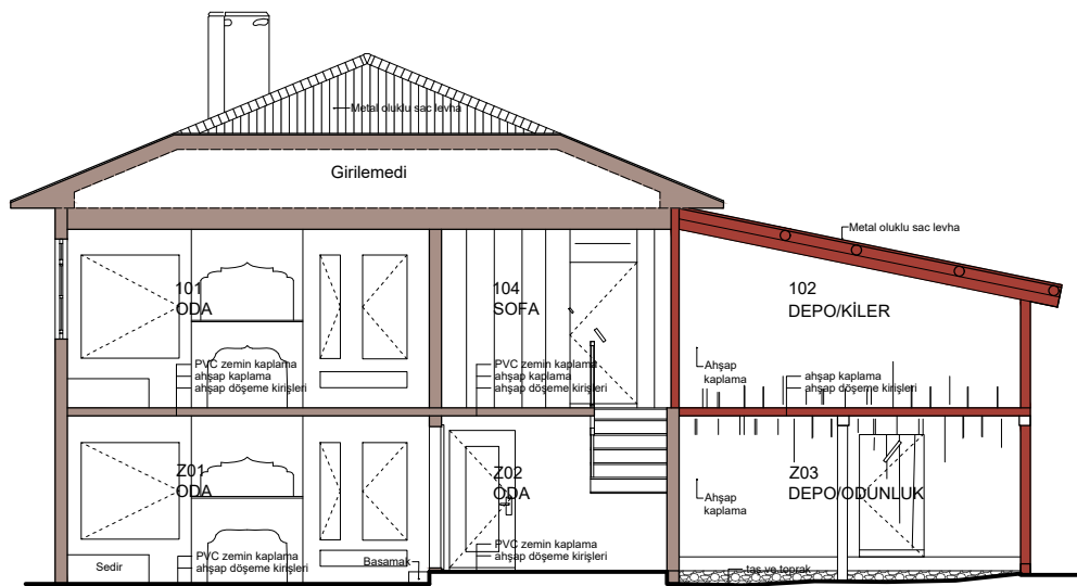
A-A KESİTİ
