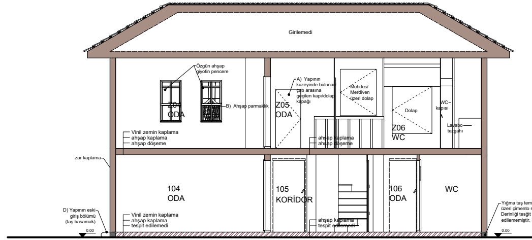
A-A KESİTİ
