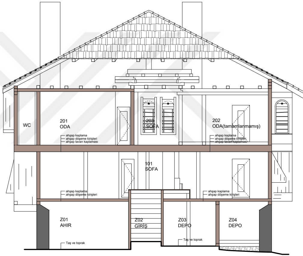
A-A KESİTİ
