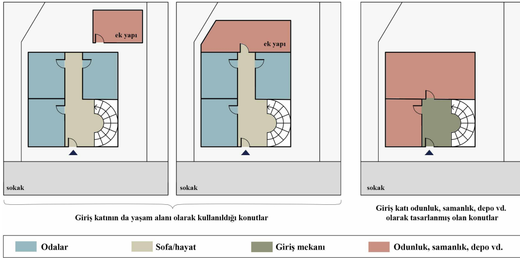
Şekil 5.8 Yapı-parsel-ek yapı ilişkileri (Ç:V.O, 2023)
