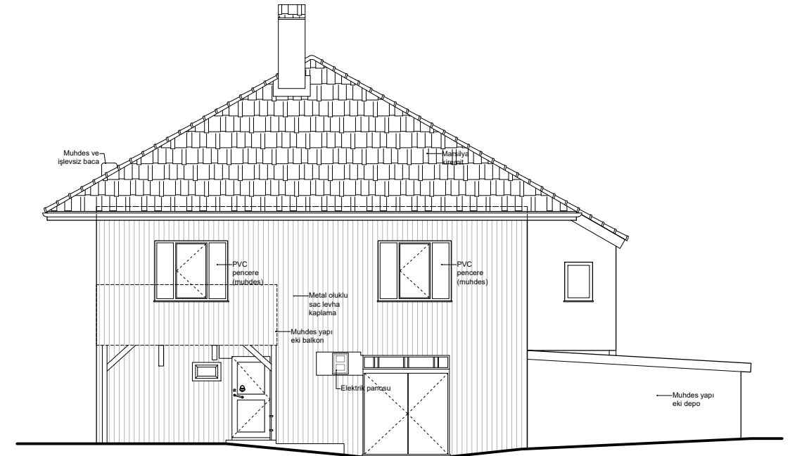
BATI CEPHESİ
