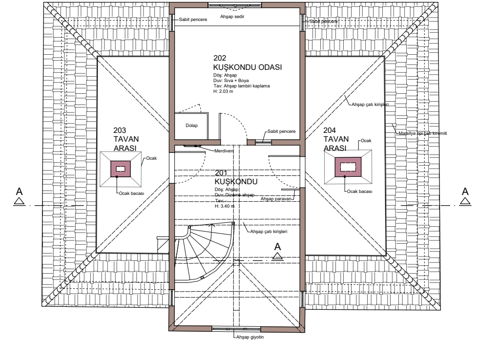
2. KAT(KUŞKONDU) PLANI
