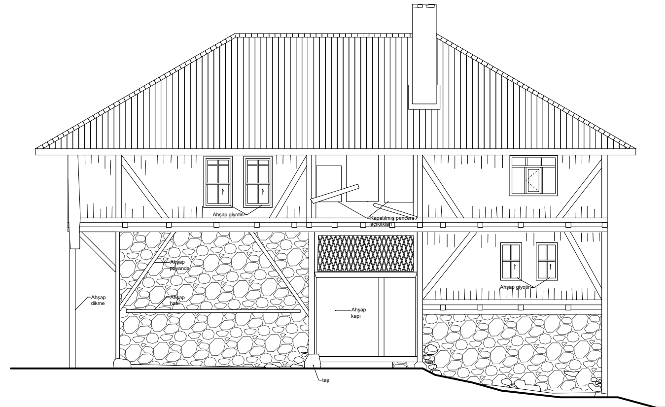
BATI CEPHESİ
