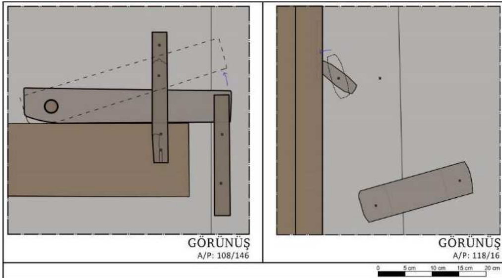
Şekil 5.40 İç mekândaki ahır kapılarının ahşap kilit sistemleri (Ç:V.O., 2022)
