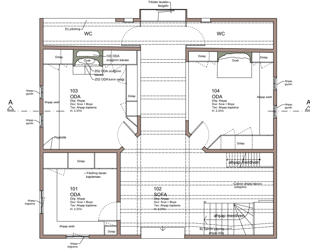
1. KAT PLANI
