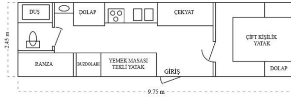
Şekil 25: Geçici römork planı (Browne, 2015)
