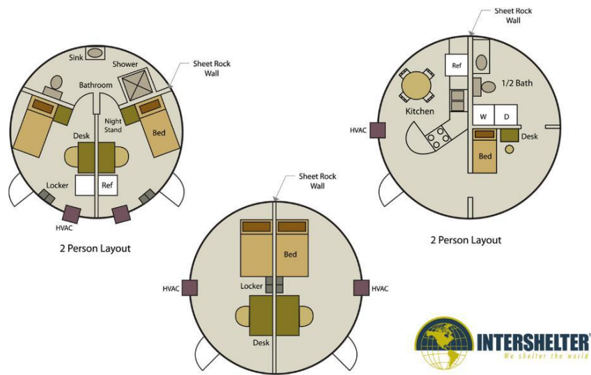
Şekil 33: Intershelter İç Plan Tasarımları 1 (Url-27)
