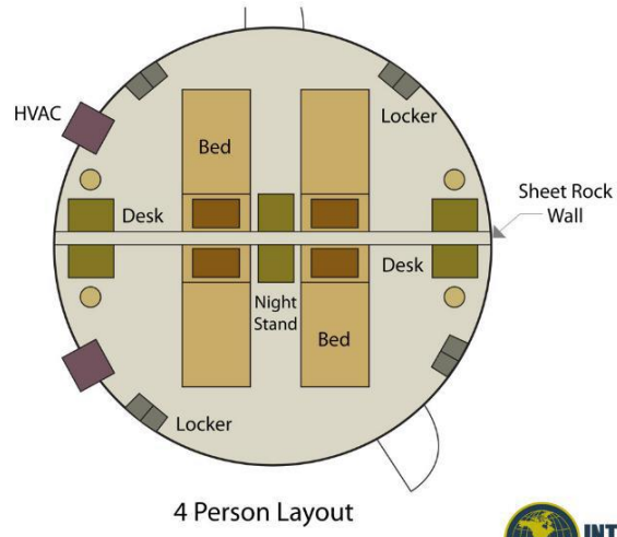
Şekil 34: . Intershelter İç Plan Tasarımları (URL-28)
