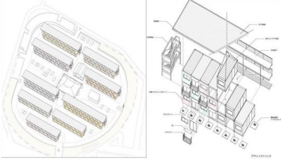
Şekil 20: Japonya geçici konteyner konutlarının aksometrik vaziyet planı ve düşey yerleşim (Url-19)
