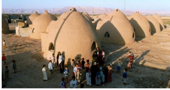
Şekil 28: Sandbag barınakları dış mekan görünümü (Url-7).
