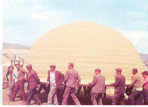
Şekil 27: 1970 Kütahya-Gediz Depreminde kullanılan bayer köpük konut birimi (Url-6)
