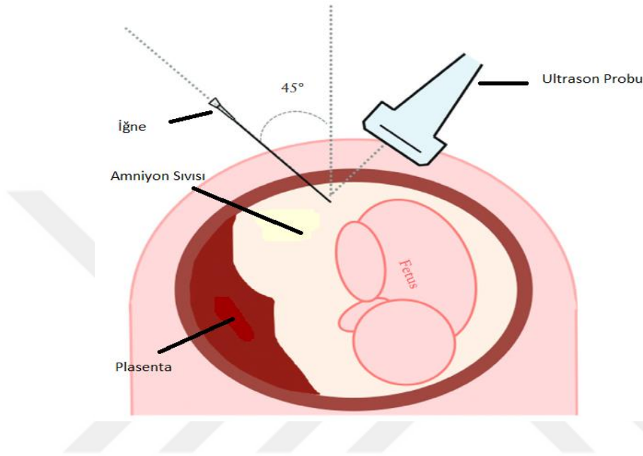
Şekil 2.4. Amniyosentez (AS) işlemi transabdominal (Cruz-Lemini vd., 2014)
