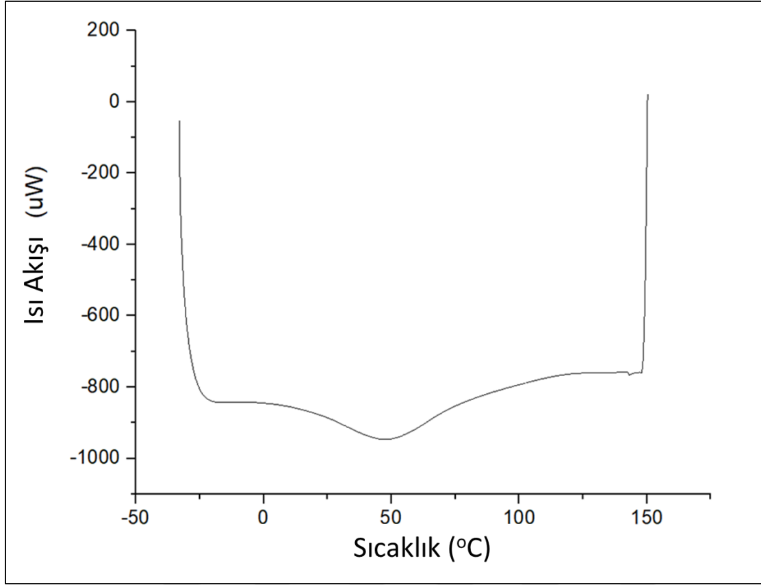
Şekil 5.21. 1125 °C’de 1 saat sinterlenen gözenekli NiTi numunenin ısıtma DSC analizi
