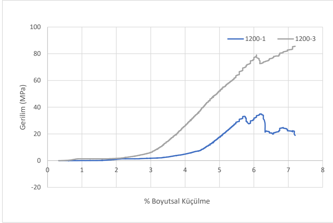
Şekil 5.28. 1200 C’de 1 saat sinterlenen gözenekli NiTi numunenin basma eğrisi
