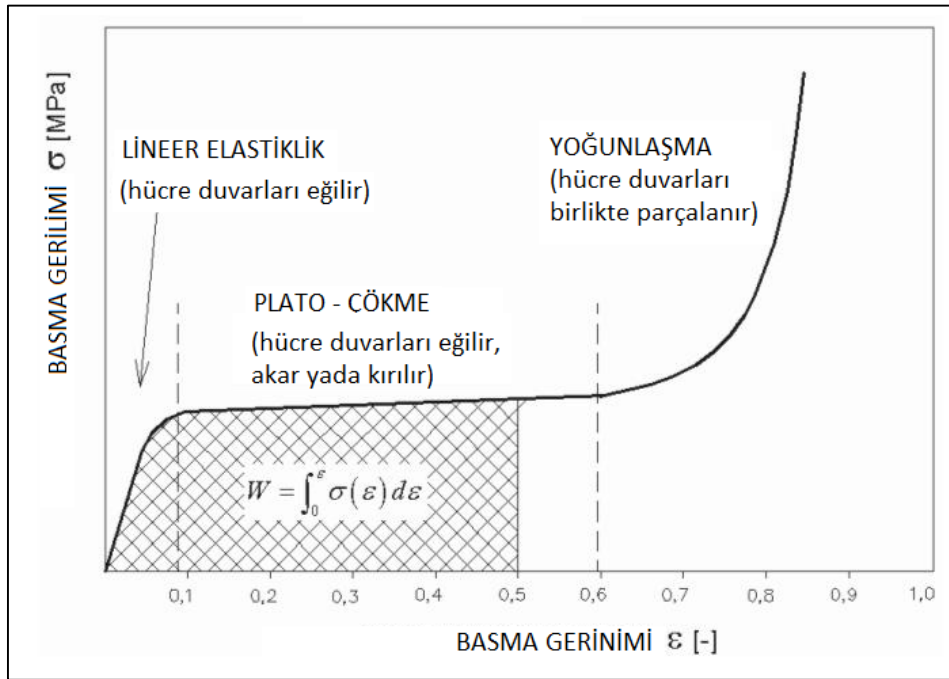
Şekil 3.4. Açık hücreli bir köpükte tipik bir gerilim-gerinim eğrisi örneği [84].
