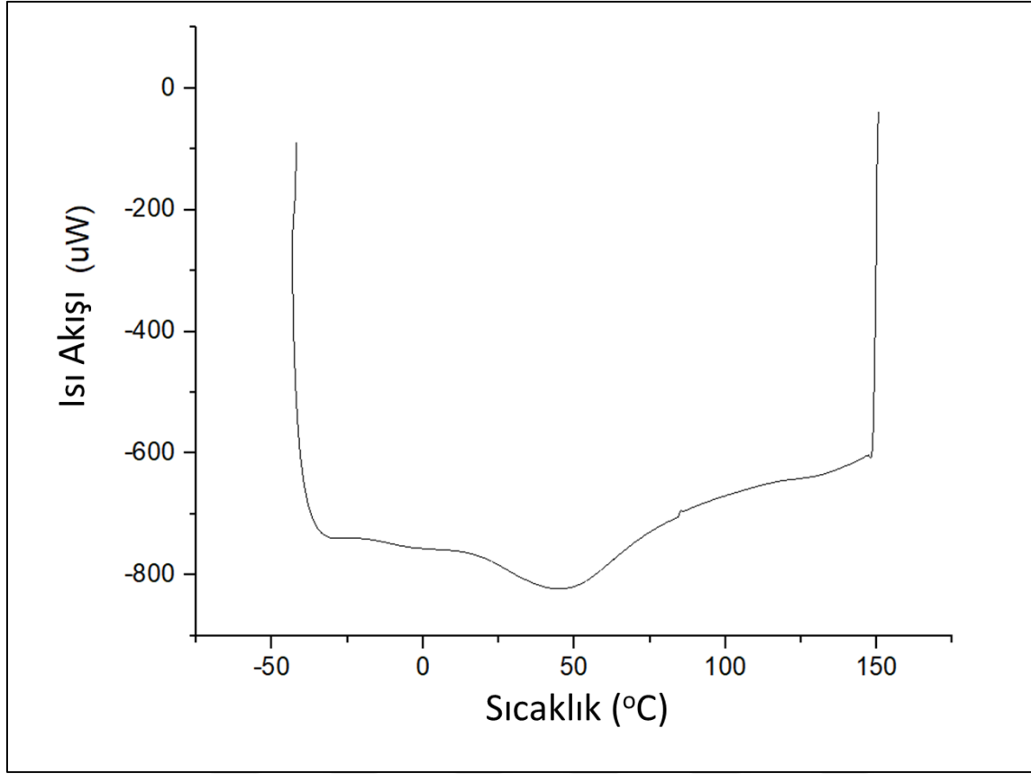
Şekil 5.23. 1200 °C’de 1 saat sinterlenen gözenekli NiTi numunenin ısıtma DSC analizi
