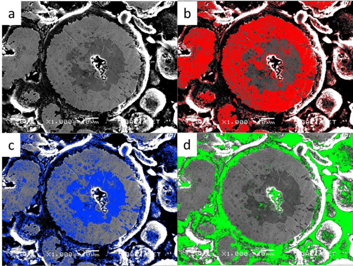
Resim 5.13. 1125 °C’de 1 saat sinterleme sonrası numunenin SEM analizlerinde belirlenen fazları a) NiTi SEM görüntüsü, b) Ni-zengin faz, c) NiTi fazı ve d) Ti-zengin faz
