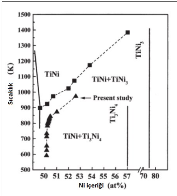
Şekil 2.6. NiTi fazı ile meta kararlı \text{Ni}_4\text{Ti}_3 çökeltisi arasındaki ön faz diyagramı [46,47].
