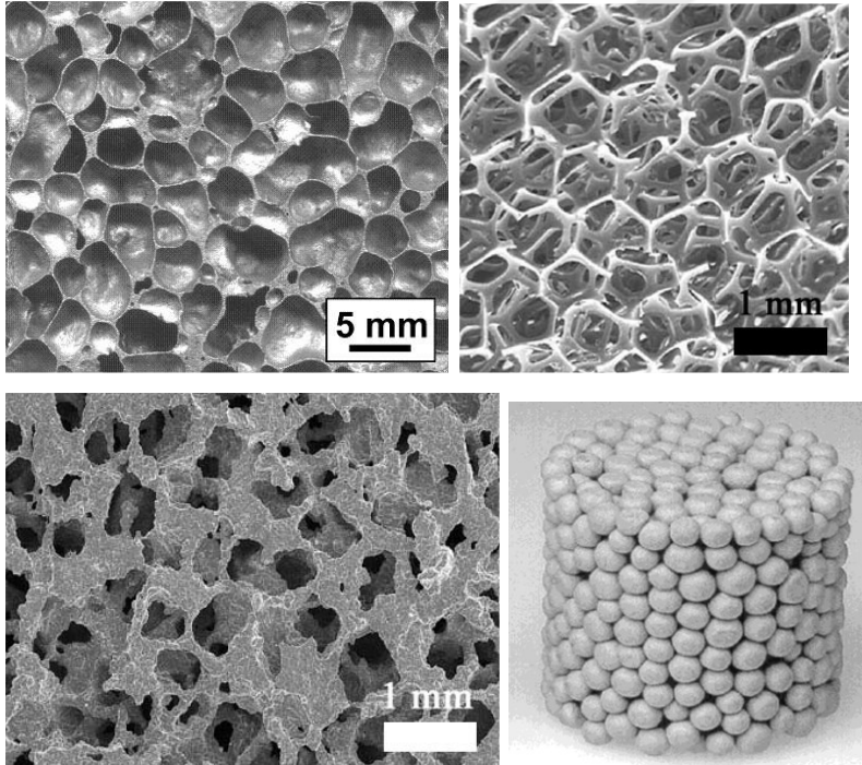
Resim 3.2. a) TiH 2 'nin erimiş alüminyum içinde parçalanmasıyla yapılan kapalı hücreli köpük, b) düşük yoğunluklu açık hücreli poliüretan köpük [84], c) yüksek yoğunluklu açık hücreli NiTi köpük ve d) içi boş paslanmaz çelik kürelerden oluşan bir yatağın sinterlenmesiyle yapılan karışık açık ve kapalı hücreler [85].
