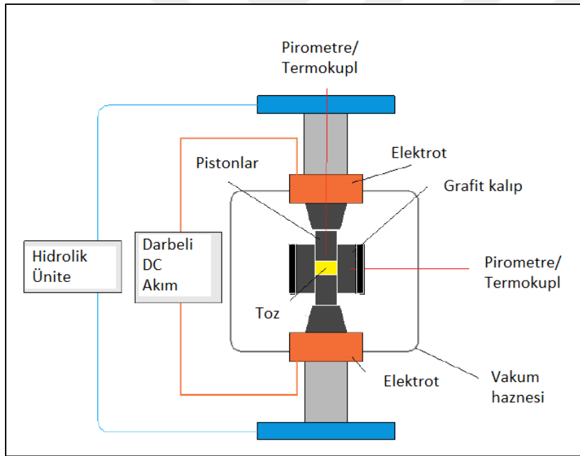
Şekil 3.9. SPS yönteminin şematik gösterimi [95]
