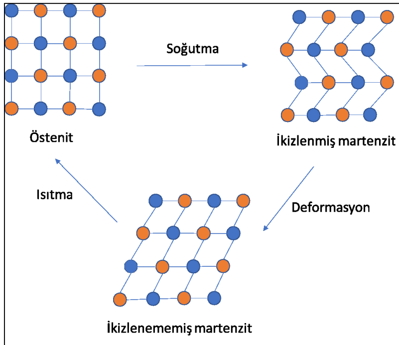
Şekil 2.4. Şekil bellek etkisinin şematik açıklaması [43]
