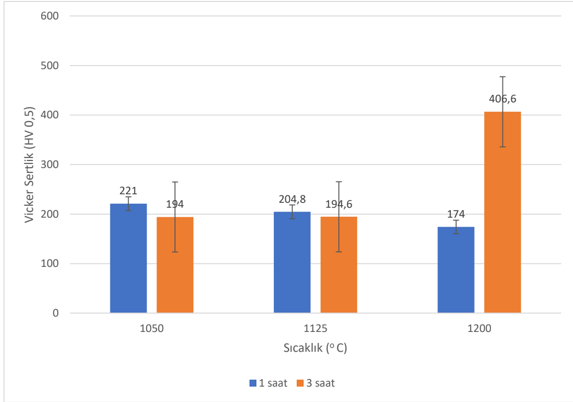
Şekil 5.25. Gözenekli NiTi numunelerin sertlik değerleri
