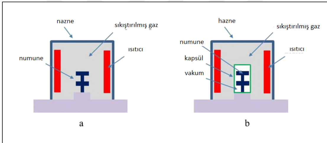
Şekil 3.10. HIP yönteminin şematik gösterimi a) kapsülsüz, b) kapsüllü yöntem [97]
