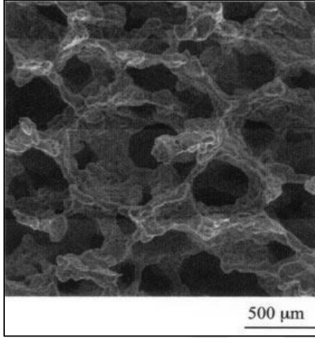
Resim 3.1. Gözenekli metal yapının tipik karakteristiğini gösteren SEM görüntüsü[76]
