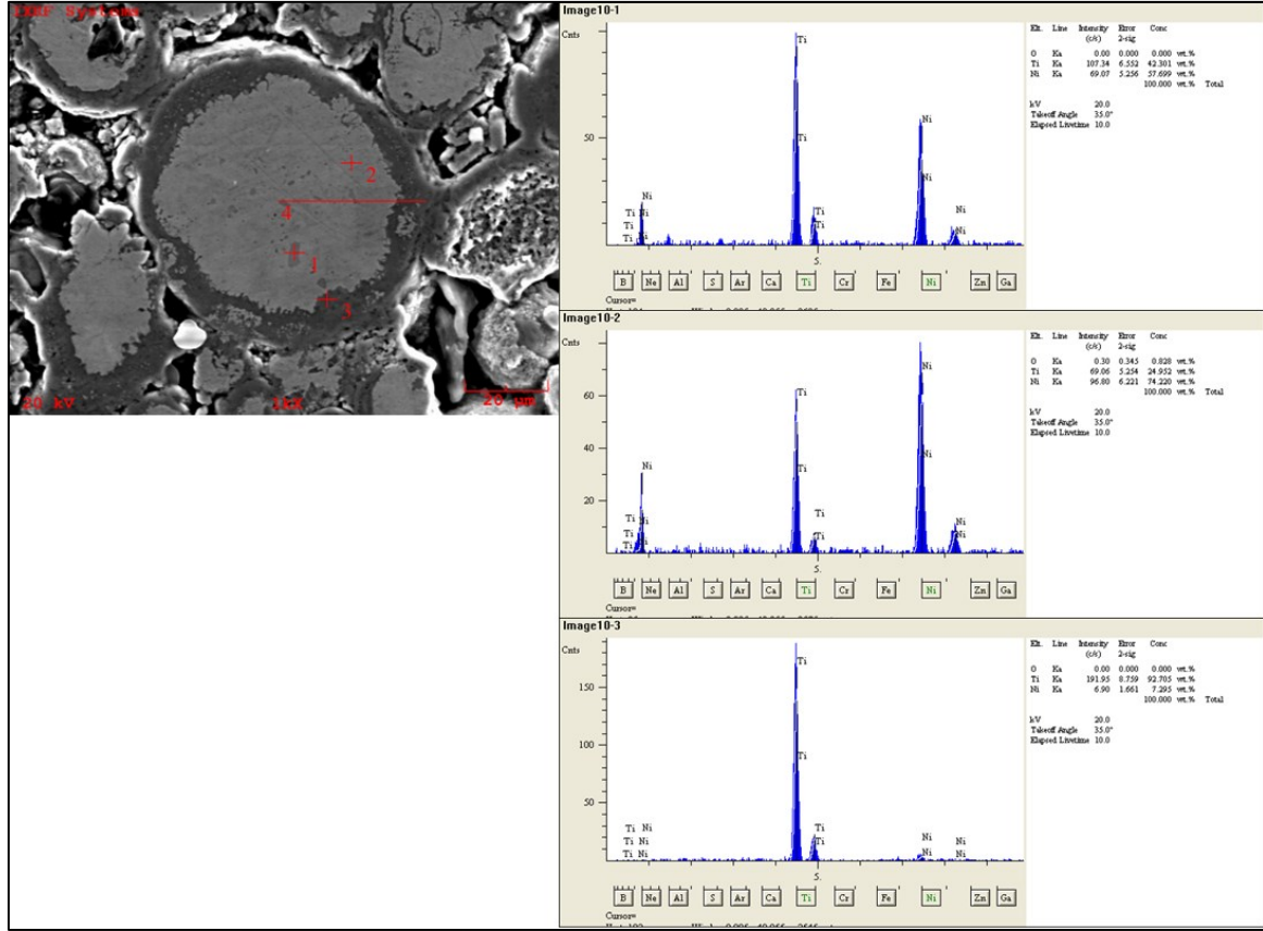
Şekil 5.4. 1050 °C de 3 saat sinterlenen gözenekli NiTi numunenin noktasal EDS analizleri
