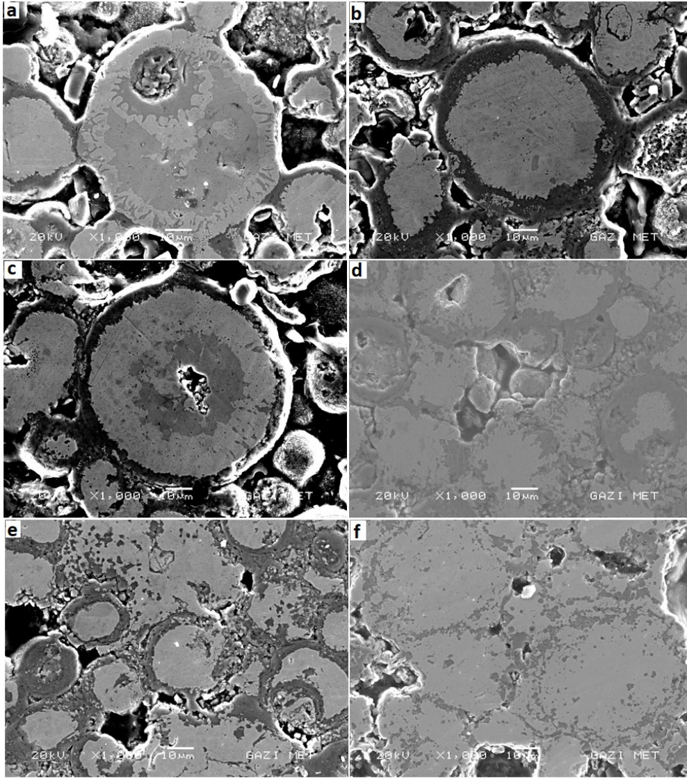
Resim 5.10. Gözenekli NiTi numunelerin 1000x SEM görüntüleri a) 1050 °C, 1 saat sinterleme, b) 1050 °C, 3 saat, c) 1125 °C, 1 saat, d) 1125 °C, 3 saat, e) 1200 °C, 1 saat, f) 1200 °C, 3 saat
