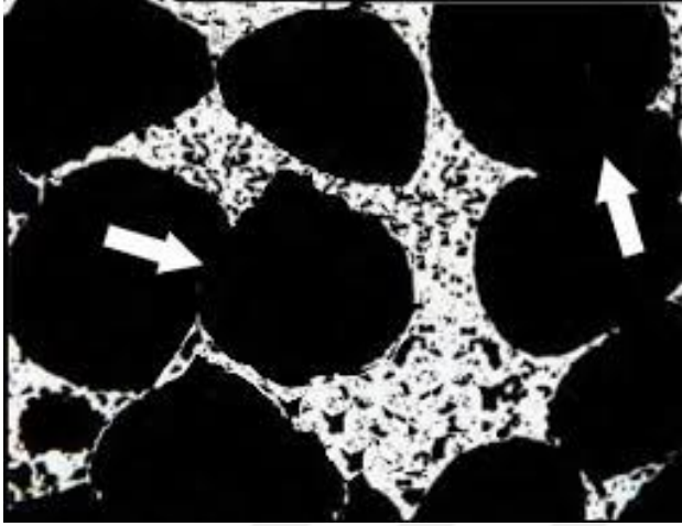
Resim 3.3. Sıkışmış argon gazının genişmesiyle işlenen, küçük pencere boyutuna sahip bir NiTi köpük örneği. Gözenekler arasındaki pencereler oklarla gösterilmiştir [6].
