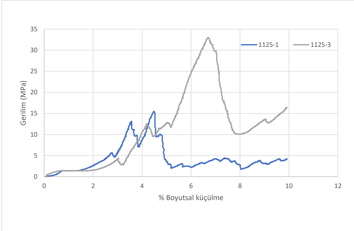
Şekil 5.27. 1125 °C’de 1 saat sinterlenen gözenekli NiTi numunenin basma eğrisi
