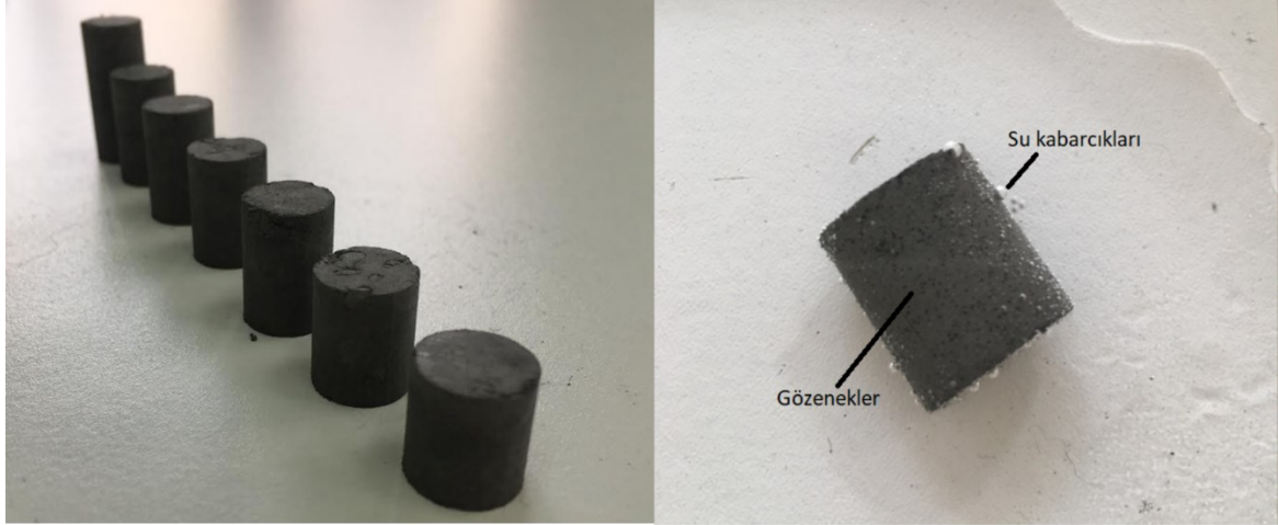
Resim 4.2. a) Suda çözündürme işlemi öncesi ve b) çözündürme işlemi sırasında gözenekli NiTi numunelerinin görüntüsü
