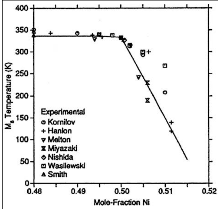
Şekil 2.7. Ni içeriğine göre dönüşüm sıcaklıklarını gösteren grafik[49]
