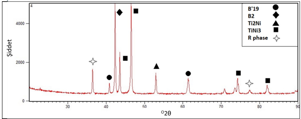
Şekil 5.11. 1125 °C de 1 saat sinterlenen gözenekli NiTi numunenin XRD analizi
