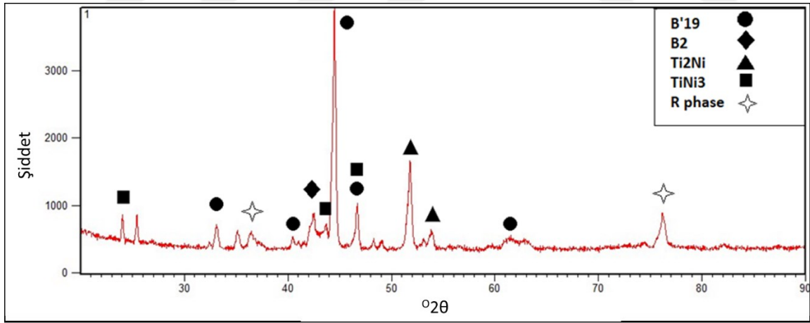
Şekil 5.10. 1050 °C de 3 saat sinterlenen gözenekli NiTi numunenin XRD analizi
