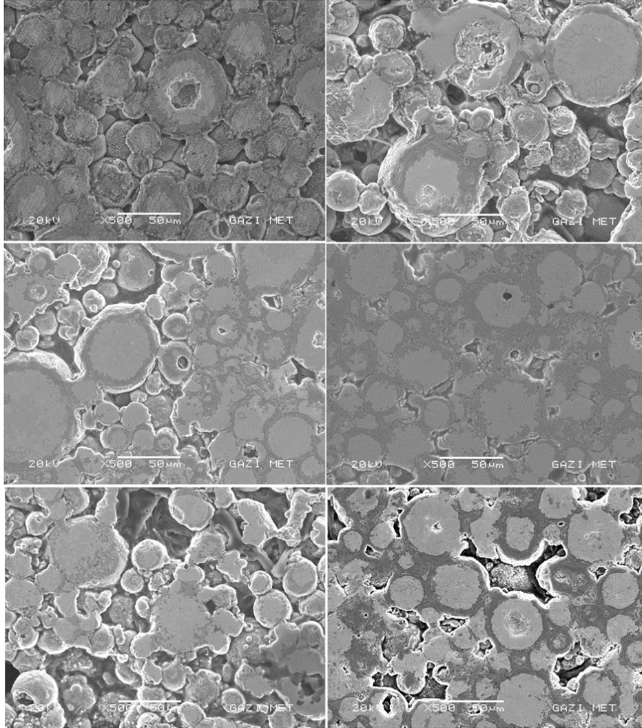
Resim 5.9. Gözenekli NiTi numunelerin 500x SEM görüntüleri a) 1050 °C, 1 saat sinterleme, b) 1050 °C, 3 saat, c) 1125 °C, 1 saat, d) 1125 °C, 3 saat, e) 1200 °C, 1 saat, f) 1200 °C, 3 saat
