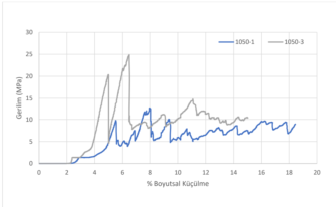
Şekil 5.26. 1050 °C’de 1 ve 3 saat sinterlenen gözenekli NiTi basma eğrisi
