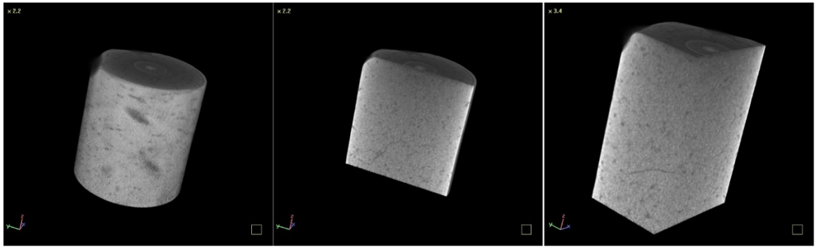
Şekil 5.17. 1250 °C de 3 saat sinterlenen numunenin mikro bilgisayarlı tomografi analizi
