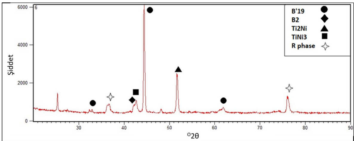
Şekil 5.14. 1200 °C de 3 saat sinterlenen gözenekli NiTi numunenin XRD analizi
