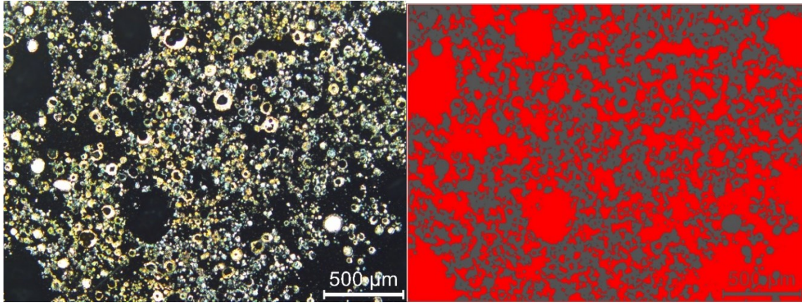
Resim 5.6. 1200 °C’de 1 saat sinterlenen gözenekli NiTi numunenin optik mikroskop ve gözenek yapısı görüntüleri
