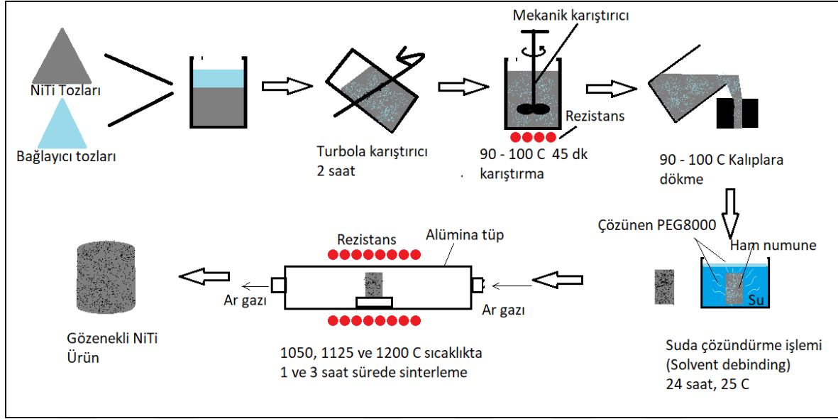
Şekil 4.2. Gözenekli NiTi numunelerin üretiminin şeması
