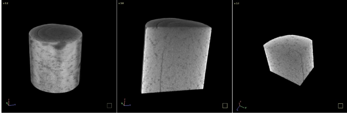
Şekil 5.16. 1125 °C de 3 saat sinterlenen numunenin mikro bilgisayarlı tomografi analizi
