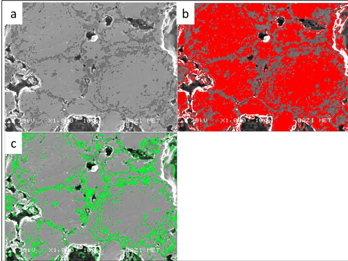
Resim 5.16. 1200 °C’de 3 saat sinterleme sonrası numunenin SEM analizlerinde belirlenen fazları a) NiTi SEM görüntüsü, b) Ni-zengin faz, c) Ti-zengin faz
