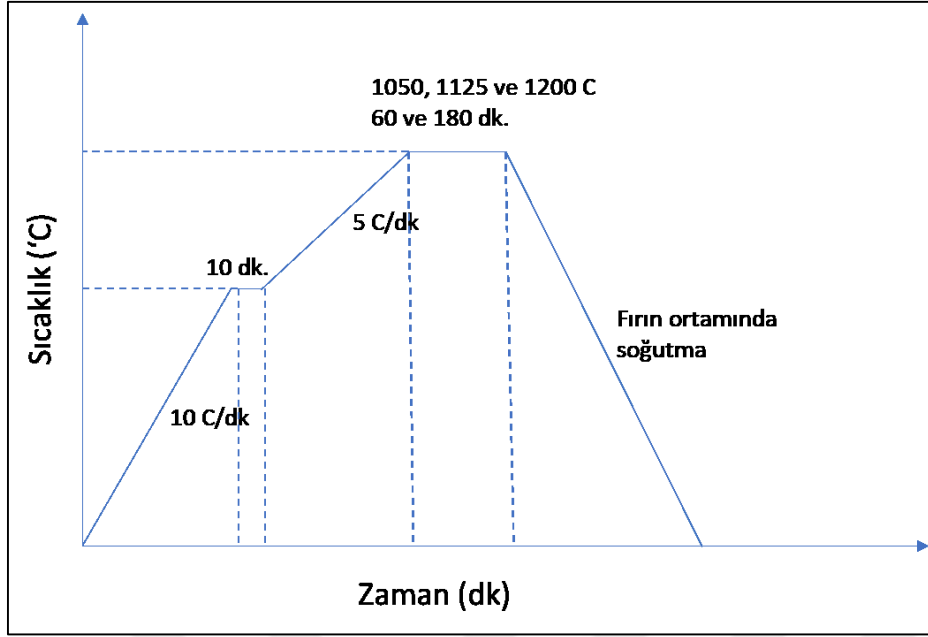
Şekil 4.3. Gözenekli NiTi numunelerinin sinterleme aşamalarının şematik gösterimi
