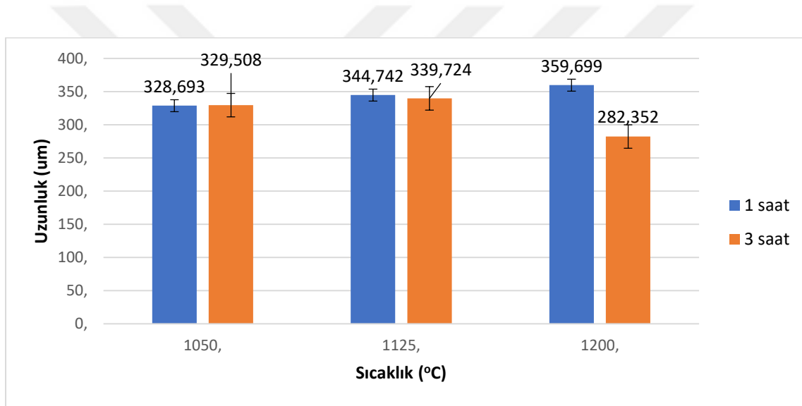
Şekil 5.1. Üretilen gözenekli NiTi alaşımlarının gözenek boyutlarının grafiği
