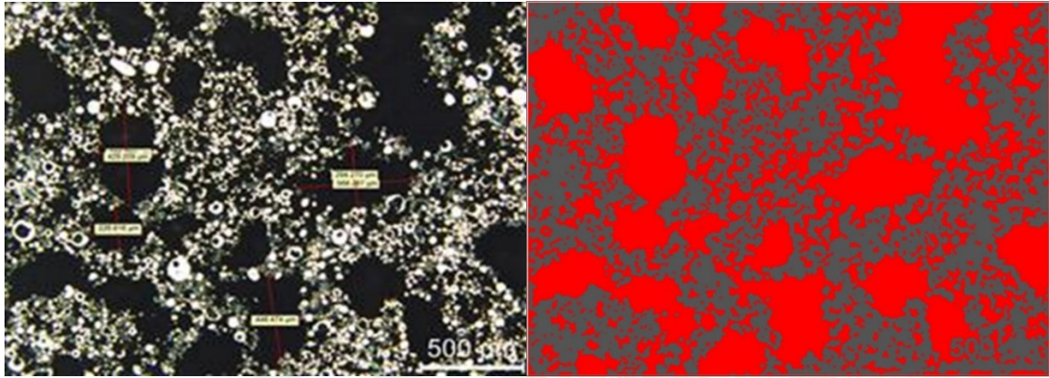
Resim 5.3. 1050 °C’de 3 saat sinterlenen gözenekli NiTi numunenin optik mikroskop ve gözenek yapısı görüntüleri
