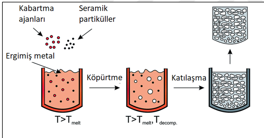
Şekil 3.6. Direk köpürtme işleminin şematik gösterimi [88]
