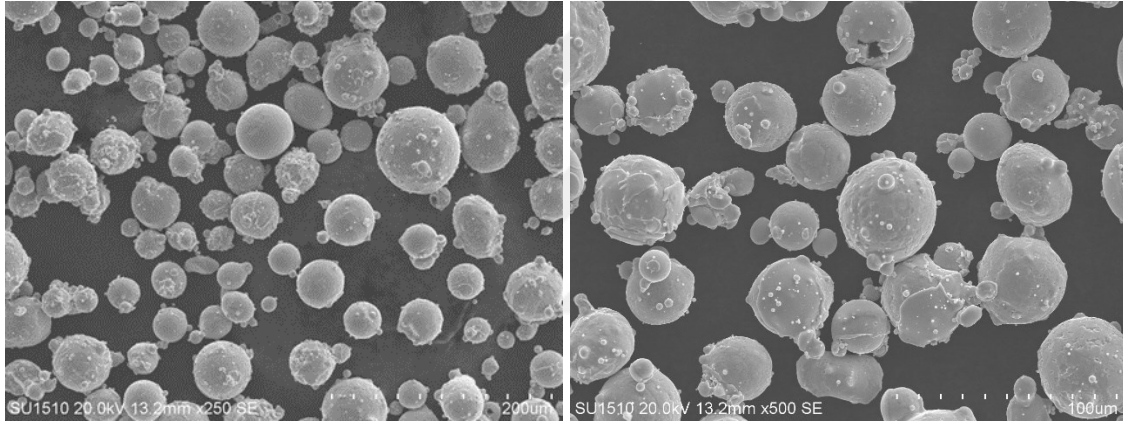
Resim 4.1. Ortalama 34 \mu\text{m} boyutunda ön alaşımlı NiTi tozlarının SEM görüntüsü
