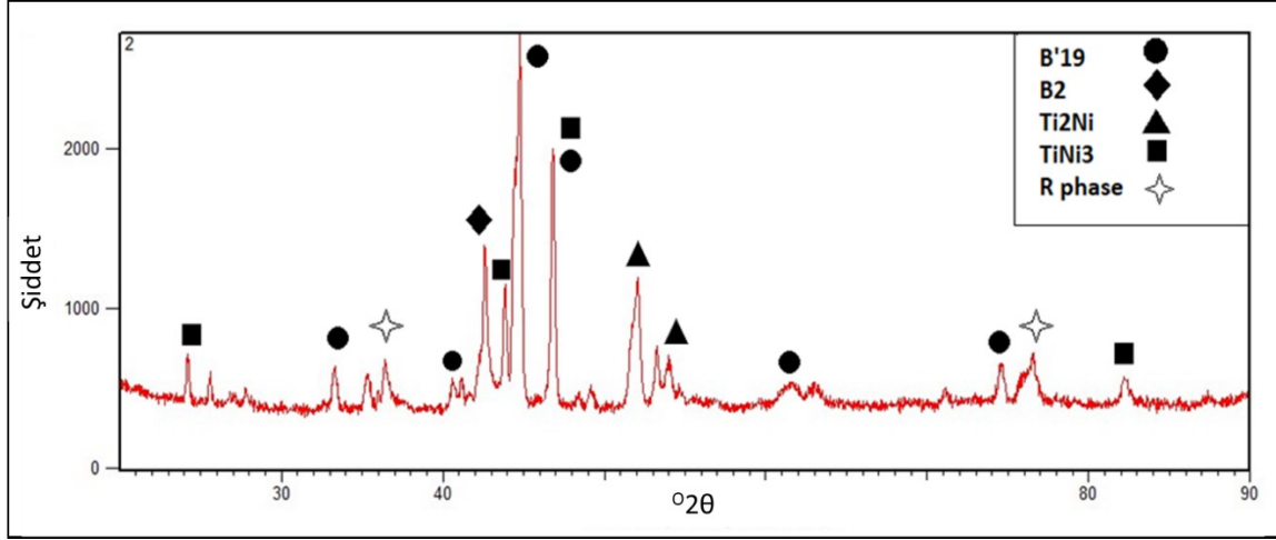
Şekil 5.9. 1050 °C de 1 saat sinterlenen gözenekli NiTi numunenin XRD analizi
