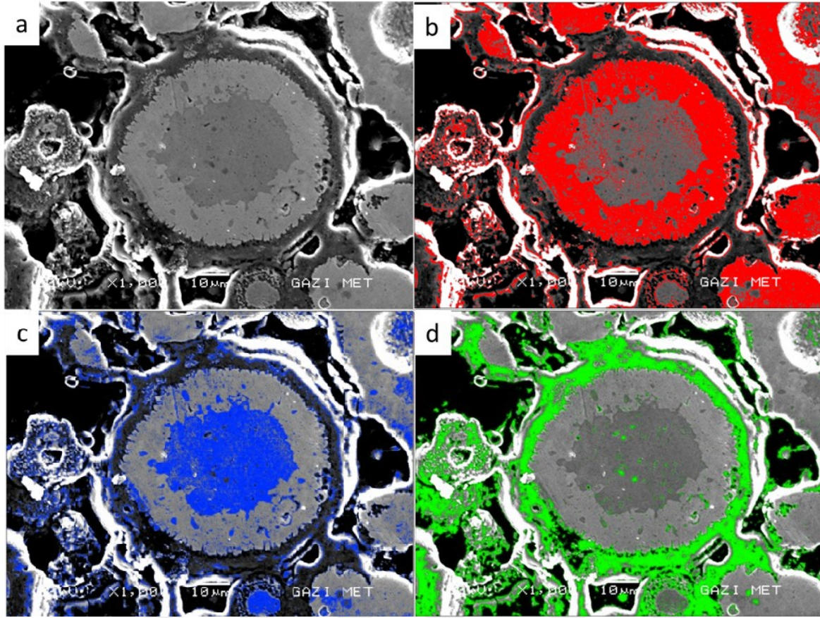
Resim 5.11. 1050 °C’de 1 saat sinterleme sonrası numunenin SEM analizlerinde belirlenen fazları a) NiTi SEM görüntüsü, b) Ni-zengin faz, c) NiTi fazı ve d) Ti-zengin faz
