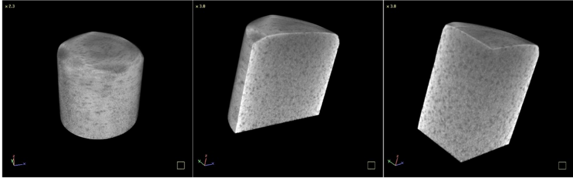
Şekil 5.15. 1050 C'de 1 saat sinterlenen numunenin mikro bilgisayarlı tomografi görüntüsü
