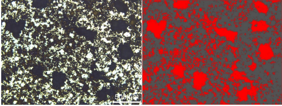
Resim 5.7. 1200 °C'de 3 saat sinterlenen gözenekli NiTi numunenin optik mikroskop ve gözenek yapısı görüntüleri
