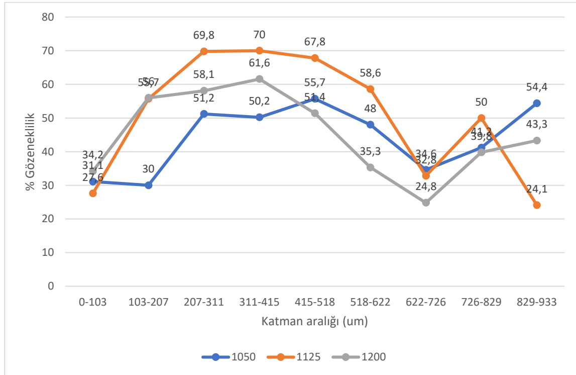
Şekil 5.18. 3 saat sinterlenmiş numunelerin 103 µm aralıklı katmanlarında gözenek oranının incelenmesi
