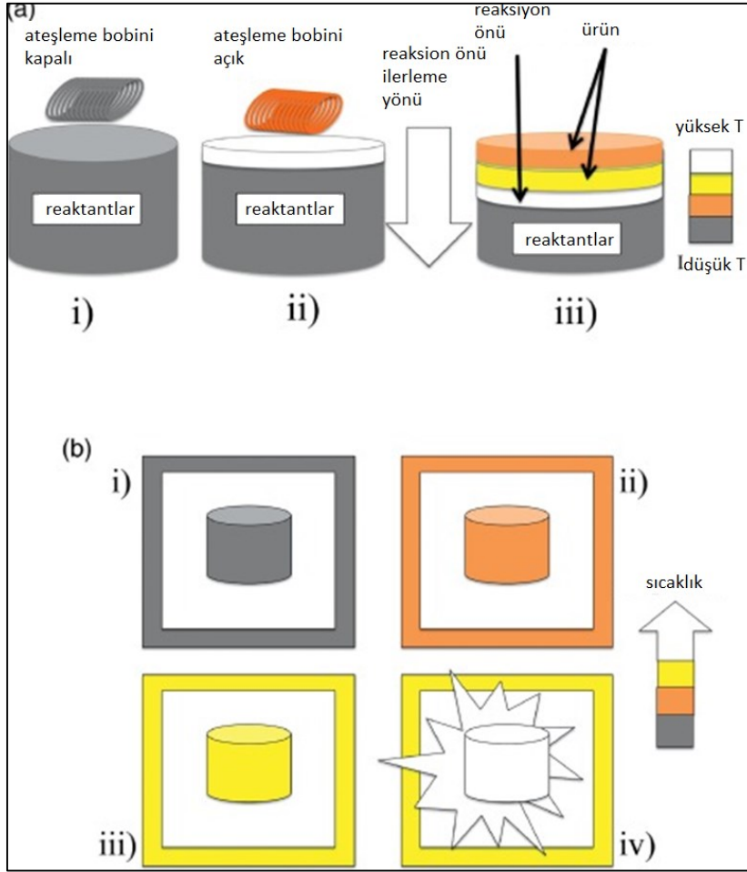
Şekil 3.8. SHS yönteminin şematik gösterimi a) yanma dalgası modu, b) patlama modu [93]
