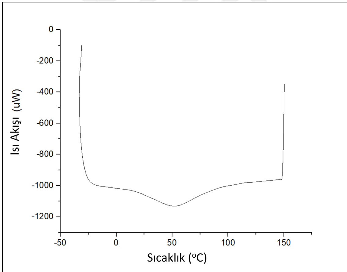
Şekil 5.19. 1050 °C’de 1 saat sinterlenen gözenekli NiTi numunenin ısıtılma DSC analizi
