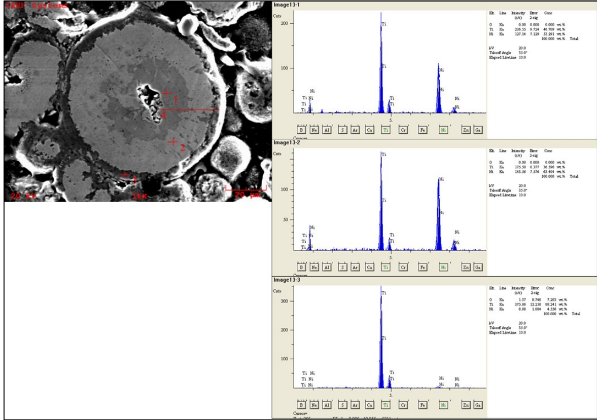
Şekil 5.5. 1125 °C de 1 saat sinterlenen gözenekli NiTi numunenin noktasal EDS analizleri
