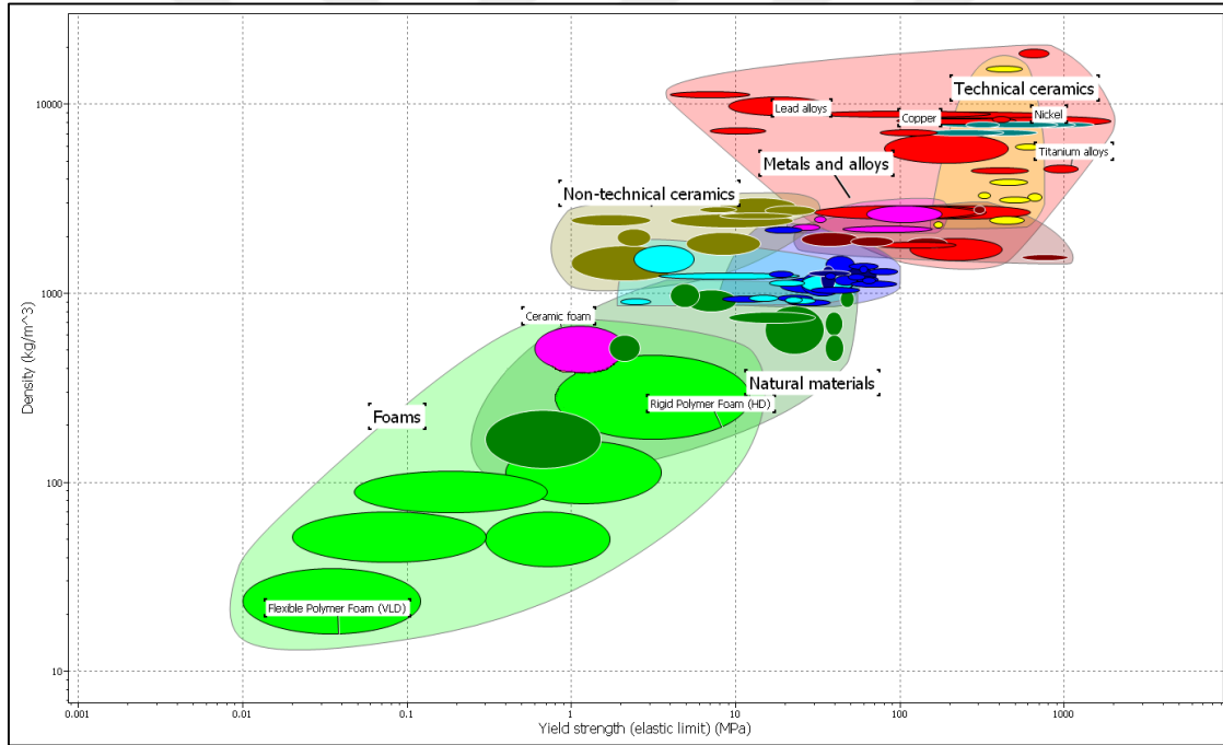
Şekil 3.2. Metal köpüklerin kaplayabileceği grafiğin bölgesinin bir temsili ile, bir dizi mühendislik malzemesinin, akma mukavemetine karşı yoğunluk grafiği üzerindeki konumunu gösteren bir grafik [81].
