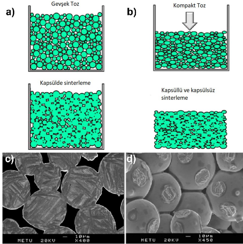
Şekil 3.12. Basıncsız sinterleme tekniği a) basıncsız sinterleme tekniği, b) kompakt toz sinterleme metodu, c) basıncsız sinterleme SEM görüntüsü ve d) kompakt toz sinterlemenin SEM görüntüsü [100]
