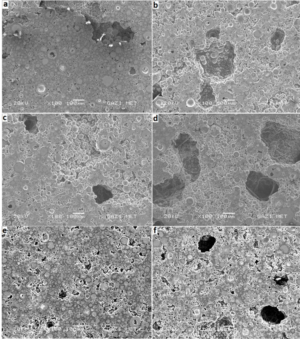
Resim 5.8. Sinterleme işlemi sonrası gözenekli NiTi alaşımların 100x SEM görüntüleri a) 1050 °C, 1 saat, b) 1050 °C, 3 saat, c) 1125 °C, 1 saat, d) 1125 °C, 3 saat, e) 1200 °C, 1 saat, f) 1200 °C, 3 saat
