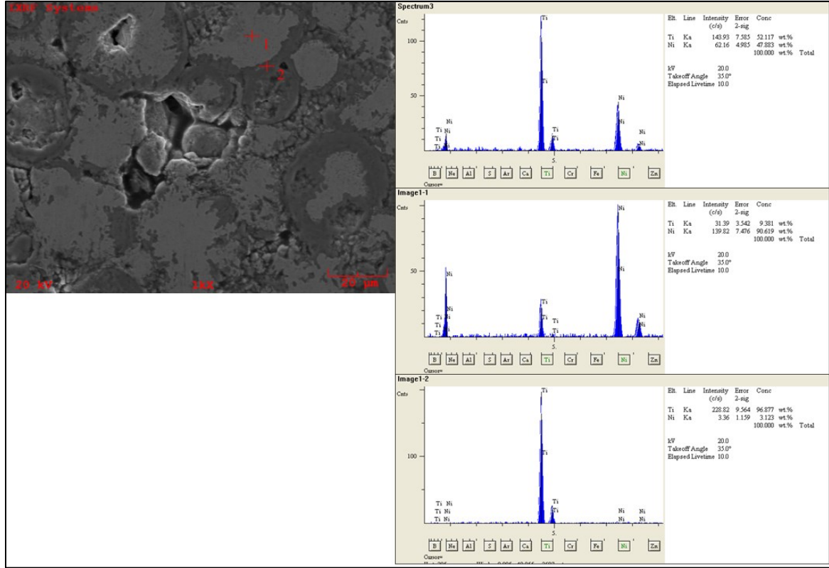
Şekil 5.6. 1125 °C de 3 saat sinterlenen gözenekli NiTi numunenin noktasal EDS analizleri
