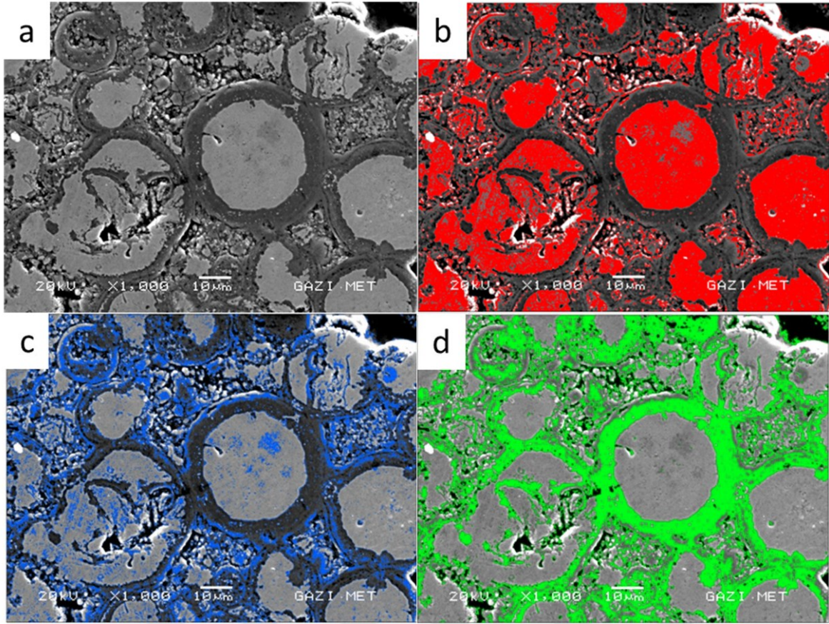
Resim 5.15. 1200 °C’de 1 saat sinterleme sonrası numunenin SEM analizlerinde belirlenen fazları a) NiTi SEM görüntüsü, b) Ni-zengin faz, c) NiTi fazı ve d) Ti-zengin faz
