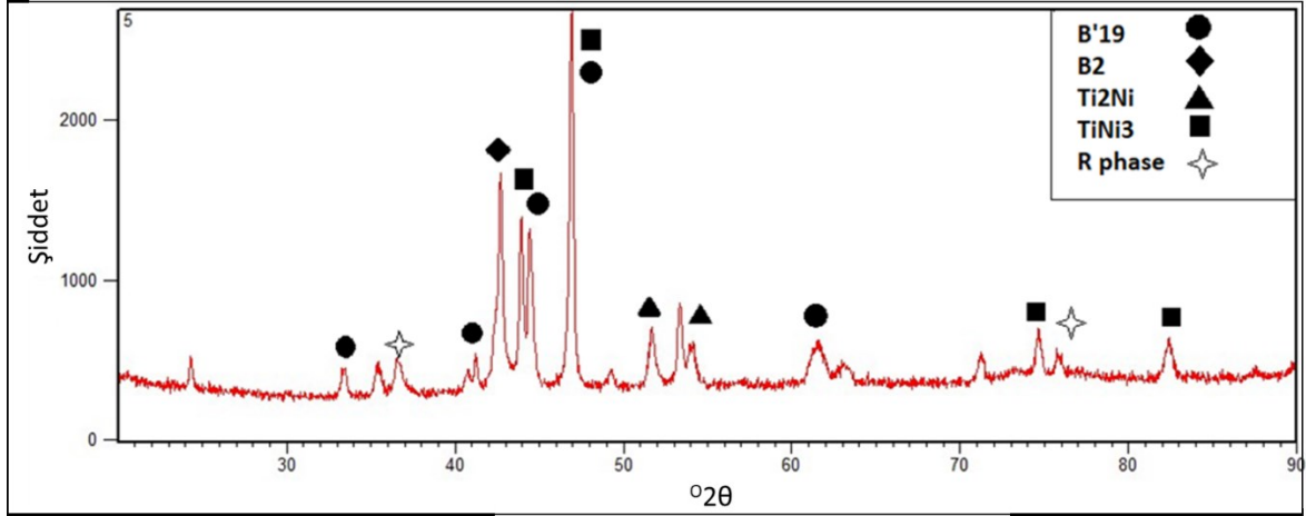
Şekil 5.13. 1200 °C de 1 saat sinterlenen gözenekli NiTi numunenin XRD analizi
