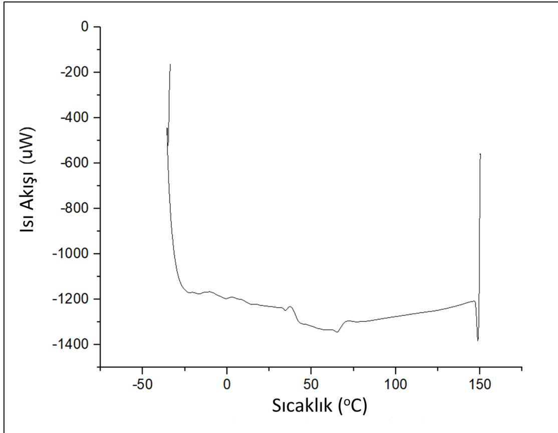
Şekil 5.24. 1200 °C’de 3 saat sinterlenen gözenekli NiTi numunenin ısıtma DSC analizi
