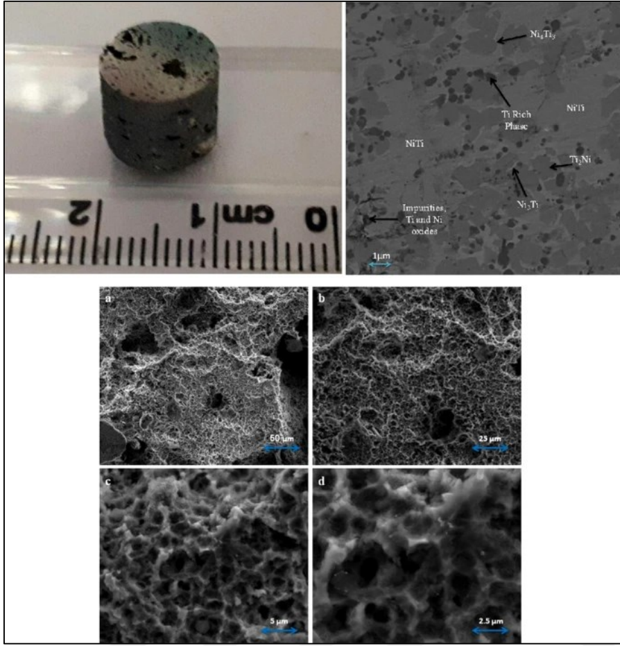
Resim 3.4. SHS yöntemi ile üretilen NiTi numunenin makro ve mikro görüntüleri [5]
