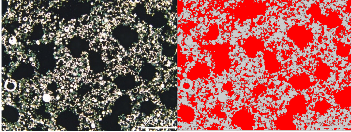
Resim 5.4. 1125 °C de 1 saat sinterlenen numunenin optik mikroskop görüntüsü ve gözenek yapısı
