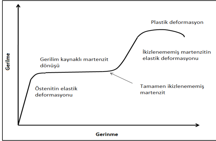
Şekil 2.9. Östenitik fazın gerilme-gerinme davranışı[53]
