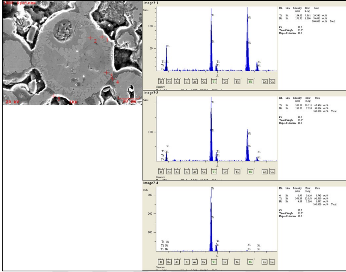
Şekil 5.3. 1050 °C de 1 saat sinterlenen gözenekli NiTi numunenin noktasal EDS analizleri
