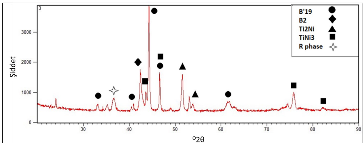
Şekil 5.12. 1125 °C de 3 saat sinterlenen gözenekli NiTi numunenin XRD analizi
