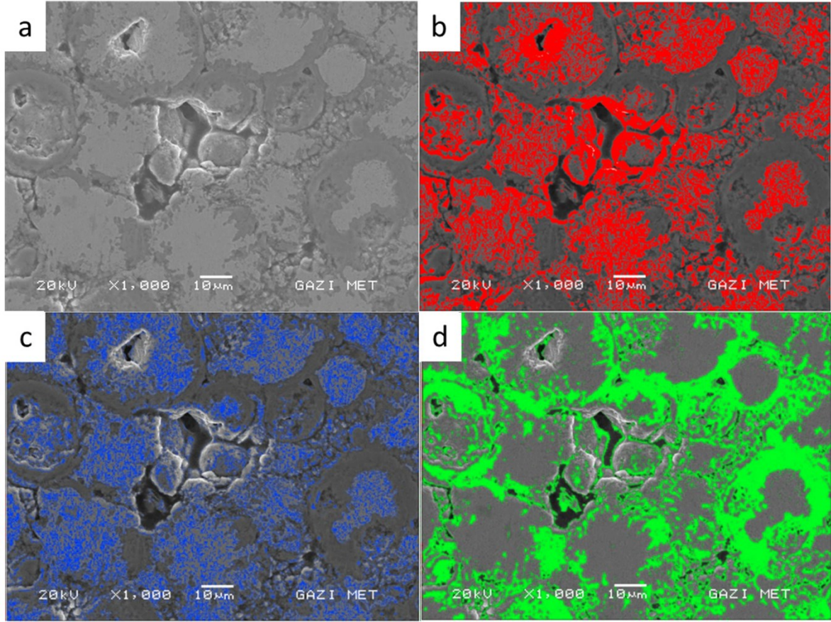
Resim 5.14. 1125 °C’de 3 saat sinterleme sonrası numunenin SEM analizlerinde belirlenen fazları a) NiTi SEM görüntüsü, b) Ni-zengin faz, c) NiTi fazı ve d) Ti-zengin faz
