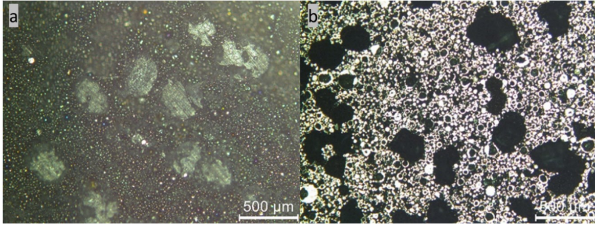
Resim 5.1. 1125 °C de 1 saat sinterlenen numunenin optik mikroskop resimleri (a) çözün - dürme işlemi öncesi, (b) sinterleme sonrası
