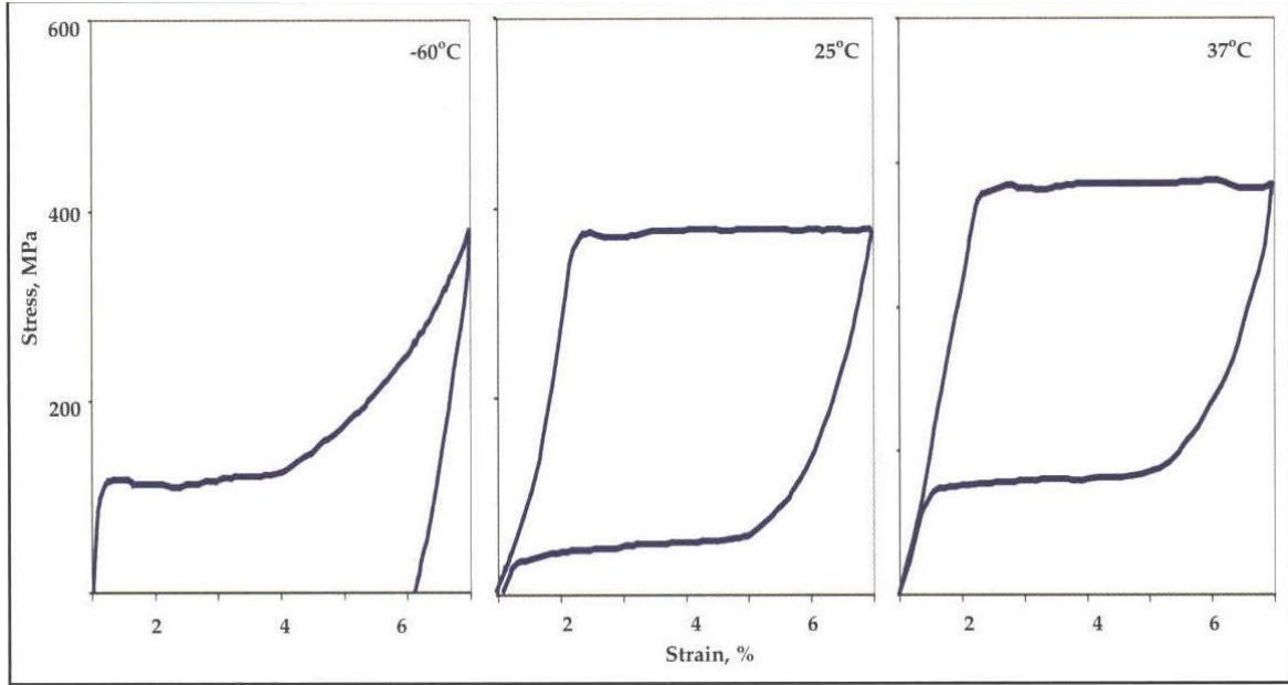
Şekil 2.5. NiTinol ( \text{Ni}_{50,8}\text{Ti}_{49,2} ) telin ( -60^\circ\text{C} ), A_f ( 25^\circ\text{C} ) ve vücut sıcaklığında ( 37^\circ\text{C} ) çekme gerilim – gerinim eğrileri [44]
