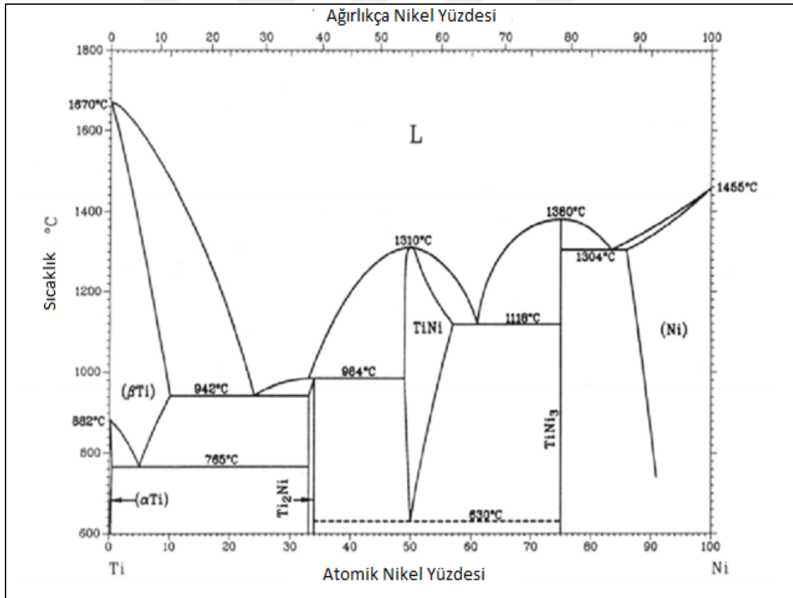
Şekil 2.1. Ti-Ni fazları denge diyagramı [20]
