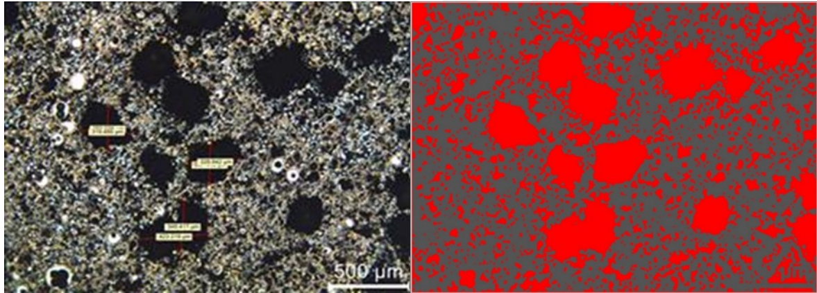
Resim 5.2. 1050 °C’de 1 saat sinterlenen gözenekli NiTi numunenin optik mikroskop ve gözenek yapısı görüntüleri
