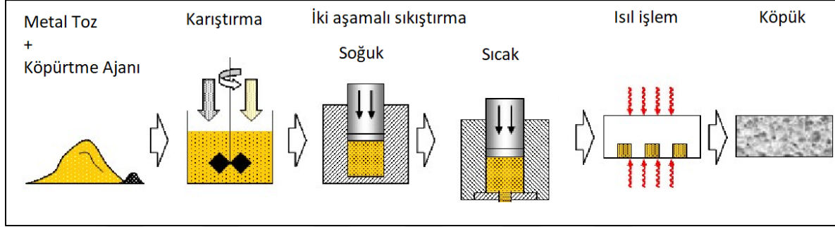
Şekil 3.7. Köpürtme ajanı ile sıkıştırma tekniğinin şematik gösterimi[90]
