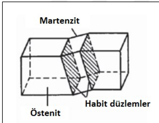
Şekil 2.3. Östenit-martenzit ara yüzeyindeki alışkanlık düzleminin şematik diyagramı [36]
