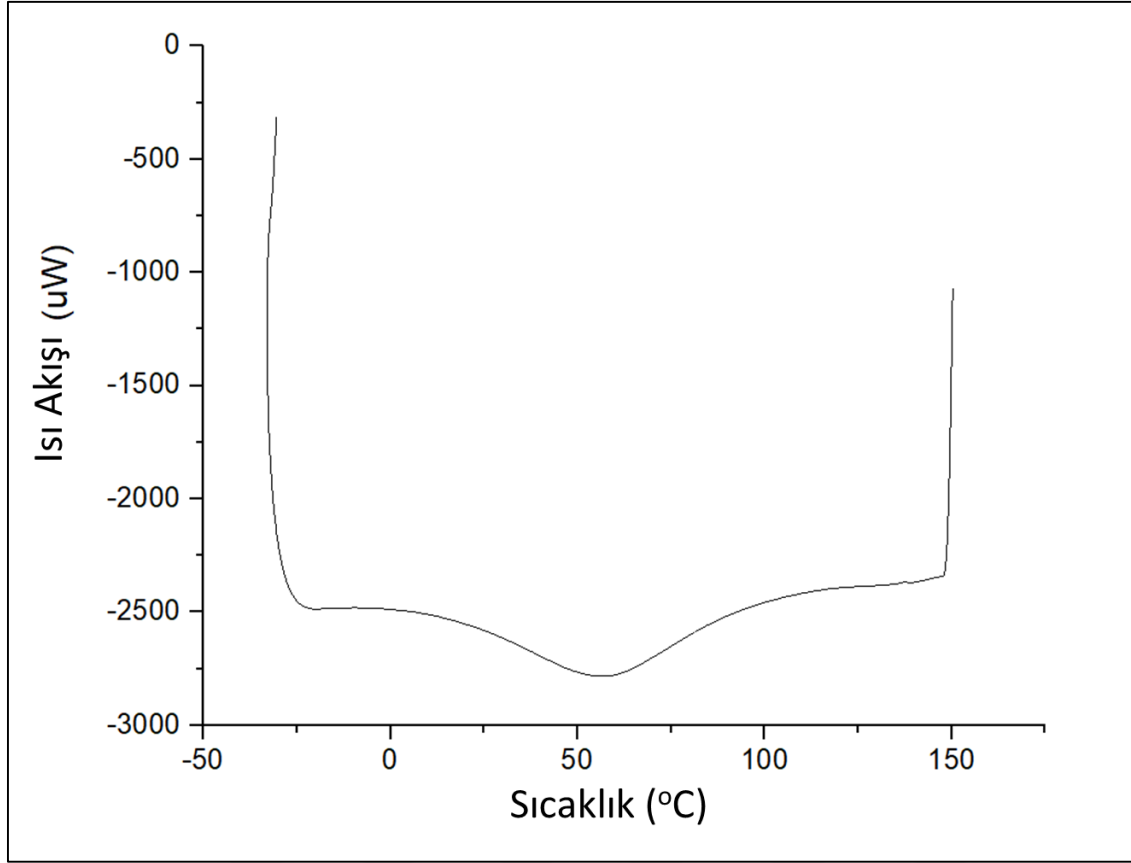
Şekil 5.22. 1125 °C’de 3 saat sinterlenen gözenekli NiTi numunenin ısıtma DSC analizi
