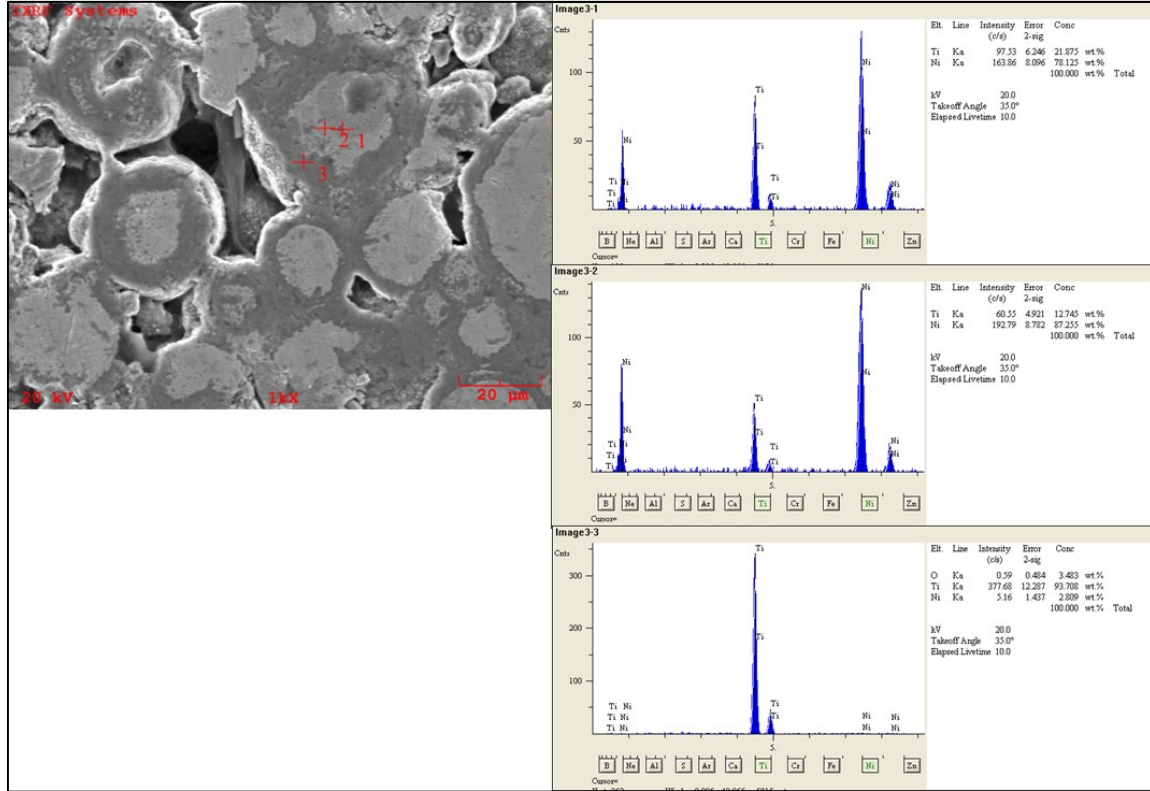
Şekil 5.8. 1200 °C de 3 saat sinterlenen gözenekli NiTi numunenin noktasal EDS analizleri
