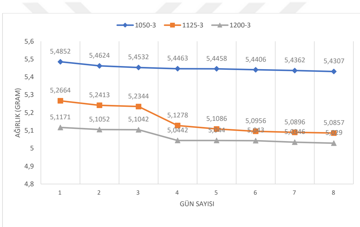
Şekil 5.29. NiTi degregasyon grafiği
