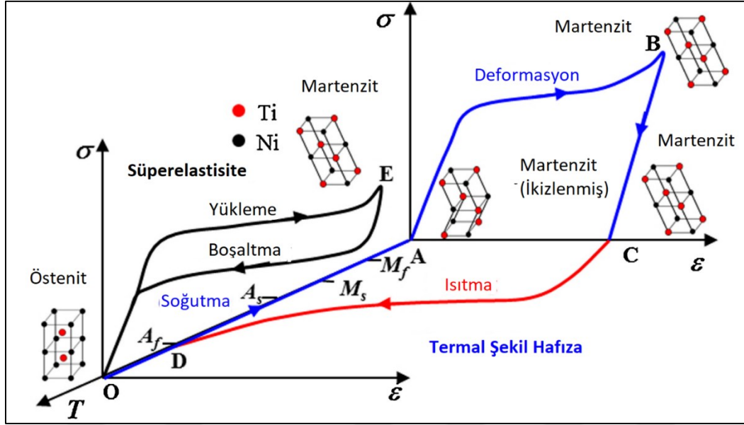
Şekil 2.2. NiTi alaşımının gerilim – genleme – sıcaklık diyagramı [25]
