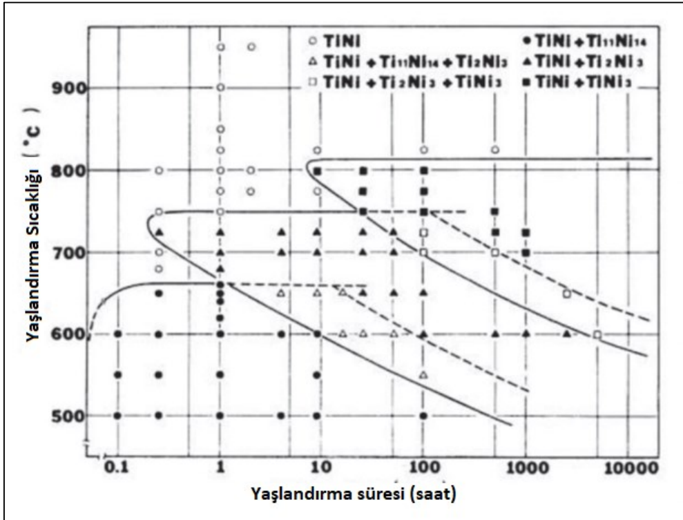
Şekil 2.8. Yaşlandırma süresi, sıcaklığı ve çökelti arasındaki bağlantı [50]
