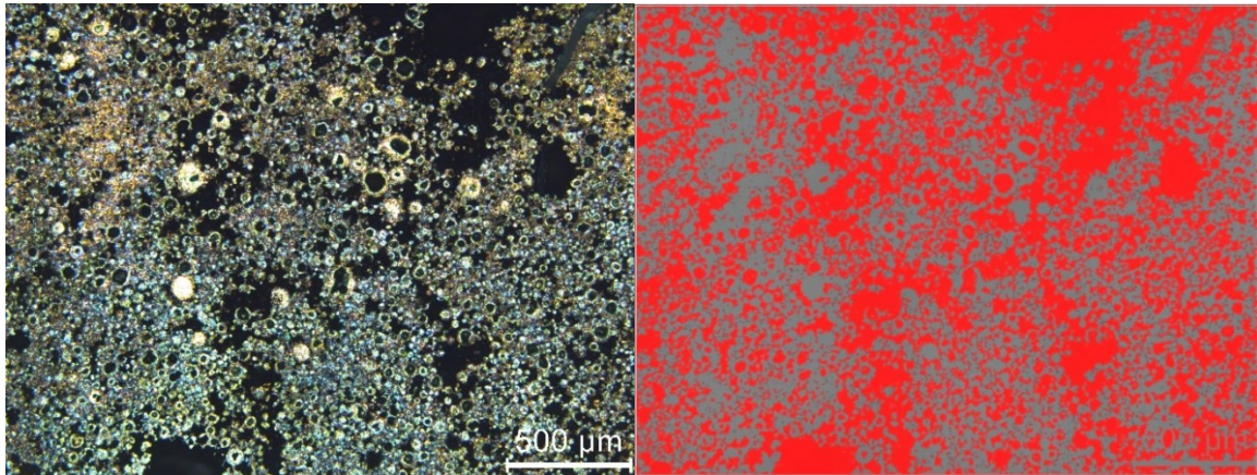
Resim 5.5. 1125 °C de 3 saat sinterlenen numunenin optik mikroskop görüntüsü ve gözenek yapısı
