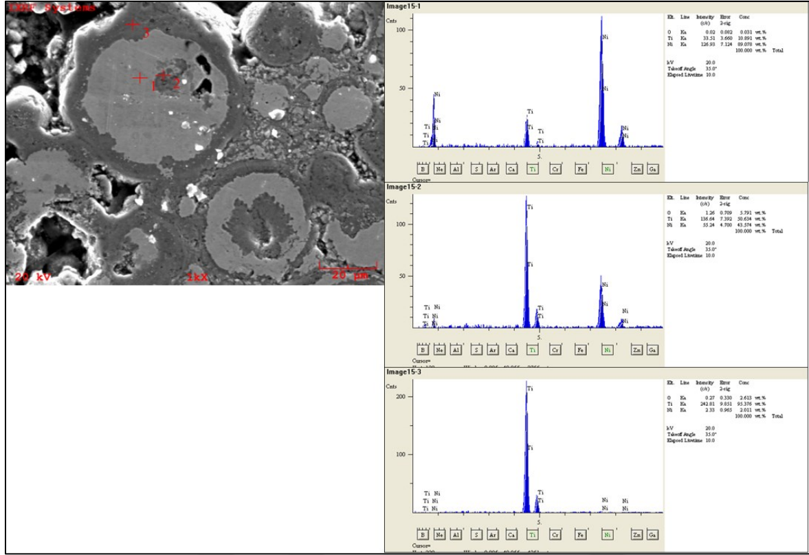
Şekil 5.7. 1200 °C de 1 saat sinterlenen gözenekli NiTi numunenin noktasal EDS analizleri
