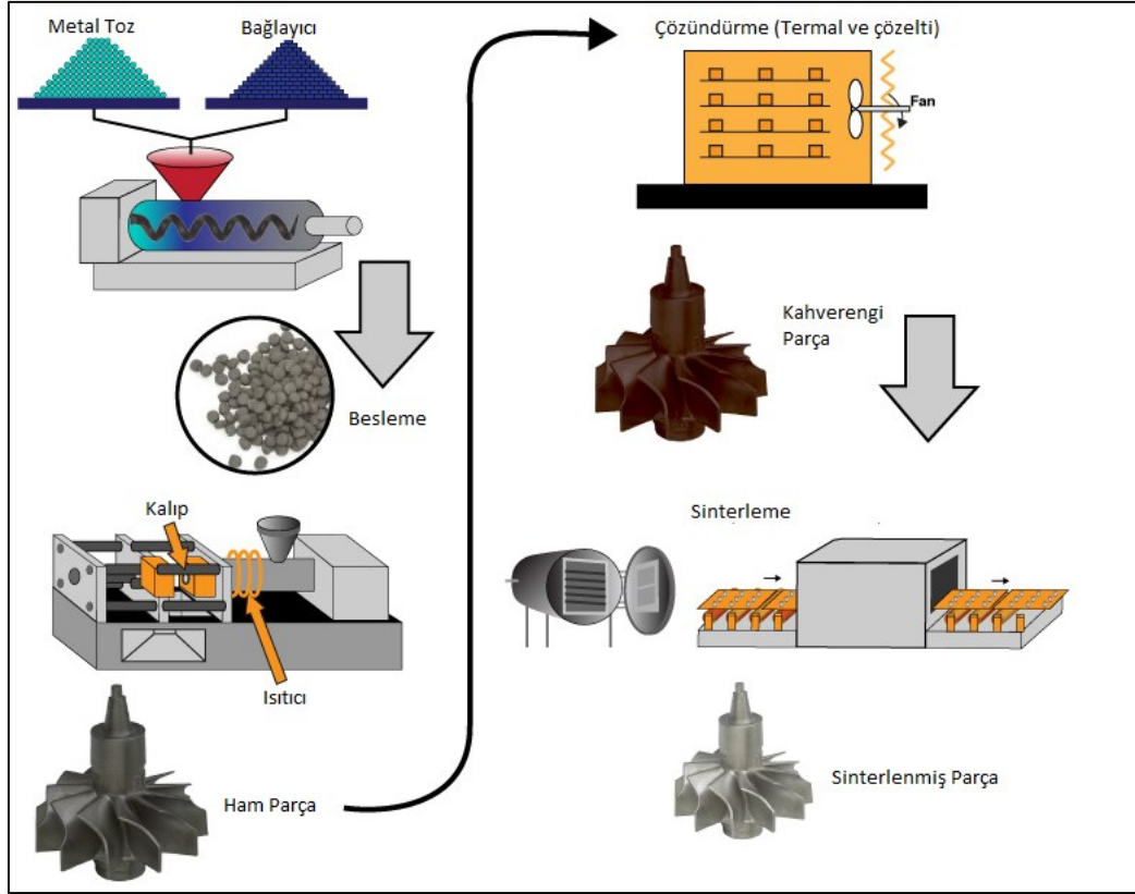
Şekil 3.11. MIM Yönteminin şematik gösterimi
