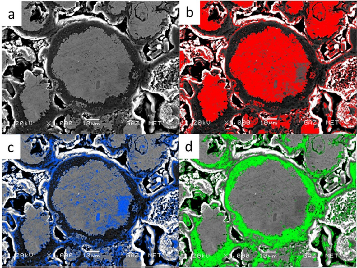
Resim 5.12. 1050 °C’de 3 saat sinterleme sonrası numunenin SEM analizlerinde belirlenen fazları a) NiTi SEM görüntüsü, b) Ni-zengin faz, c) NiTi fazı ve d) Ti-zengin faz
