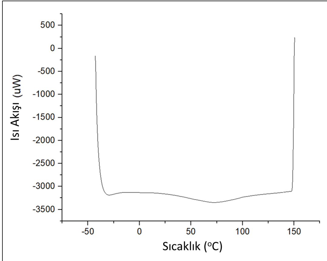
Şekil 5.20. 1050 °C’de 3 saat sinterlenen gözenekli NiTi numunenin ısıtılma DSC analizi
