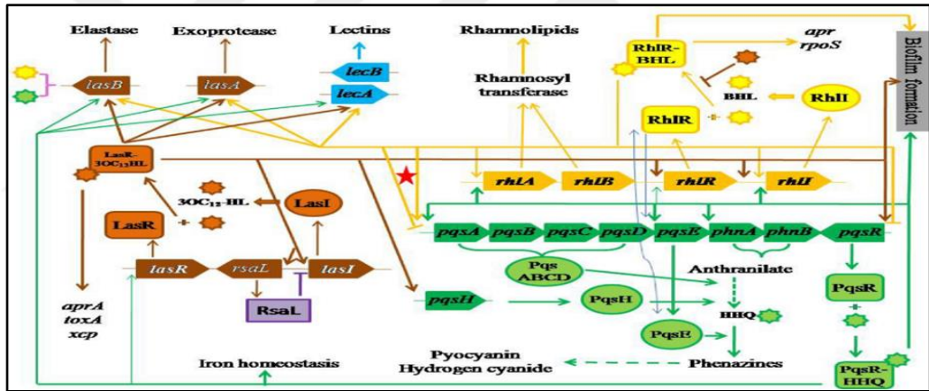
Şekil 2.4 Üç quorum algılama sistemi (Yan and Wu 2019)
