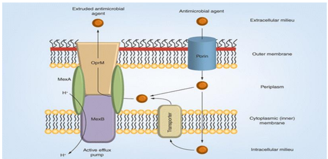
Şekil 2.2 Bakteriye ilaç akış pompasının üç bileşeni ve hücre zarı bileşeni
