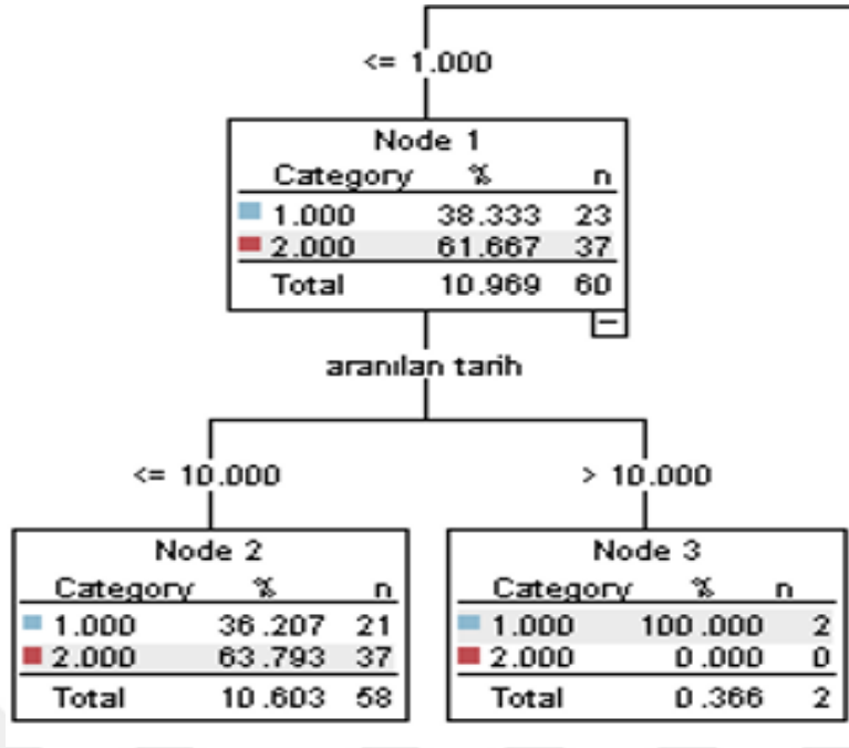
Şekil 4.8. Karar Ağacı Dallanması Örneği 2.
