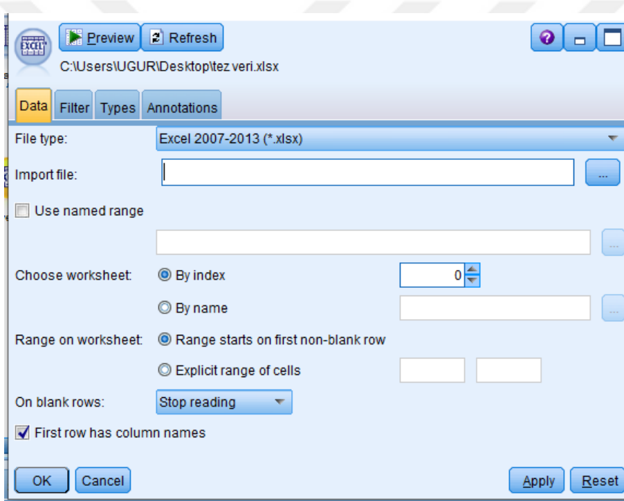
Şekil 4.1. Verinin Yüklenmesi.
