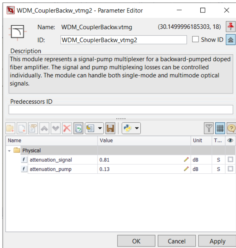
Figure 0.3. WDM parameters
