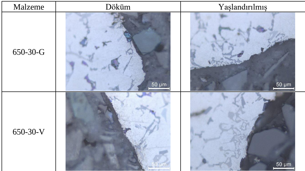
Resim 7.7. 30 ppi gözenek yoğunluklu FDM malzemelerin matris-takviye ara yüzey görüntüleri
