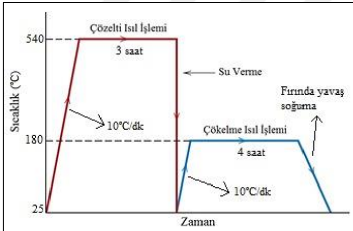
Şekil 6.3. T6 ısıtım işlemi uygulama adımları ve işlem şartları
