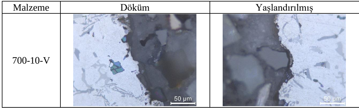
Resim 7.6. (devam) 10 ppi gözenek yoğunluklu FDM malzemelerin matris-takviye ara yüzey görüntüleri
