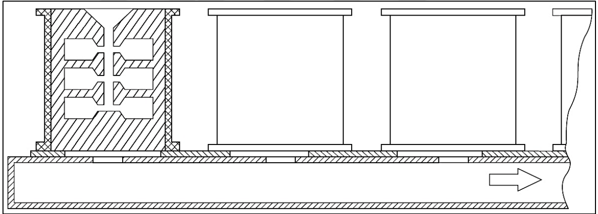
Şekil 5.10. Vakum destekli dökümde döküm için sıralanmış bir vakum manifoldu üzerinde oturan alçı kalıplar [47]
