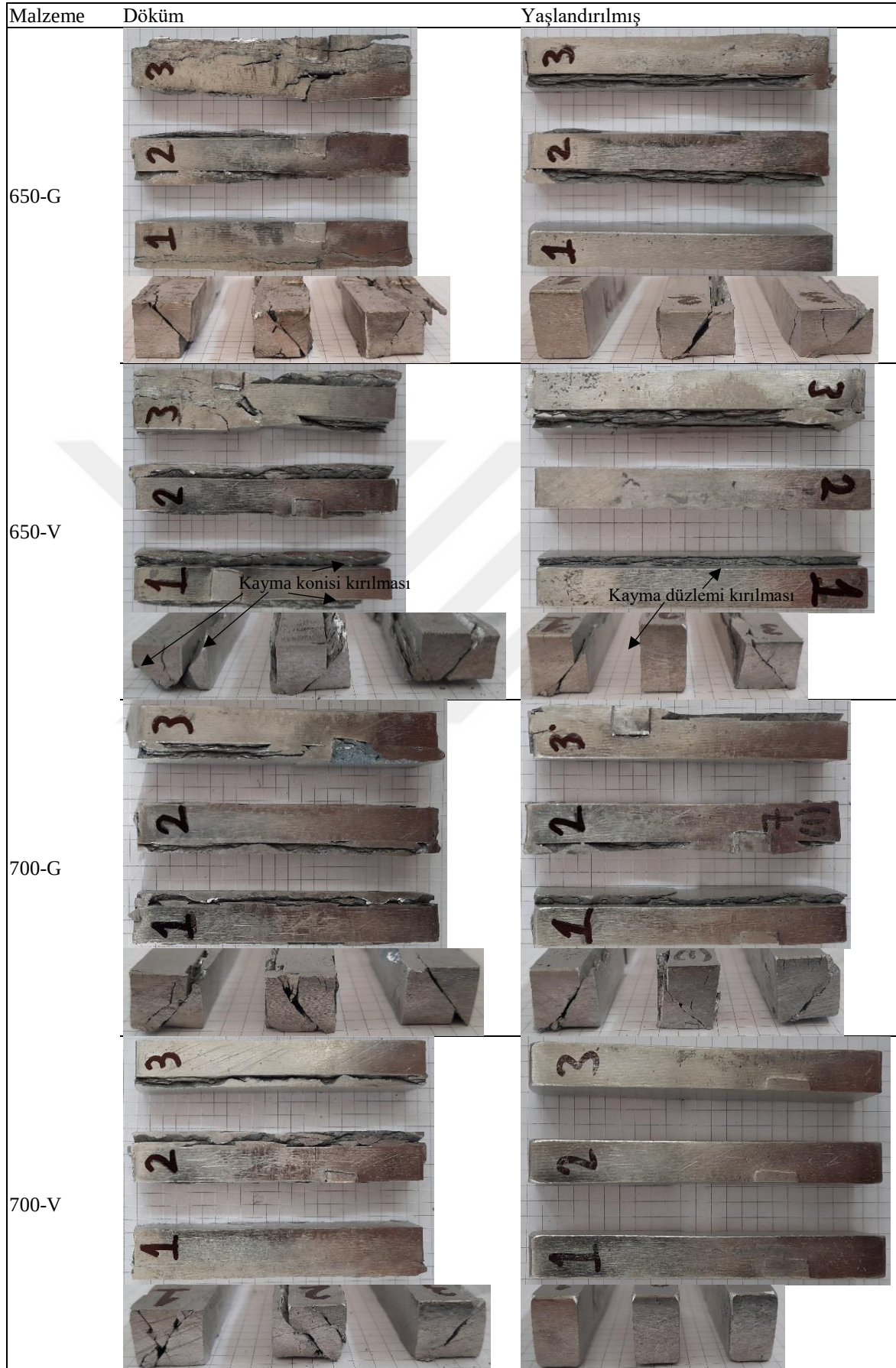
Resim 7.20. Takviyesiz alüminyum numunelerin basma testi sonrası görüntüleri
