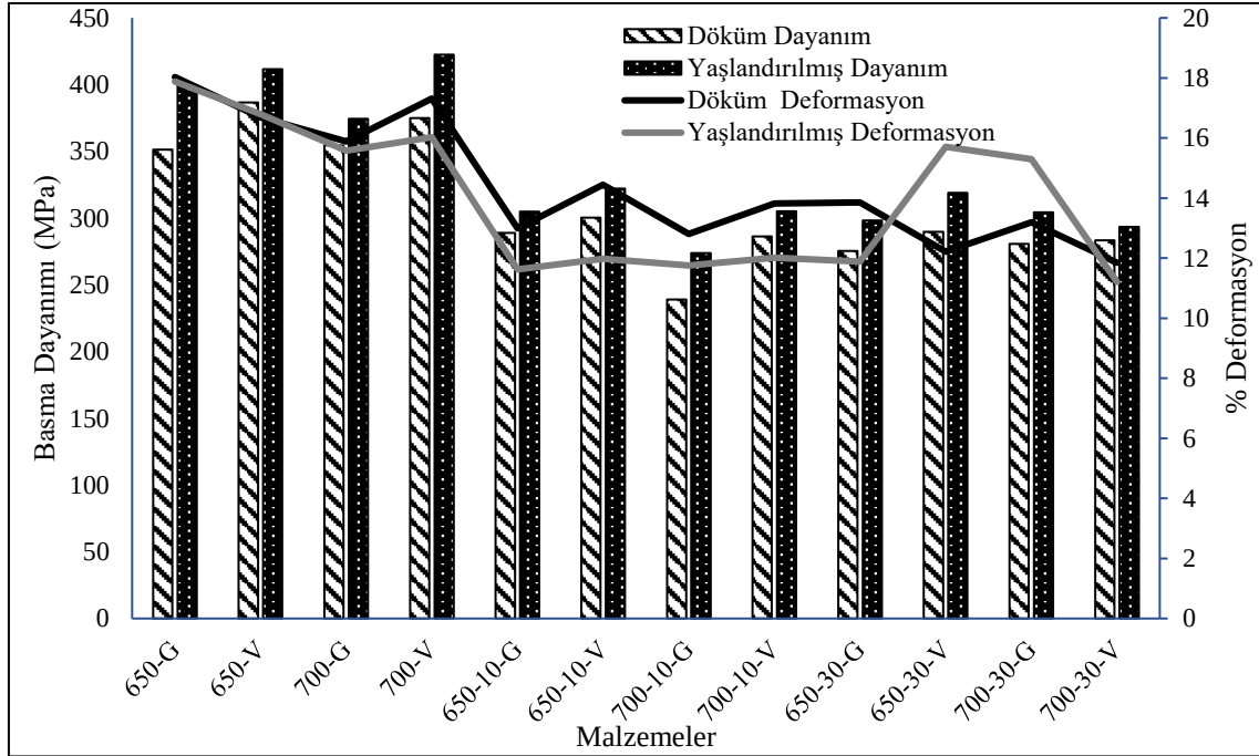
Şekil 7.9. Takviyesiz alüminyum ve FDM'lerin basma dayanımları ve boyutsal kısıalma miktarları
