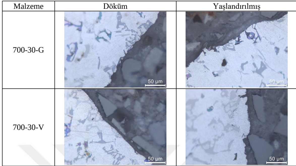
Resim 7.7. (devam) 30 ppi gözenek yoğunluklu FDM malzemelerin matris-takviye ara yüzey görüntüleri
