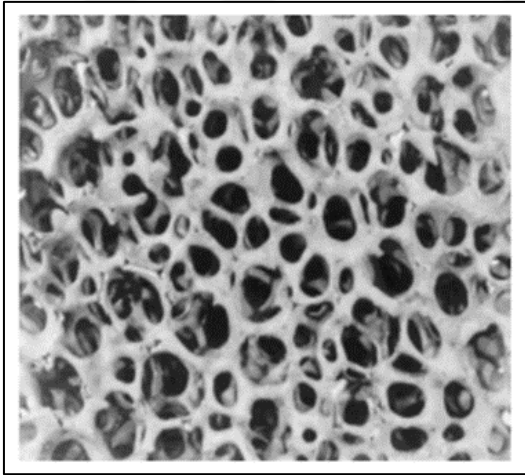
Resim 3.1. Replikasyon yöntemi ile üretilmiş gözenekli seramik [34]
