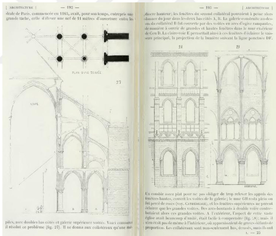
Figure 3.6.3. "Coupe / Plan d'une Travée" and "Exterior and Interior of Notre-Dame de Paris" in the Dictionnaire Raisoné by Viollet-le-Duc, 1854.
