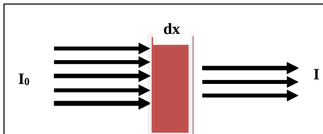
Şekil 2.11. dx kesitli malzemeden geçen elektromanyetik radyasyonun absorblanması
