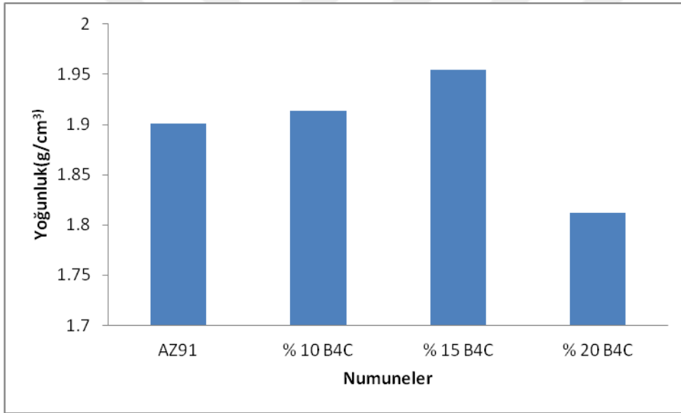
Şekil 4.1. Numunelerin yoğunluk sonuçları
