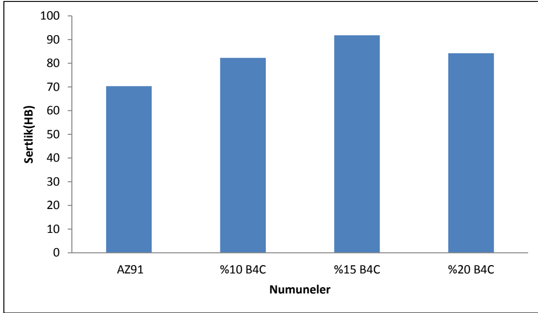
Şekil 4.2. Numunelerin sertlik sonuçları
