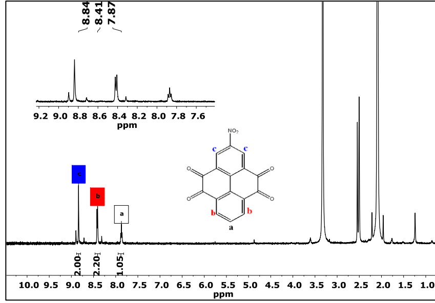
Şekil 6.7: PTO-NO 2 yapısının ^1\text{H} NMR spektrumu.
