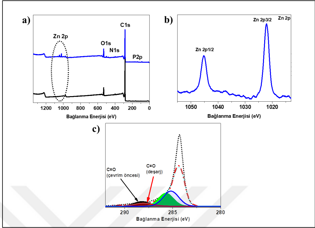
Şekil 7.37: 10/KB'nin Çevrim öncesi, ilk deşarj çevrimleri için a) Genel XPS spektrumu b) Kısmi Zn2p spektrumu c) Kısmi C1s spektrumu.
