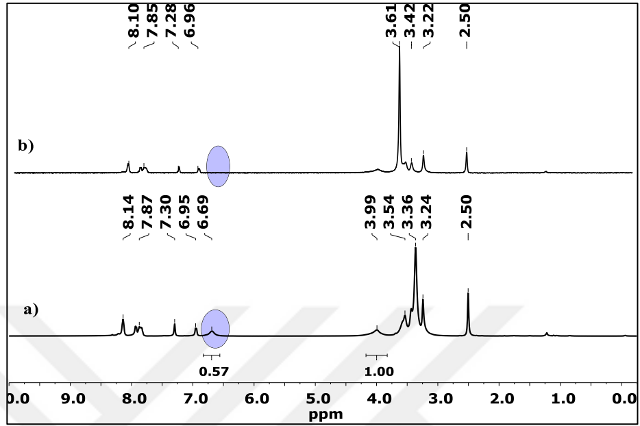
Şekil 6.33: Polimer 10'un a) DMSO-d 6 ve b) DMSO-d 6 + D 2 O içinde alınan 1 H NMR spektrumları.
