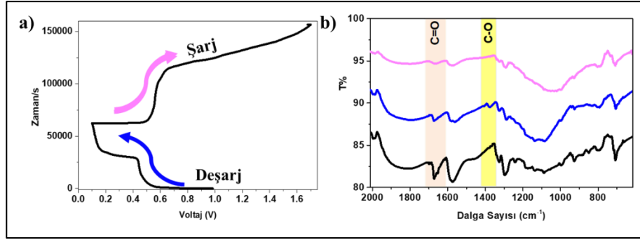
Şekil 7.32: Bileşik 5'in a) Zamana bağlı ilk şarj-deşarj grafiği b) Çevrim öncesi, ilkdeşarj ve şarj çevrimleri için FT-IR spektrumu.
