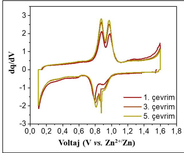
Şekil 7.7: 6/KB katodunun dq/dv karşı voltaj grafiği.
