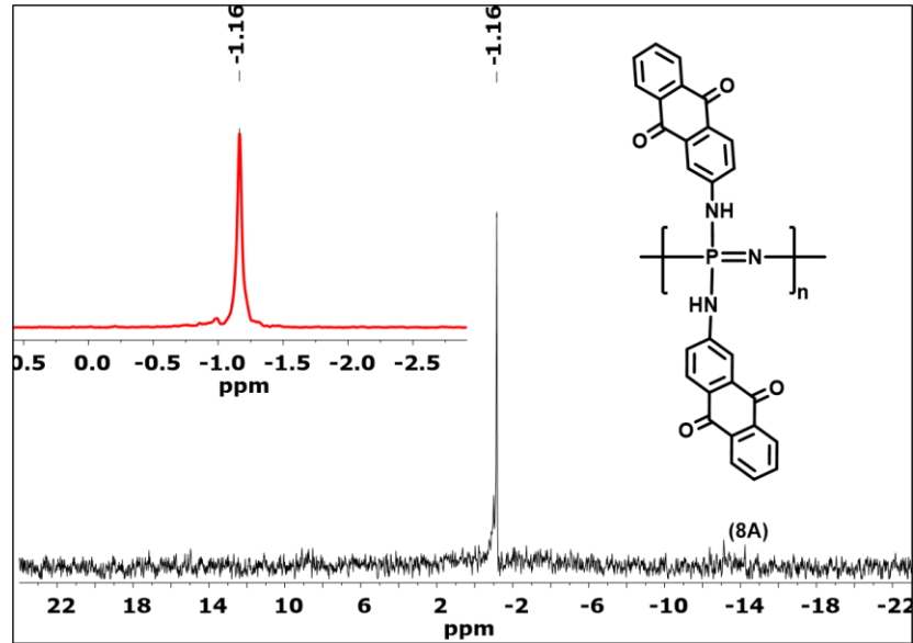
Şekil 6.19: Polimer 8A'nın ^{31}\text{P} NMR spektrumu.
