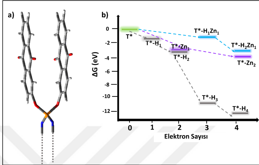
Şekil 7.46: a) Basitleştirilmiş T* yapısı b) Zn^{2+}/H^{+} iyonlarının koordinasyonuna bağlı \Delta G(E_b) grafiği.
