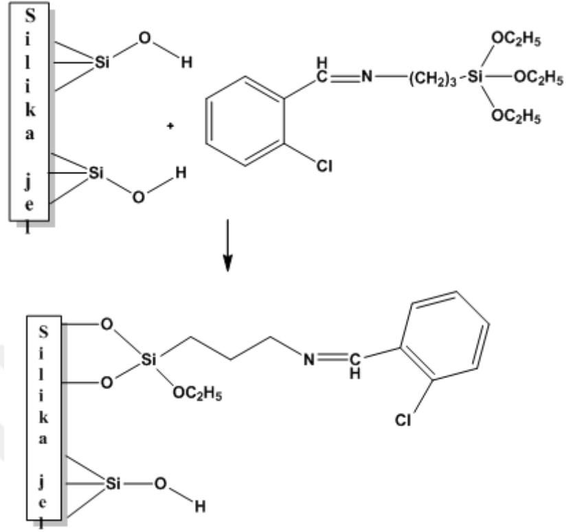
SG-[N-(2-klorobenzilidin)-3-(trietoksisilil)propan-1-amin]
