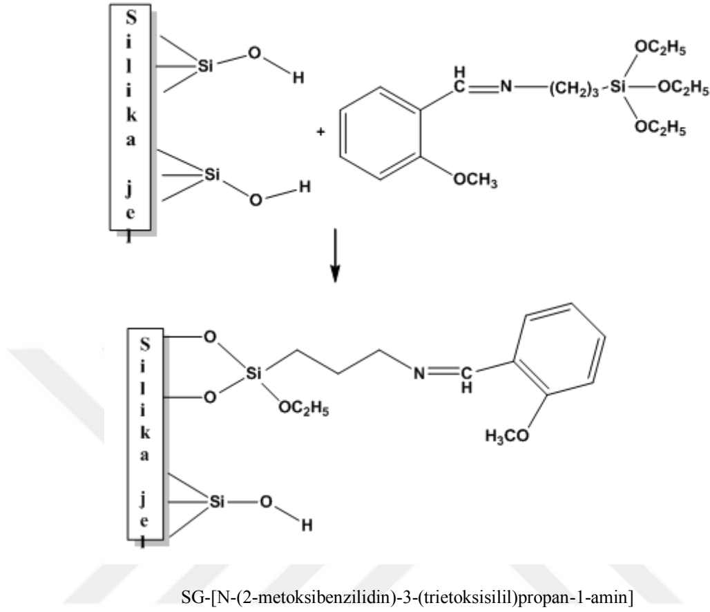
Şekil 2.9: MI bileşiğinin silika jel yüzeyine modifikasyonu.
