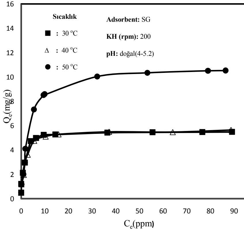
Şekil 3.12: SG yüzeyinde farklı sıcaklıklarda Cu(II) adsorpsiyonu.
