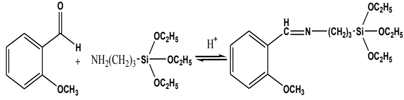
N-(2-metoksibenzilidin)-3-(trietoksisilil)propan-1-amin
