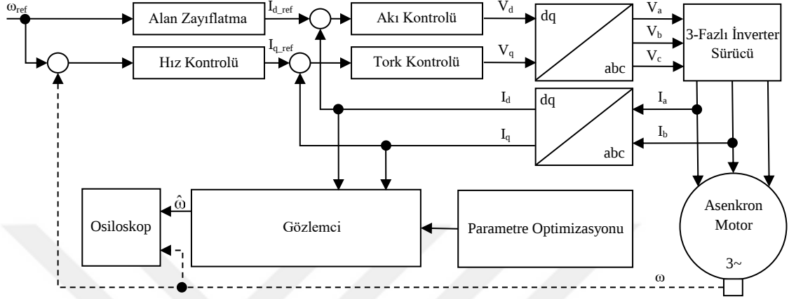
Şekil 4.1: Asenkron motor hız kontrol sistemindeki gözlemci testleri için hazırlanan blok şeması.
