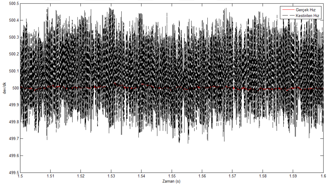
Şekil 5.8: STSM gözlemci için gerçek ve kestirilen hız karşılaştırması (yakınlaştırılmış).
