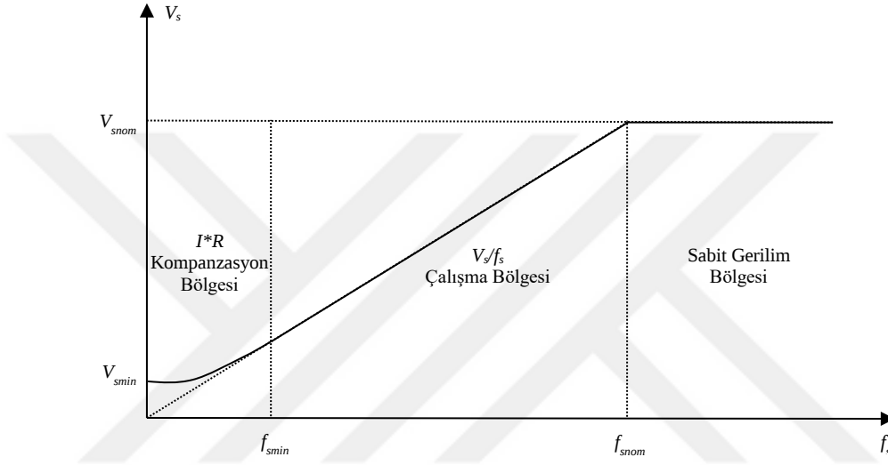
Şekil 2.10: Asenkron motorun gerilim/frekans oranı ile çalışma eğrisi.
