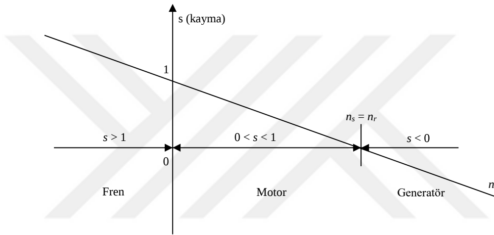
Şekil 2.4: Asenkron makinanın motor, generatör ve fren çalışma durumları.
