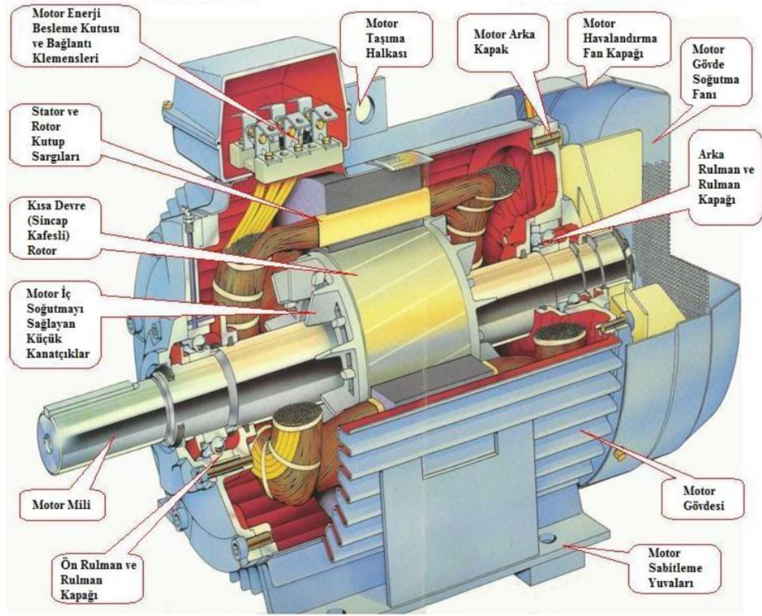
Şekil 2.1: Sincap kafesli asenkron motor.
