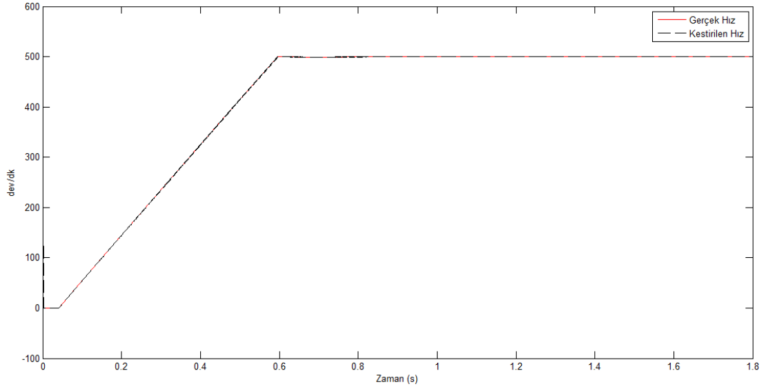
Şekil 5.9: FOSM gözlemci için gerçek ve kestirilen hız karşılaştırması.
