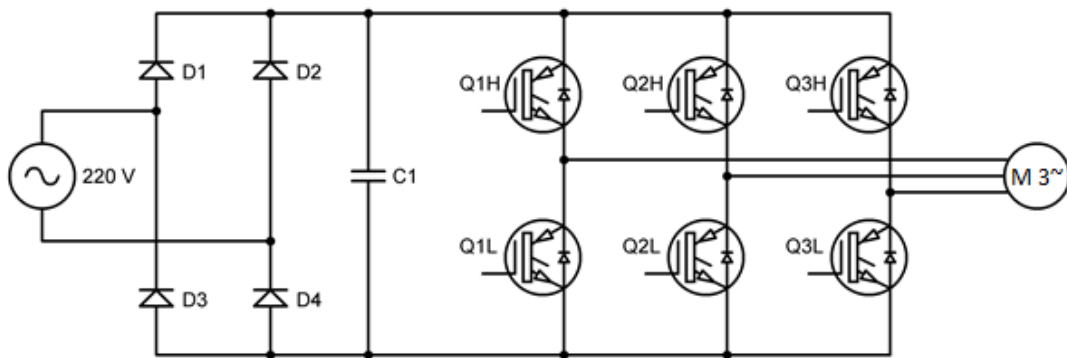
Şekil 2.17: İnverter sürücü devresi.
