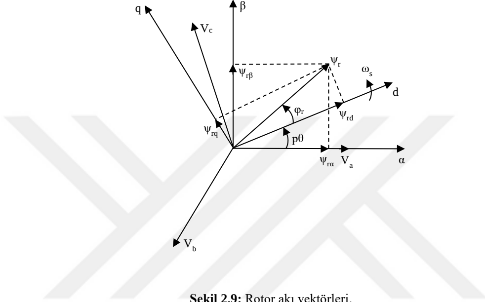
Şekil 2.9: Rotor akı vektörleri.
