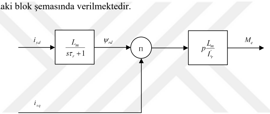
Şekil 2.13: Statorun dq eksen akım bileşenleri ile moment arasındaki ilişki.
