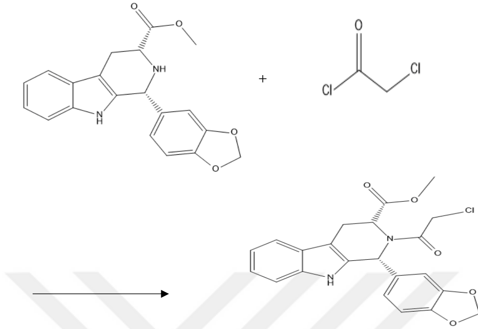
Şekil 3.2. Oluşan bileşiğin asetillendirilmesi
