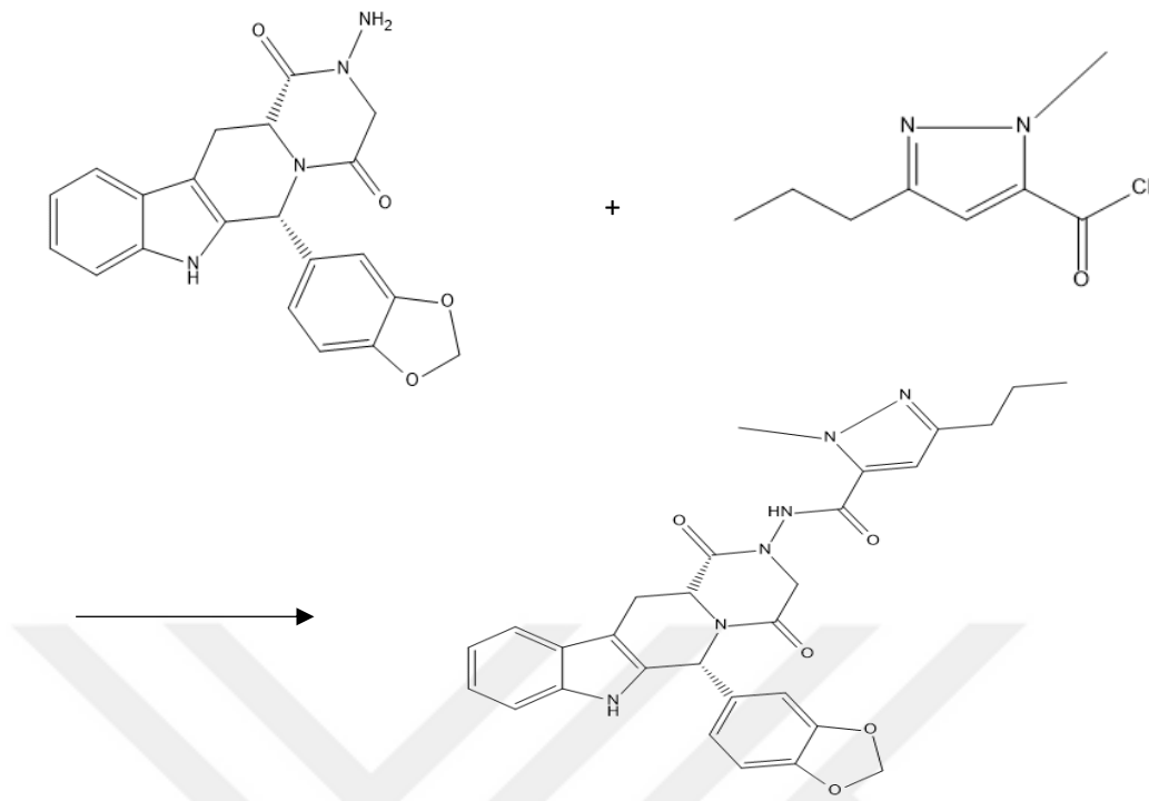
Şekil 3.11. N-pirazol türevli tadalafil sentezi
