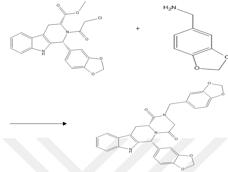
Şekil 3.3. Piperon türevli tadalafil sentezi
