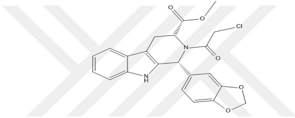
Şekil 5.2. Asetilleme Reaksiyonu Ürünü
