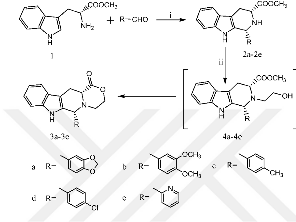
Şekil 2.5. Tadalafil sentezi (Reaktifler: i, TFA, CH 2 Cl 2 , CH 3 OH, rt, 4 gün; ii, oksiran, CH 3 OH, rt, 5 – 7 gün)
