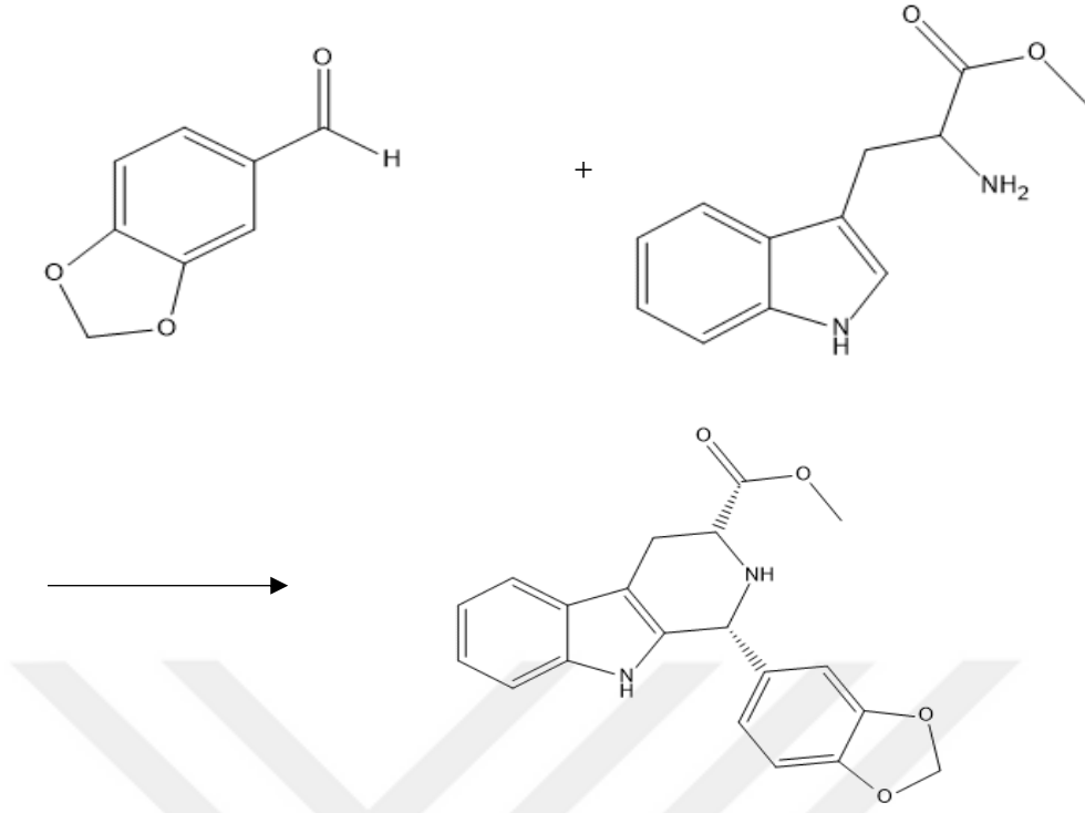
Şekil 3.1. D-triptofan metil esterinin halkalaşması
