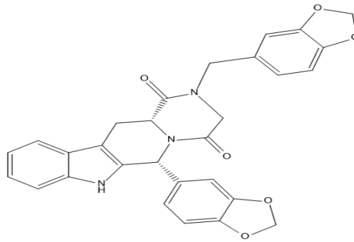
Şekil 5.3. Piperon türevli tadalafil
