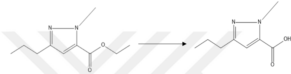
Şekil 3.6. 1-metil-3-propil-1H-pirazol-5-karboksilik asit sentezi
