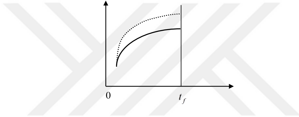
Şekil 3.4: Düşey bitiş doğrusundaki değişim problemi.
