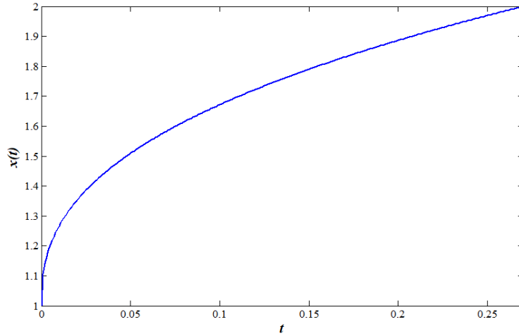
Şekil 3.10: Yatay bitiş doğrusu probleminde x(t) minimizasyon fonksiyonu.
