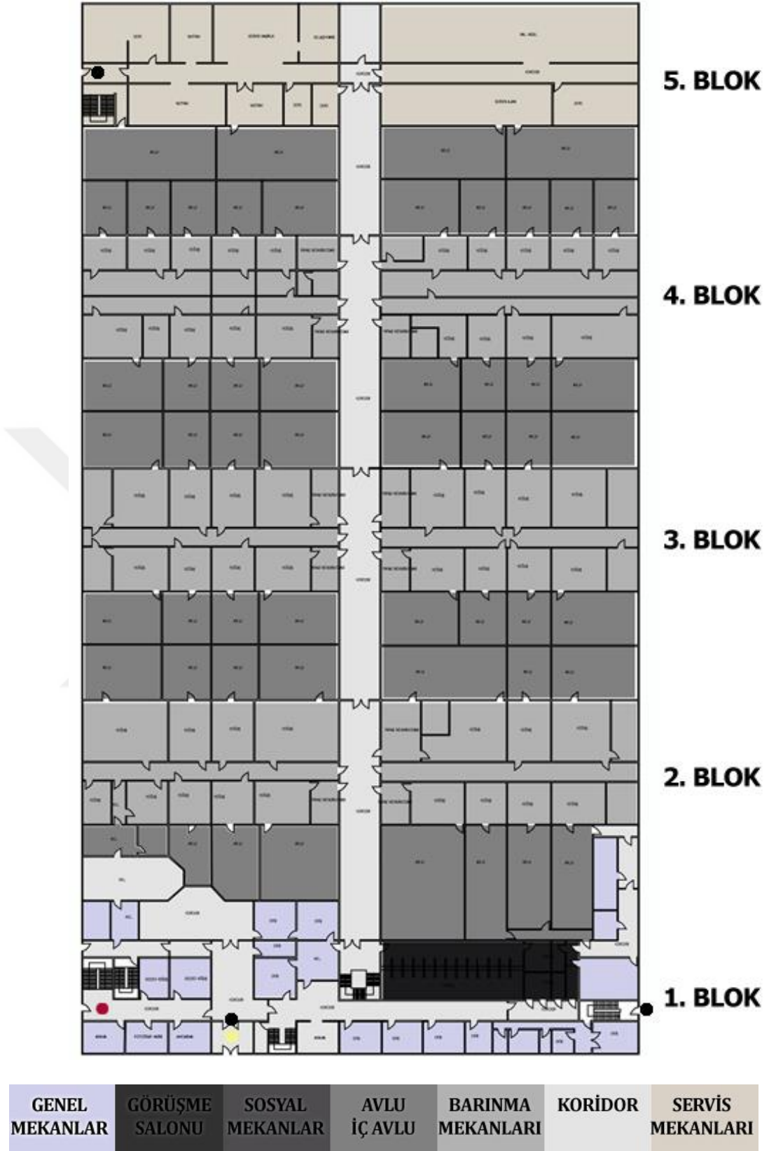
Şekil 4. 14. E tipi cezaevi mimari tip proje (Ağaçkale,2010)
