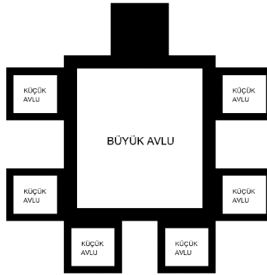
Şekil 3. 20. Genel avlulu cezaevi şeması (Emiroğlu, 2003)
