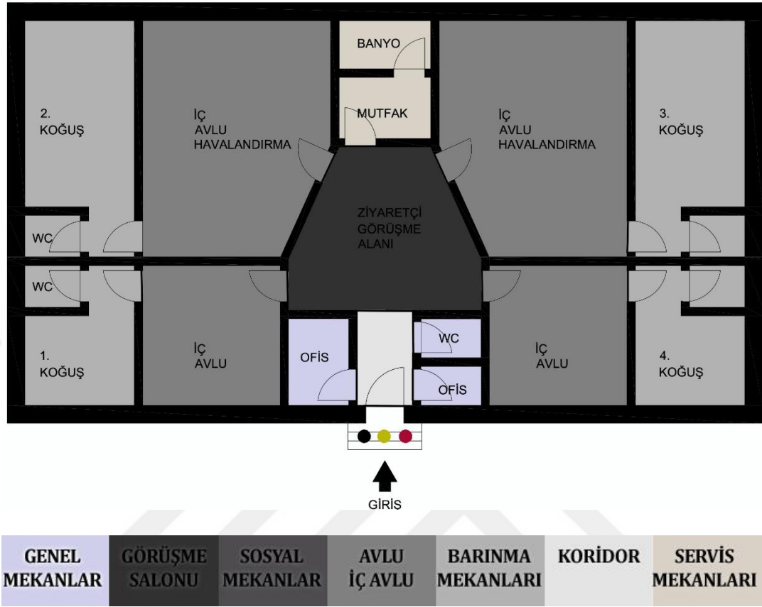
Şekil 4. 5. A tipi cezaevi mimari tip proje (Bayındırlık Bakanlığı Arşivi, Ağaçkale, 2010)
