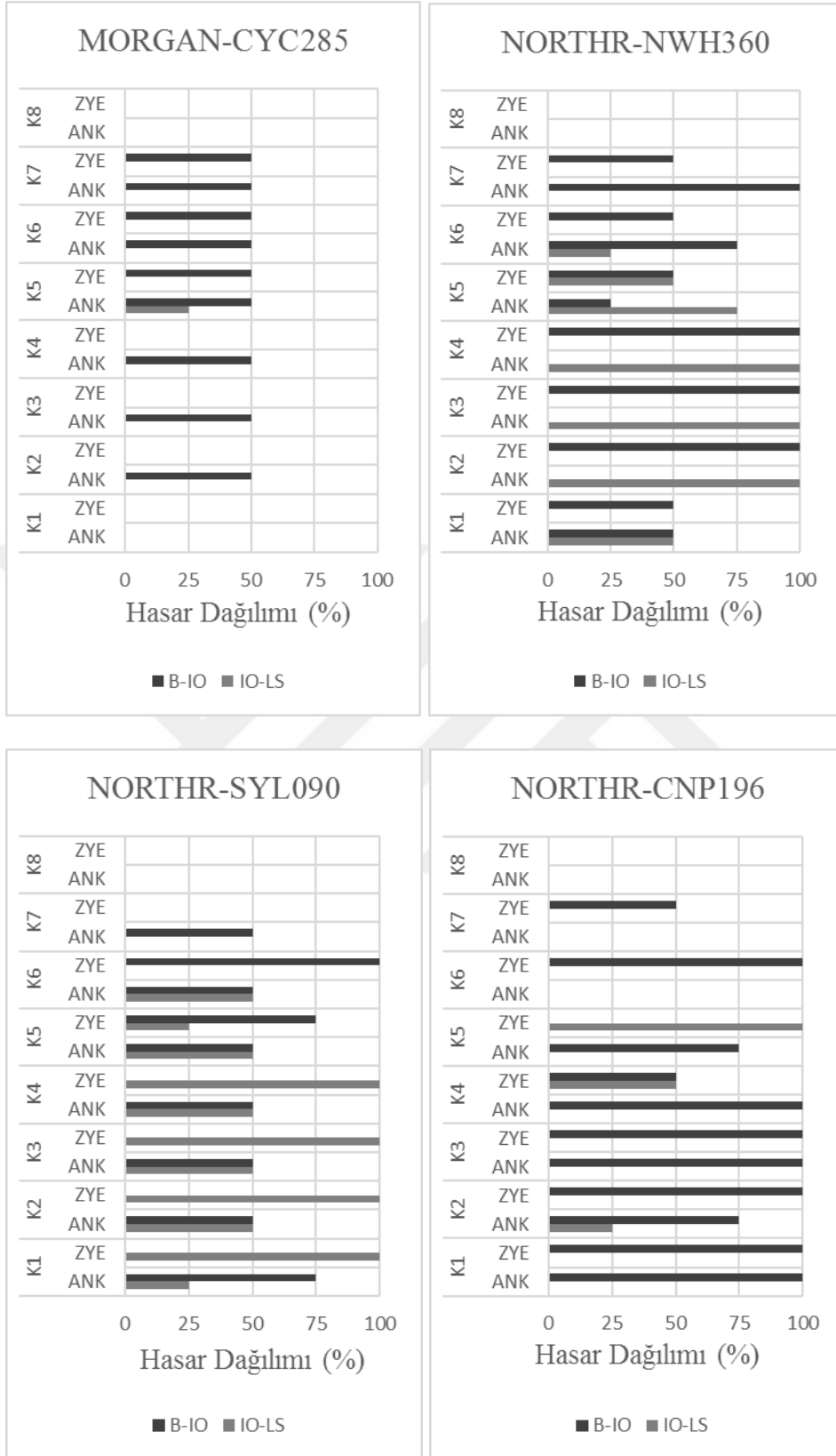
Şekil 4.31 : 8K_C-C Hasar Dağılımlarının Karşılaştırılması (Devamı)
