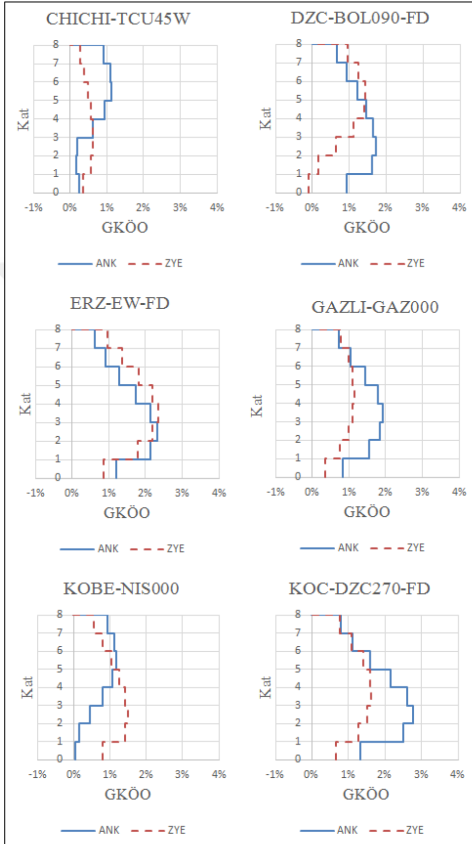
Şekil 8.12 : 8K_C-C GKÖÖ Karşılaştırılması
