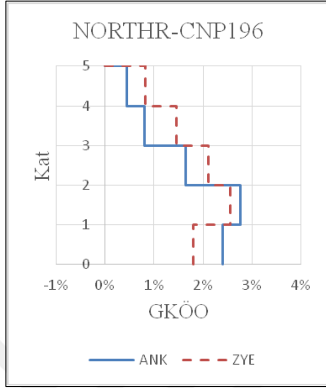
Şekil 4.14 : 5K_2-2 GKÖÖ Karşılaştırılması
