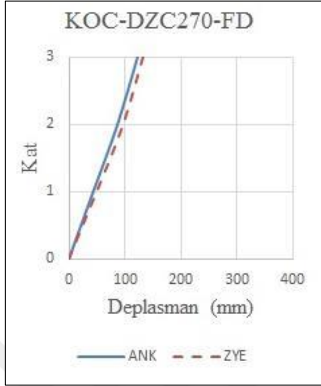
Şekil 4.10 : 3K_C-C Kat Deplasmanlarının Karşılaştırılması
