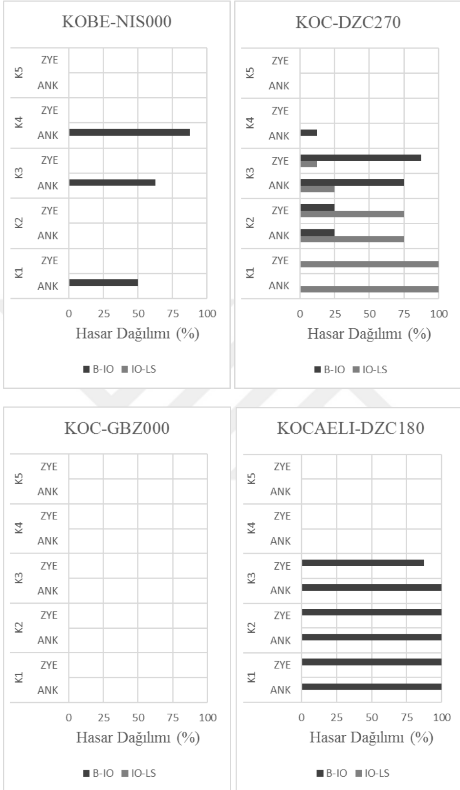
Şekil 4.32 : 5K_2-2 Hasar Dağılımlarının Karşılaştırılması (Devamı)
