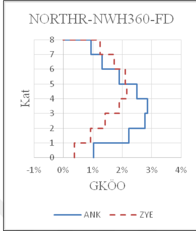
Şekil 4.13 : 8K_C-C GKÖO Karşılaştırılması
