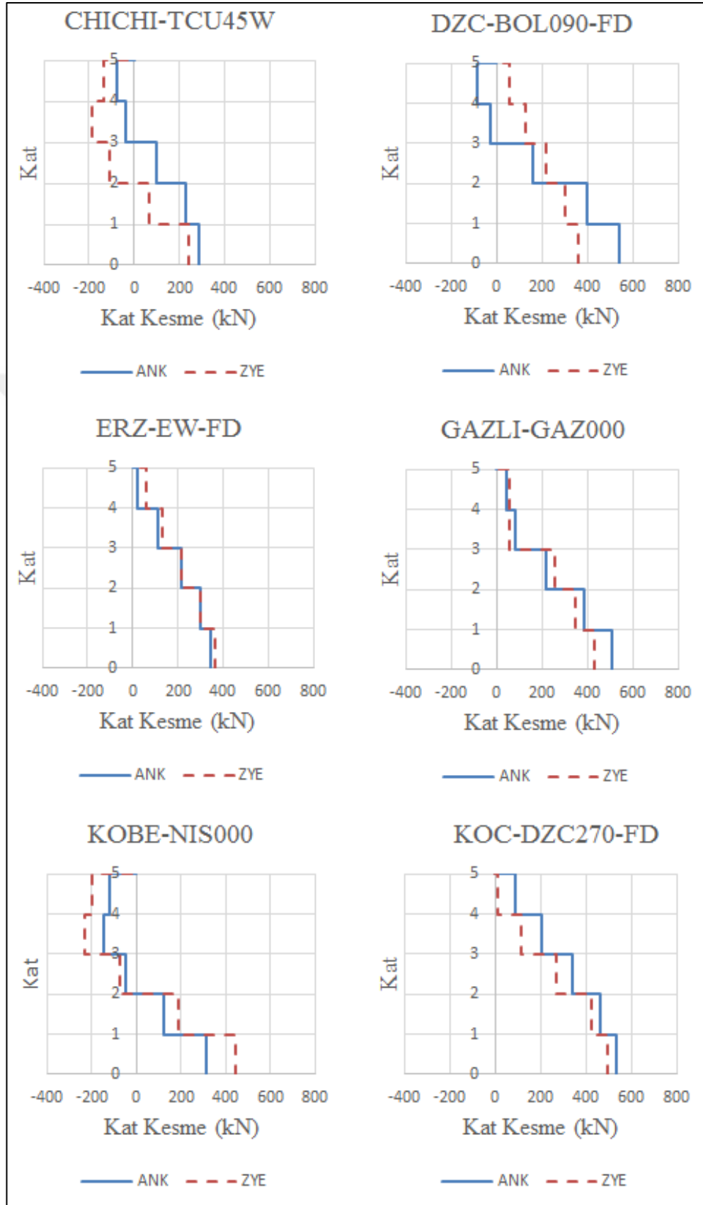
Şekil 8.23 : 5K_B-B Kat Kesme Kuvvetlerinin Karşılaştırılması
