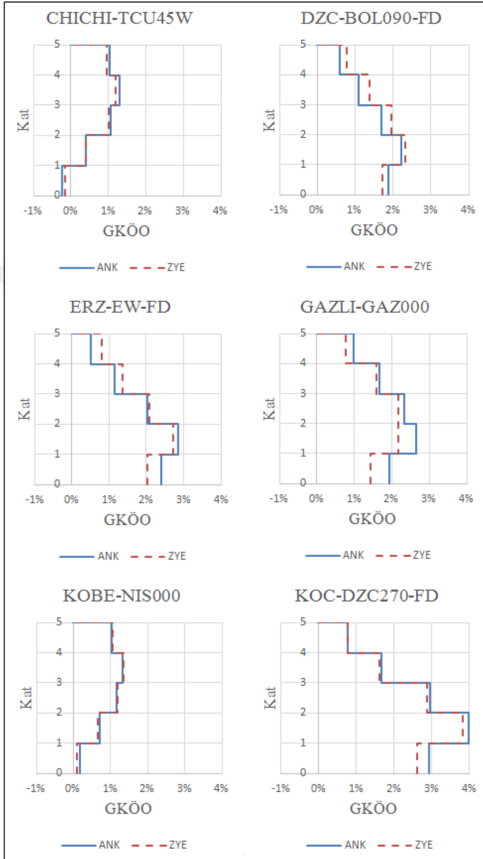
Şekil 8.13 : 5K_2-2 GKÖÖ Karşılaştırılması
