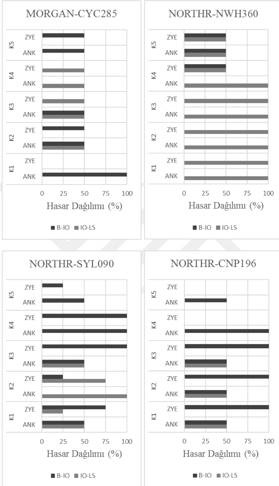
Şekil 4.33 : 5K_B-B Hasar Dağılımlarının Karşılaştırılması (Devamı)
