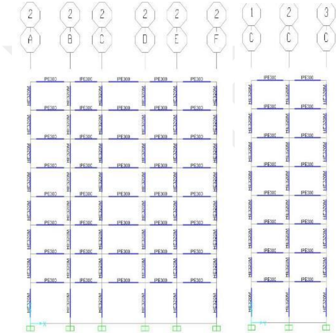
Şekil 2.2: 8 katlı model sistem kesitleri
