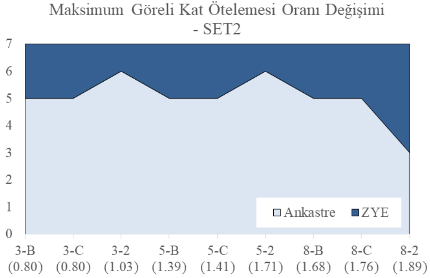
Şekil 4.45 : Maksimum görelî kat ötelemesi oranında artım olasılığı – Set2
