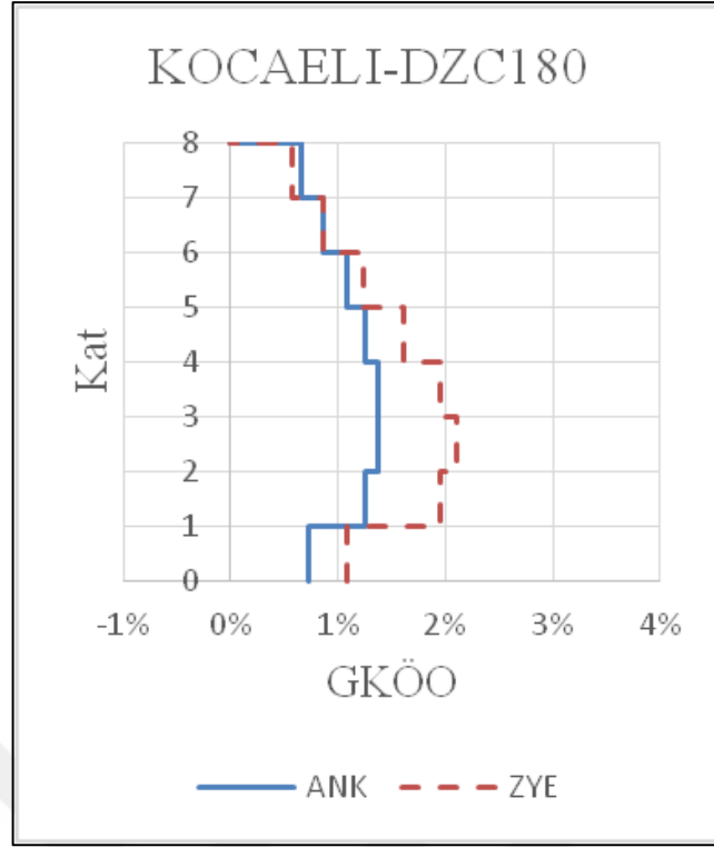
Şekil 4.12 : 8K_B-B GKÖO Karşılaştırılması
