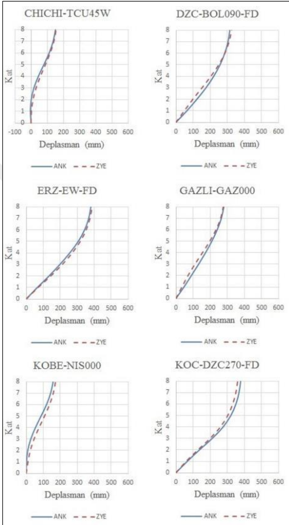
Şekil 8.1 : 8K_2-2 Kat Deplasmanlarının Karşılaştırılması
