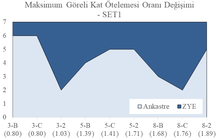
Şekil 4.44 : Maksimum görelî kat ötelemesi oranında artım olasılığı – Set1
