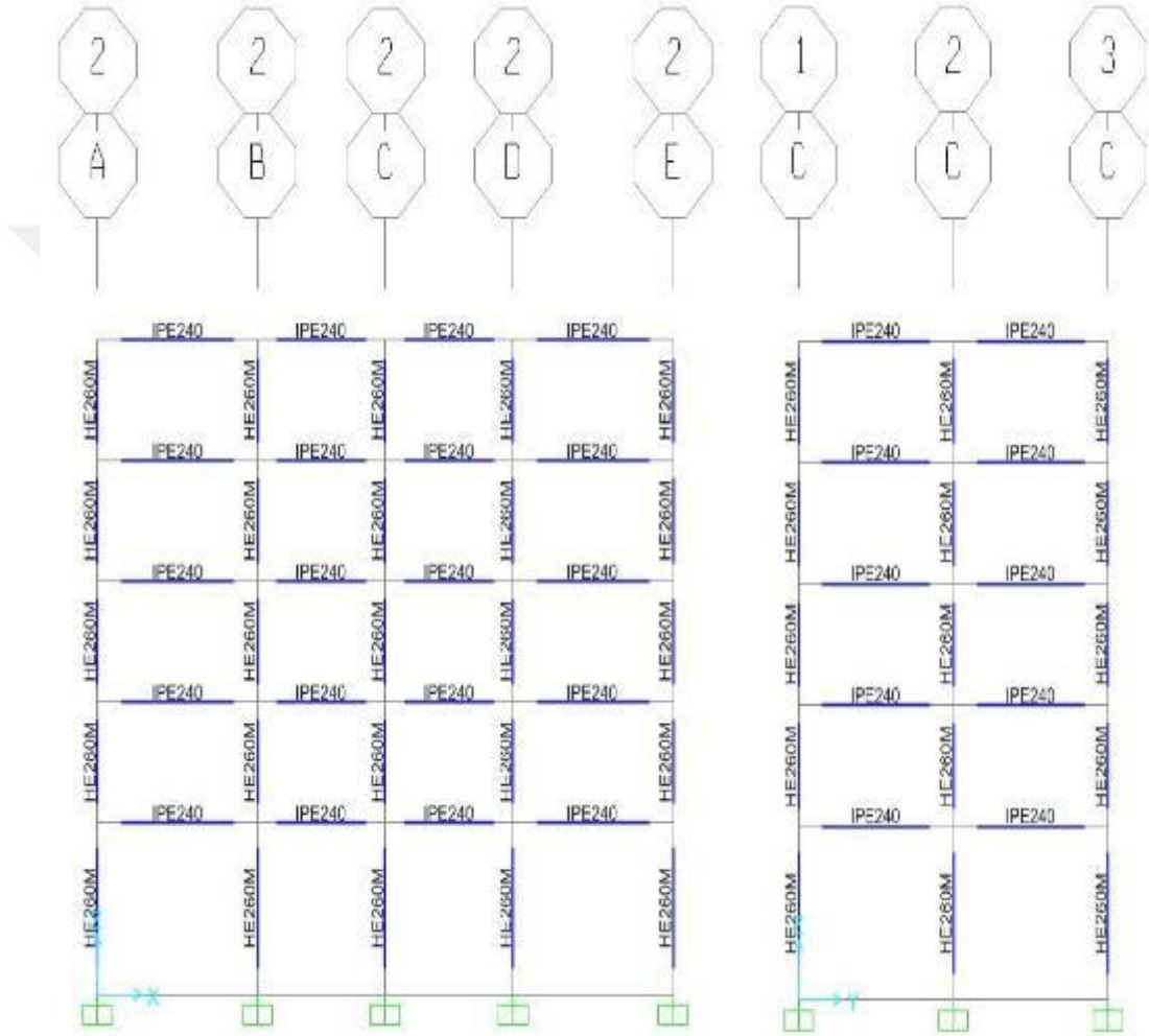
Şekil 2.5: 5 katlı model sistem kesitleri
