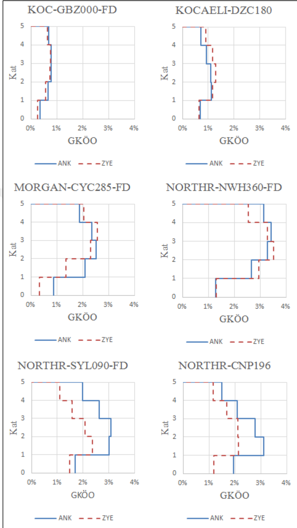
Şekil 8.14 : 5K_B-B GKÖÖ Karşılaştırılması (Devamı)
