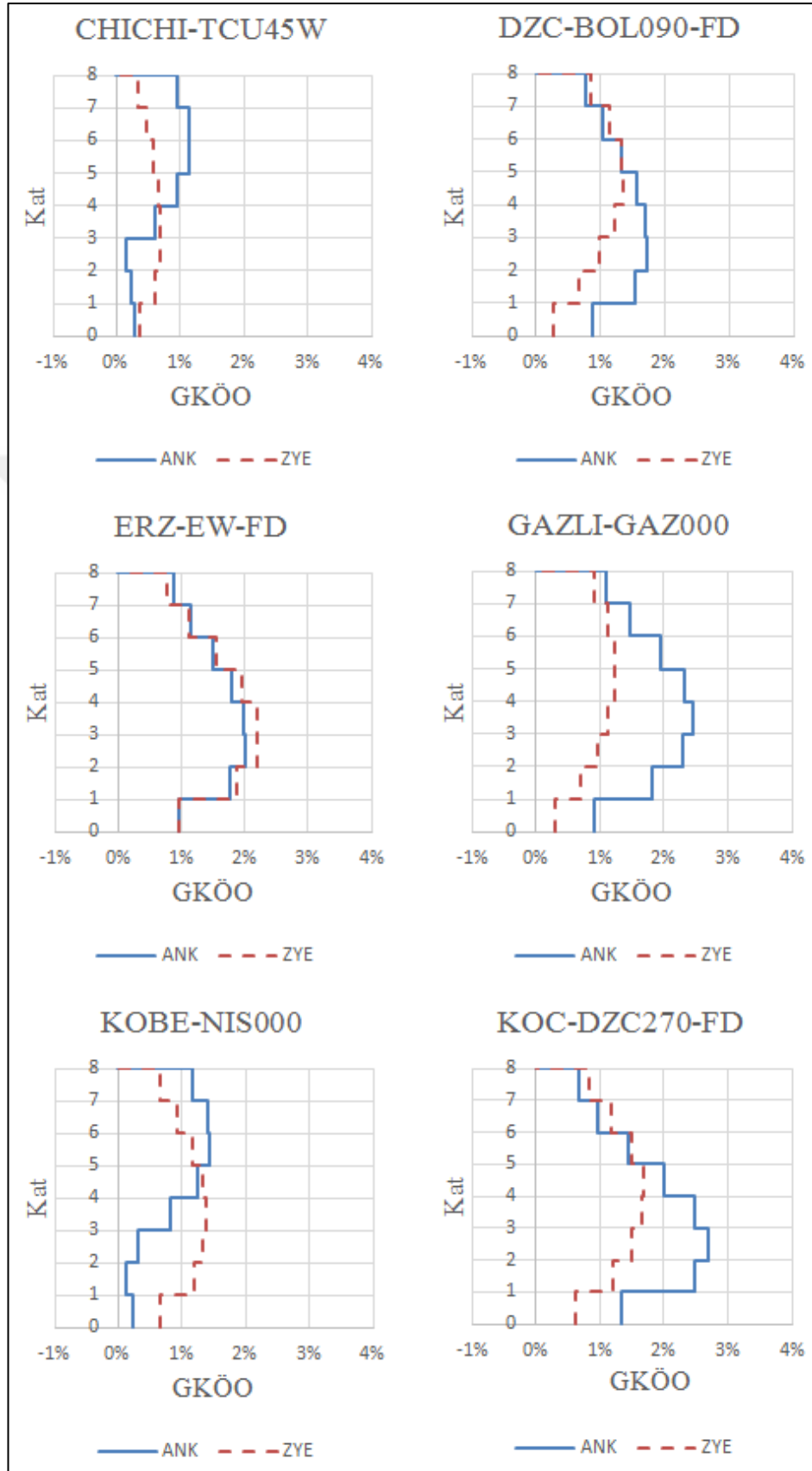
Şekil 8.11 : 8K_B-B GKÖÖ Karşılaştırılması
