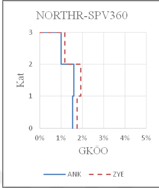
Şekil 4.17 : 3K_2-2 GKÖO Karşılaştırılması
