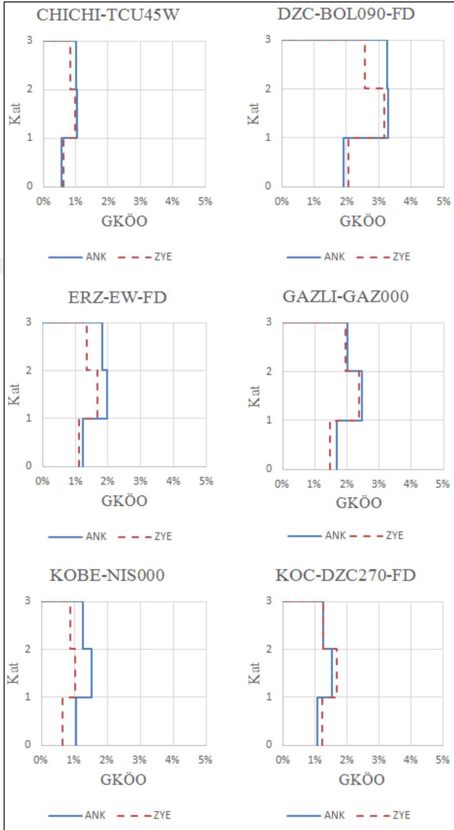
Şekil 8.18 : 3K_C-C GKÖO Karşılaştırılması
