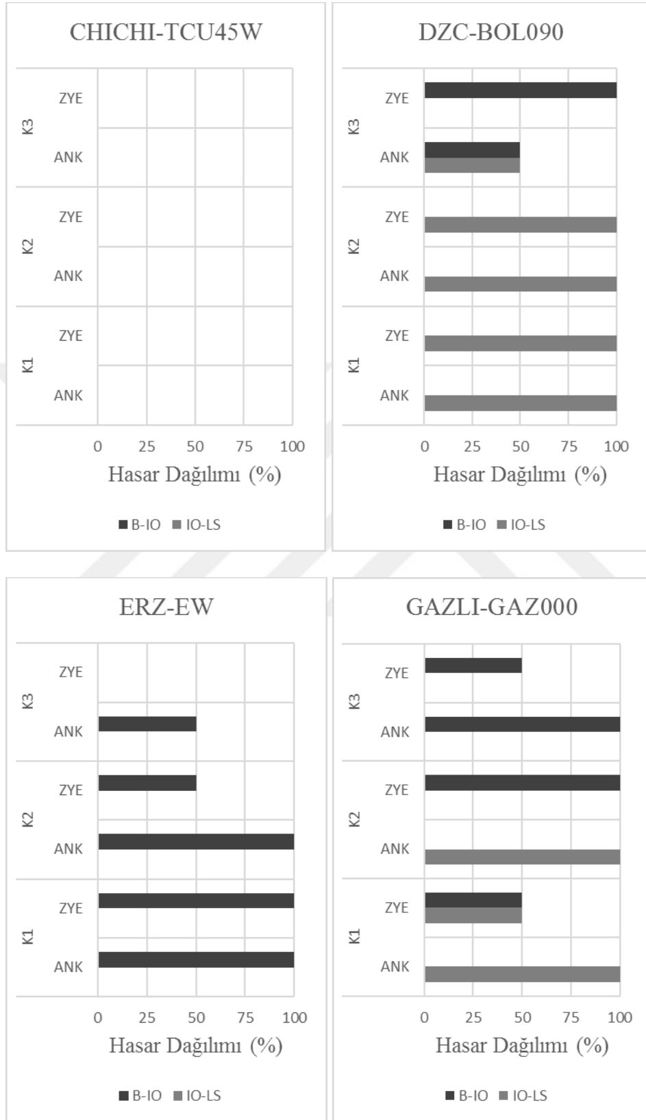
Şekil 4.37 : 3K_C-C Hasar Dağılımlarının Karşılaştırılması
