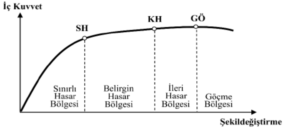
Şekil 3.2: Moment-Eğrilik ilişkisi
