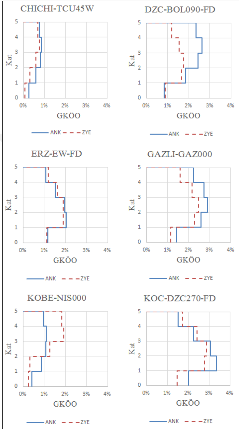
Şekil 8.14 : 5K_B-B GKÖÖ Karşılaştırılması
