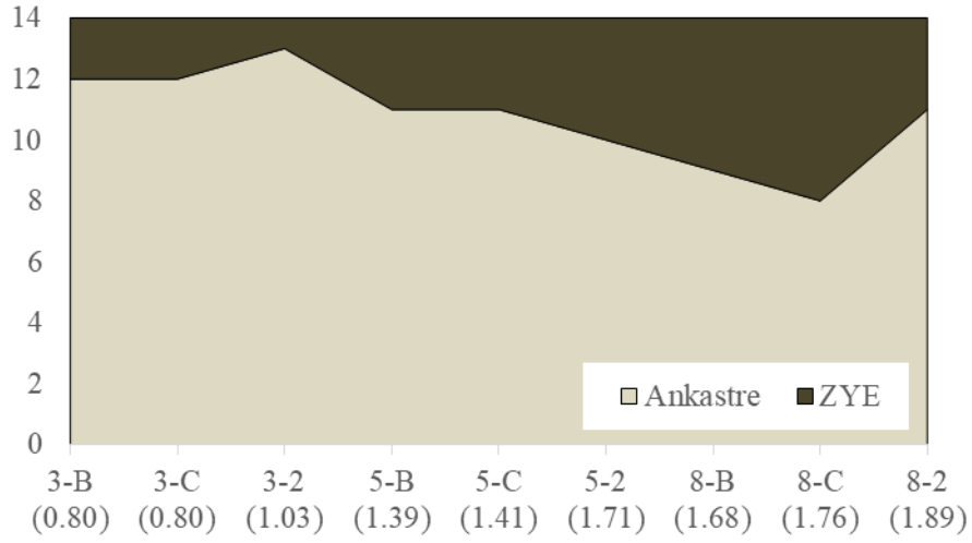
Şekil 4.40 : Maksimum taban kesme kuvveti talebinde artım olasılığı
