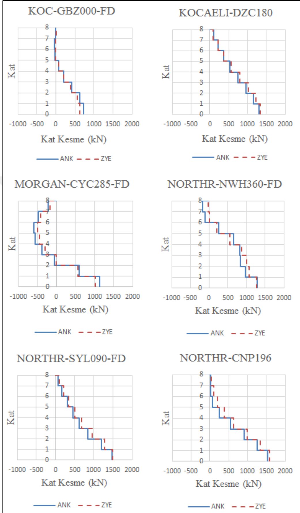
Şekil 8.19 : 8K_2-2 Kat Kesme Kuvvetlerinin Karşılaştırılması (Devamı)
