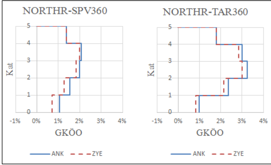
Şekil 8.13 : 5K_2-2 GKÖO Karşılaştırılması (Devamı)
