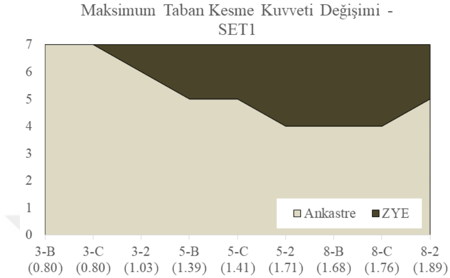
Şekil 4.47 : Maksimum taban kesme kuvveti talebinde artım olasılığı – Set1
