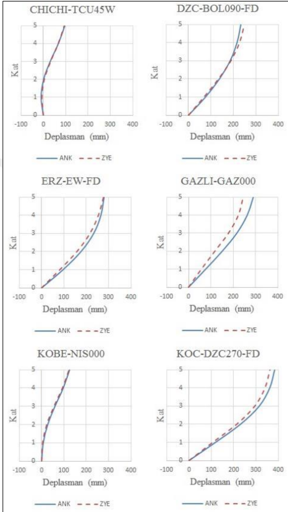
Şekil 8.4 : 5K_2-2 Kat Deplasmanlarının Karşılaştırılması
