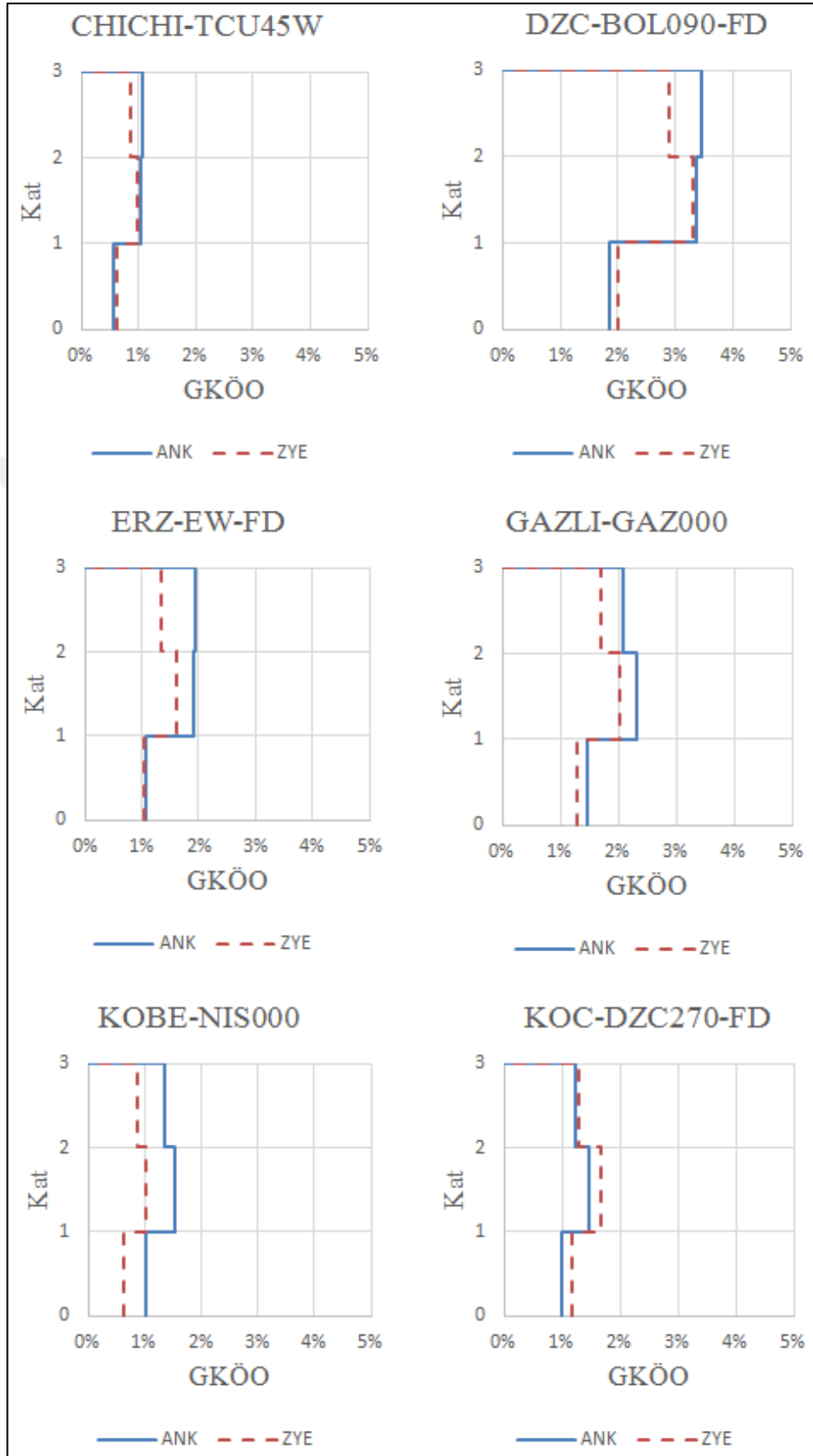
Şekil 8.17 : 3K_B-B GKÖÖ Karşılaştırılması
