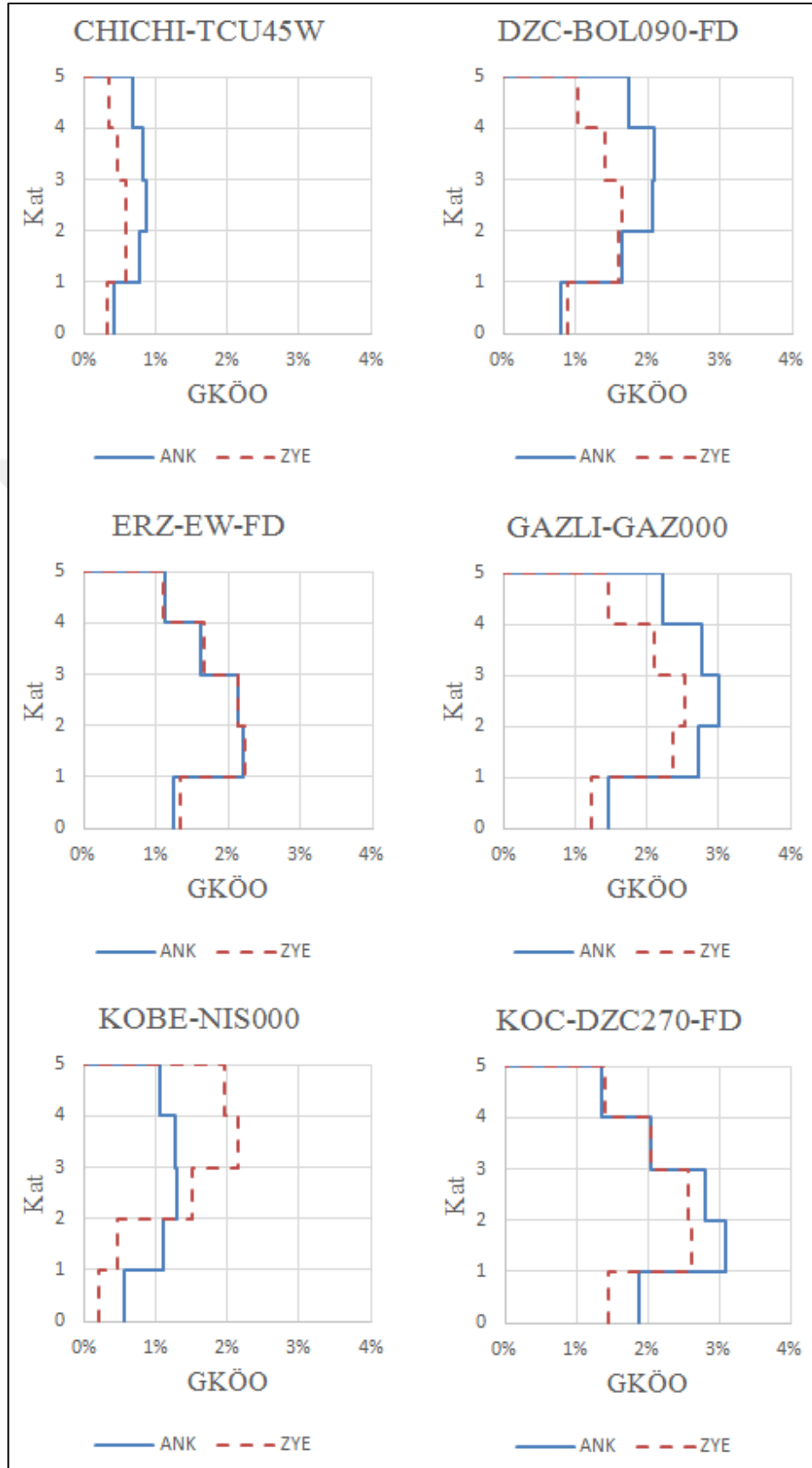
Şekil 8.15 : 5K_C-C GKÖÖ Karşılaştırılması
