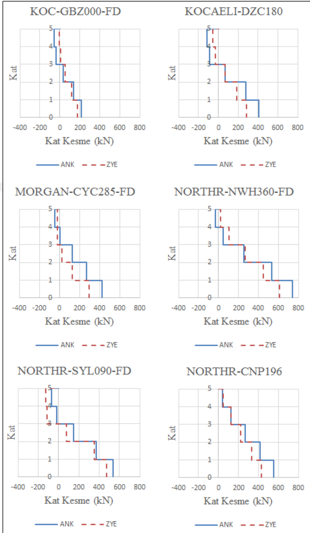
Şekil 8.23 : 5K_B-B Kat Kesme Kuvvetlerinin Karşılaştırılması (Devamı)
