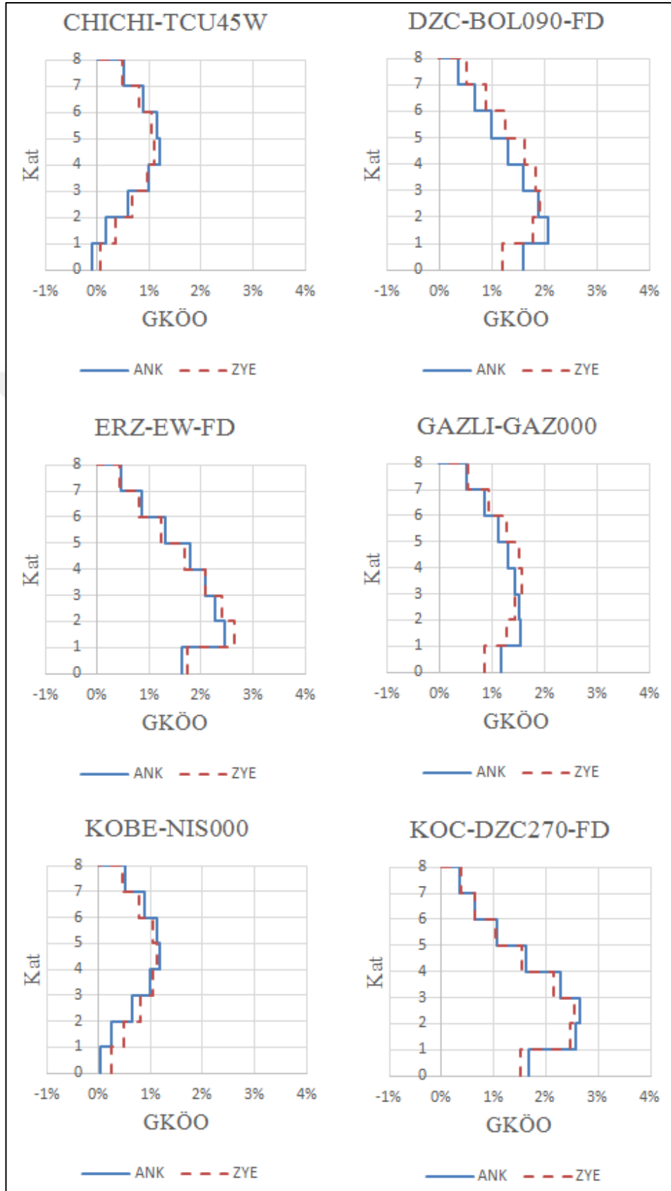
Şekil 8.10 : 8K_2-2 GKÖÖ Karşılaştırılması
