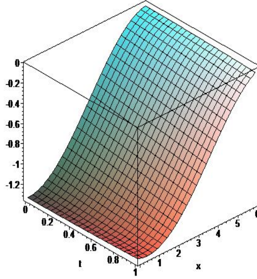
Şekil 5.2. \alpha = 1.0 ve c = 0.5 için kesirli Rosenau-Hyman denkleminin analitik çözümünün grafiği
