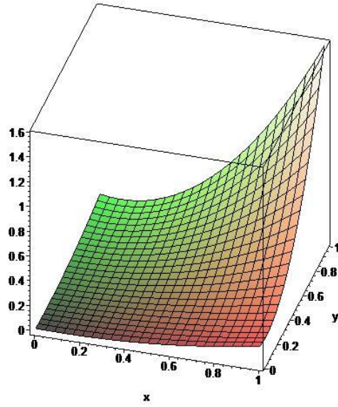
Şekil 5.4. \gamma = 1.0 , p = 0.1 ve t = 0.5 için kesirli ZK (2,2,2) denkleminin yaklaşık çözümünün grafiği
