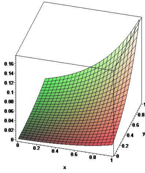
Şekil 5.3. \gamma = 1.0 , p = 0.1 ve t = 0.5 için kesirli ZK (2,2,2) denkleminin analitik çözümünün grafiği
