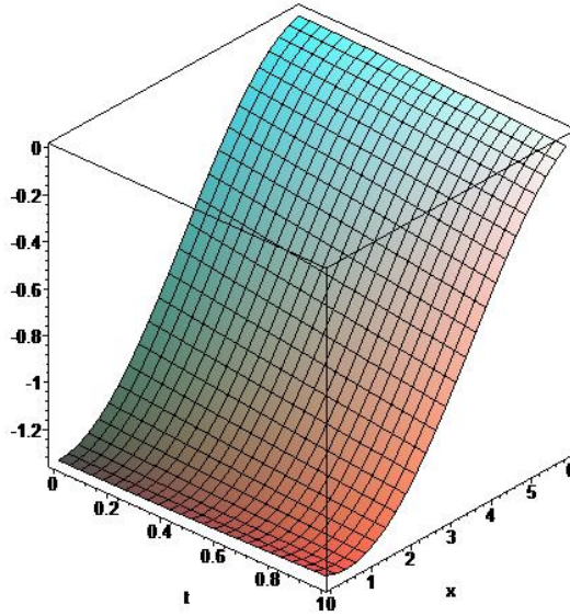
Şekil 5.1. \alpha=1.0 ve c=0.5 için kesirli Rosenau-Hyman denkleminin yaklaşık çözümünün grafiği
