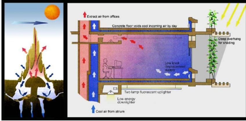
Resim 3.6. Eastgate Merkezi ve termit tepciğinin havalandırma sistemi (URL-29)
