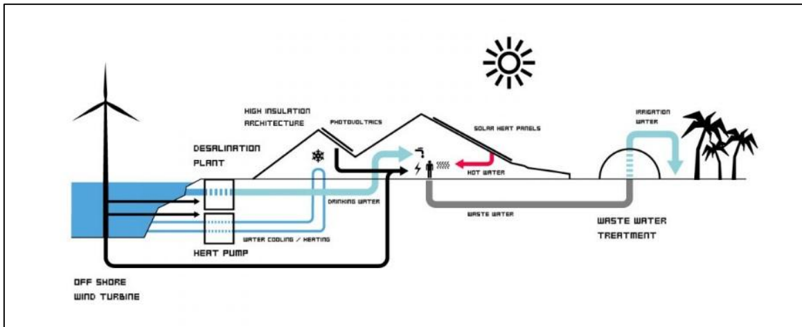
Resim 3.10. Zira Adası su döngüsü (URL-33)
