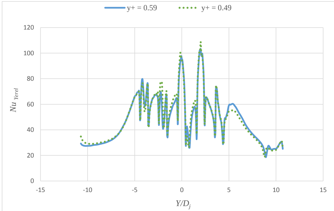
Şekil B4.7. Tümsek şekilli plakada maksimum çapraz akışta ağ doğruluğu, Z_n/D_j = 4 , X_n/D_j = 2 , Re = 8565 , t/D_j = 0.25 , D_d/D_j = 1
