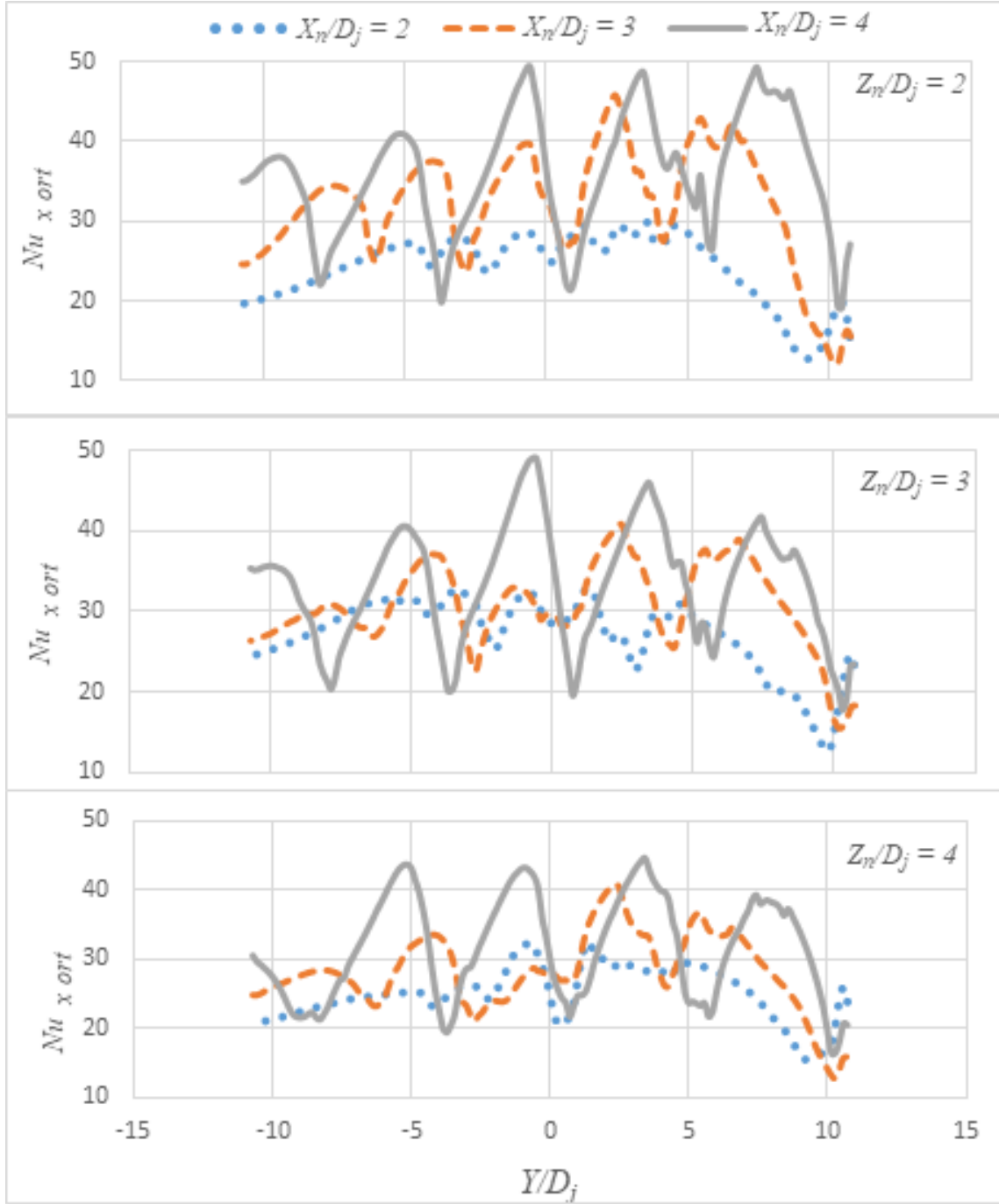
Şekil 4.9. Tümssek şekilli plakada, maksimum çapraz akışta X_n/D_j etkisi, Re = 8565 , D_d/D_j = 1 , t/D_d = 0.25
