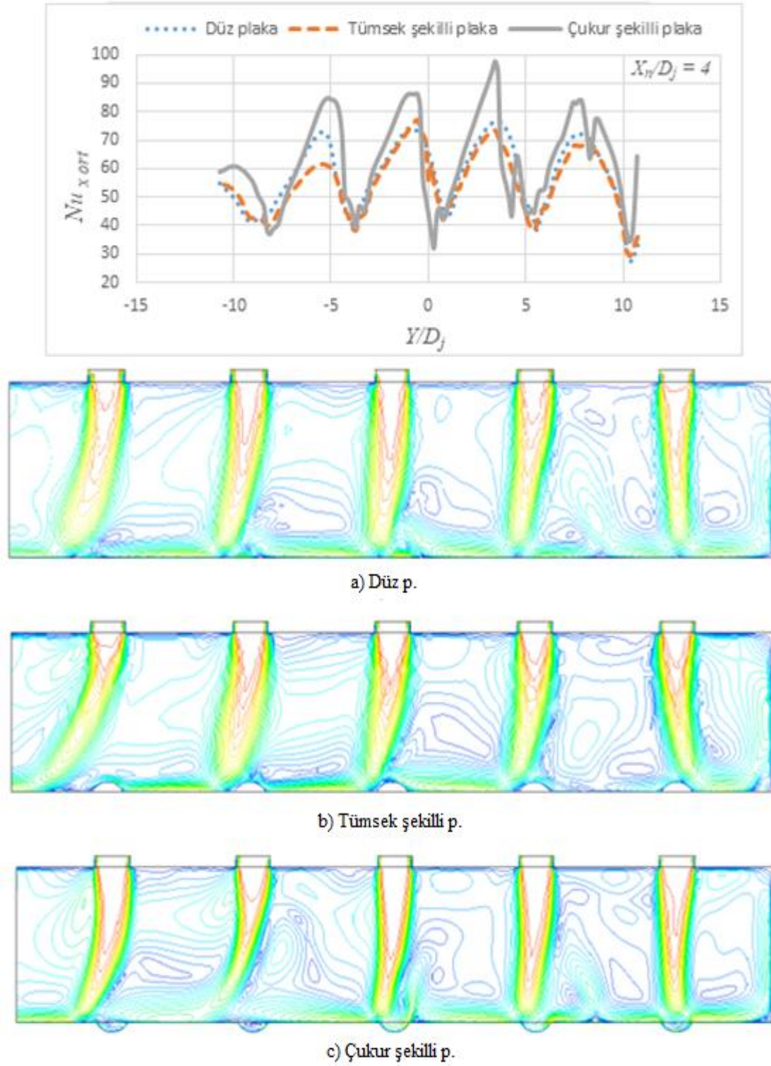
Şekil 4.30. Hız diyagramları, Z_n/D_j = 4 , X_n/D_j = 4 , Re = 20000 , D_d/D_j = 1 , t/D_d = 0.25
