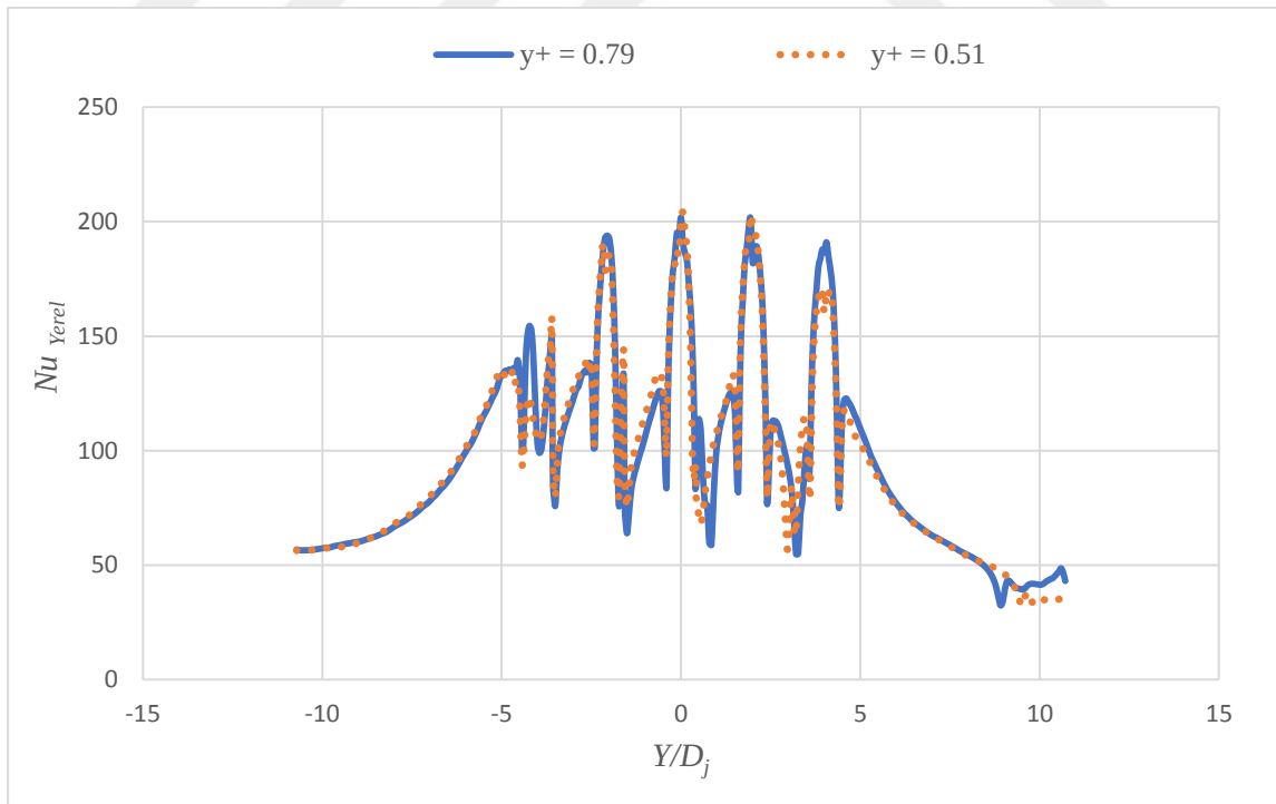
Şekil B5.4. Tümsek şekilli plakada maksimum çapraz akışta ağ doğruluğu, Z_n/D_j = 3 , X_n/D_j = 2 , Re = 20000 , t/D_j = 0.25 , D_d/D_j = 1
