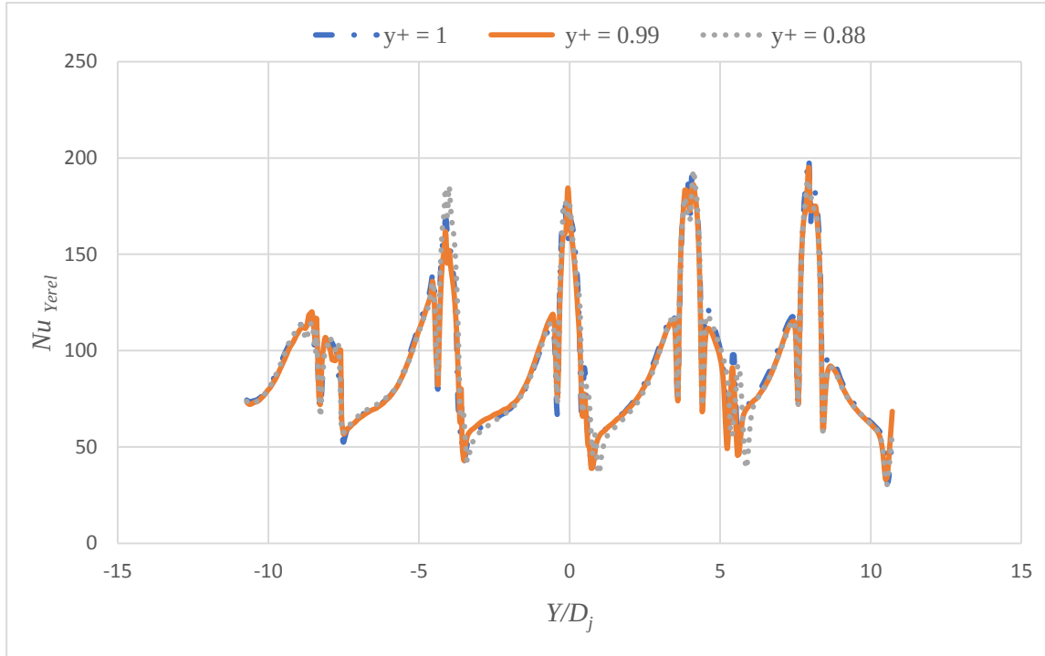
Şekil B5.3. Tümsek şekilli plakada maksimum çapraz akışta ağ doğruluğu, Z_n/D_j = 2 , X_n/D_j = 4 , Re = 20000 , t/D_j = 0.25 , D_d/D_j = 1
