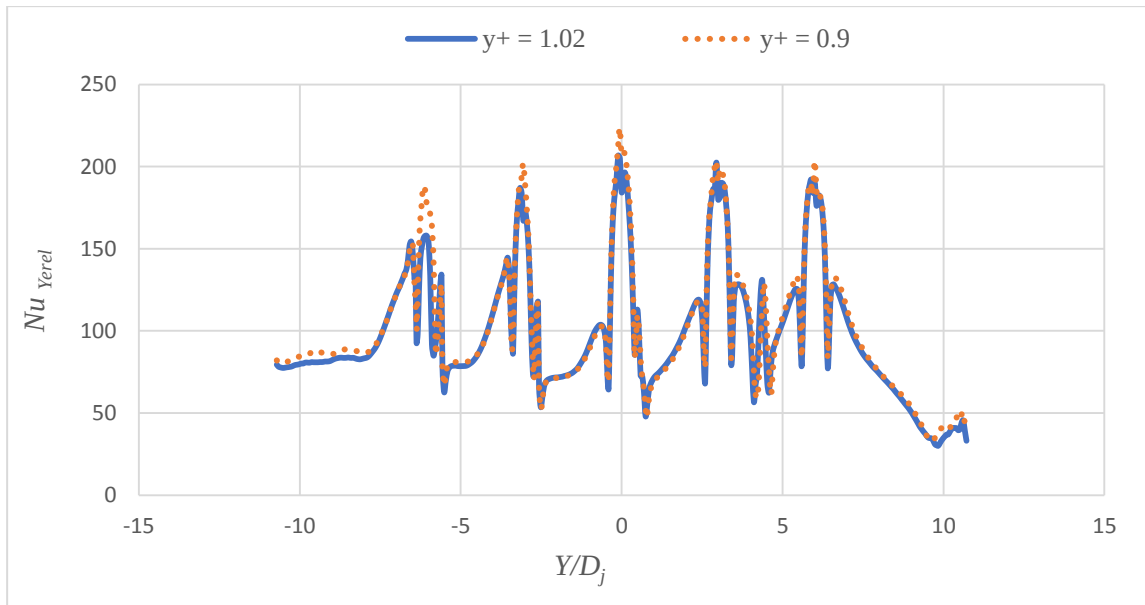
Şekil B5.2. Tümsek şekilli plakada maksimum çapraz akışta ağ doğruluğu, Z_n/D_j = 2 , X_n/D_j = 3 , Re = 20000 , t/D_j = 0.25 , D_d/D_j = 1
