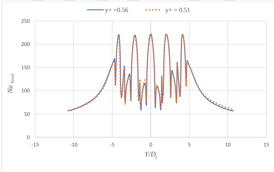
Şekil B7.4. Tümsek şekilli plakada minimum çapraz akışta ağ doğruluğu, Z_n/D_j = 3 , X_n/D_j = 2 , Re = 20000 , t/D_j = 0.25 , D_d/D_j = 1.43
