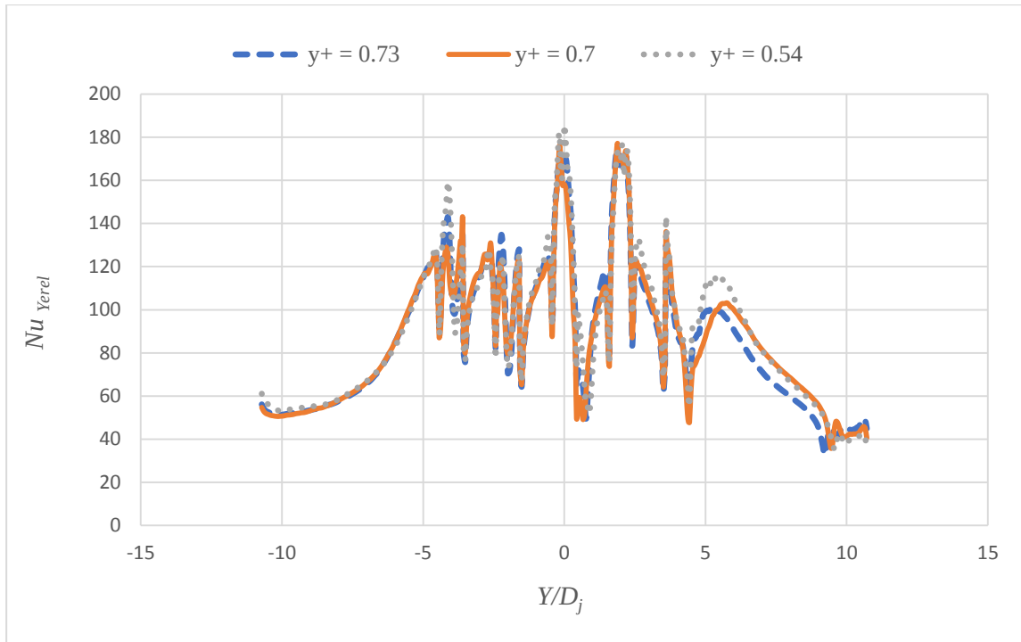
Şekil B5.7. Tümsek şekilli plakada maksimum çapraz akışta ağ doğruluğu, Z_n/D_j = 4 , X_n/D_j = 2 , Re = 20000 , t/D_j = 0.25 , D_d/D_j = 1
