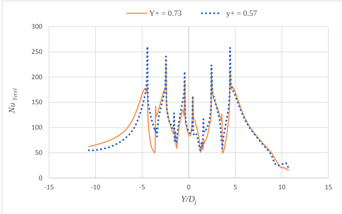
Şekil B9.7. Çukur şekilli plakada maksimum çapraz akışta ağ doğruluğu, Z_n/D_j = 4 , X_n/D_j = 2 , Re = 20000 , t/D_j = 0.25 , D_d/D_j = 1
