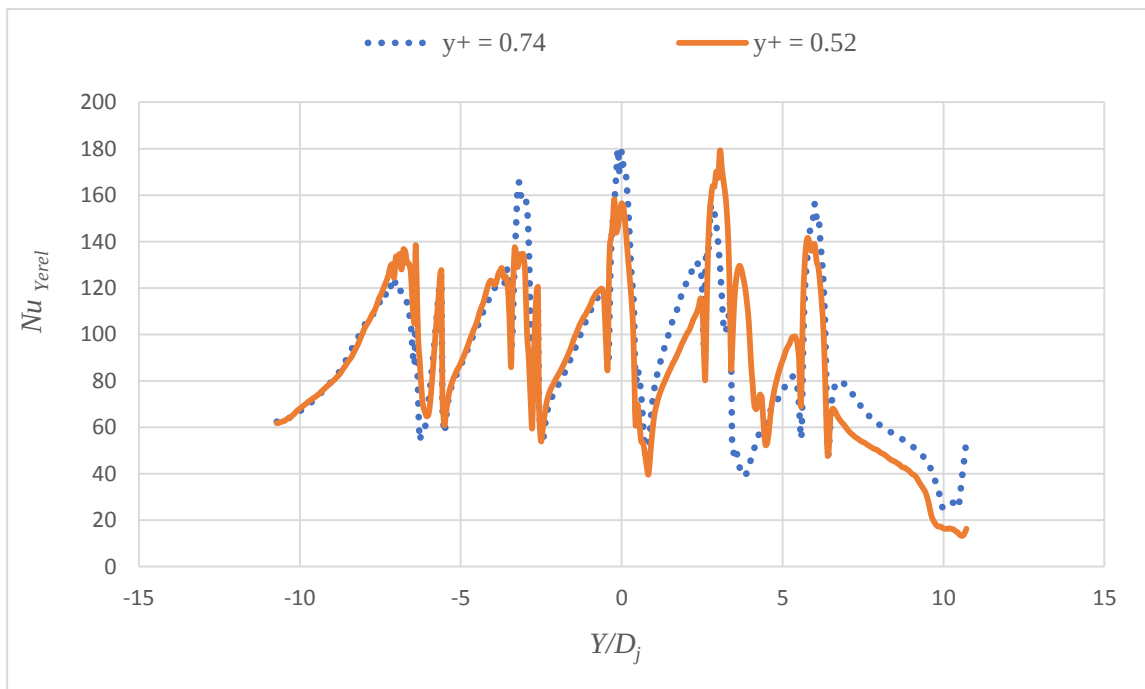
Şekil B5.8. Tümsek şekilli plakada maksimum çapraz akışta ağ doğruluğu, Z_n/D_j = 4 , X_n/D_j = 3 , Re = 20000 , t/D_j = 0.25 , D_d/D_j = 1
