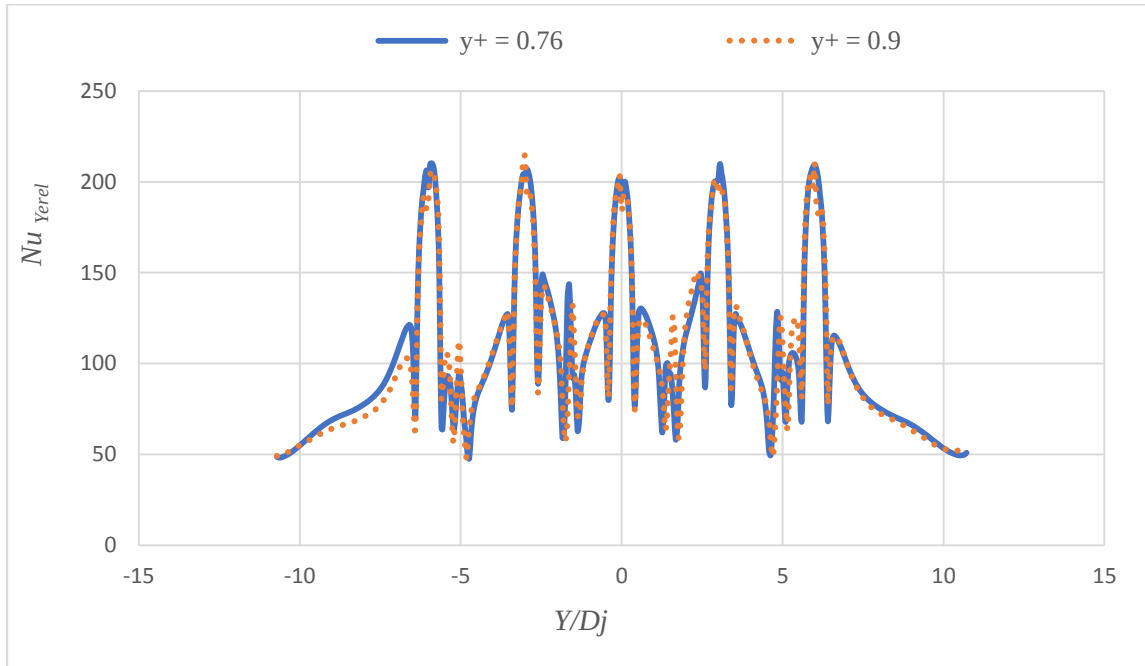
Şekil B6.2. Tümsek şekilli plakada minimum çapraz akışta ağ doğruluğu, Z_n/D_j = 2 , X_n/D_j = 3 , Re = 20000 , t/D_j = 0.25 , D_d/D_j = 1
