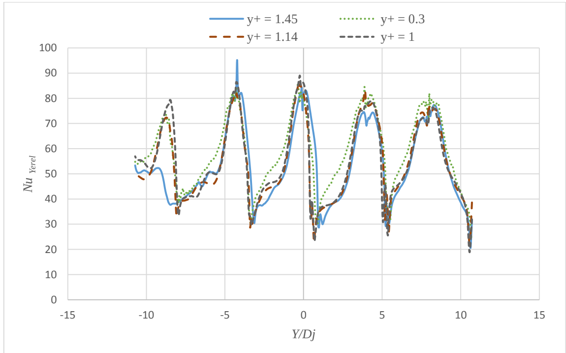
Şekil B1.2. Düz plakada maksimum çapraz akışta ağ doğruluğu, Z_n/D_j = 2 , X_n/D_j = 4 , Re = 8565
