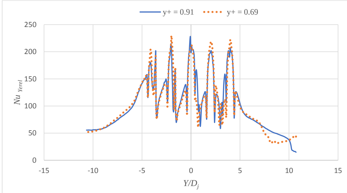
Şekil B5.1. Tümsek şekilli plakada maksimum çapraz akışta ağ doğruluğu, Z_n/D_j = 2 , X_n/D_j = 2 , Re = 20000 , t/D_j = 0.25 , D_d/D_j = 1
