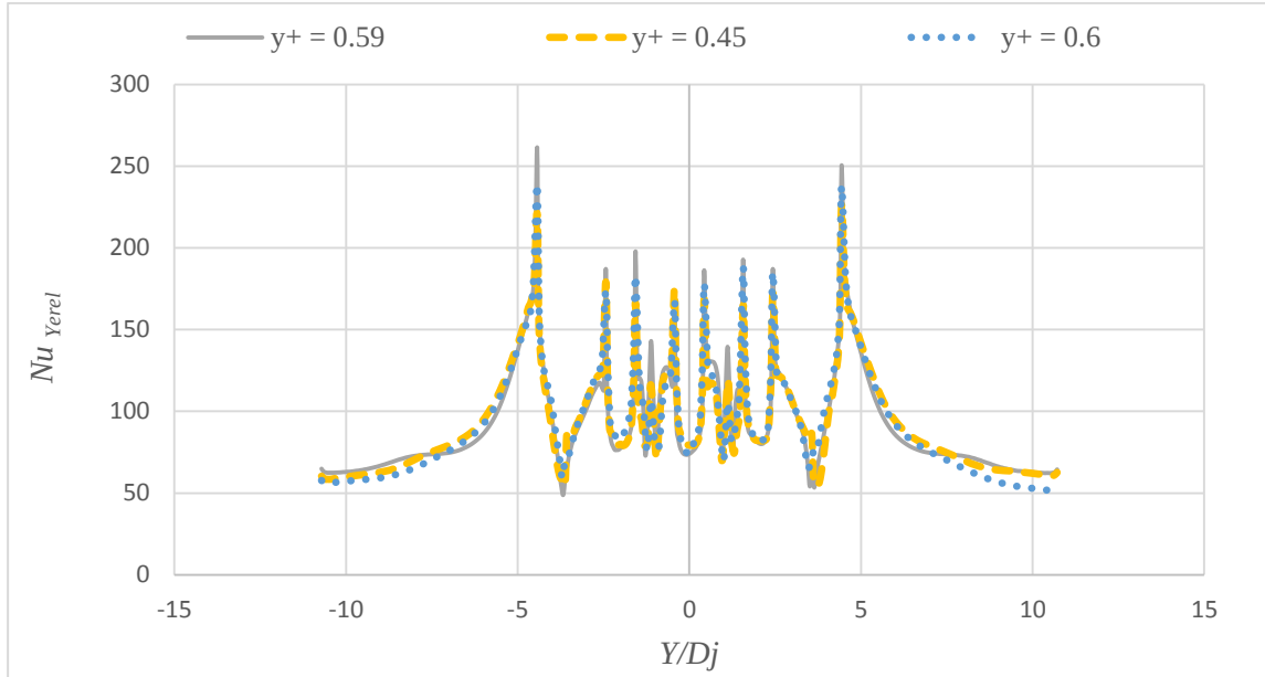
Şekil B10.1. Çukur şekilli plakada minimum çapraz akışta ağ doğruluğu, Z_n/D_j = 2 , X_n/D_j = 2 , Re = 20000 , t/D_j = 0.25 , D_d/D_j = 1
