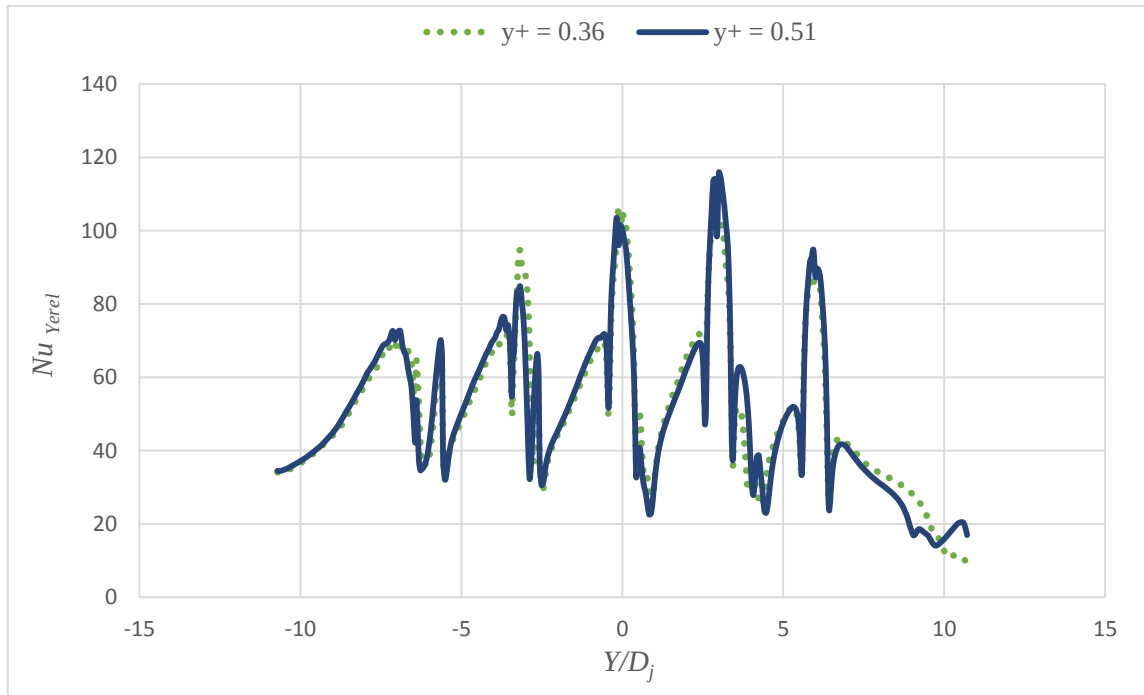
Şekil B4.8. Tümsek şekilli plakada maksimum çapraz akışta ağ doğruluğu, Z_n/D_j = 4 , X_n/D_j = 3 , Re = 8565 , t/D_j = 0.25 , D_d/D_j = 1
