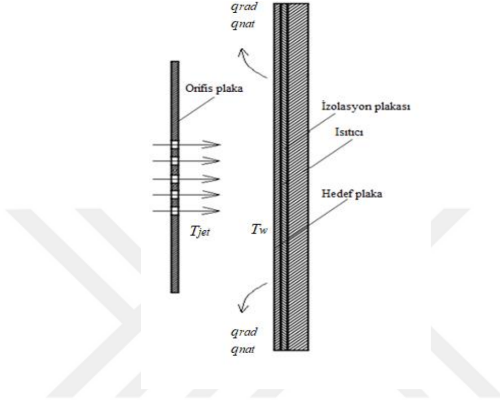
Şekil 3.3. Deney düzeneği test detayı
