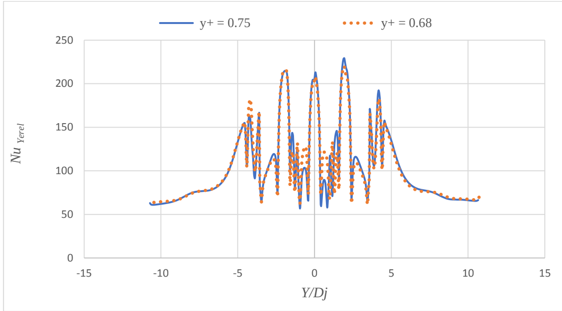
Şekil B6.1. Tümsek şekilli plakada minimum çapraz akışta ağ doğruluğu, Z_n/D_j = 2 , X_n/D_j = 2 , Re = 20000 , t/D_j = 0.25 , D_d/D_j = 1
