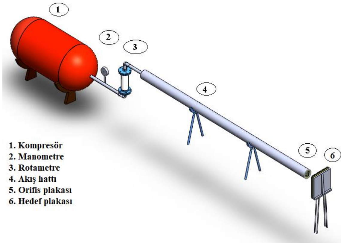
Şekil 3.2. Deney düzeneği tasarımı
