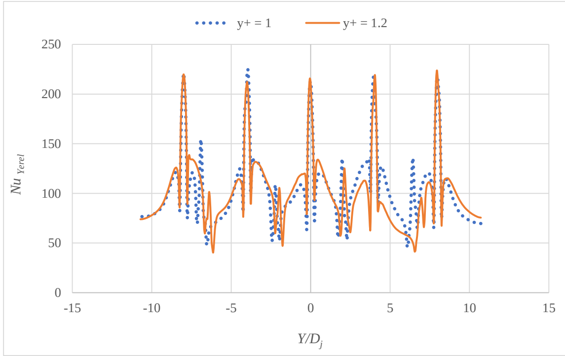
Şekil B8.3. Tümsek şekilli plakada minimum çapraz akışta ağ doğruluğu, Z_n/D_j = 2 , X_n/D_j = 4 , Re = 20000 , t/D_j = 0.25 , D_d/D_j = 0.57
