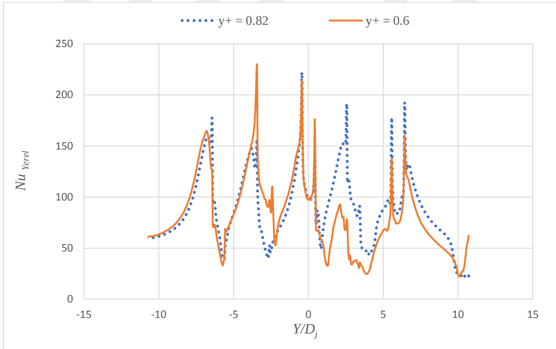
Şekil B9.8. Çukur şekilli plakada maksimum çapraz akışta ağ doğruluğu, Z_n/D_j = 4 , X_n/D_j = 3 , Re = 20000 , t/D_j = 0.25 , D_d/D_j = 1
