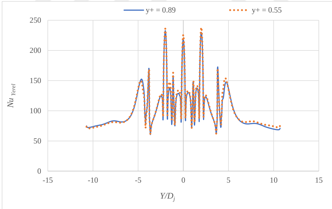
Şekil B8.4. Tümsek şekilli plakada minimum çapraz akışta ağ doğruluğu, Z_n/D_j = 3 , X_n/D_j = 2 , Re = 20000 , t/D_j = 0.25 , D_d/D_j = 0.5
