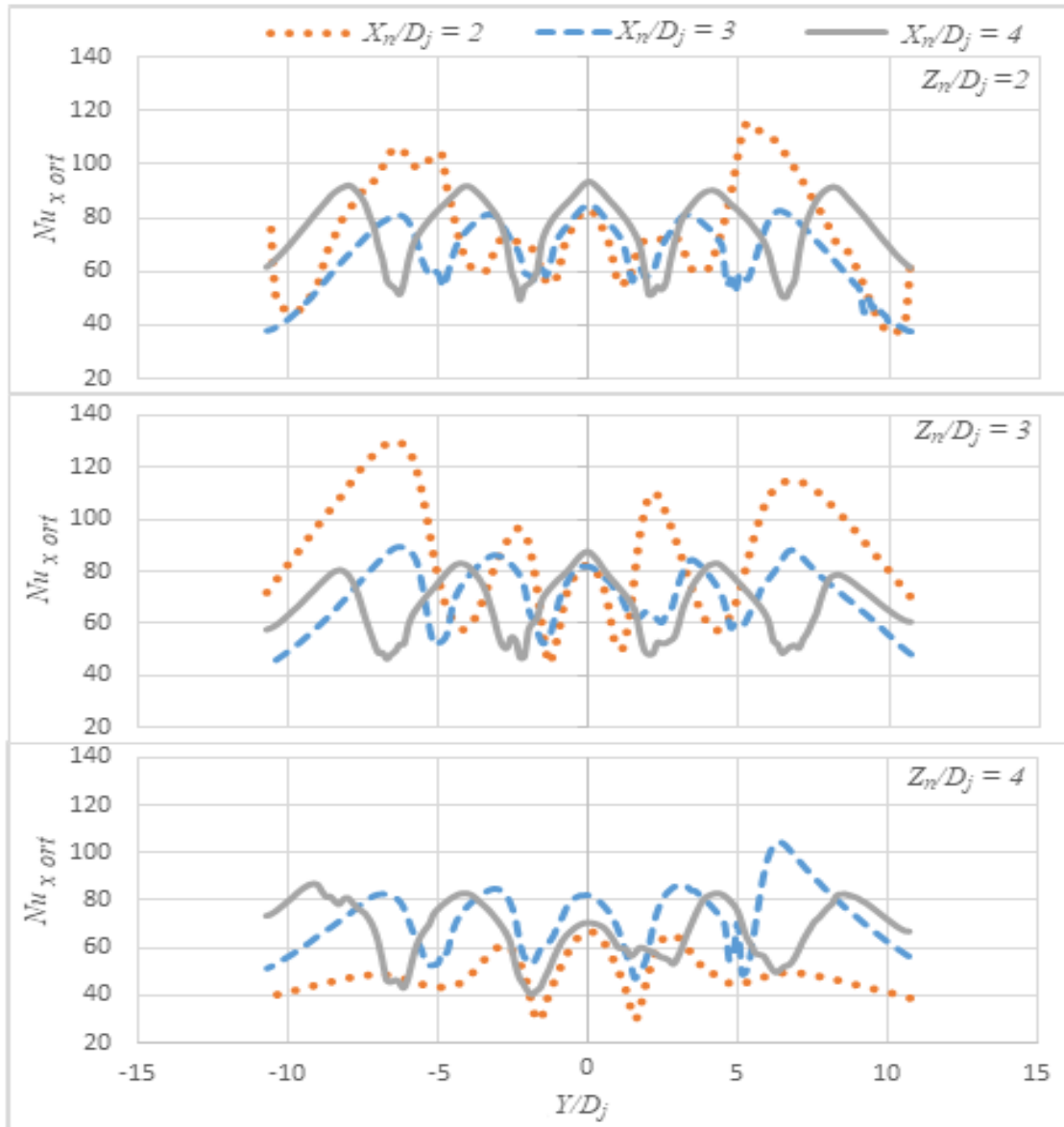
Şekil 4.32. Düz plakada minimum çapraz akışta X_n/D_j etkisi, Re = 20000
