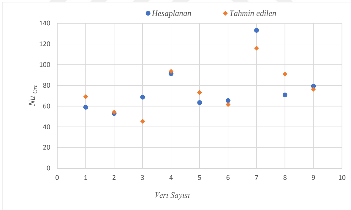
Şekil 4.70. Minimum çapraz akış tümsek şekilli plaka (Denklem 4.1)
