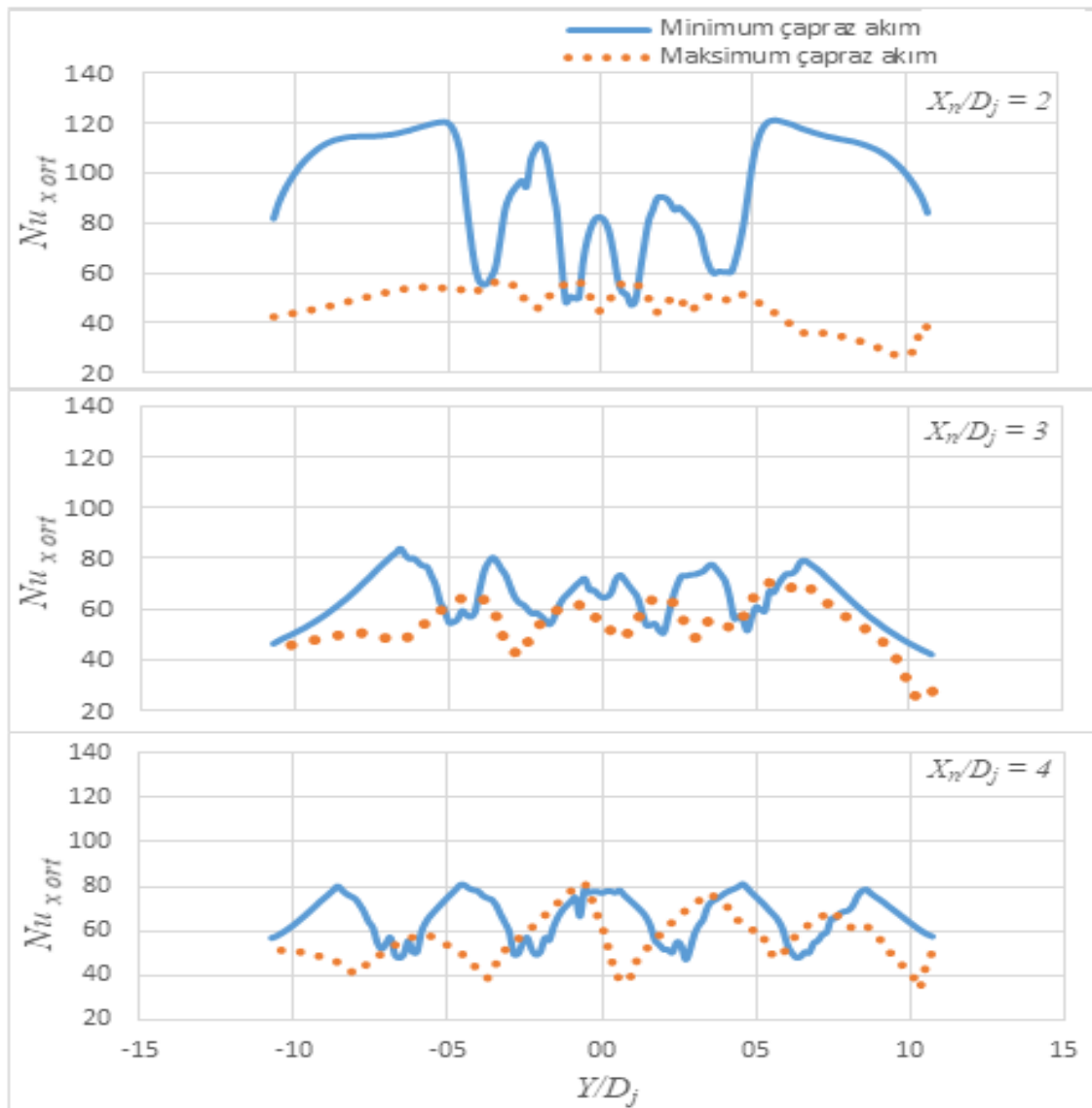
Şekil 4.56. Tümssek şekilli plakada sıra ortalamalı Nusselt sayısı, Z_n/D_j = 3 , Re = 20000 D_d/D_j = 1 , t/D_d = 0.25
