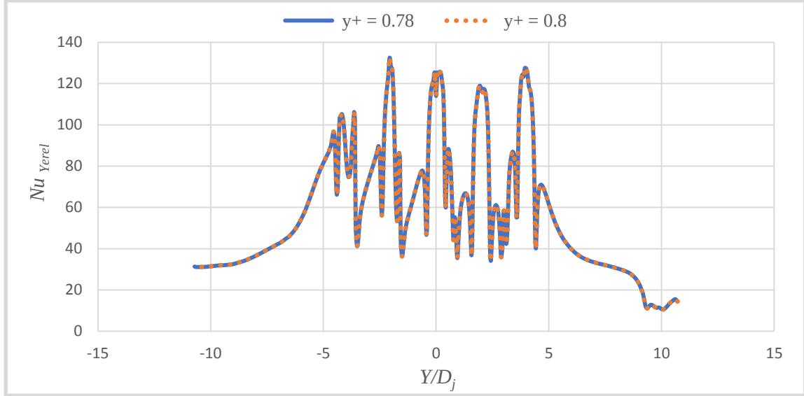
Ek B4. Tümsek şekilli plakada maksimum çapraz akışta ağ doğruluğu, D_d/D_j = 1 , t/D_d = 0.25 , Re = 8565
