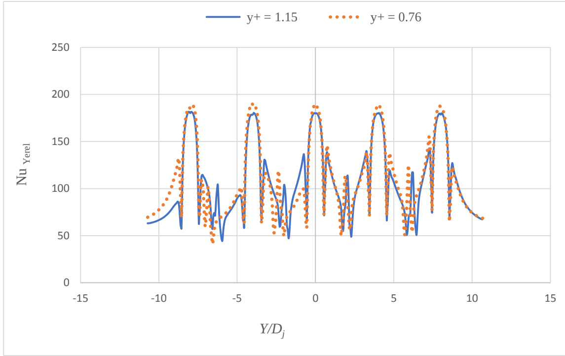
Şekil B7.3. Tümsek şekilli plakada minimum çapraz akışta ağ doğruluğu, Z_n/D_j = 2 , X_n/D_j = 4 , Re = 20000 , t/D_j = 0.25 , D_d/D_j = 1.43
