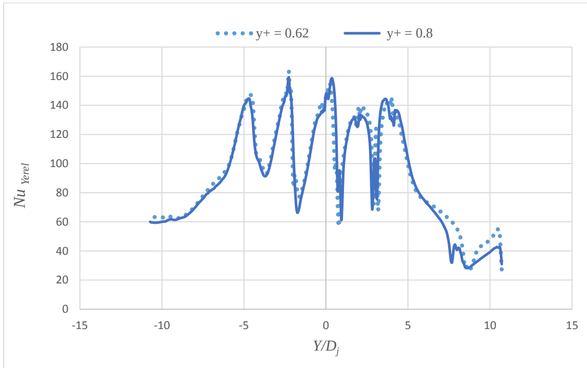
Şekil B2.1. Düz plakada maksimum çapraz akışta ağ doğruluğu, Z_n/D_j = 2 , X_n/D_j = 2 , Re = 20000
