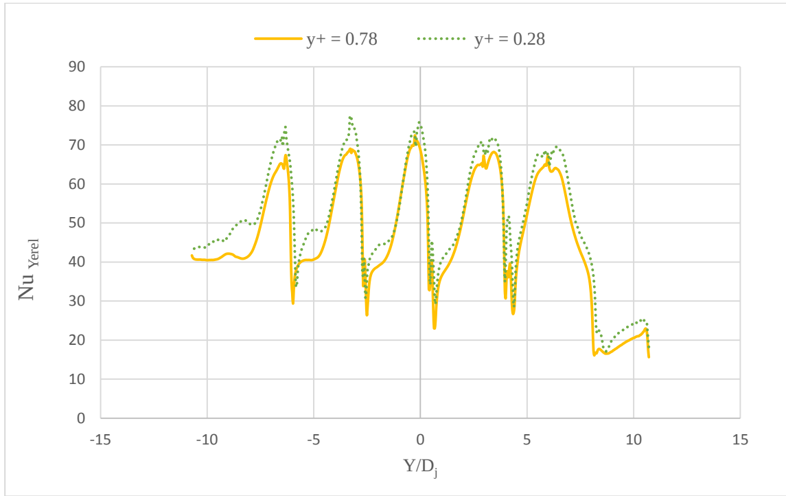
Şekil B1.1. Düz plakada maksimum çapraz akışta ağ doğruluğu, Z_n/D_j = 2 , X_n/D_j = 3 , Re = 8565
