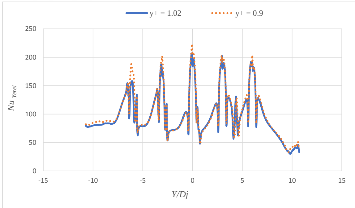
Şekil B4.2. Tümsek şekilli plakada maksimum çapraz akışta ağ doğruluğu, Z_n/D_j = 2 , X_n/D_j = 3 , Re = 8565 , t/D_j = 0.25 , D_d/D_j = 1
