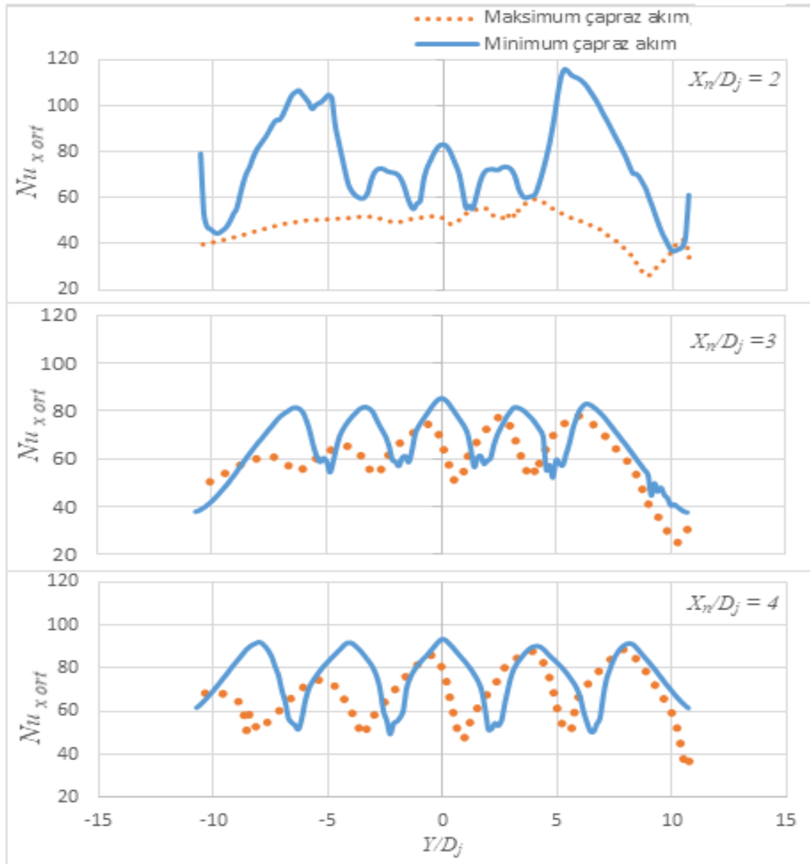
Şekil 4.52. Düz plakada çapraz akışın etkisi, Z_n/D_j = 2 , Re = 20000
