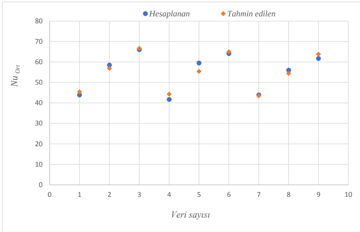
Şekil 4.69. Maksimum çapraz akış çukur şekilli plaka (Denklem 4.1)
