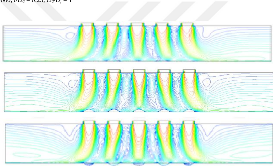
Şekil 4.50. Farklı plakaların minimum çapraz akışta hız dağılımı ve akım çizgileri, Z_n/D_j = 2 , X/D_j = 2 , Re = 20000 , t/D_d = 0.25 , D_d/D_j = 1
