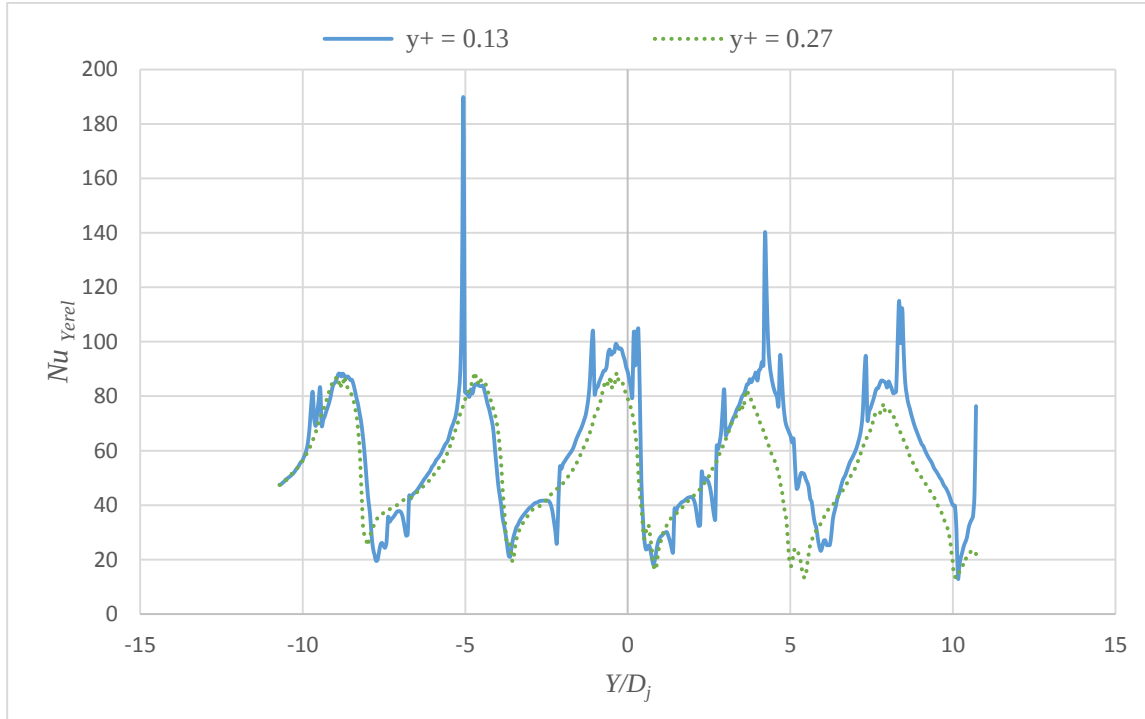
Şekil B1.7. Düz plakada maksimum çapraz akışta ağ doğruluğu, Z_n/D_j = 4 , X_n/D_j = 4 , Re = 8565
