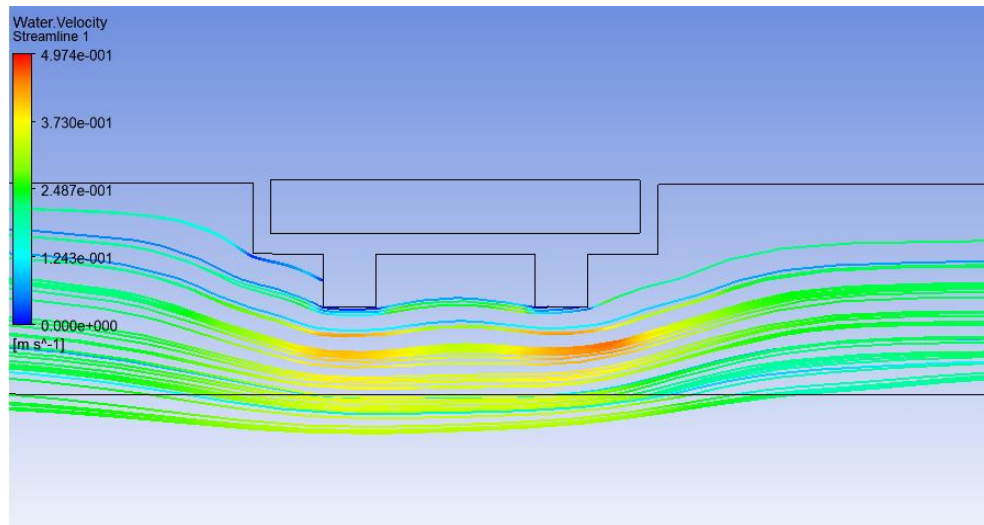
Şekil 5.24. k-\epsilon türbülans modeline ait 70 lt/sn debi ve 30,0 cm yaklaşım akım derinliği için elde edilen akım iplikcikleri
