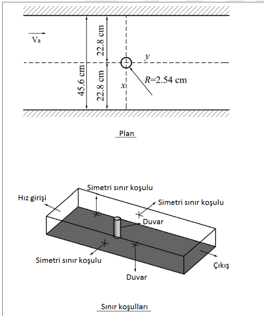
Şekil 2.13. Zhu ve Liu (2012)'nin çalışmasına ait sayısal modelin planı ve sınır koşulları
