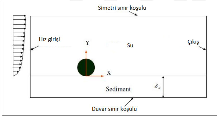
Şekil 2.1. Zhao ve diğerleri (2007)'nin çalışmasına ait sayısal modelin geometrisi ve sınır koşulları
