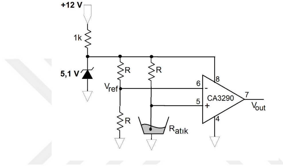
Şekil 6.13 Atık seviyesi belirleme sistemi şematik gösterimi
