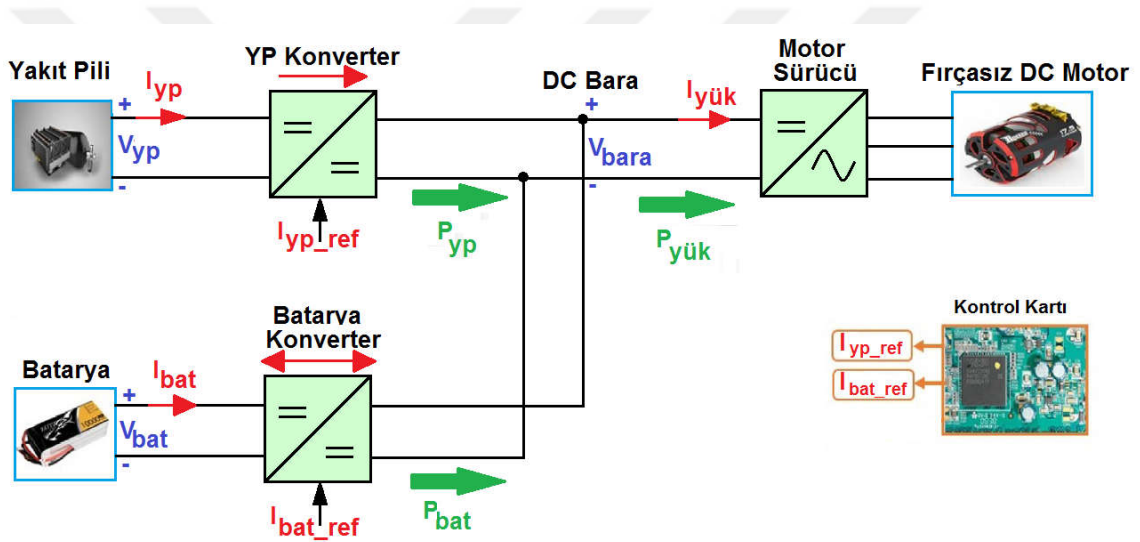
Şekil 5.1 Aktif kontrollü hibrit güç sistemi genel yapısı
