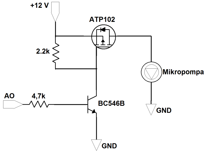
Şekil 6.12 Pompa DC-DC dönüştürücüsünün besleme kontrolü
