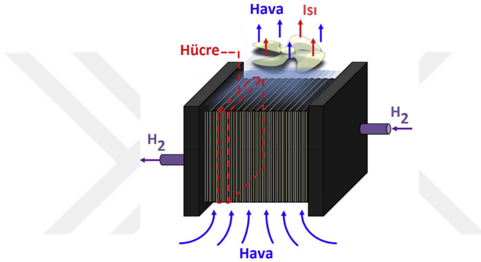
Şekil 3.5 Hava solumalı PEM yakıt pili sistemi genel yapısı [108]
