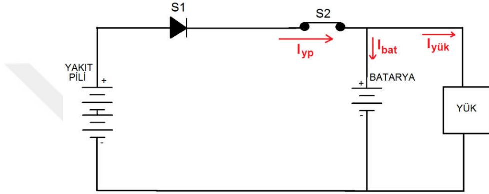
Şekil 6.16 I. çalışma aralığına ait eşdeğer devre
