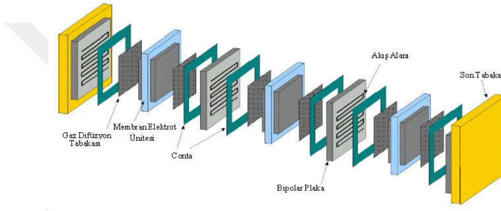
Şekil 3.3 Yakıt pili modülü ve alt bileşenleri
