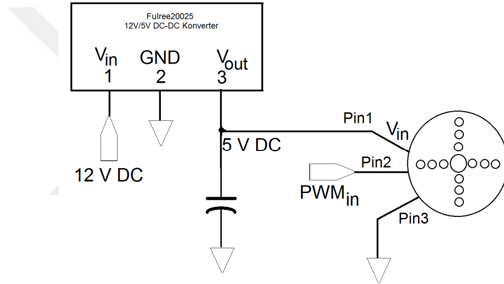
Şekil 6.14 Servo motor besleme ve kontrol şematik gösterimi
