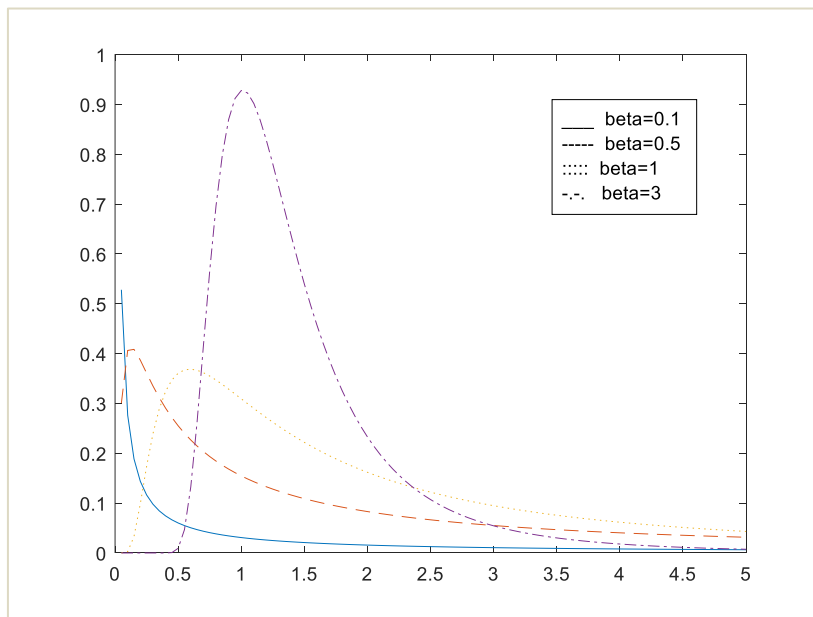
Şekil 2.6. DIW(\sigma, \beta) dağılımının \beta 'nin farklı değerleri için pdf grafiği.
