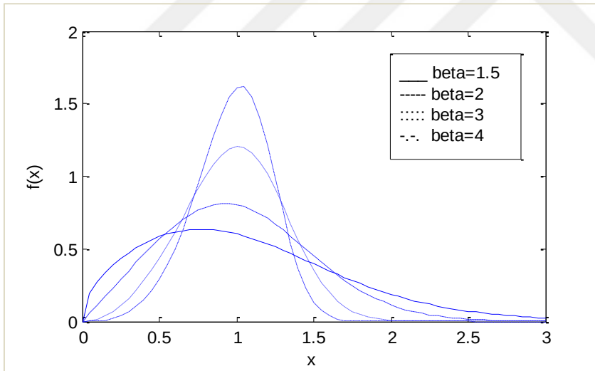
Şekil 2.2. DW(\sigma, \beta) dağılımının \beta 'nın farklı değerleri için pdf grafiği.
