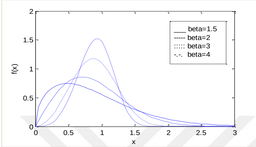
Şekil 2.1. W(\sigma, \beta) dağılımının \beta 'nın farklı değerleri için pdf grafiği.
