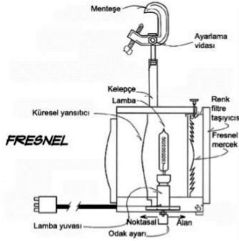
Şekil 25. Fresnel Mercekli Aydınlatmanın Teknik Yapısı
