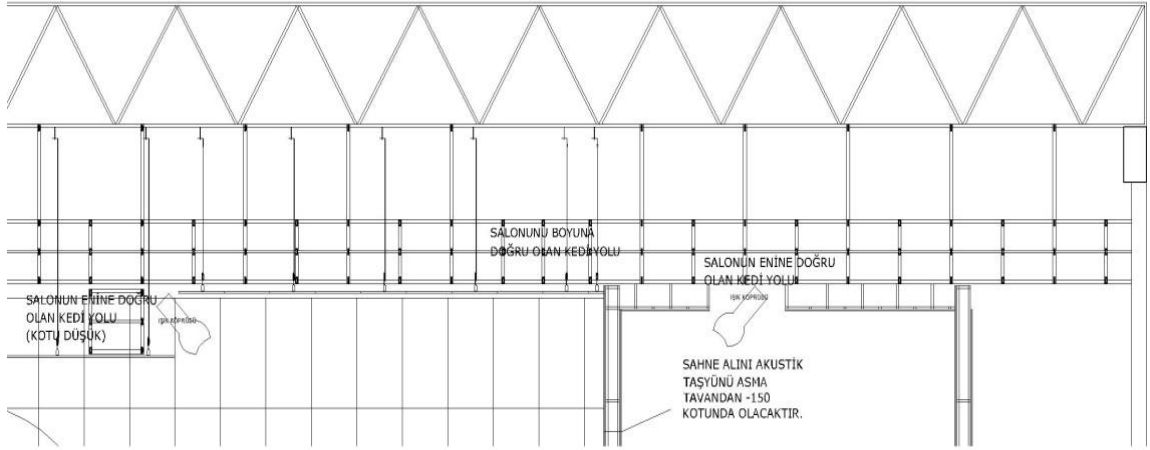
Şekil 68. Sahne Aydınlatma Kesiti( EK 9 )
