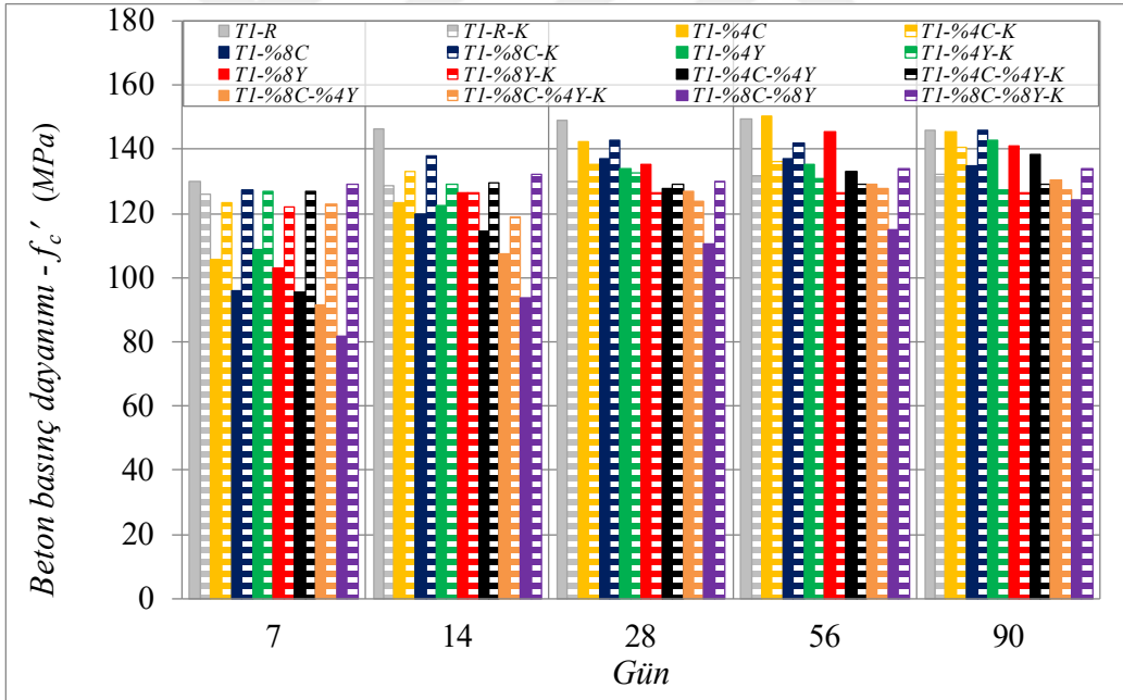
Őekil 3.6: Tip-1 karıŐımı i in buhar k r n n beton basın  dayanımına etkisi.
