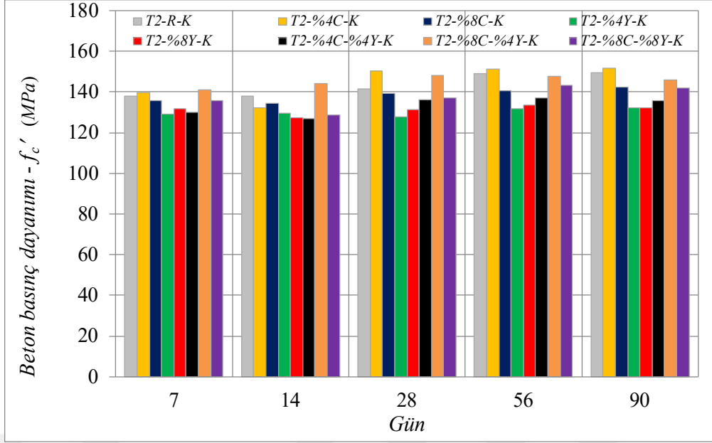
Şekil 3.16: Buhar kürlü karışımlarda CT ve/veya YFC kullanımlarının basınç dayanımına etkisi ( Tip-2 )
