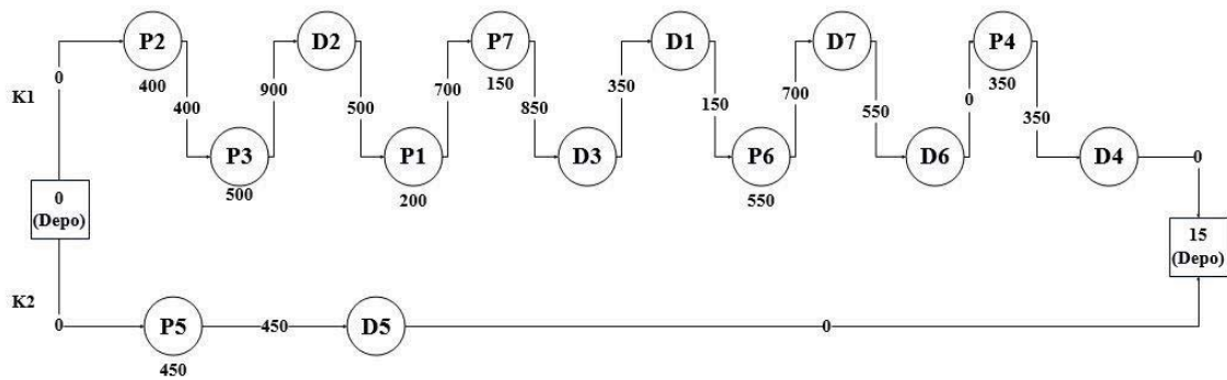
Şekil 7. K1 (dizel) ve K2 (elektrikli) araçlarının izledikleri rota
