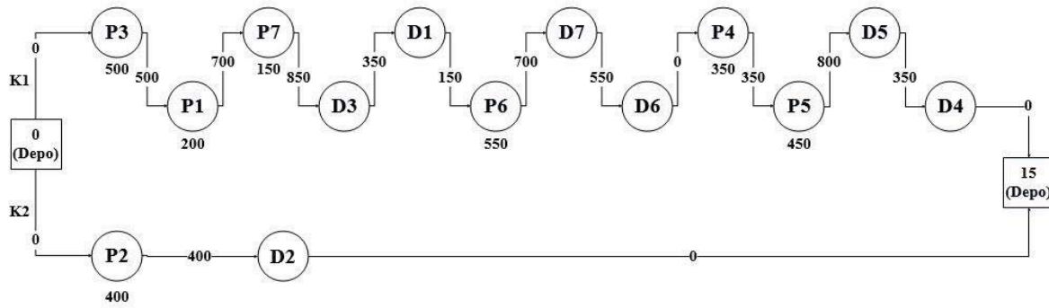
Şekil 13. K1 (dizel) ve K2 (elektrikli) araçlarının izledikleri rota
