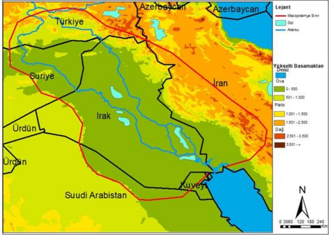
Şekil 12: Mezopotamya ve Yakın Çevresinin Fiziki Haritası
