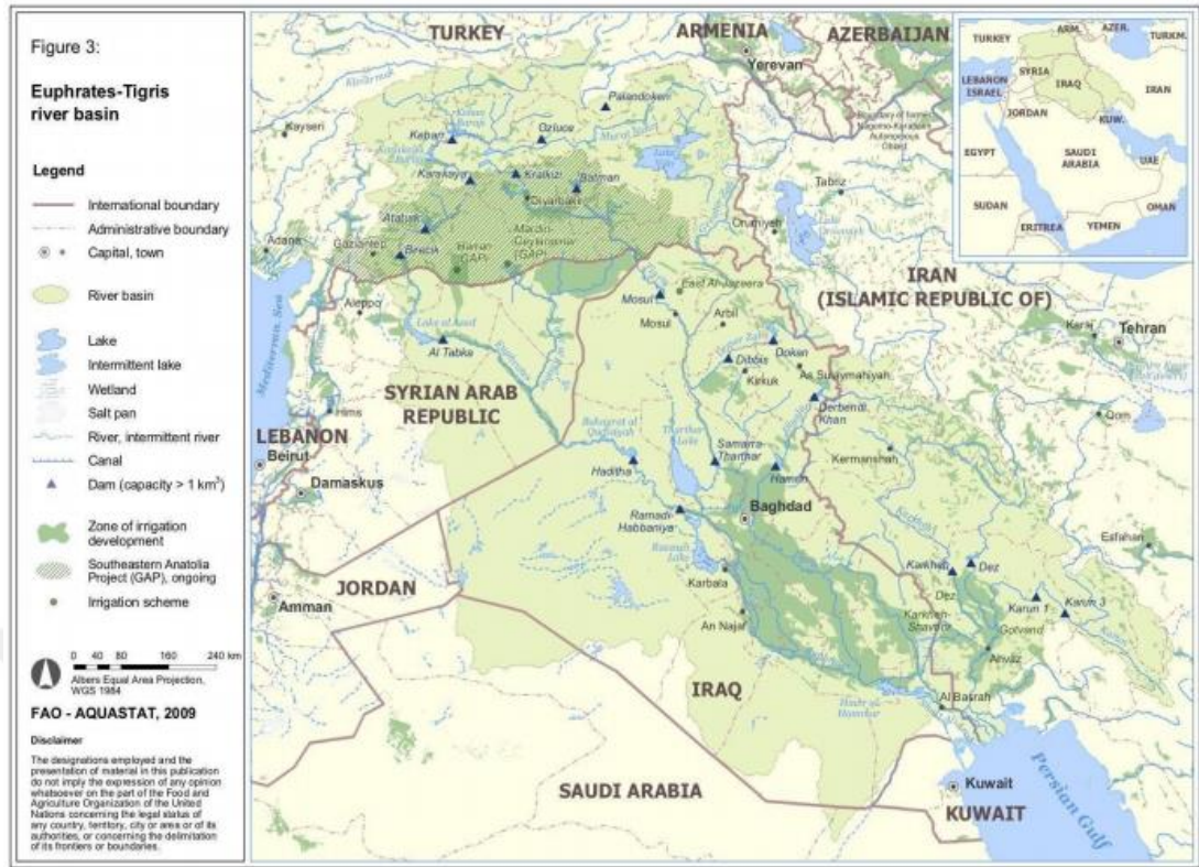
Şekil 3: Dicle ve Fırat Havzası Haritası 34
