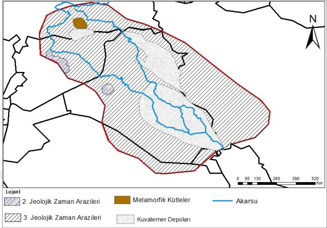
Şekil 10: Mezopotamya Coğrafyası'nın Jeoloji Haritası 203
