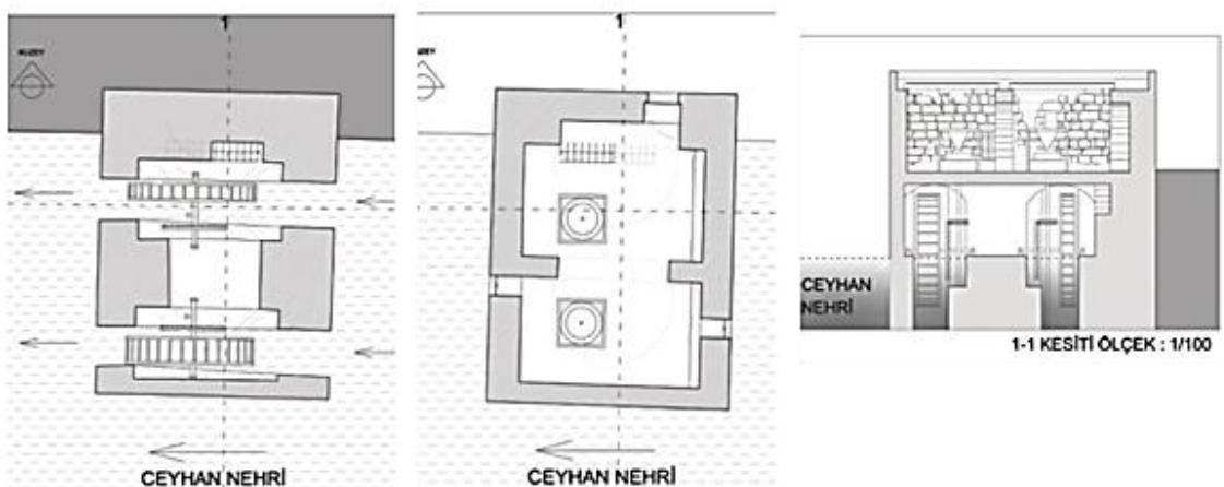
Şekil 142. 1. Dönem restitüsyon plan ve kesitleri
