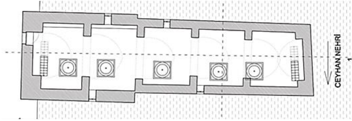
Şekil 144. Misis Doğu Değirmeni restitüsyon plan
