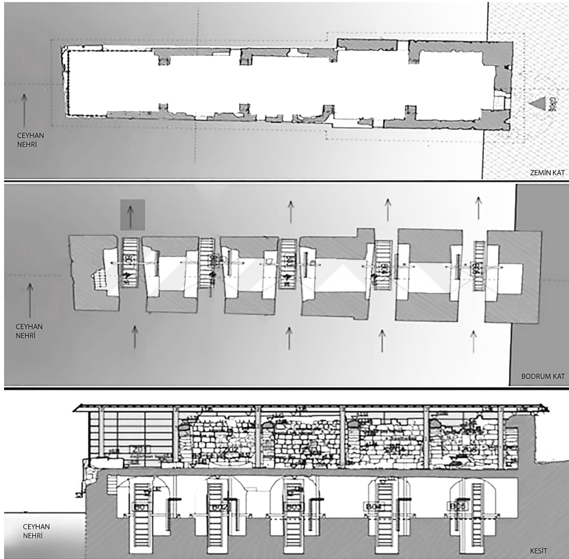
Şekil 146. Misis Doğu Değirmeni restorasyon projesi; planlar ve boyuna kesit
