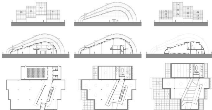
Şekil 41. Baksı Müzesi Ana Bina Z Kat, 1. Kat, Ara Kat Planları, Kesit ve Görünüşleri
