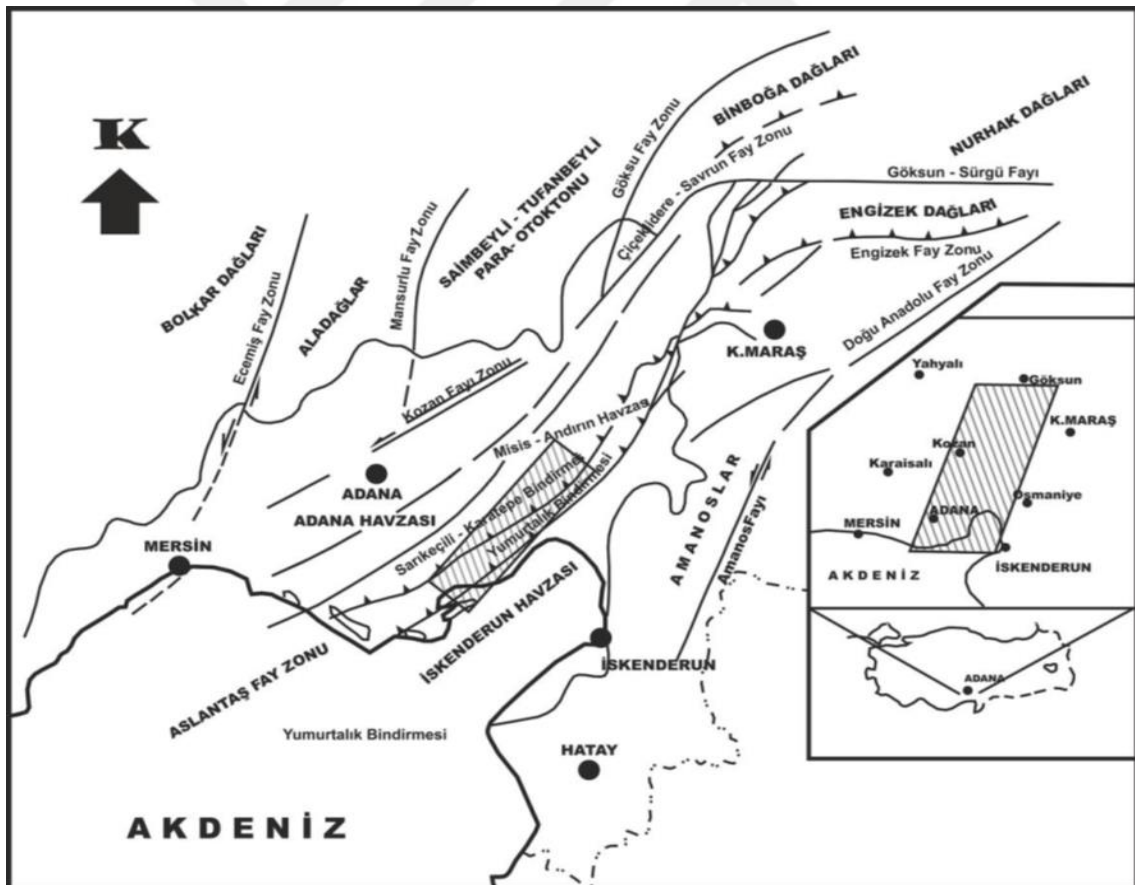
Şekil 53. Misis-Andırın Havzası'nın Doğu Akdeniz bölgesi içindeki konumunu ve ana tektonik hatlar ile olan ilişkisini gösteren yapısal harita
