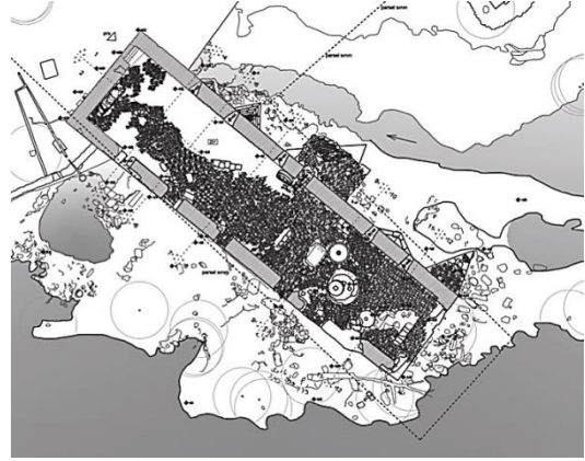
Şekil 153. Batı Değirmeni Zemin Kat Rölövesi
