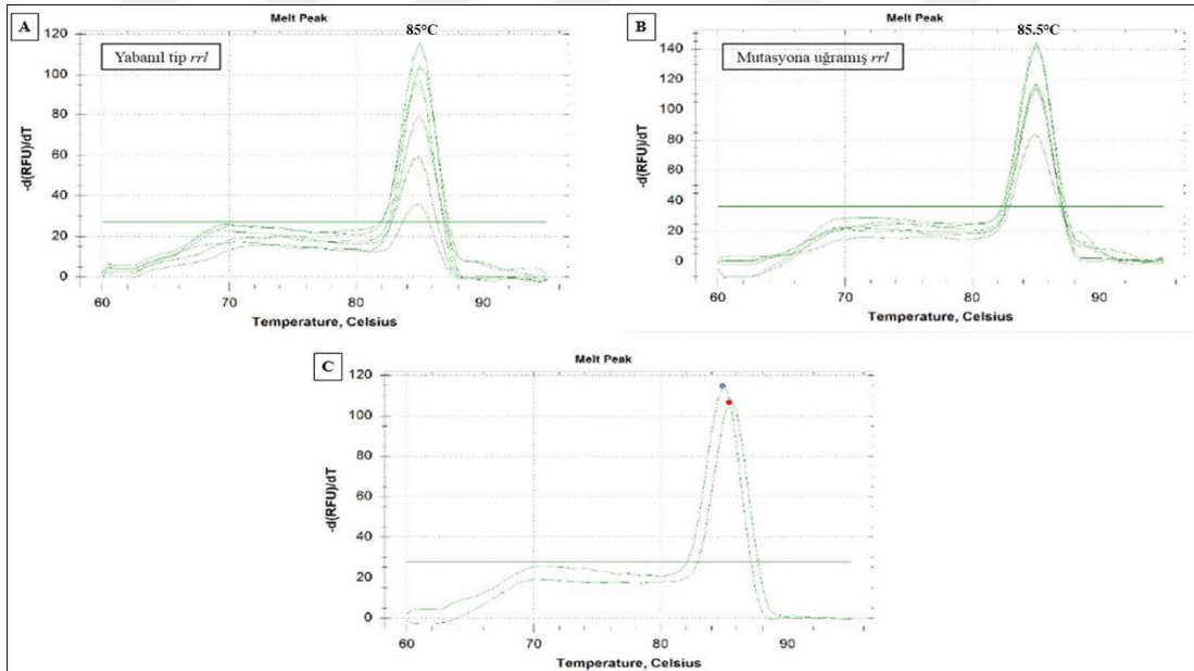
Şekil 4.1. Yabancı tip rrl ve mutasyona uğramış rrl genine ait erime eğrileri: A) Yabancı tip rrl ait erime eğrileri (85°C) B) Mutasyona uğramış rrl genine ait erime eğrileri (85,5°C) C) Yabancı tip rrl ile mutasyona uğramış rrl geninin birlikte (mavi tepe noktalı olan yabancı tip rrl ; kırmızı tepe noktalı olan mutasyona uğramış rrl ) erime eğrileri.
