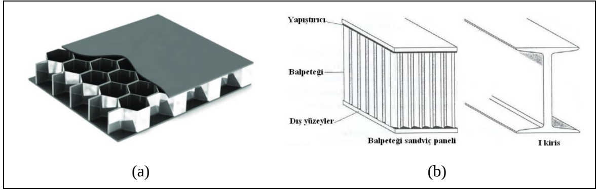
Resim 2.8. (a) Bal peteği sandviç panel (Kamaliev ve Charkviani, 2017) (b) Bal peteği sandviç panel ve I profil karşılaştırılması(CIBA, 1995)
