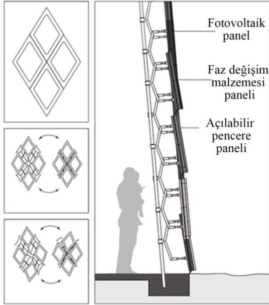
Şekil 3.4. Kertenkeleden esinlenerek tasarlanan cephe sisteminin sıcak ve soğukta değişimi (Mazzoleni, 2013:112)
