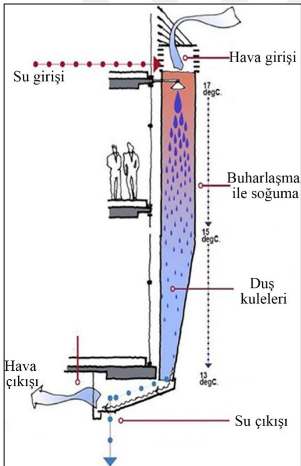
Şekil 3.6. CH2 Binası çatıdan indirilen borularla havanın nemlendirilmesiyle ile soğuma sağlanması (www.mickpearce.com)
