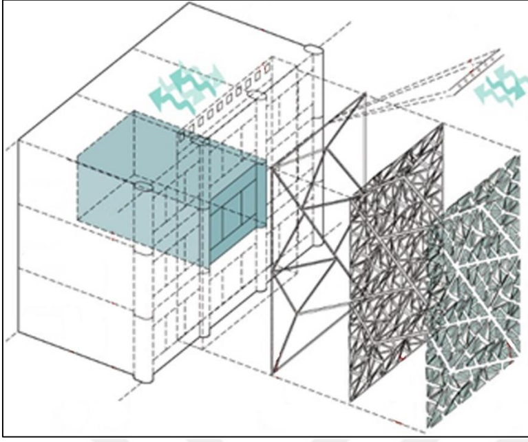
Şekil 3.9. Ofis binaları için gözenekli katlanmış bir cephe kesiti (El Ahmar ve Fioravanti, 2015)
