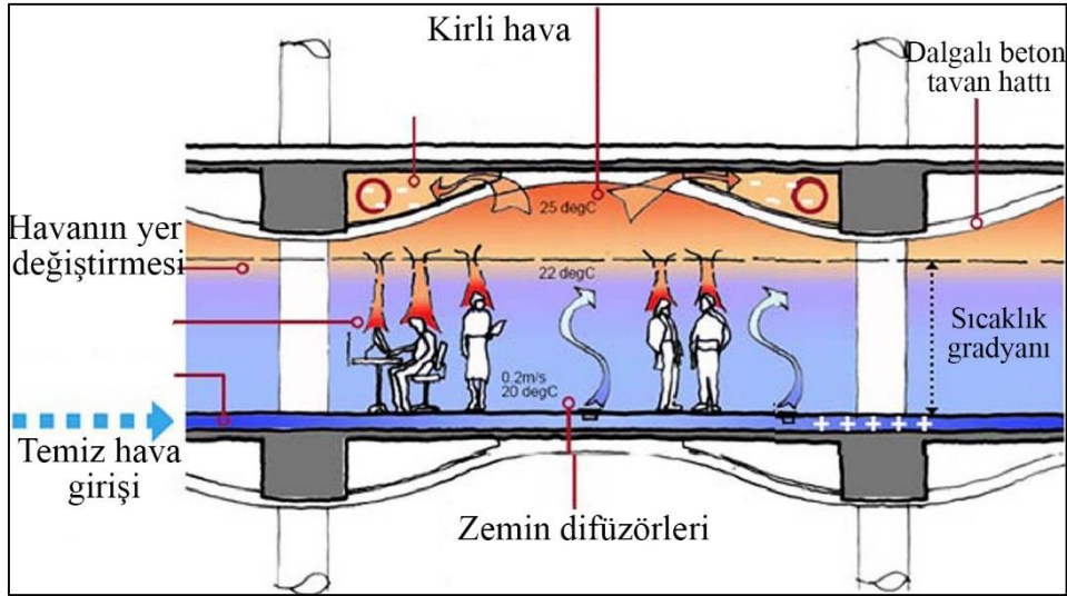
Şekil 3.5. CH2 Binası yapı içi hava sirkülasyon şeması (Tan, 2007)
