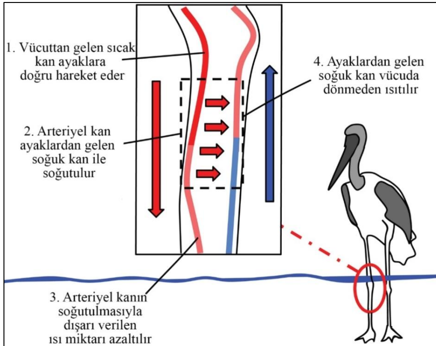
Şekil 3.12. Kuşların termoregülasyon sağlamak için kan akış kontrolü şeması (www.khanacademy.org)
