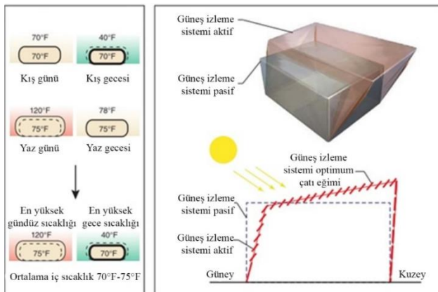
Şekil 3.3. Kertenkeleden esinlenerek tasarlanan cephe sisteminin sıcak ve soğukta değişimi (Mazzoleni, 2013:110)
