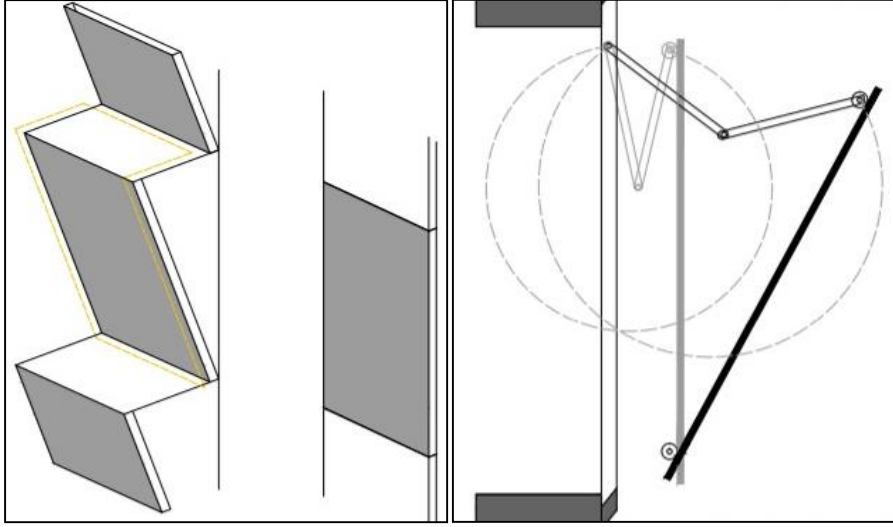
Şekil 3.11. Kuşlardan ilham alınarak tasarlanan yapı kabuğu (Kalatha, 2016)
