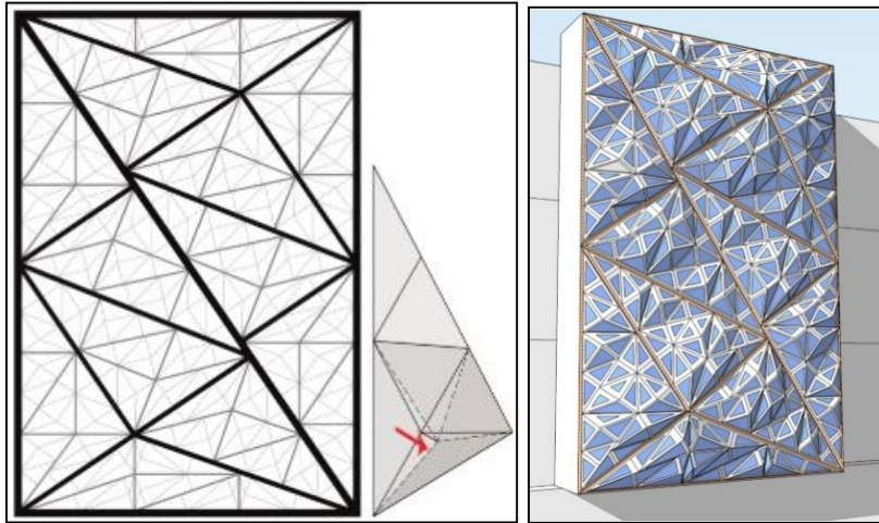
Şekil 3.8. Ofis binaları için gözenekli katlanmış bir cephe modeli (El Ahmar ve Fioravanti, 2015)
