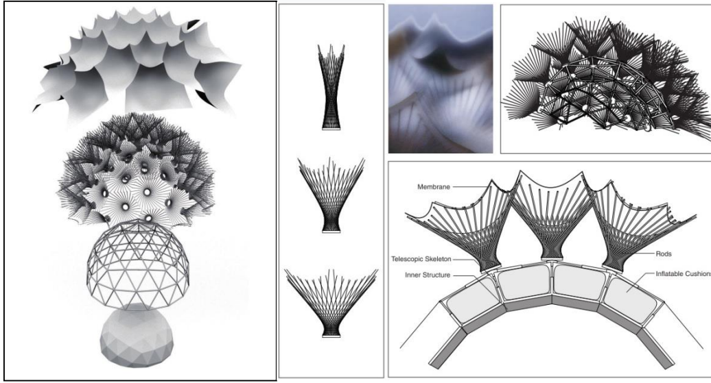
Şekil 3.10. Kar leoparının esinlenilerek tasarlanan yapı kabuğu (Mazzoleni, 2013:121)
