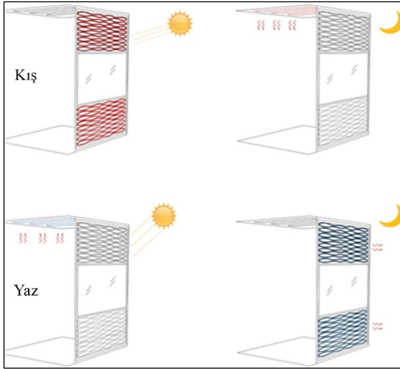
Şekil 3.13. Kuşların kan akışı ile termoregülasyon sağlamasından esinlenerek tasarlanan yapı kabuğu (Kalatha, 2016)
