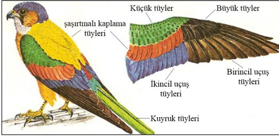
Resim 3.4. Kuşların tüy yapıları (www.daviddarling.info)
