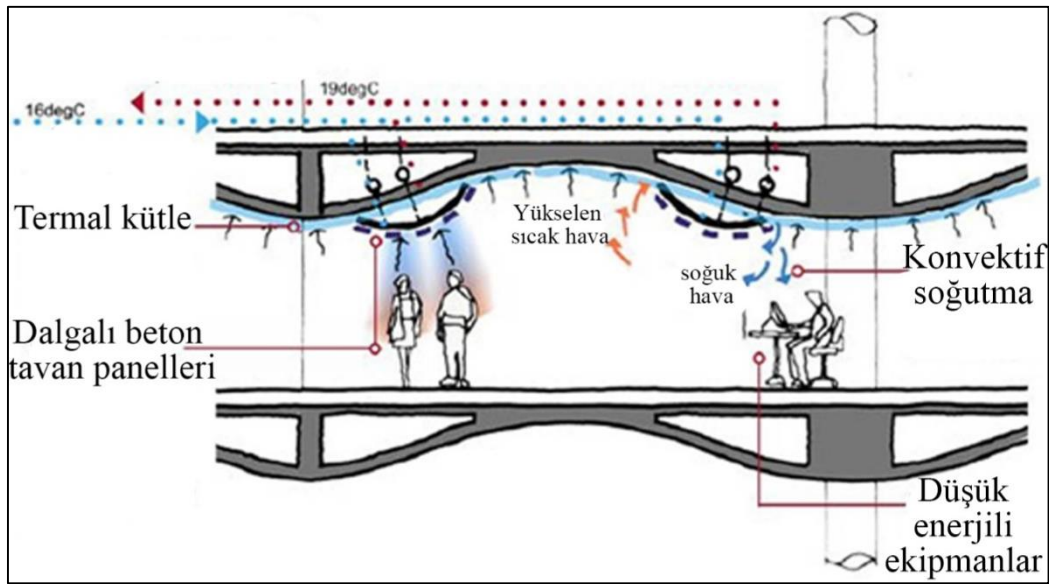
Şekil 3.7. CH2 Binası beton döşemeler ile soğuma sağlanması (Tan, 2007)
