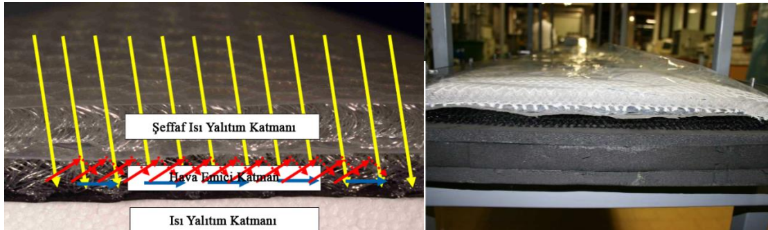
Şekil 3.15. Kutup ayısının kürkünden esinlenerek tasarlanan membran (docplayer.net)
