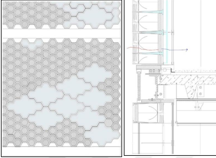
Şekil 3.22. Farchi Nachman (2009) tarafından stomalardan esinlenerek tasarlanan cephe ve yapı kabuğu kesiti
