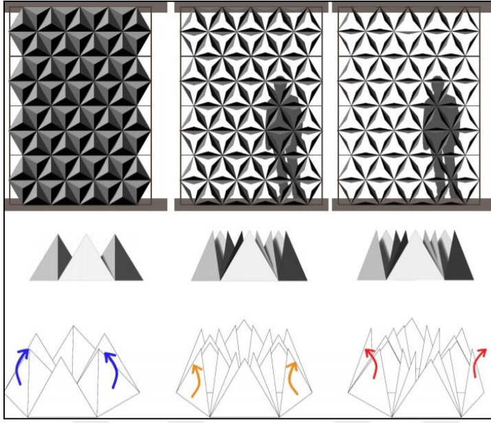
Şekil 3.21. Stomalardan esinlenerek tasarlanan yapı kabuğunun ısındıkça açılmasını gösteren modelleme (Kalatha, 2016)
