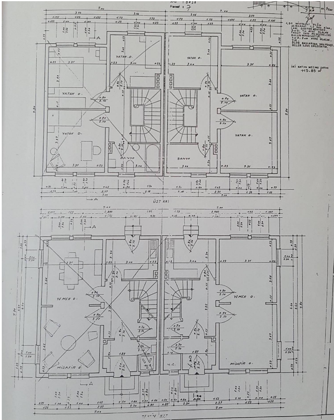
Şekil 4.19. İki kat beş odalı konut tipi plan çizimi (Önen, 1995)
