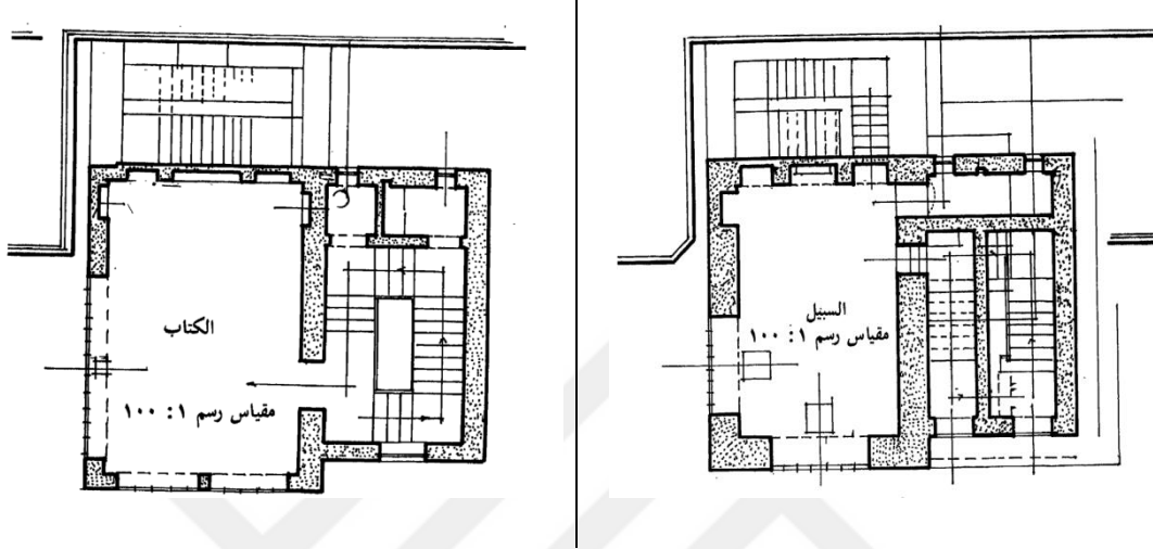
Şekil 4.19. Hüsrev Paşa Sebili ve Mektebin Yatay Krokisi, Mahmud Hamed el-Hüseyni, Kahire Arkeolojik Dairesi, 1903.
