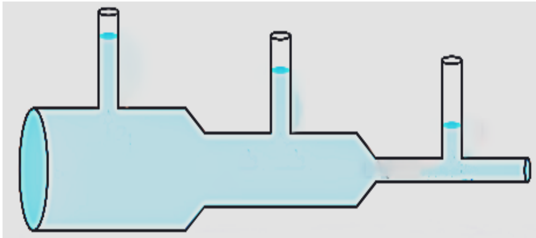
Şekil 3.3 Bernoulli İlkesi
