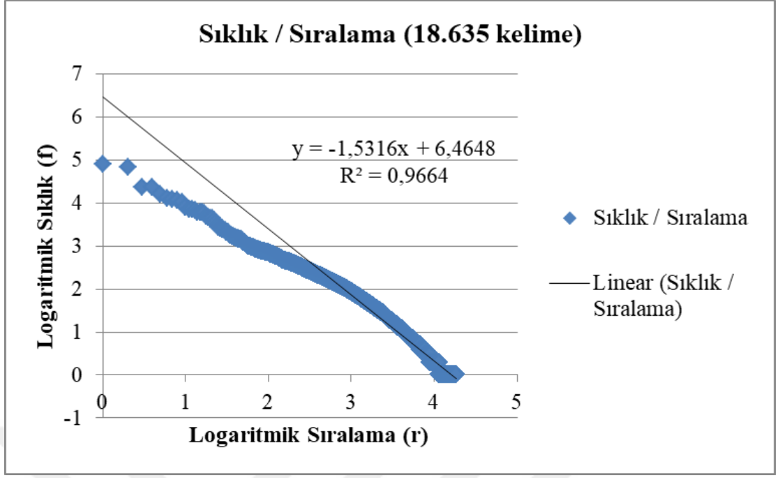
Şekil 4.1. Tüm derlem için logaritmik zipf analizi
