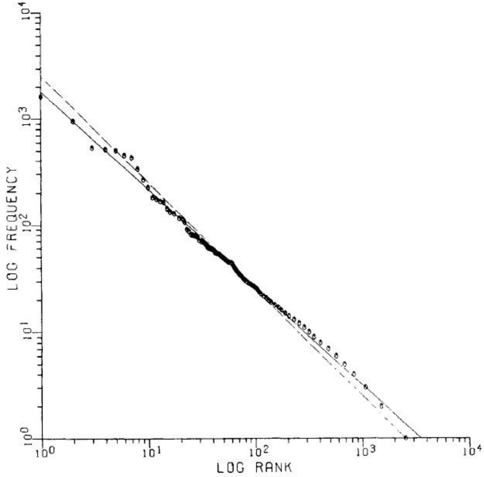
Şekil 2.1. Standart zipf dağılımı örneği
