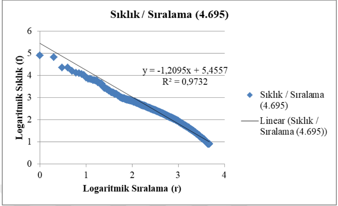
Şekil 4.2. En sık kullanılan kelimeler için logaritmik zipf analizi
