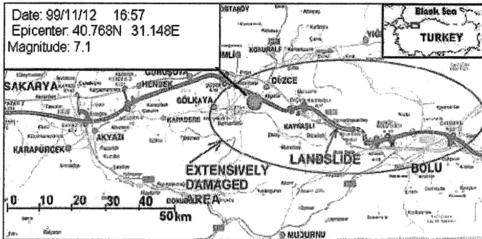
Figure 4.9 Epicenter of Düzce Earthquake (Kandilli, 2000)
