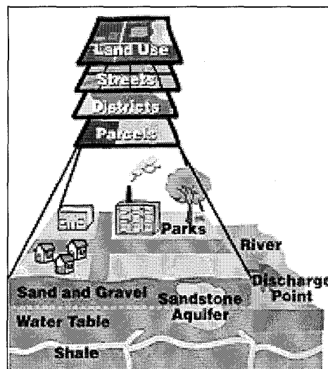
Fig. 3.22. GIS Layers
