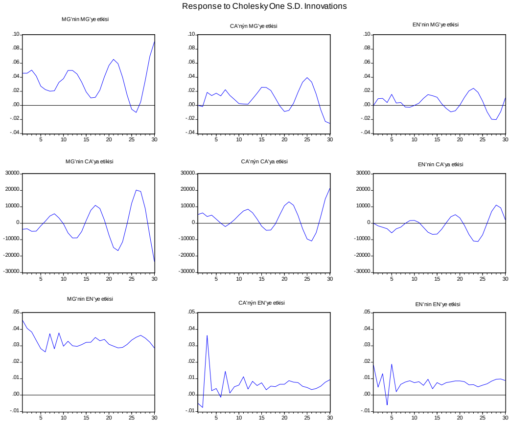
Şekil 5.4. Etki-Tepki Analizi
