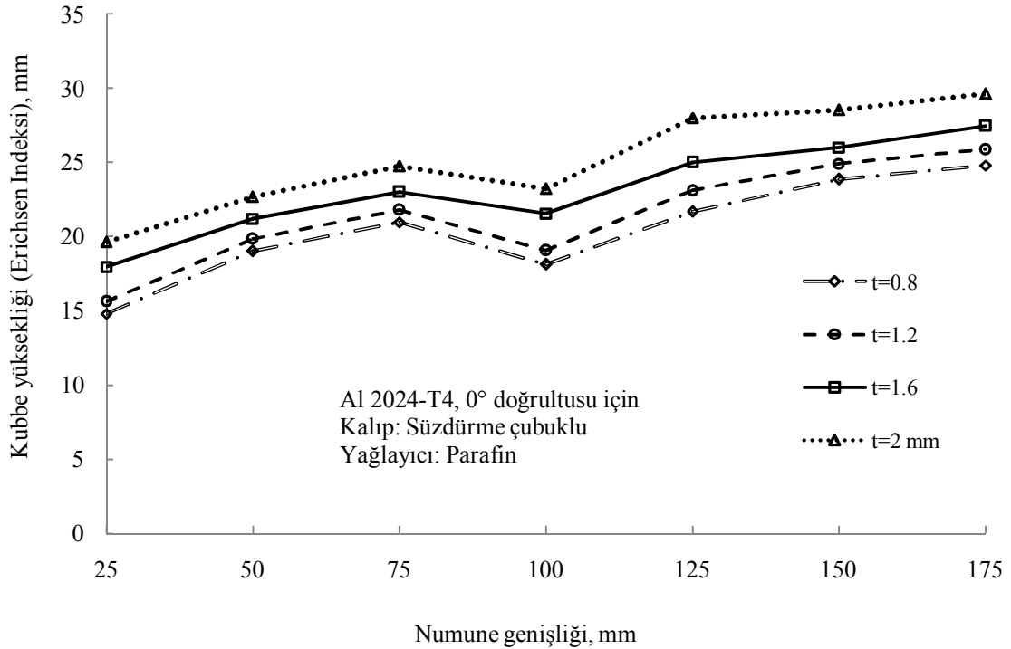
Şekil 4.37. Sınır kubbe yüksekliklerinin sac kalınlığına göre değişimi
