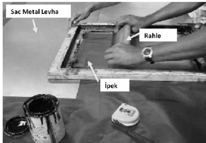
Şekil 3.10. Serigrafi yöntemi ile numunelere gridlerin oluşturulması (Hariharan ve Balaji, 2009)
