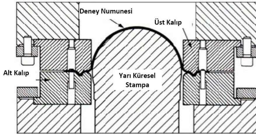
Şekil 3.13. Nakajima deneyi kalıp seti (Öztürk ve Lee, 2005)
