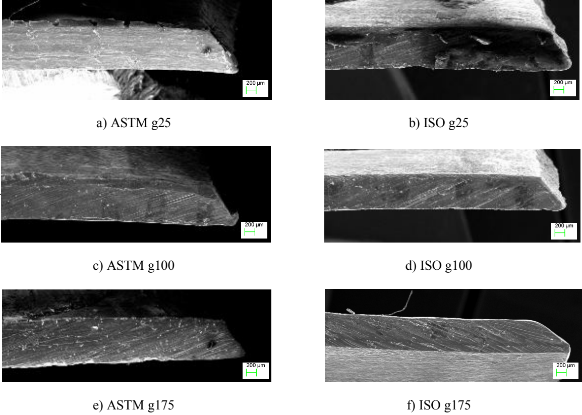
Şekil 4.14. ASTM ve ISO standartlarına göre şekillendirilen Al 2024-T4 malzemelerin boyunlaşma davranışları (1 mm ve 0° doğrultusu için)
