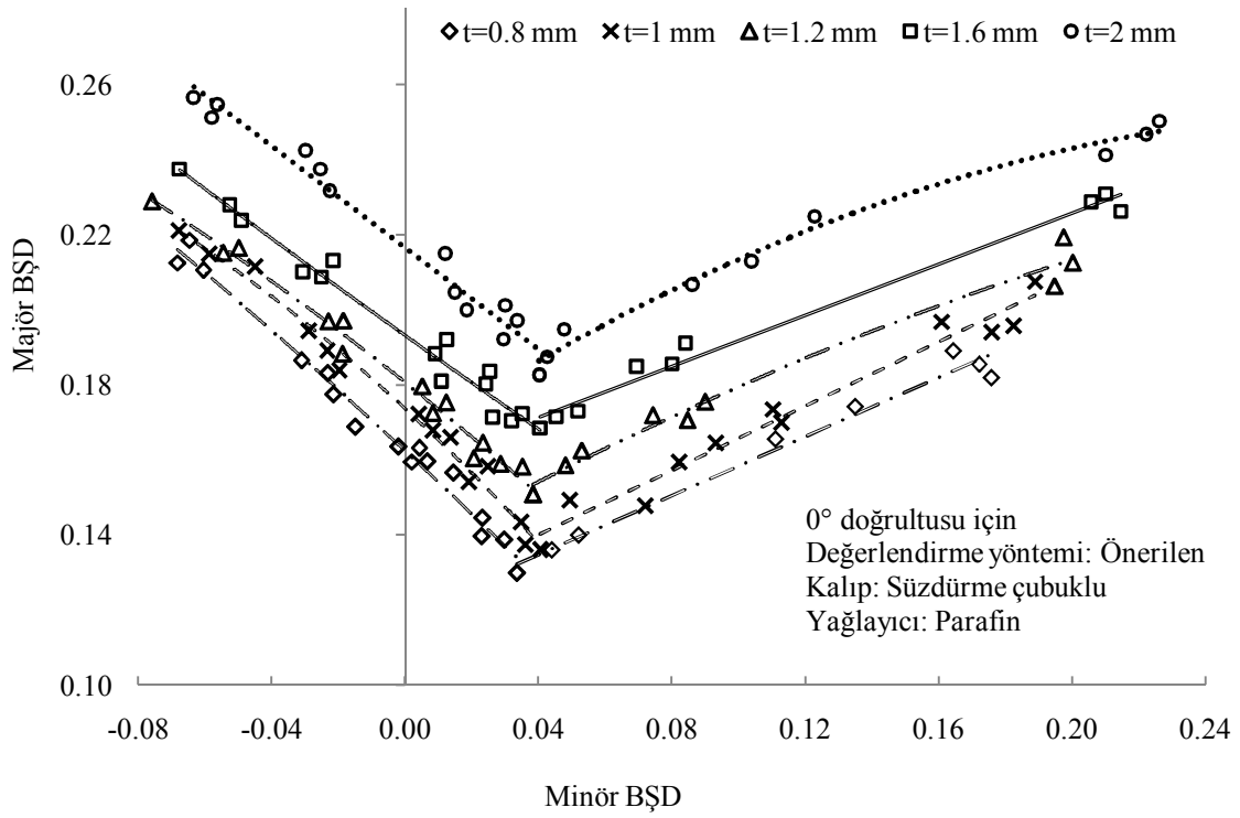
Şekil 4.34. Al 2024-T4 alaşımının ŞSE'sinin kalınlığa göre değişimi
