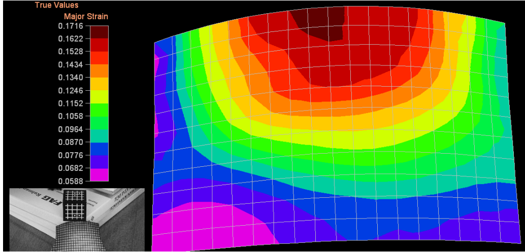
Şekil 3.19. Bilgisayarlı grid analiziyle belirlenen tipik BŞD dağılımı
