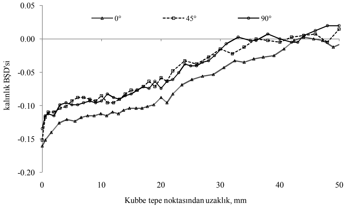
Şekil Ek4.2. 0.8 mm sac kalınlığı için kalınlık BŞD dağılımının haddeleme doğrultusuna göre değişimi
