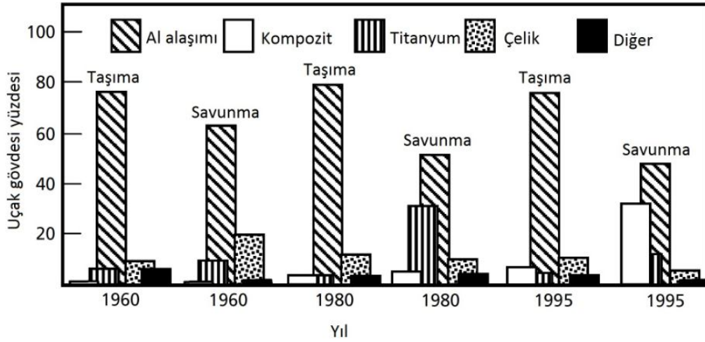
Şekil 2.3. Uçak gövdesindeki malzeme oranlarının yıllara göre değişimi (Campbell, 2006)
