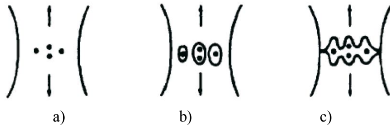
Şekil 2.10. a) Boşluk başlangıcı, b) boşluk büyümesi ve c) boşluk birleşmesi (Öztürk, 2002)
