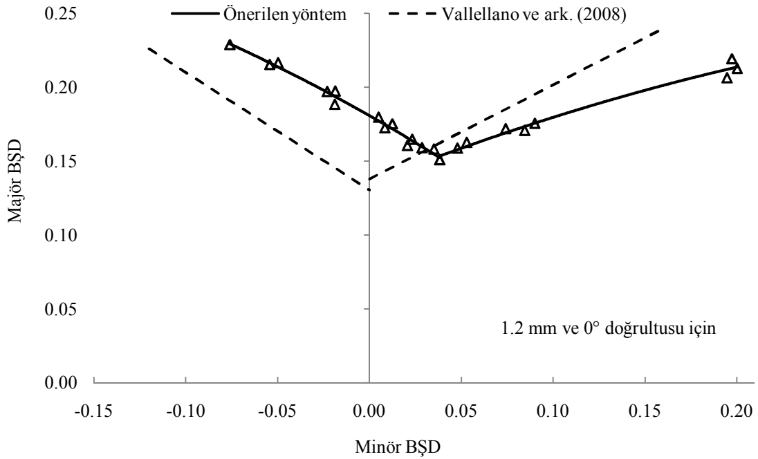
Şekil 4.35. 1.2 mm için ŞSE'nin literatür ile karşılaştırılması
