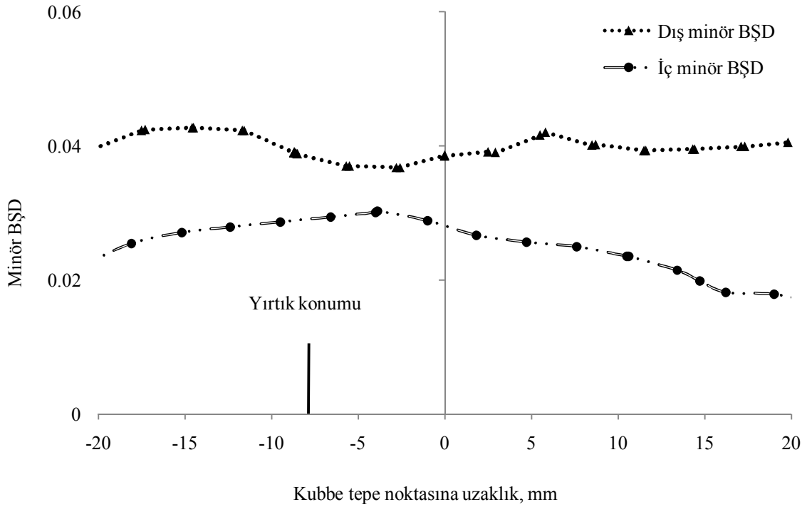
Şekil 4.32. Al 2024-T4 0.8 mm g125 numunesinin iç ve dış yüzeylerinden belirlenen gerçek BŞD dağılımı, a) majör, b) minör BŞD
