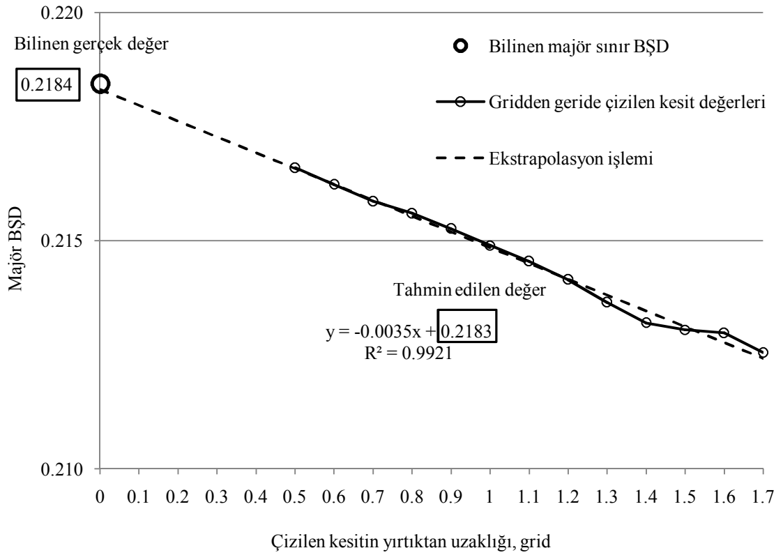
Şekil 3.27. Kesit değerlerinin ortalamaları yırtıktan uzaklığa göre yaklaşık doğrusal değişiyor
