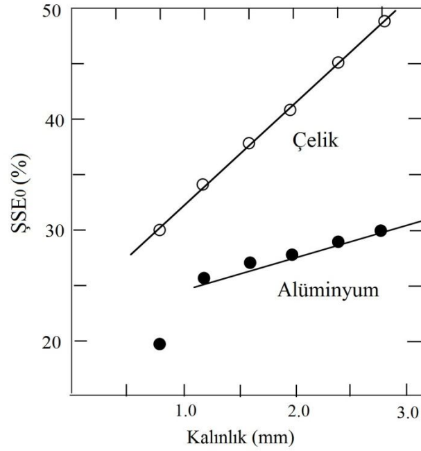
Şekil 2.16. Alüminyum ve çelikler için genel olarak sac kalınlığının \dot{\epsilon}_{SE0} 'a etkisi (Hosford ve Caddell, 2007)
