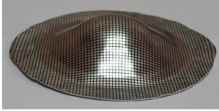
Şekil 4.45. Gerdirmeli çekme prosesiyle şekillendirilen 100 mm çapında yarıküresel parça
