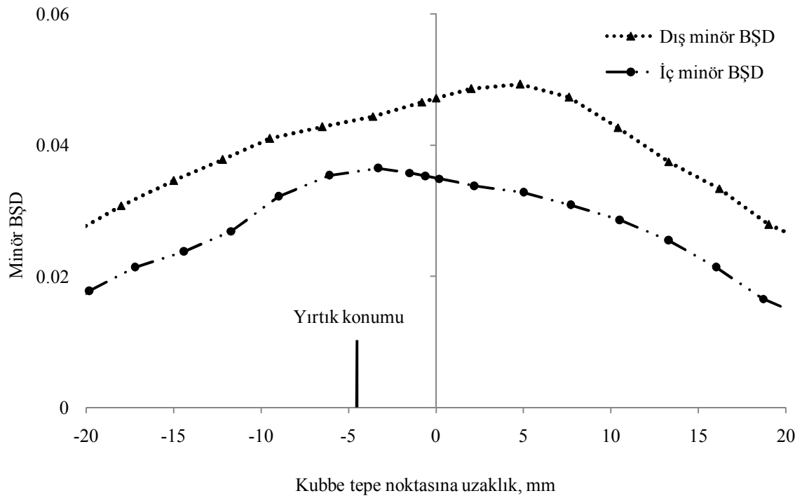
Şekil 4.33. Al 2024-T4 2 mm g125 numunesinin iç ve dış yüzeylerinden belirlenen gerçek BŞD dağılımı, a) majör, b) minör BŞD
