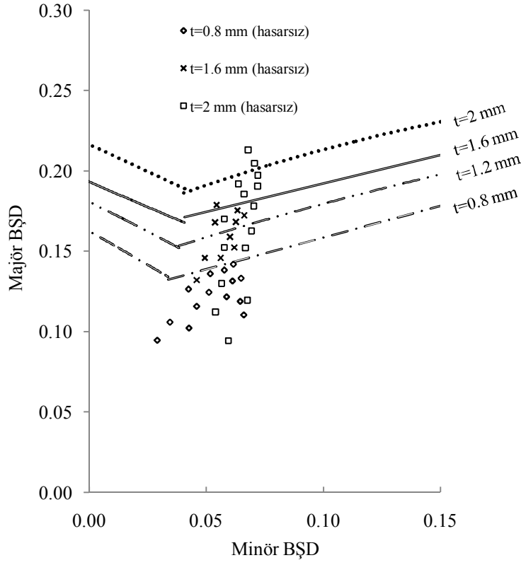
Şekil 4.55. Gerdirmeli çekme sayısal durum çalışması
