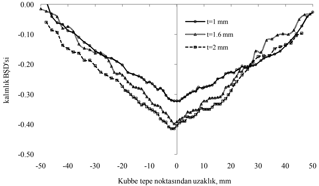
Şekil 4.42. Al 2024-T4 malzeme için gerçek kalınlık BŞD dağılımının sac kalınlığına göre değişimi, a) g25 ve b) g175 için
