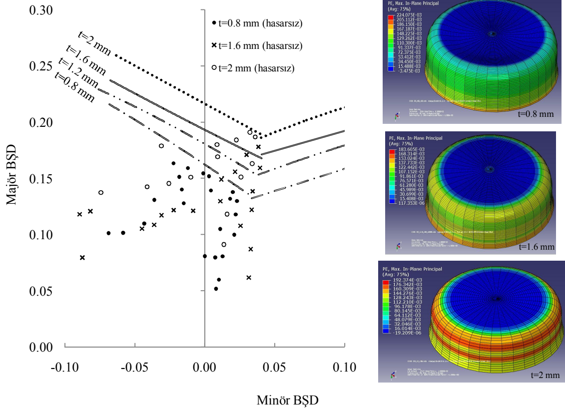
Şekil 4.54. Klasik derin çekme sayısal durum çalışması
