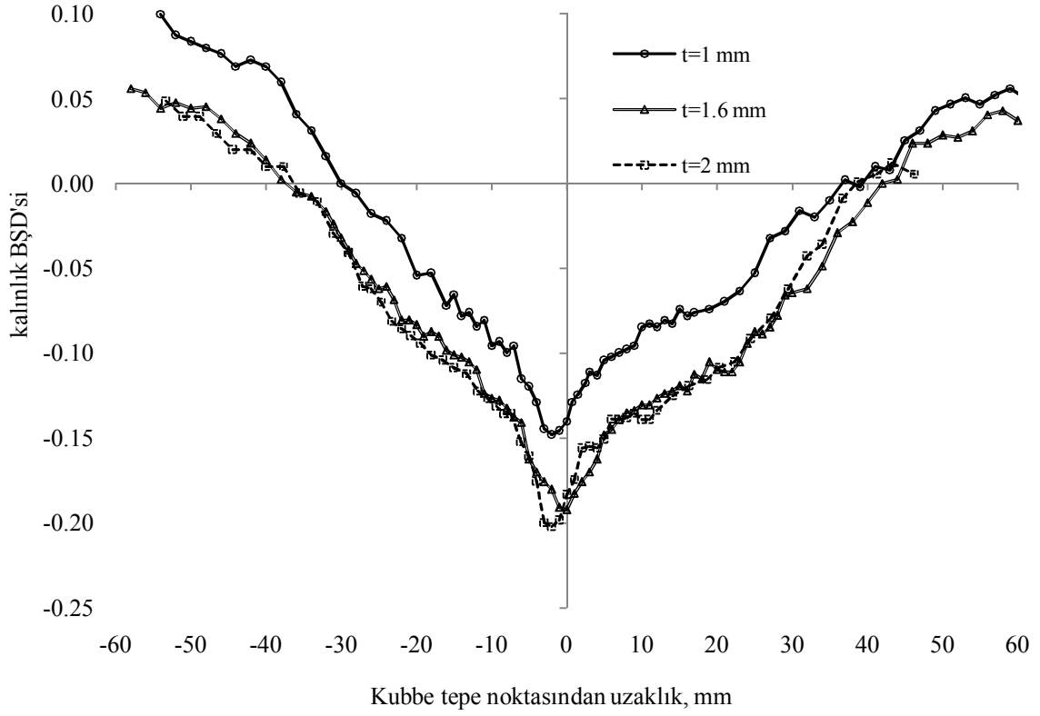
Şekil Ek4.1. g100 numunesi için kalınlık BŞD dağılımının sac kalınlığına göre değişimi
