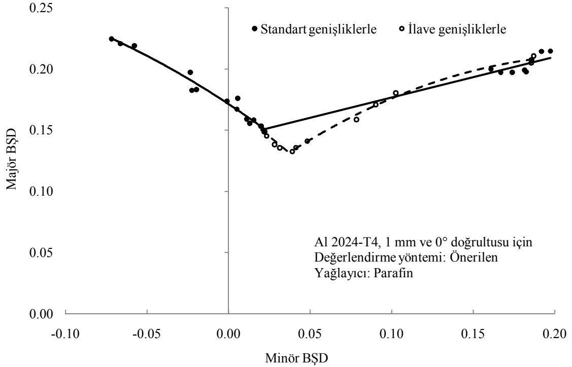
Şekil 4.25. İlave genişliklerle yapılan deneylerin etkisi
