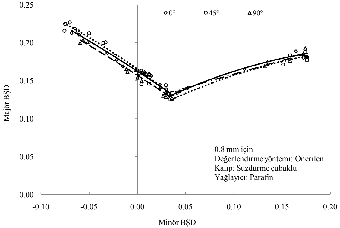
Şekil 4.38. Al 2024-T4'ün ŞSE'sinin haddeleme doğrultusuna göre değişimi
