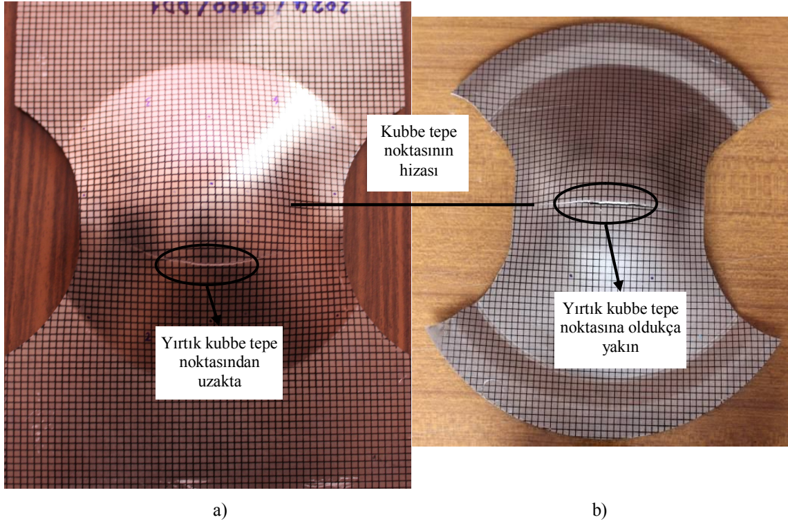
Şekil 4.8. a) ASTM E 2218-02 ve b) ISO 12004-2 standartlarına göre şekillendirilen Nakajima numunelerinde yırtığın konumu (Al 2024-T4 g100 için)
