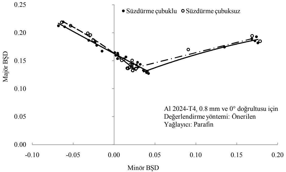
Şekil 4.29. T4 temperi için süzdürme çubuklu ve süzdürme çubuksuz elde edilen ŞSE'ler
