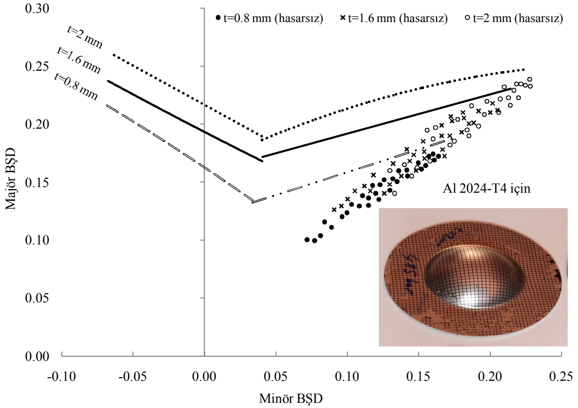
Şekil 4.52. Hidrolik şişirme deneysel durum çalışması
