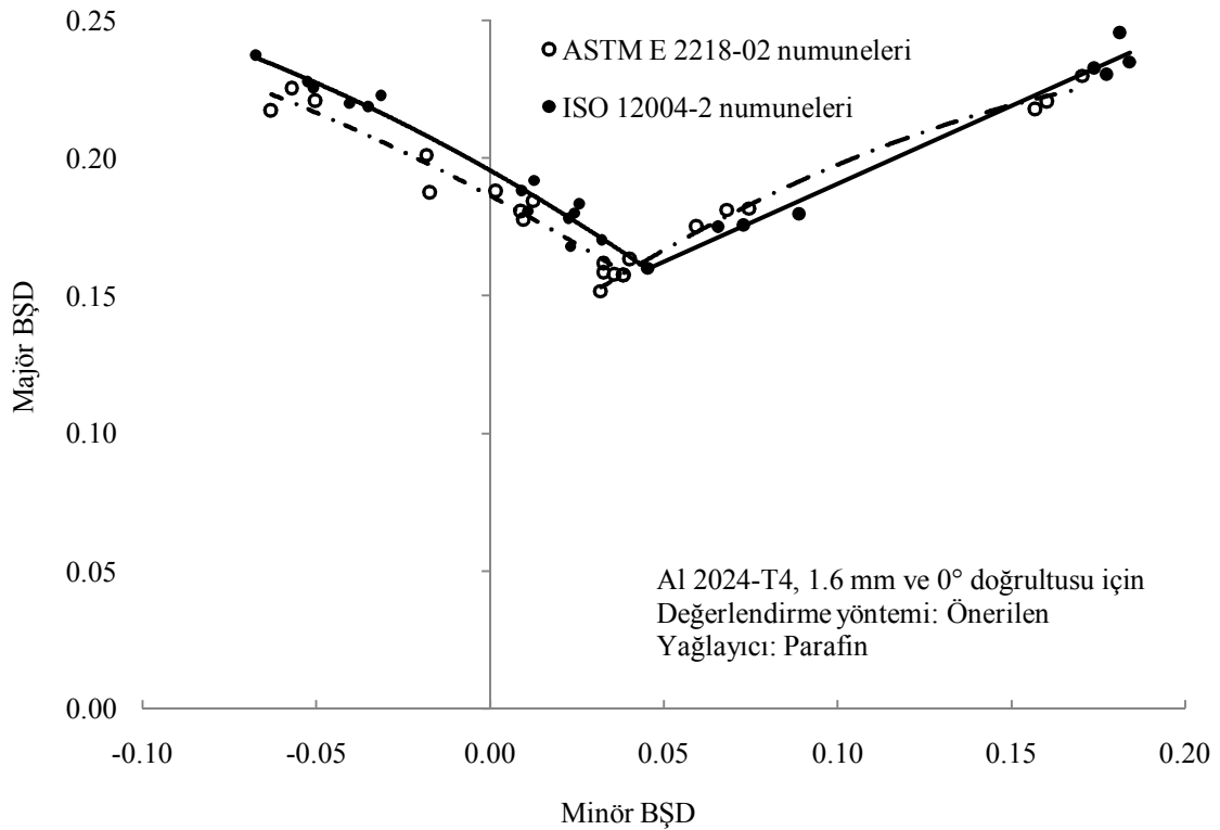
Şekil 4.11. ASTM E 2218-02 ve ISO 12004-2 standartlarındaki numune geometrilerinin etkisi
