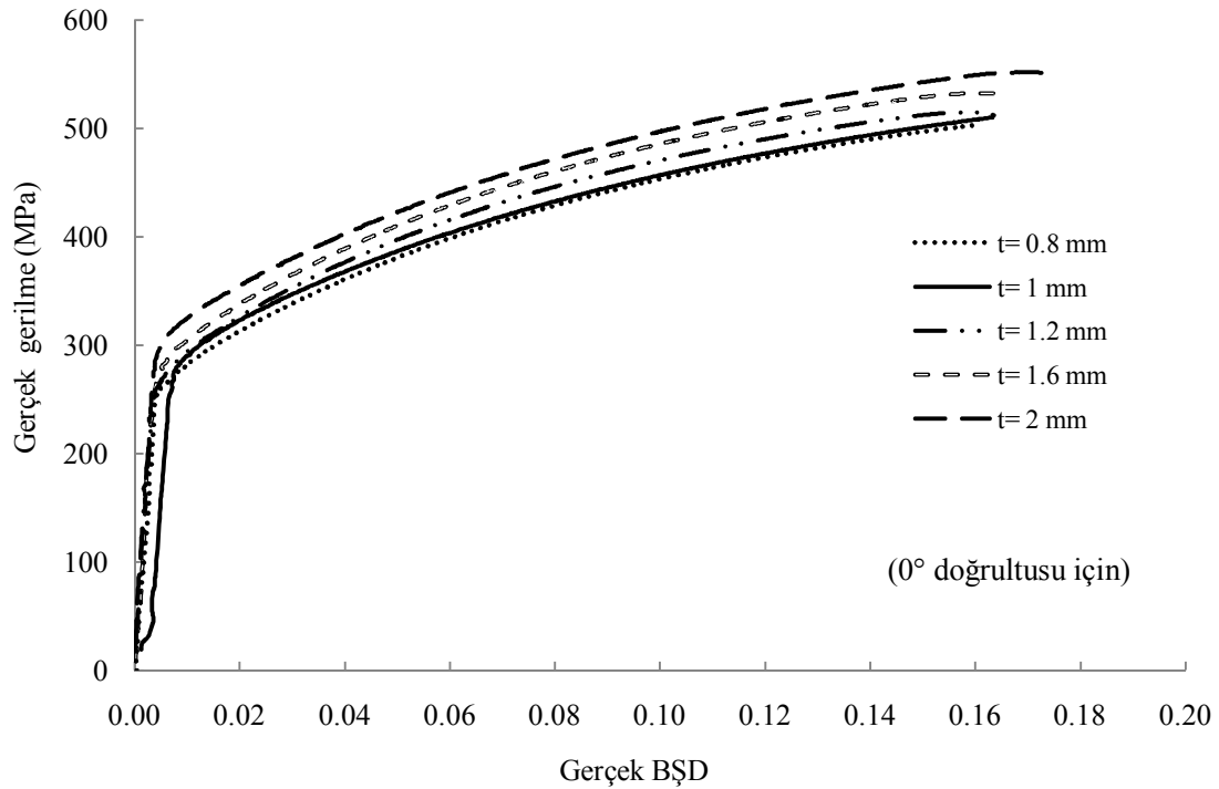
Şekil 4.3. Çeşitli kalınlıktaki Al 2024-T4 sacların gerçek gerilme-BŞD diyagramları
