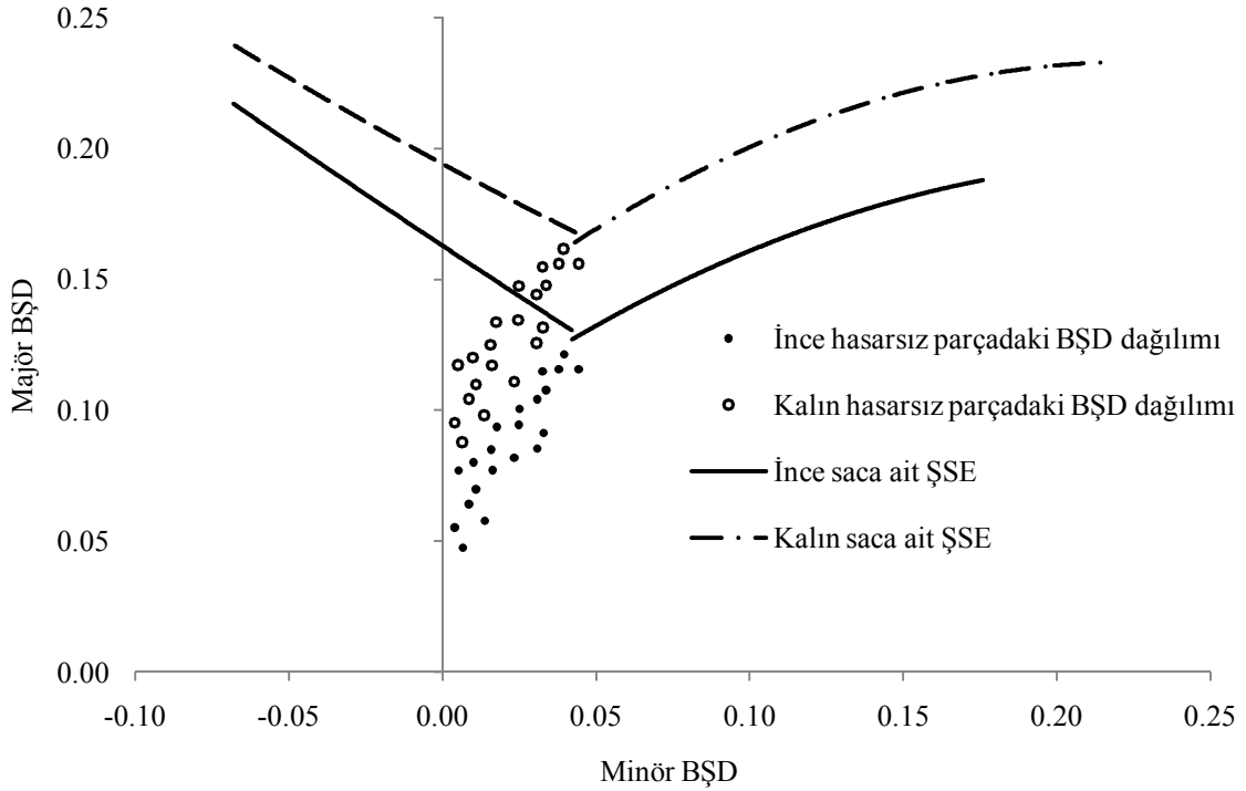
Şekil 3.34. Sac kalınlığının etkisi için yapılacak durum çalışması
