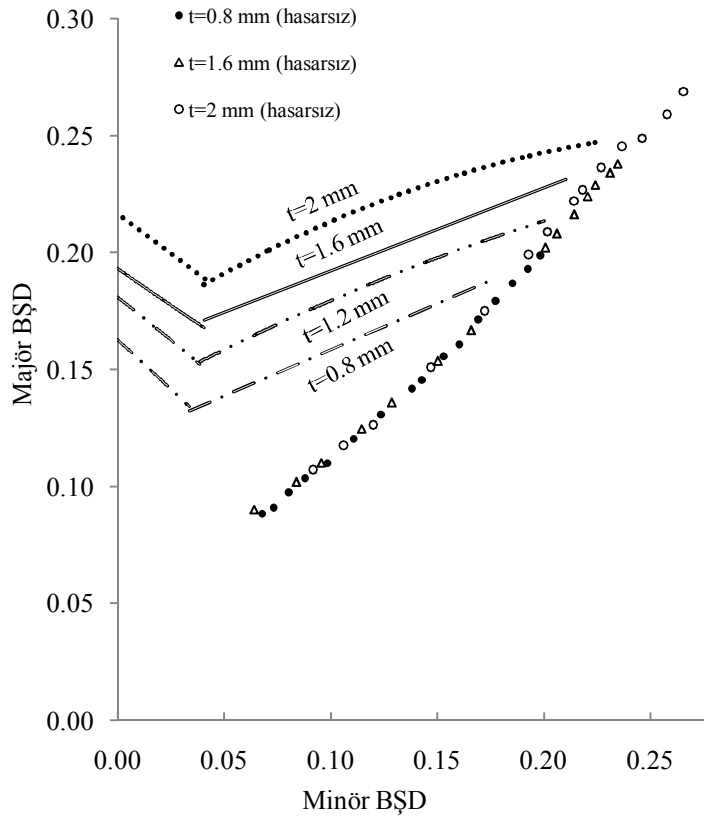
Şekil 4.56. Hidrolik şişirme sayısal durum çalışması
