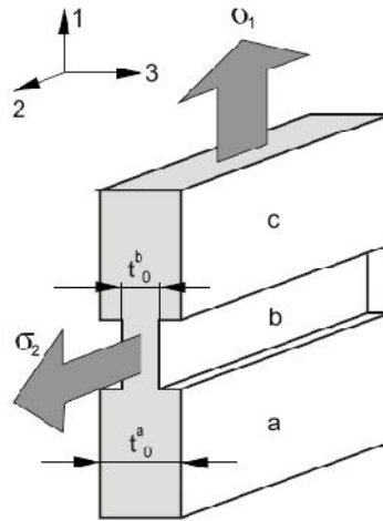
Şekil 2.9. M-K Modeli (Hosford ve Duncan, 1999)
