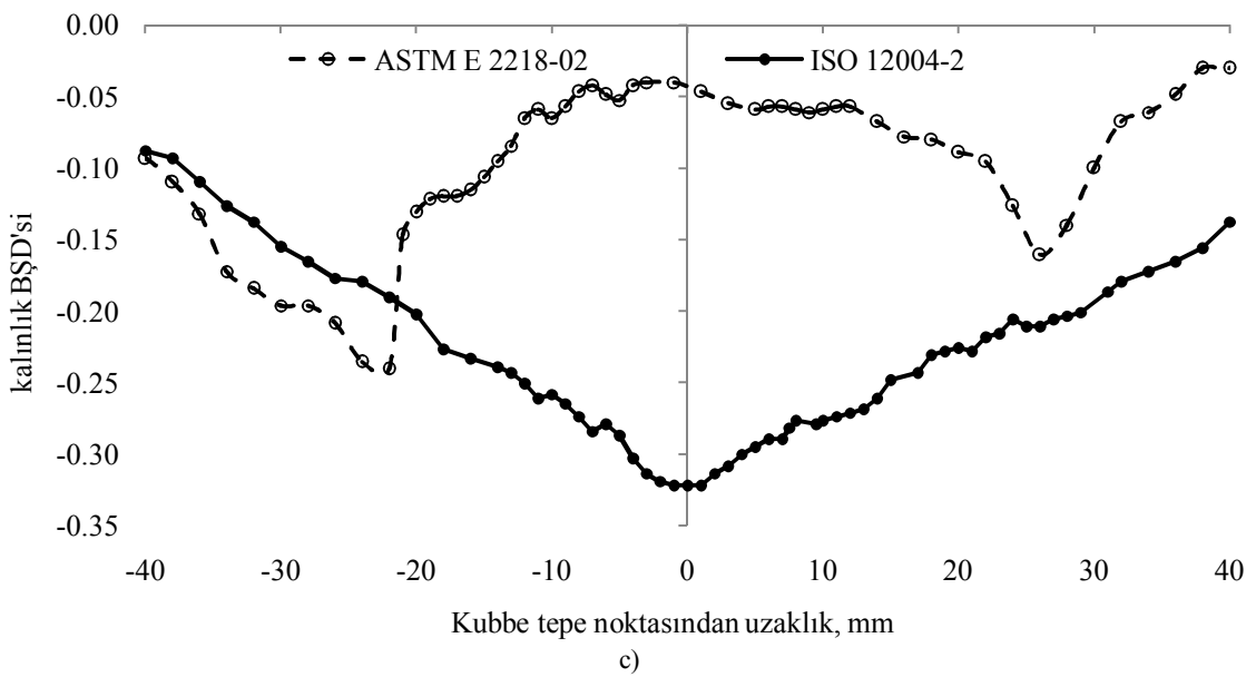
Şekil 4.13. ASTM ve ISO standartlarına göre şekillendirilen Al 2024-T4 1 mm a) g25, b) g100 ve c) g175 numuneleri için gerçek kalınlık BŞD dağılımları
