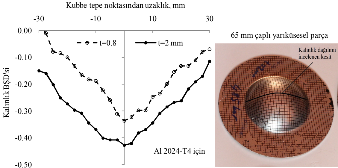
Şekil 4.53. Hidrolik şişirme durum çalışmasında elde edilen parçaların kalınlık dağılımı
