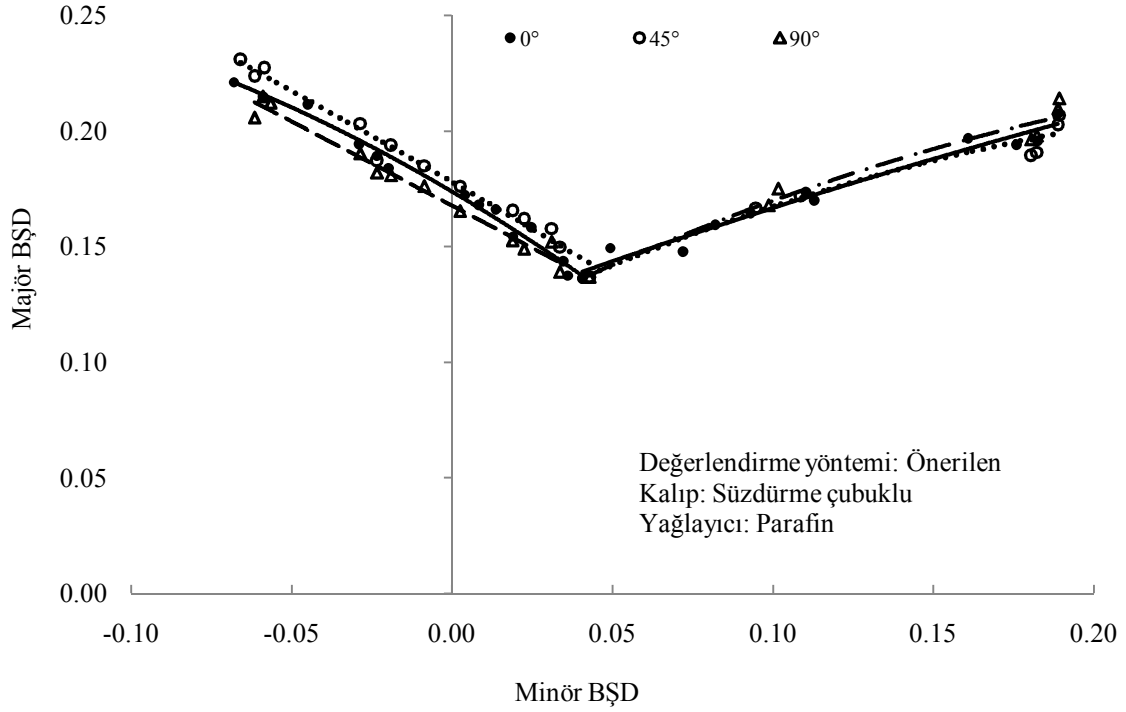
Şekil Ek3.1. 1 mm kalınlıklı Al 2024-T4'ün ŞSE'sinin haddeleme doğrultusuna göre değişimi
