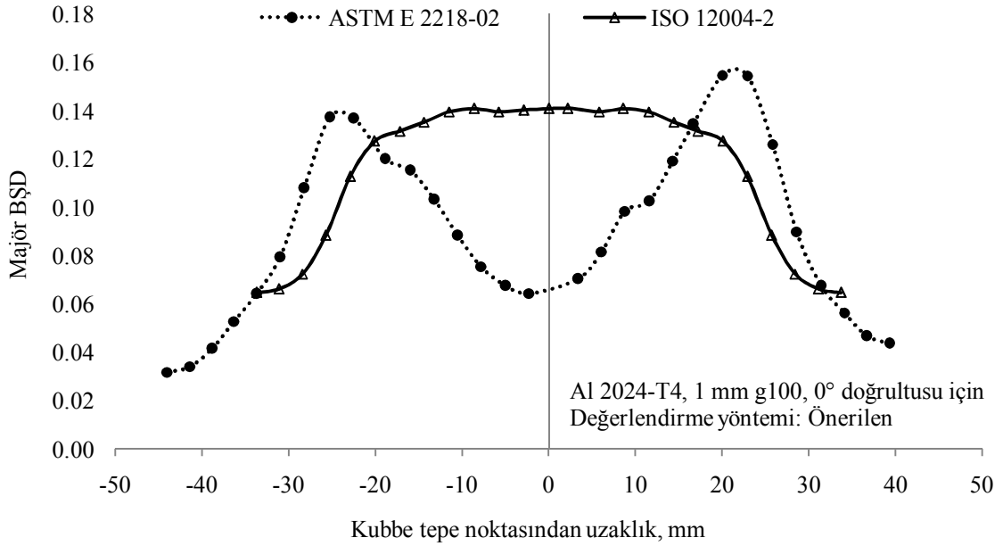
Şekil 4.7. ASTM E 2218-02 ve ISO 12004-2 standartlarından elde edilen majör BŞD dağılımları
