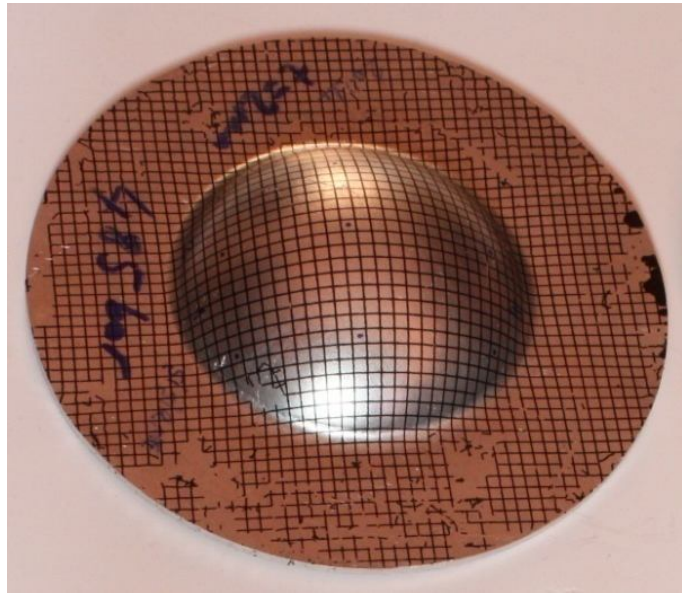
Şekil 4.46. Hidrolik şişirme prosesiyle şekillendirilen 65 mm çapında yarıküresel parça
