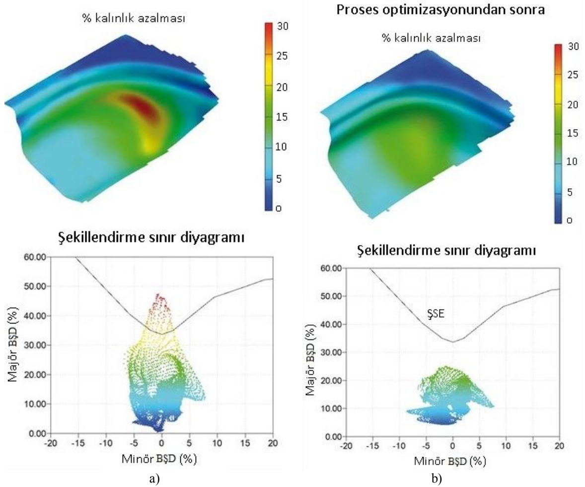
Şekil 2.7. a) Hasarlı ve b) hasarsız örnek SEY analizi ( http:// www.gom.com )
