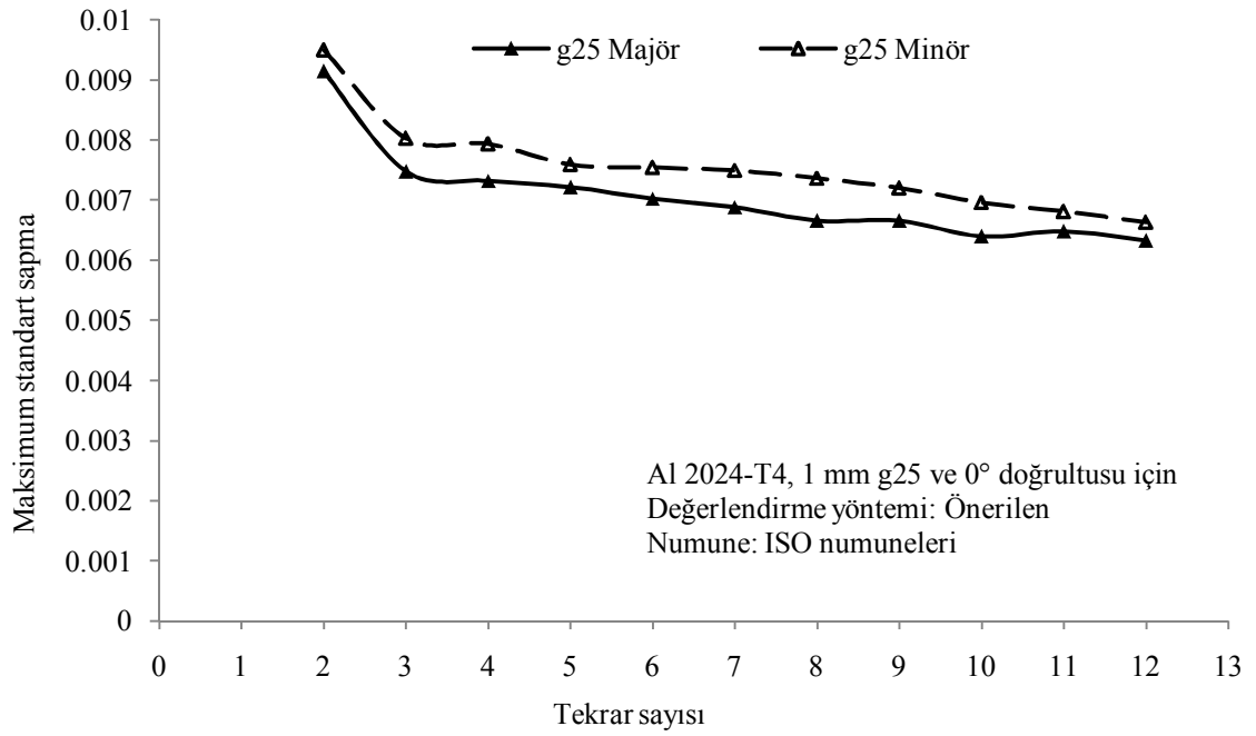
Şekil 4.16. Majör ve minör BŞD değerleri için tekrar sayısına göre elde edilen maksimum standart sapma değerleri
