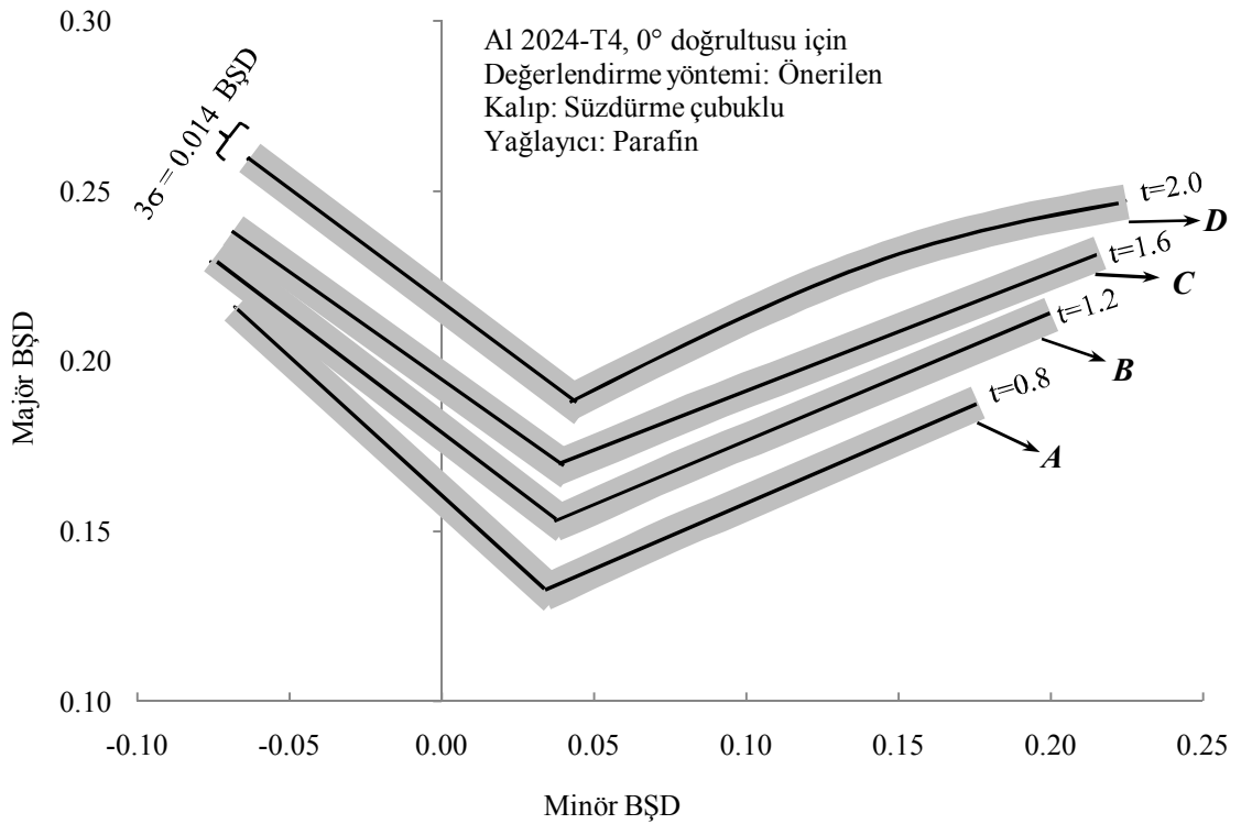
Şekil 4.36. Hata bantlarını içeren çeşitli kalınlıklı ŞSE'ler
