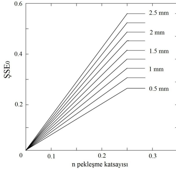
Şekil 2.15. Çelik için \text{ŞSE}_0 'ın n ve kalınlığın fonksiyonu olarak değişimi (Keeler ve Brazier, 1977)
