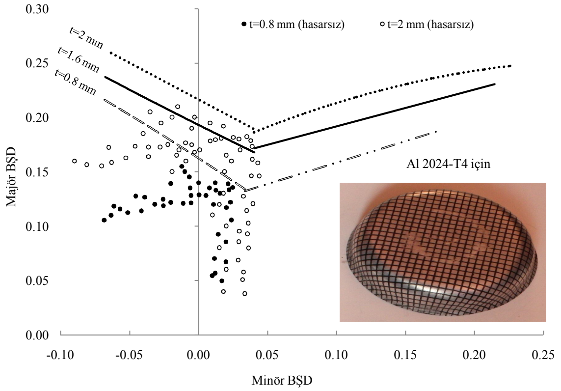
Şekil 4.50. Klasik derin çekme deneysel durum çalışması
