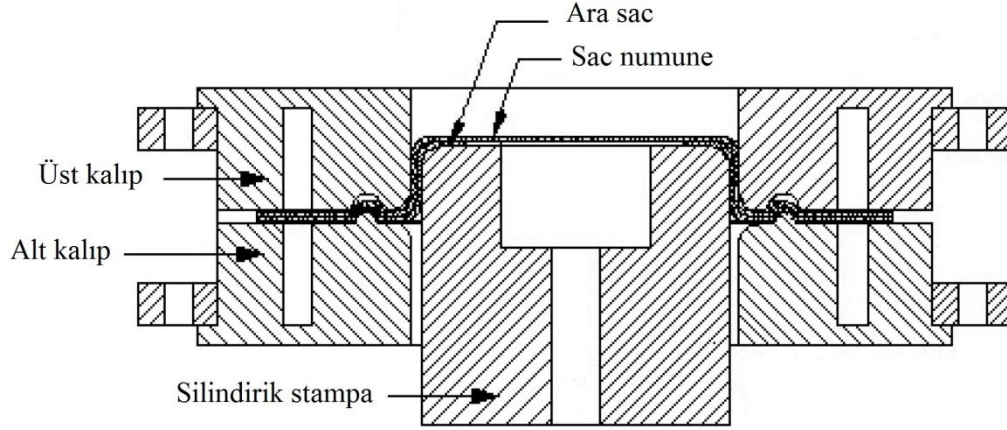
Şekil 2.14. Marciniak düzlem şekillendirme deneyi (Öztürk, 2002)
