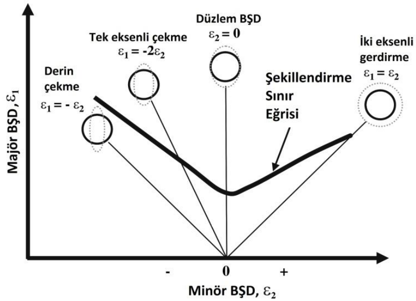
Şekil 2.6. a) Farklı BŞD durumları oluşturarak ŞSE'nin elde edilmesi, b) tipik bir ŞSE (Lamberts, 2005)
