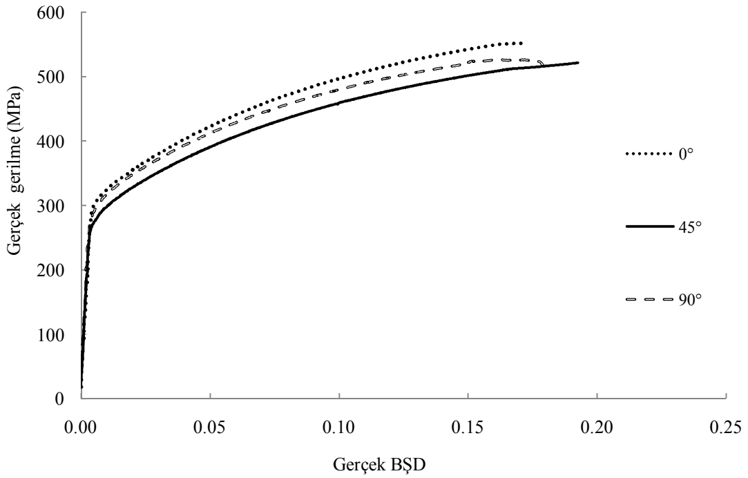
Şekil Ek2.2. devam ediyor.. a) 0.8, b) 1, c) 1.6 ve d) 2 mm sac kalınlığına sahip Al 2024-T4 sacların 0°, 45° ve 90° doğrultuları için akma eğrileri
