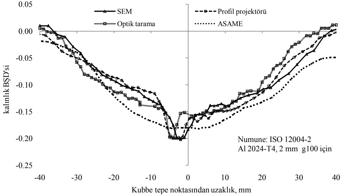
Şekil 4.39. Kalınlık dağılımı ölçme yöntemlerinin karşılaştırılması
