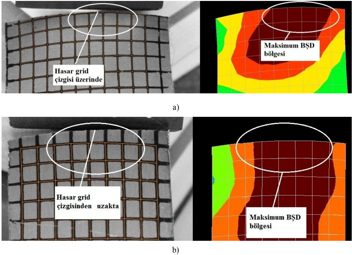
Şekil 3.24. Hasarın a) grid çizgisinin hemen üzerinde b) grid çizgisinden uzakta olması durumu
