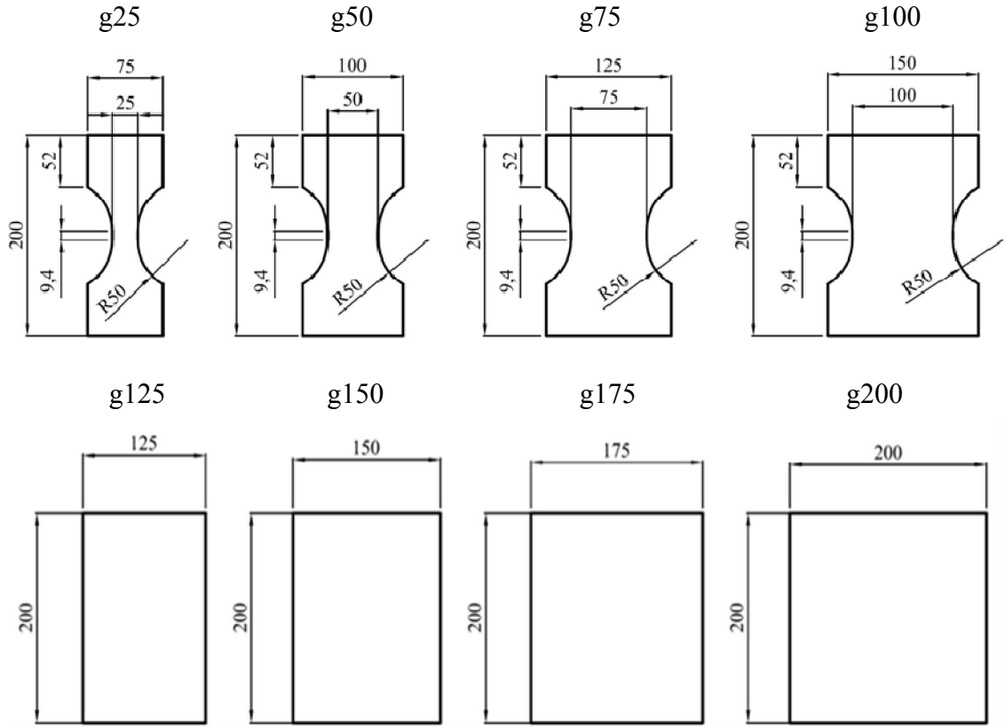
Şekil 3.7. ASTM E 2218-02 standardında kullanılan Nakajima deney numunesi takımı
