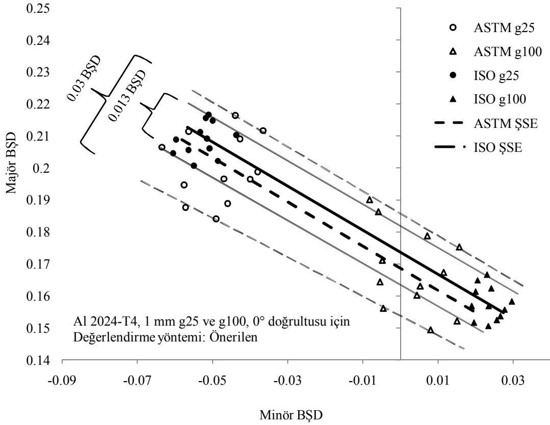
Şekil 4.9. ASTM E 2218-02 ve ISO 12004-2'ye göre tekrarlanabilirliğin karşılaştırılması
