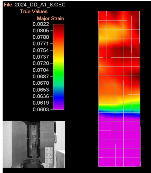
Şekil 4.4. Tipik bir anizotropi numunesindeki üniform BŞD dağılımı
