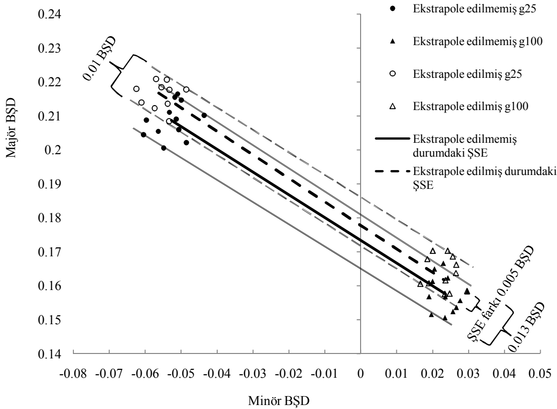
Şekil 4.17. Hasarsız gridden hasarlıya ekstrapolasyon işleminin tekrarlanabilirliğe etkisi
