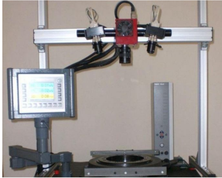
Şekil 3.20. Yüksek çözünürlüğe sahip CCD kameralara sahip ARAMIS ekipmanı
