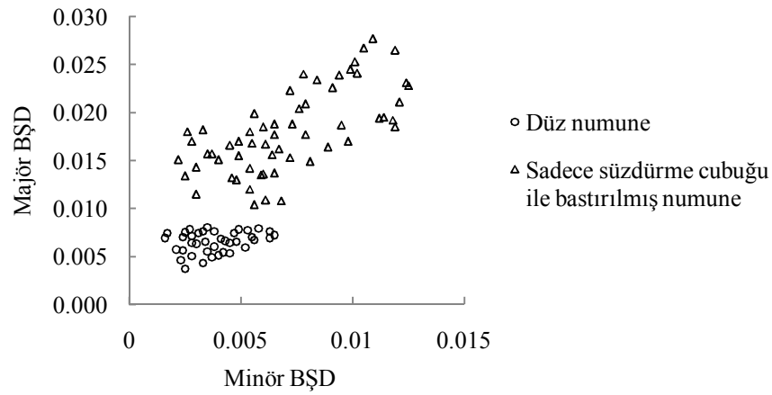
Şekil 4.28. Sadece süzdürme çubuğu ile bastırmanın etkisi
