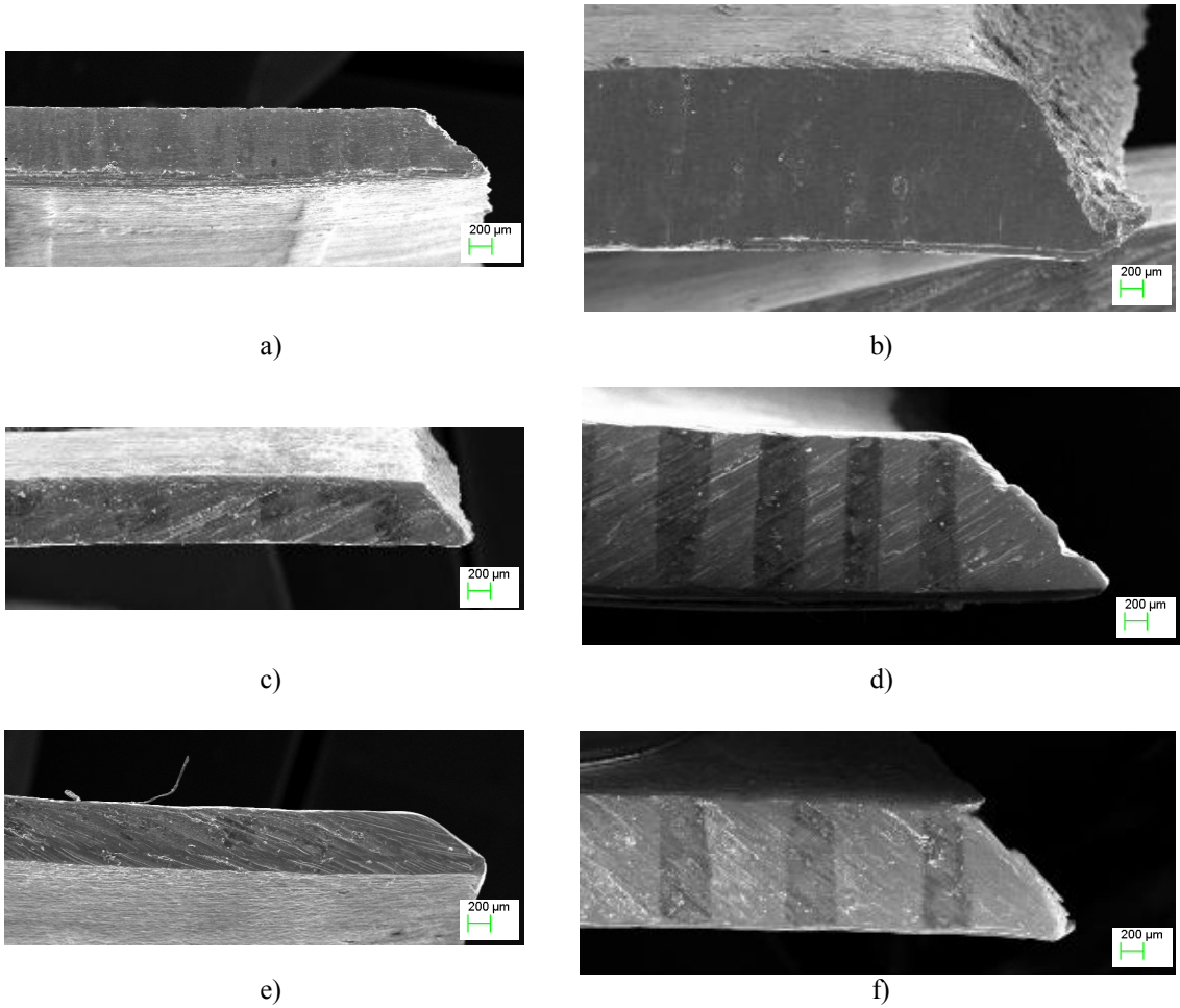
Şekil 4.43. Al 2024-T4 malzemelerin çeşitli kalınlıklar için boyunlaşma davranışları, a) t1_g25, b) t2_g25, c) t1_g100, d) t2_g100, e) t1_g175 ve f) t2_g175 için
