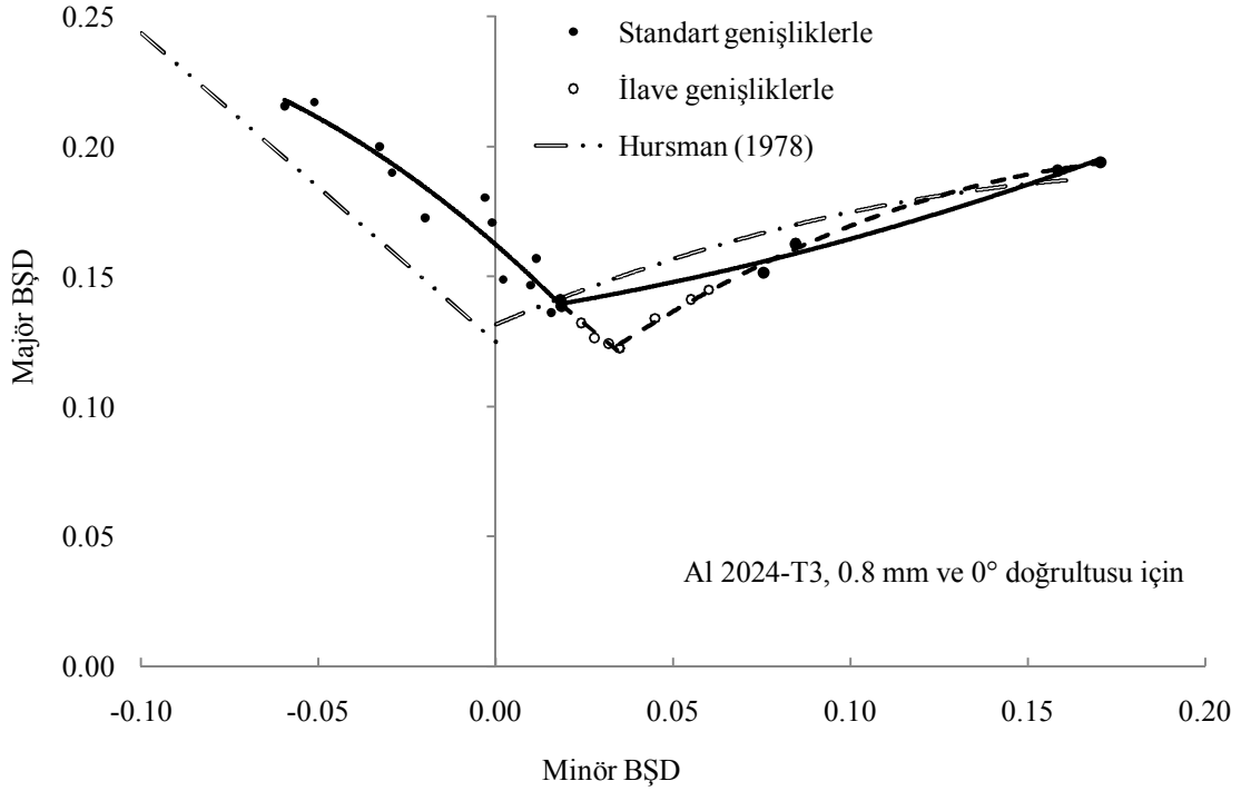
Şekil 4.26. İlave genişlikler kullanılarak elde edilen ŞSE'nin literatürle karşılaştırılması
