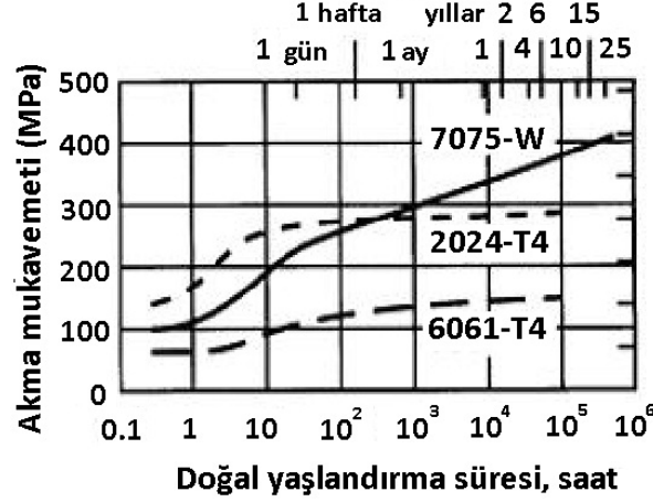
Şekil 2.1. Farklı alaşımlar için yaşlandırma süresiyle akma mukavemetinin değişimi (Elwin, 1990)
