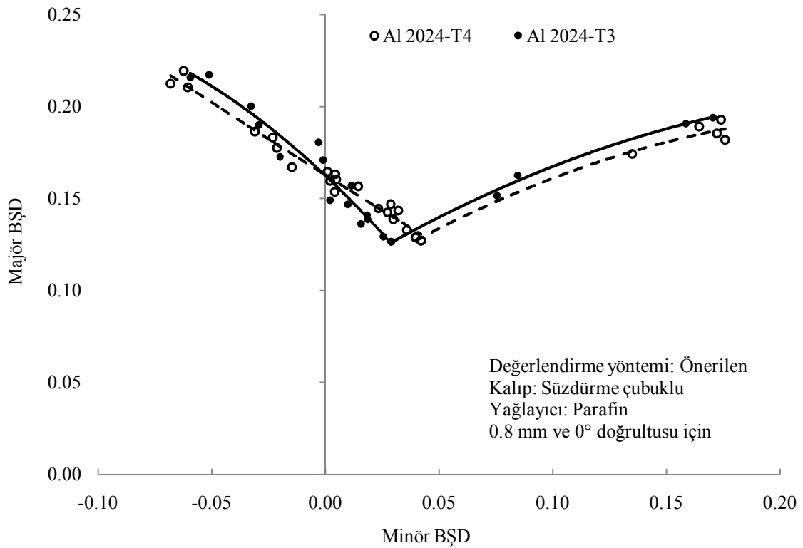
Şekil 4.27. T3 ve T4 temperlerinin karşılaştırılması
