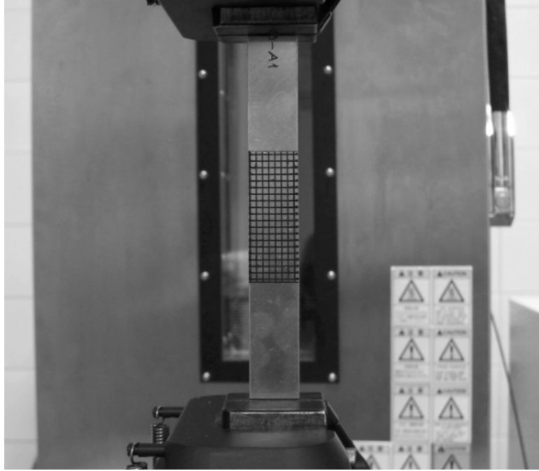
Şekil 3.5. Anizotropi değerinin belirlenmesi için çekilen örnek bir fotoğraf
