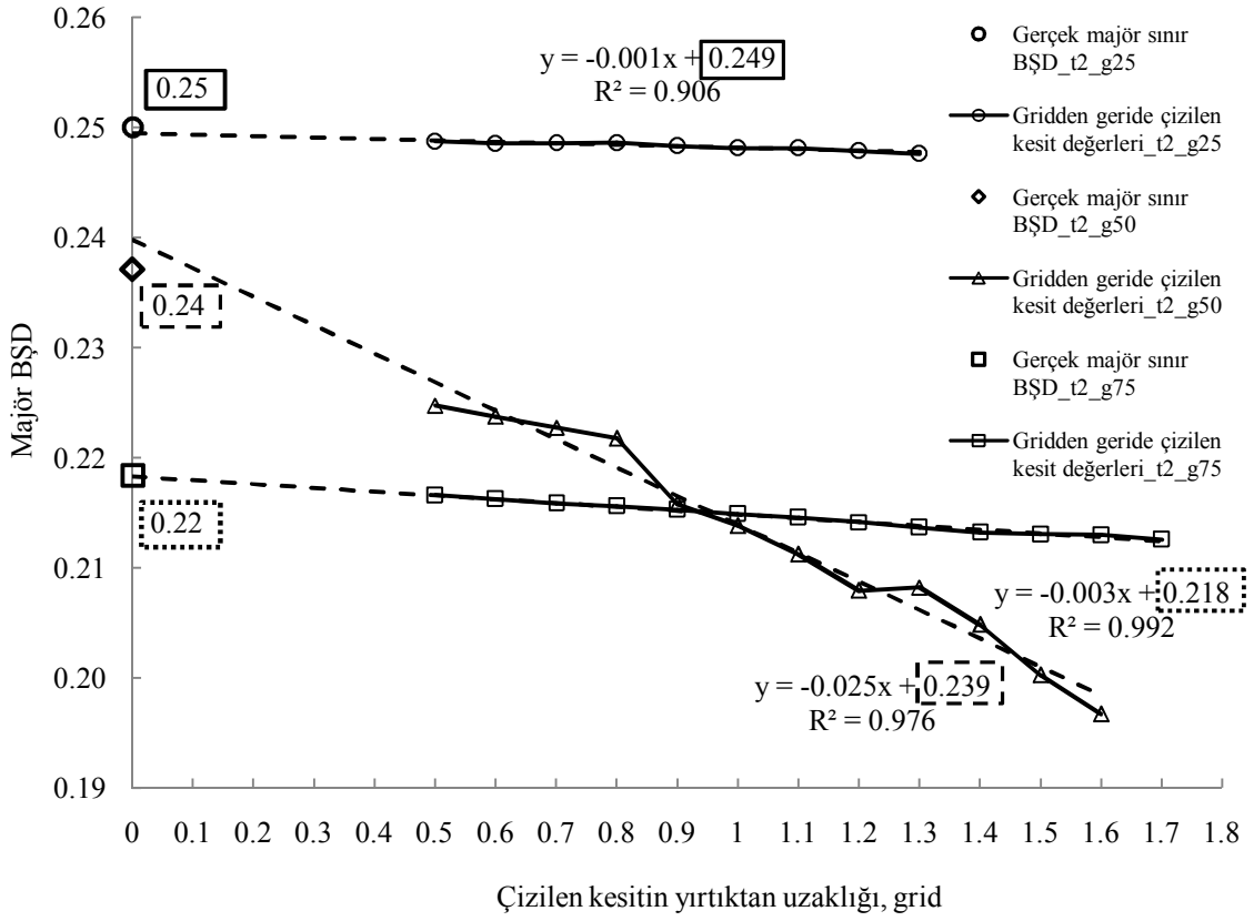
Şekil 4.18. Bazı numuneler için ekstrapolasyon işlemi (Al 2024-T4, t=2 mm için)
