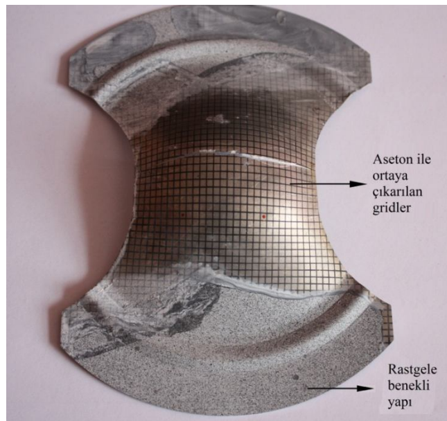
Şekil 4.19. Aseton ile rastgele benekli yapının grid yapısı bozunmadan çıkarıldığı tipik bir numune
