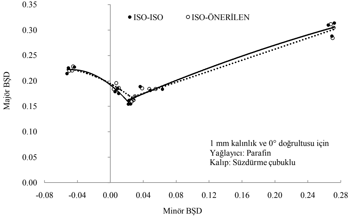
Şekil 4.22. Önerilen yöntemin Al 5754-O için geçerliliği
