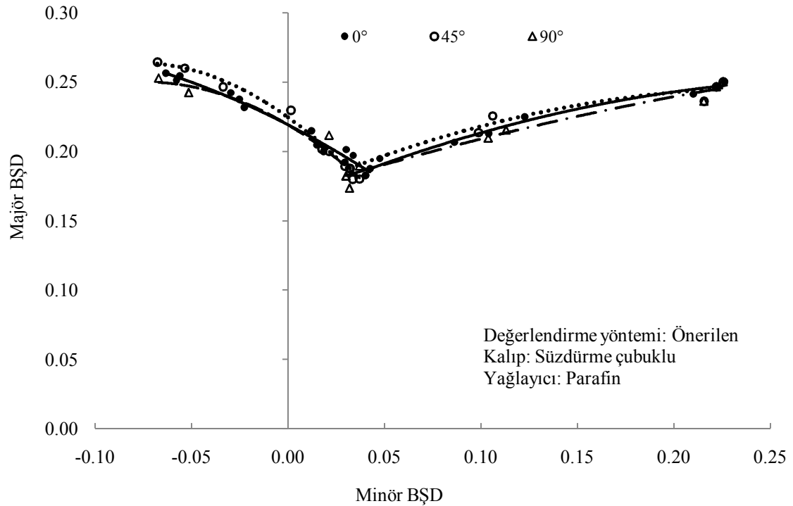
Şekil Ek3.2. 2 mm kalınlıklı Al 2024-T4'ün ŞSE'sinin haddeleme doğrultusuna göre değişimi
