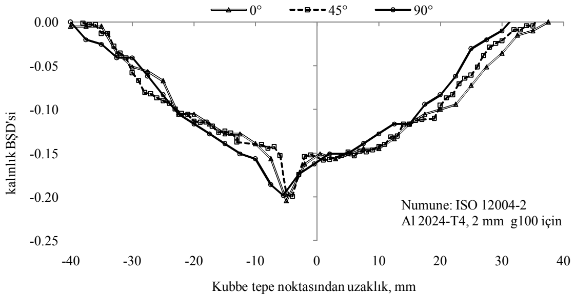
Şekil 4.41. Gerçek kalınlık BŞD dağılımının haddeleme doğrultusuna göre değişimi
