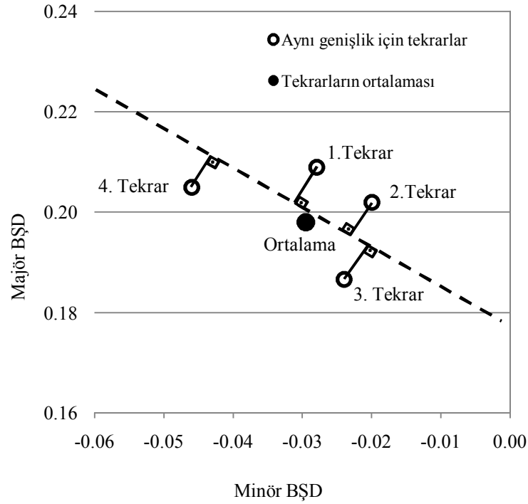
Şekil 3.29. ŞSE oluşturulurken tüm verilere eğri uydurulması
