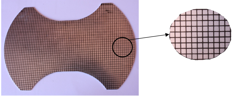
Şekil 3.11. Gridlenen örnek bir Nakajima numunesi
