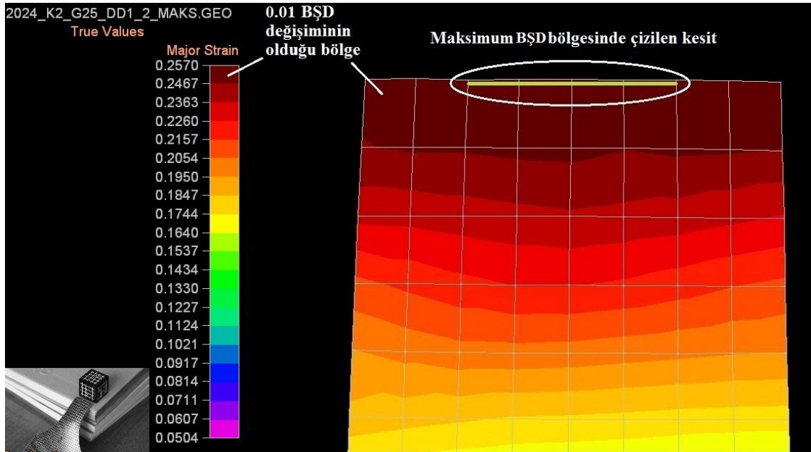
Şekil 3.25. Maksimum BŞD bölgesinde çizilen kesit
