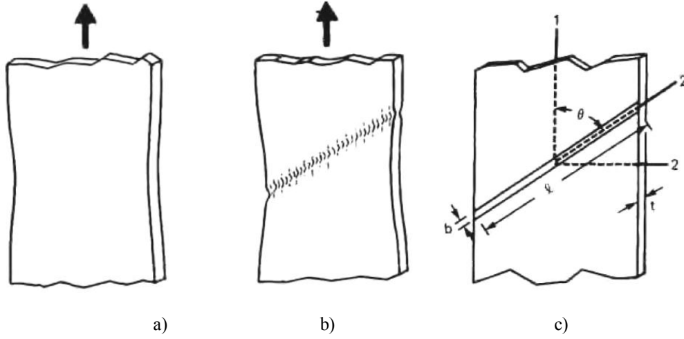
Şekil 2.8. a) Yayılmış b) bölgesel boyunlaşma c) analizde kullanılan koordinat sistemi (Hosford ve Caddell, 2007)
