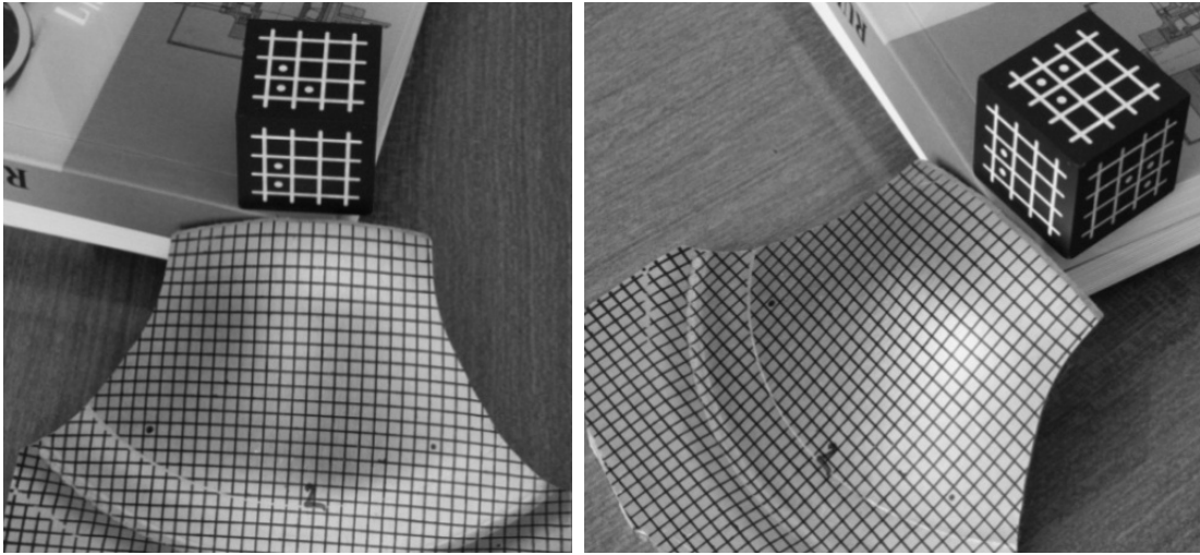
Şekil 3.15. Ölçme alanının iki farklı açıdan çekildiği örnek fotoğraflar
