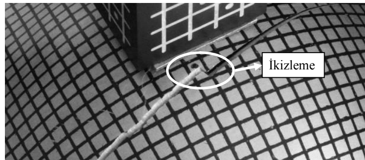
Şekil 3.14. Yırtık bölgesinde ikizleme meydana gelen örnek bir numune
