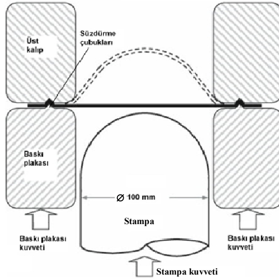
Şekil 2.13. Nakajima deney takımı (Emilie ve ark., 2008)
