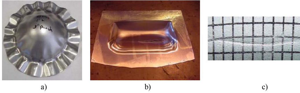
Şekil 2.4. Sac metal şekillendirmede meydana gelebilecek problemler a) buruşma, b) yırtılma, c) bölgesel boyunlaşma (Altan, 1998)
