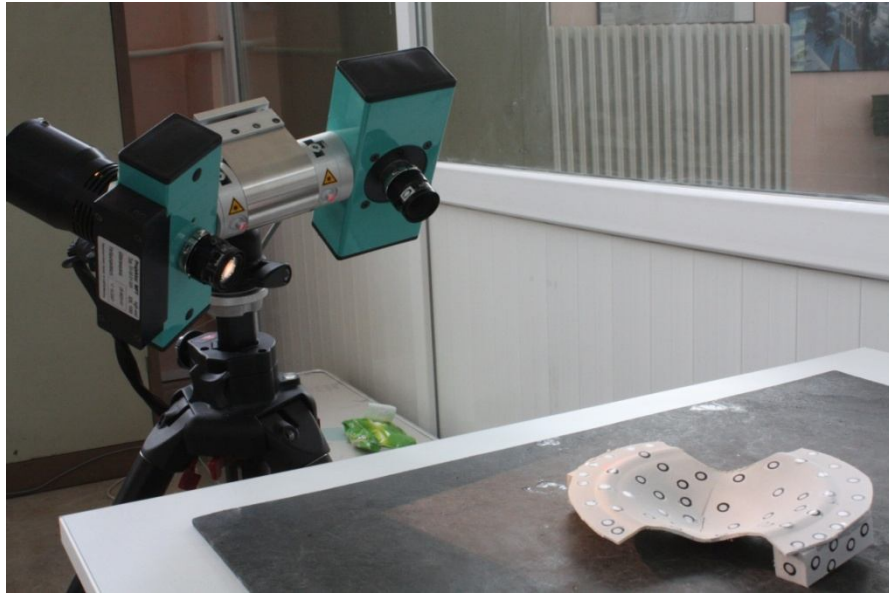
Şekil 3.31. Nakajima numunelerinin optik tarama cihazı ile taranması
