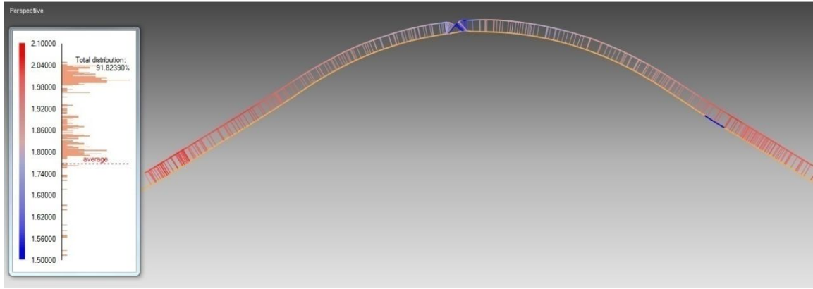
Şekil 3.33. Optik tarama cihazı ile ölçülen örnek bir kalınlık profili
