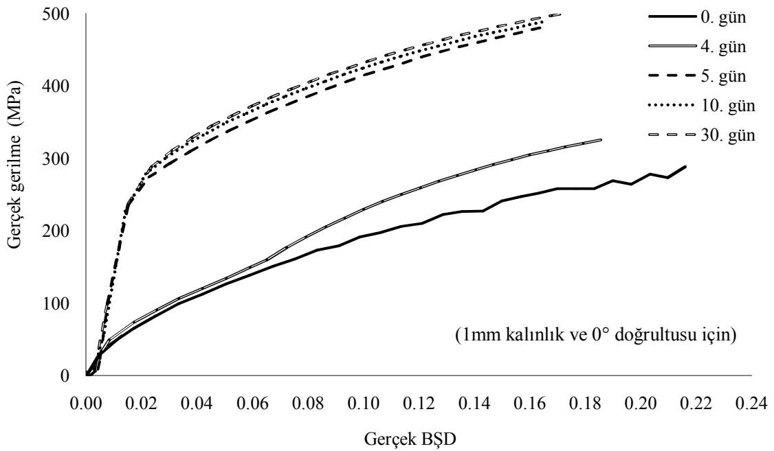
Şekil 4.2. Al 2024 alaşımının doğal yaşlandırma ile mekanik özelliklerinin stabil hale gelmesi
