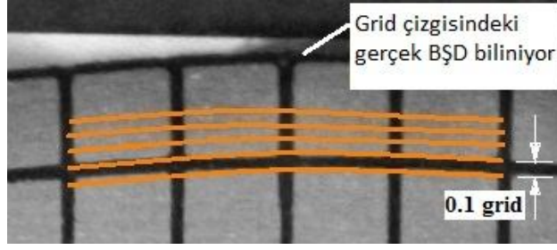
Şekil 3.28. Ekstrapolasyonla elde edilen BŞD değerinin bilinen değerle karşılaştırılması yöntemi
