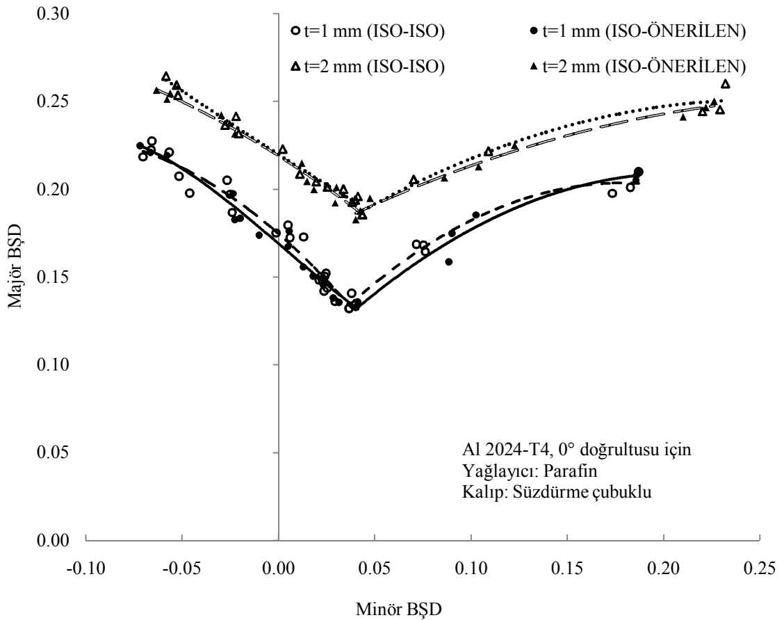
Şekil 4.20. Al 2024-T4 malzemelerin ISO-ISO ve ISO-ÖNERİLEN yöntemlerine göre elde edilen ŞSE'leri
