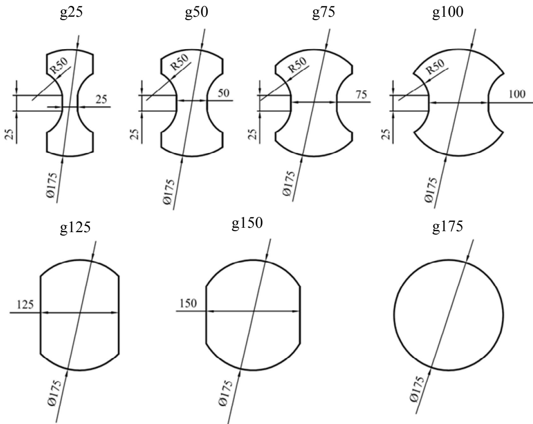
Şekil 3.9. ISO 12004-2 standardında kullanılan Nakajima deney numunesi takımı
