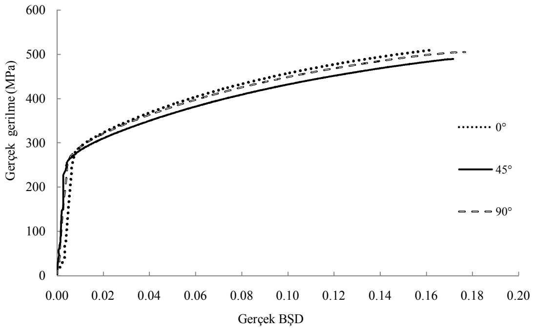
Şekil Ek2.2. a) 0.8, b) 1, c) 1.6 ve d) 2 mm sac kalınlığına sahip Al 2024-T4 sacların 0°, 45° ve 90° doğrultuları için akma eğrileri
