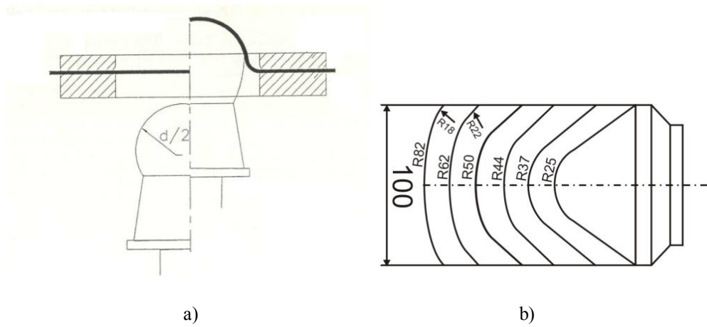
Şekil 2.12. Keeler'in önerdiği a) deney takımı, b) stampa çapları (Keeler ve Backofen, 1963)
