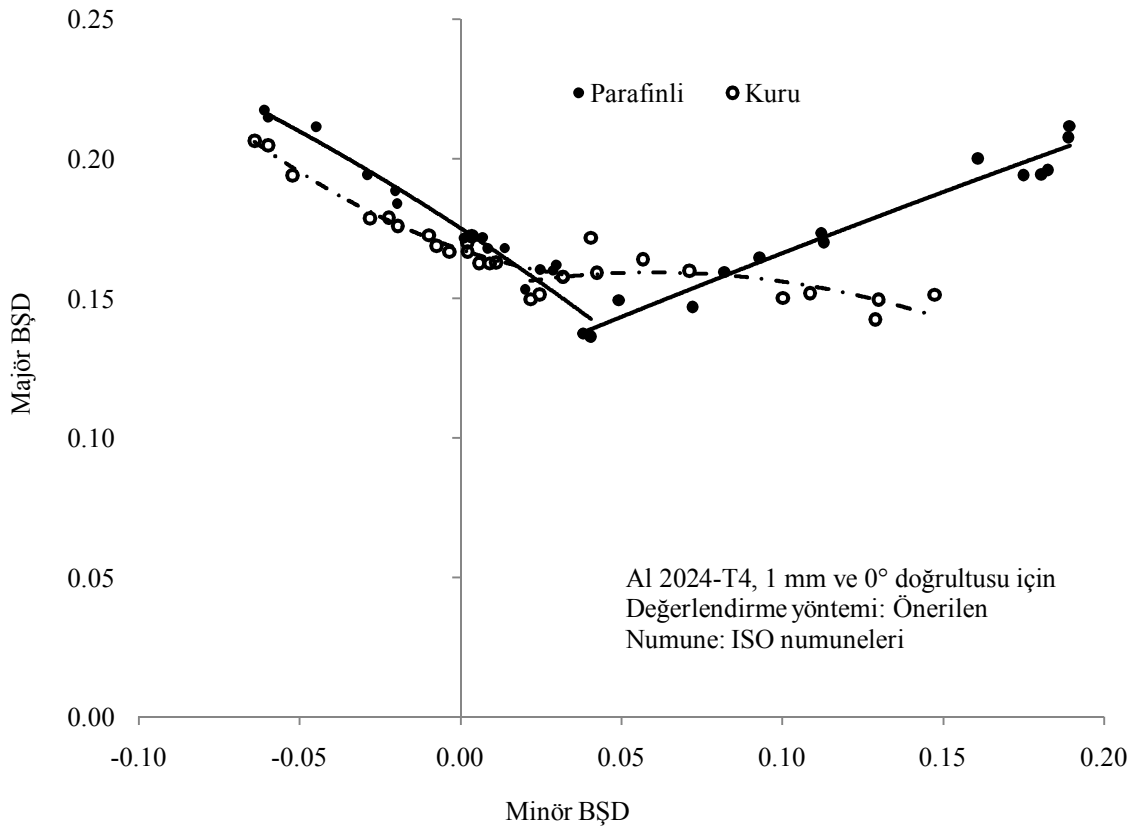
Şekil 4.12. Yağlama durumunun ŞSE üzerindeki etkisi
