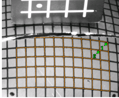
Şekil 3.18. Grid analiz programında oluşturulan tipik bir ızgara yapısı
