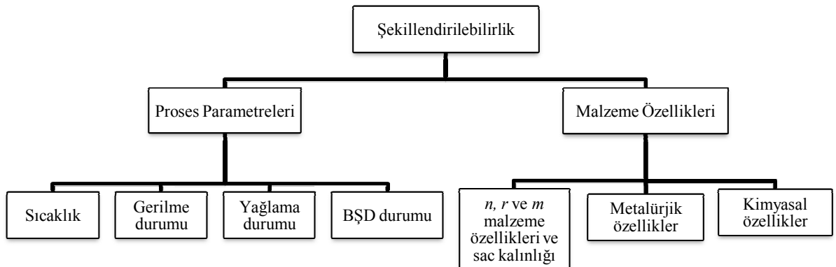
Şekil 2.5. Sac metallerin şekillendirilebilirliğine etki eden parametreler (Önder, 2005)
