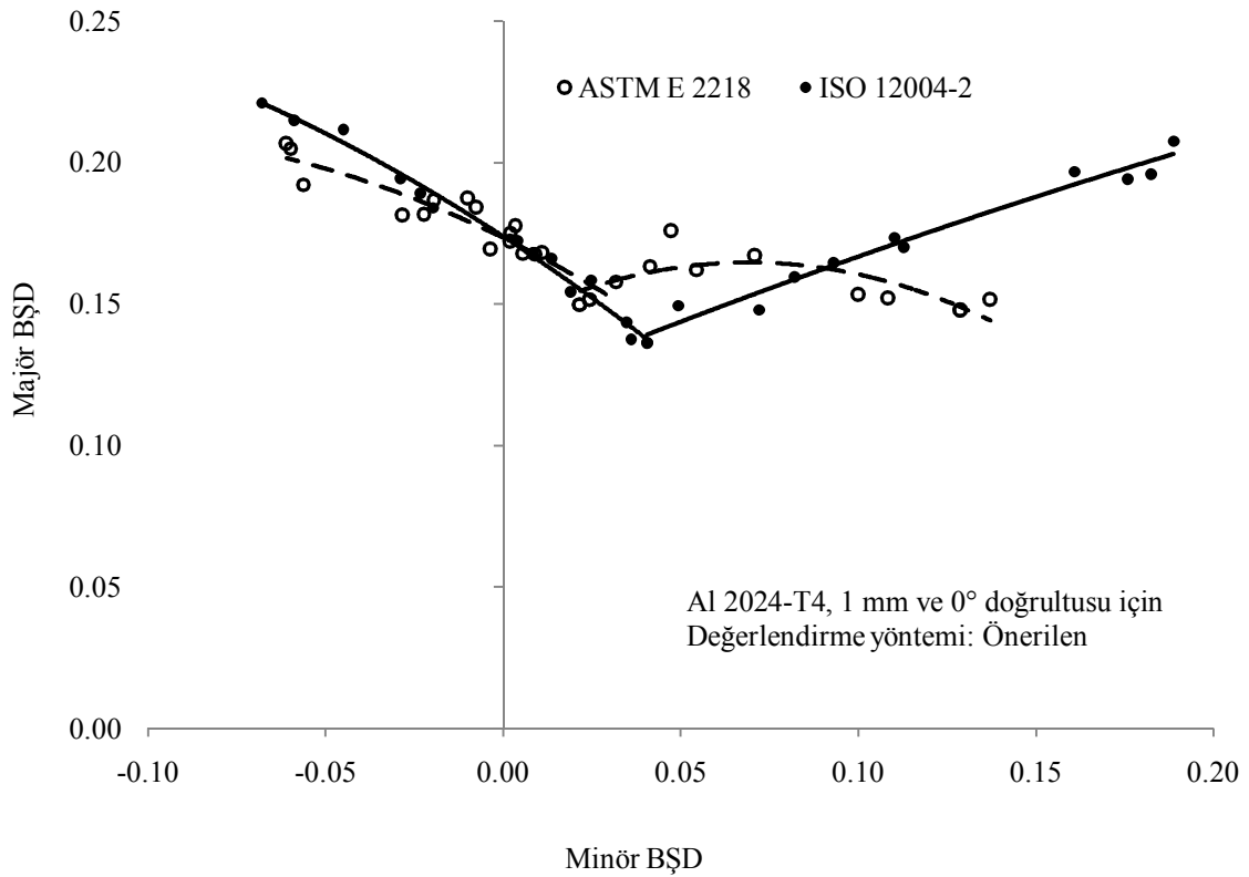
Şekil 4.10. ASTM E 2218-02 ve ISO 12004-2 standartlarına göre elde edilen ŞSE'ler
