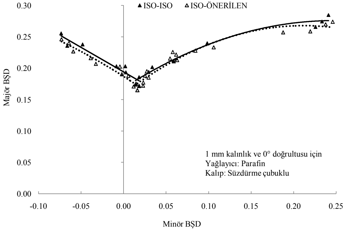
Şekil 4.24. Önerilen yöntemin Al 2024-O için geçerliliği
