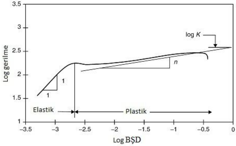
Şekil 3.3. Logaritmik gerilme-BŞD diyagramı (Marciniak ve ark. 2002)
