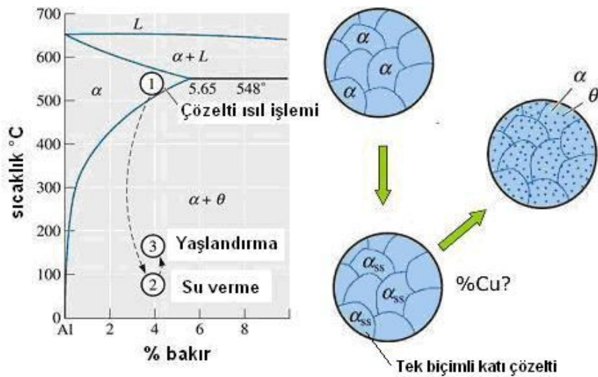
Şekil 3.1. Al-Cu alaşımının çökelme sertleşmesi basamakları ( http://www.keytometals.com )
