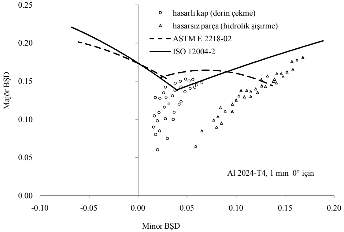
Şekil 4.47. ISO 12004-2 ve ASTM E 2218 standartlarına göre elde edilen ŞSE'lerin güvenilirliğinin durum çalışmasıyla incelenmesi
