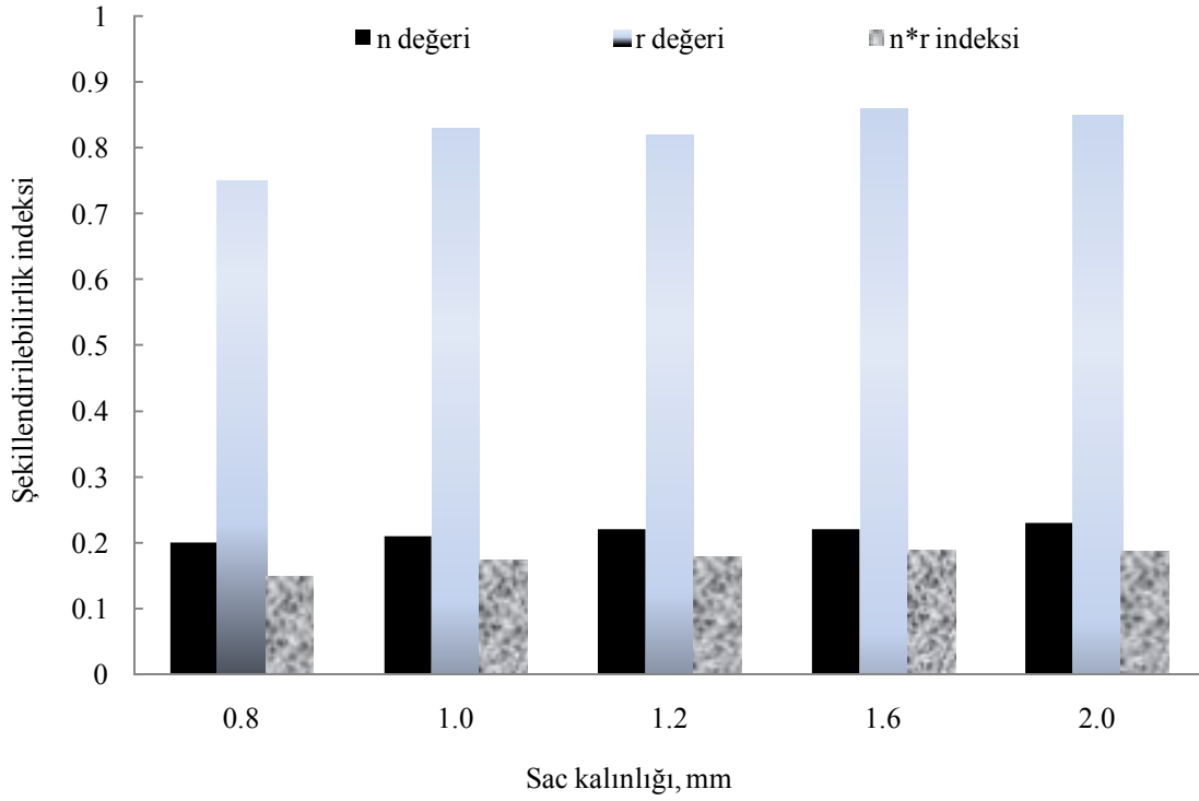
Şekil 4.5. Çeşitli kalınlıktaki Al 2024-T4 saclar için şekillendirilebilirlik indeksi
