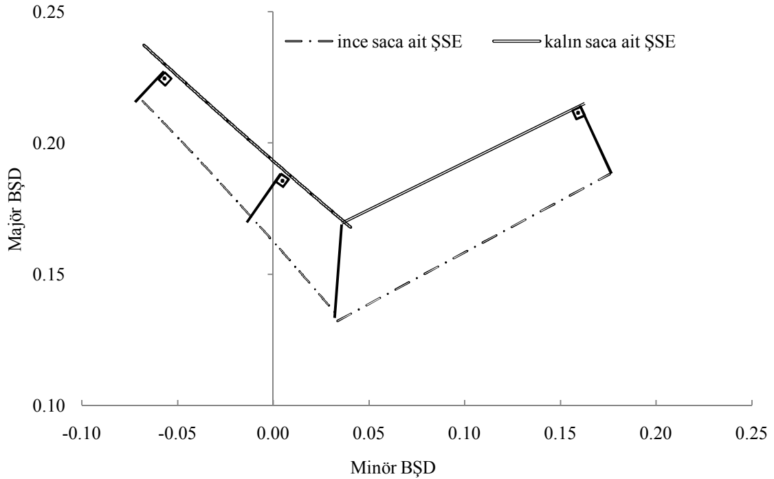
Şekil 3.30. Çeşitli kalınlıklar için ŞSE'ler arasındaki farkın belirlenmesi
