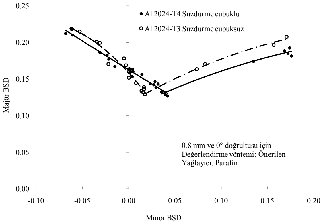
Şekil 4.30. T3 süzdürme çubuksuz ve T4 düz kalıpla elde edilen ŞSE'ler
