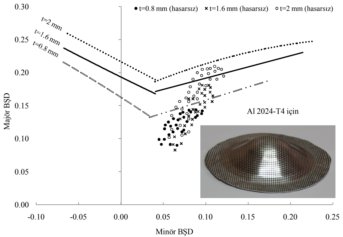
Şekil 4.51. Gerdirmeli çekme deneysel durum çalışması
