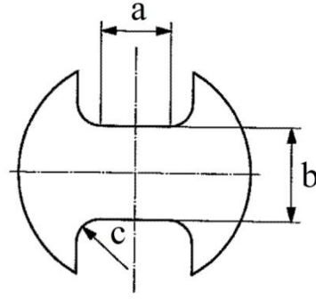
Şekil 3.8. ISO 12004-2 standardında kullanılan tipik Nakajima numune geometrisi
