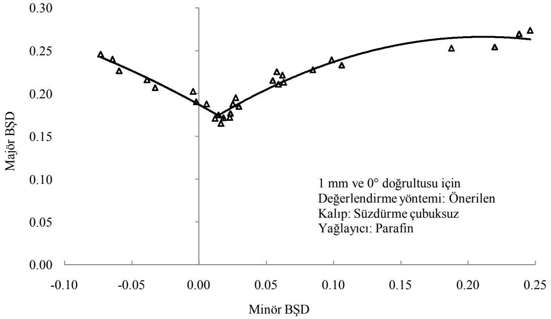
Şekil 4.31. Al 2024-O için ŞSE
