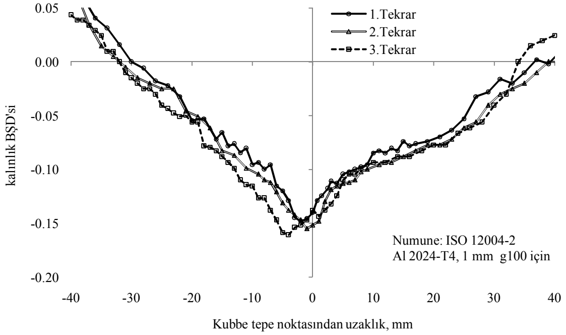
Şekil 4.40. Optik tarama ile kalınlık ölçümünün tekrarlanabilirliği
