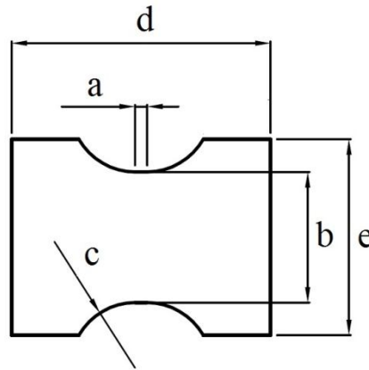
Şekil 3.6. ASTM standardında kullanılan tipik Nakajima numune geometrisi
