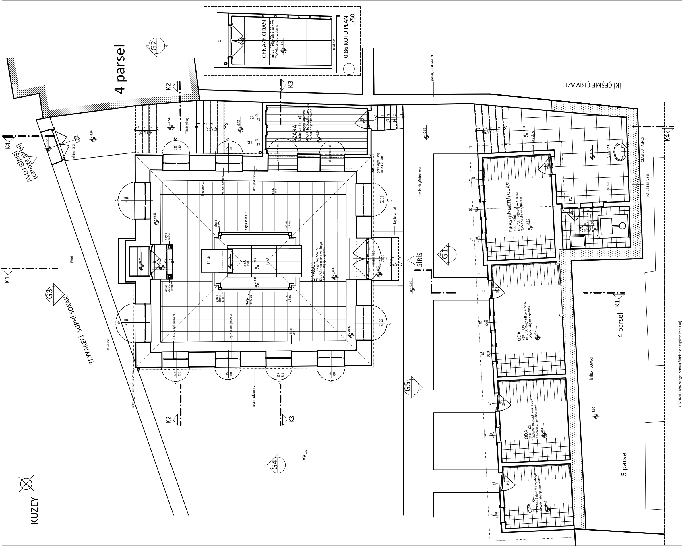
Çizim C.28. Zemin Kat Planı (Restitüsyon- II. Dönem)
