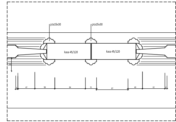
B DETAYI ÖLÇEK: 1/2
