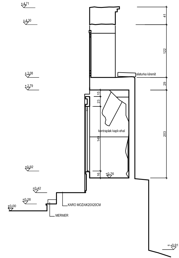
KESİT
