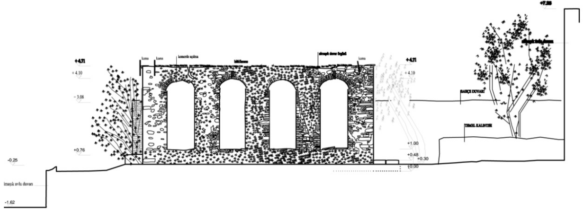
Kuzeydoğu Cephesi-Rölöve
