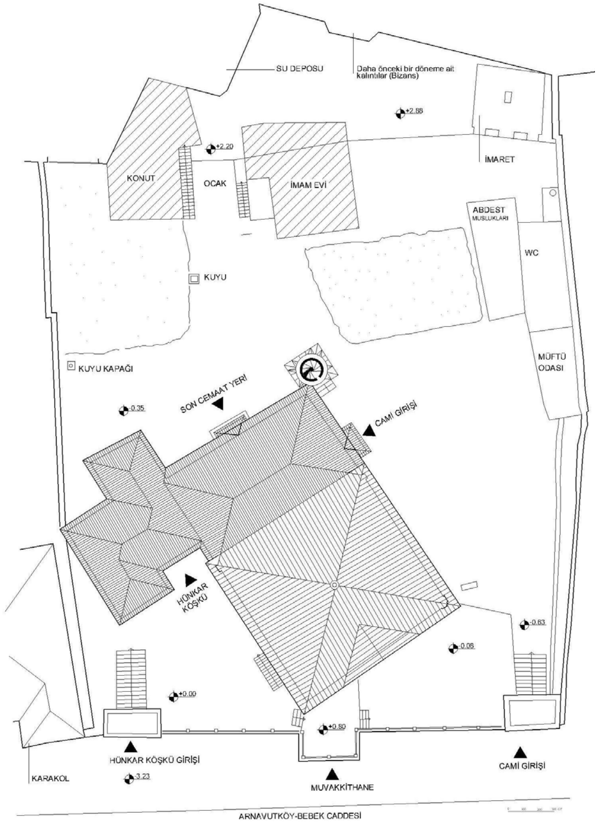
Çizim 2.5. Tefikiye Camii Vaziyet Planı. (KTVKK Arşivi.(Dijital Ortama Aktarılıp Güncellenmiştir)
