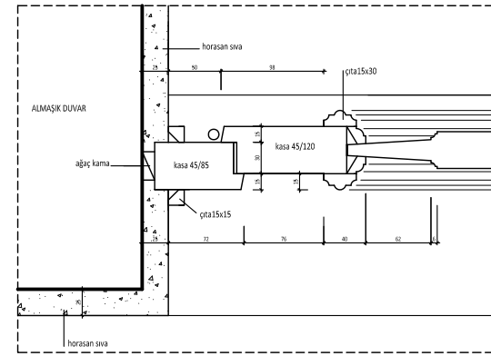
A DETAYI ÖLÇEK: 1/2
