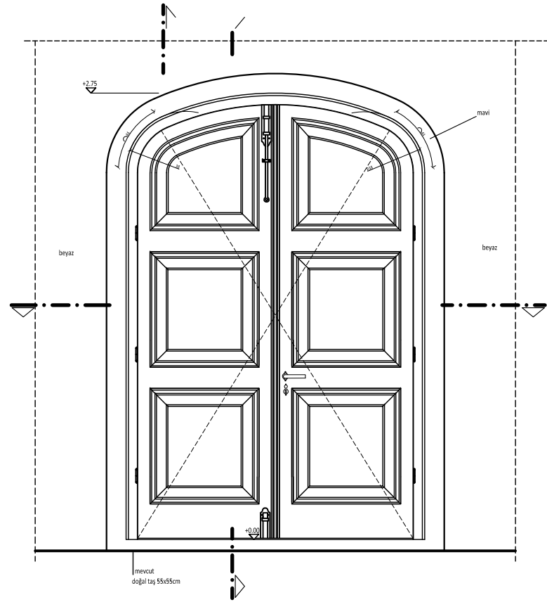
İÇ GÖRÜNÜŞ
