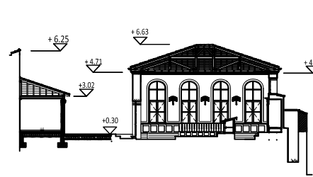
K1 KESİTİ ÖLÇEK:1/200
