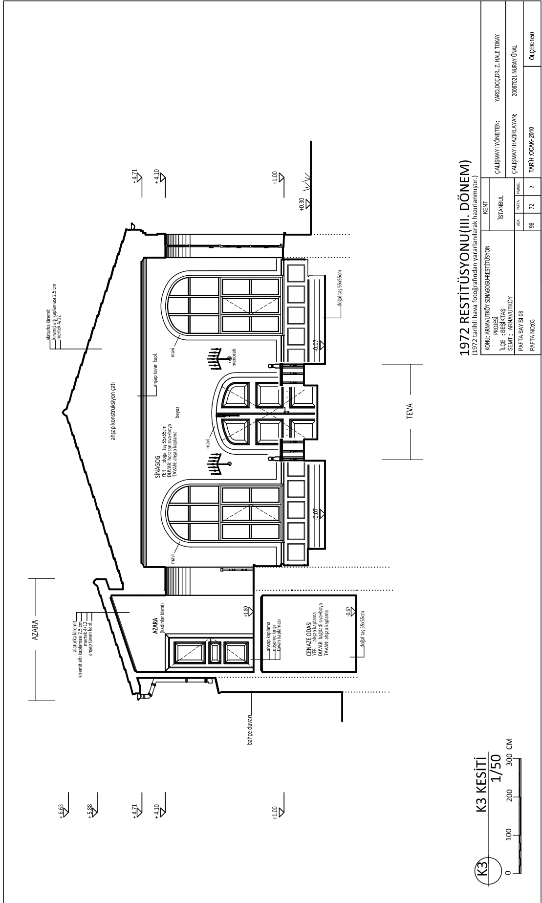
Çizim C.41. K3 Kesiti (Restitüsyon- III. Dönem)
