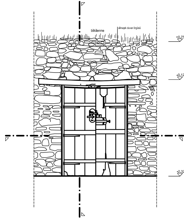
İÇ GÖRÜNÜŞ
