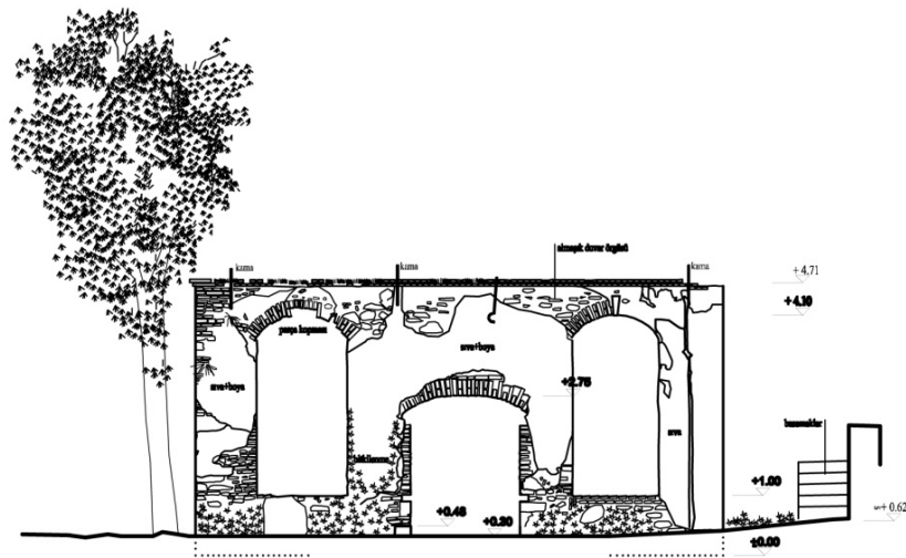
Kuzeybatı Cephesi-Rölöve
