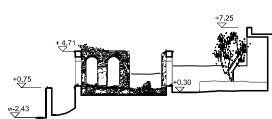
K1 KESİTİ 1/200
