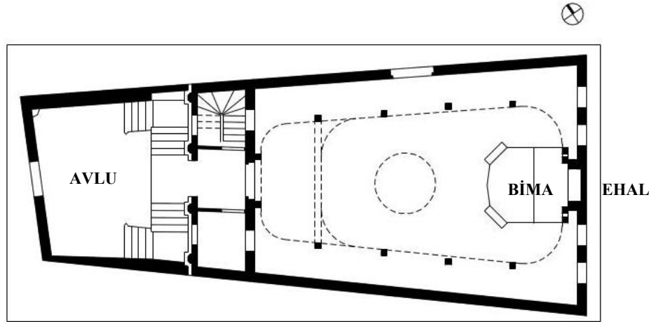
Şekil 1.5. Merkezi Planlı Yenilikçi Sinagog Plan Şeması Örneği, İtalyan Sinagogu-Karaköy (Tuna,S.,2006,s.139)
