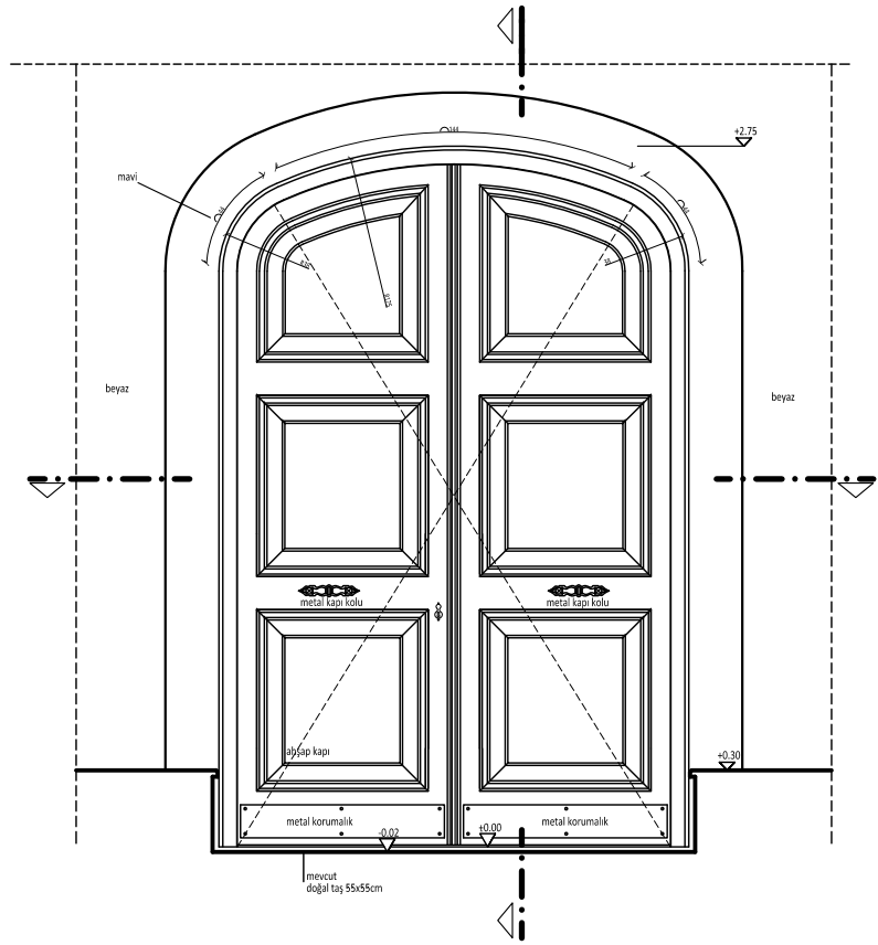
DİŞ GÖRÜNÜŞ
