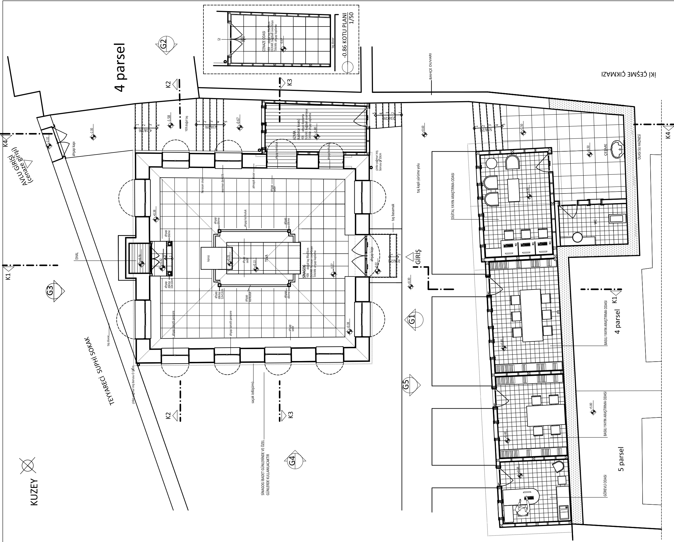
Çizim C.50. Zemin Kat Planı- Tefrişli (Restorasyon)
