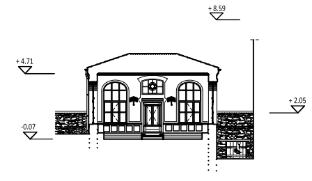
K2 KESİTİ ÖLÇEK:1/200
