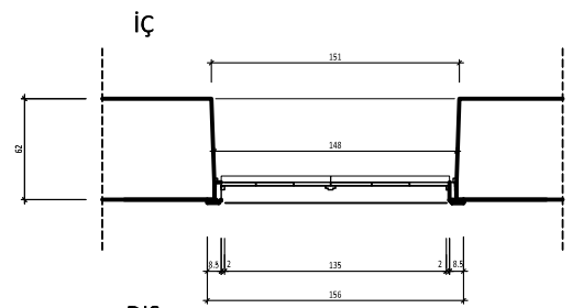
DIŞ
