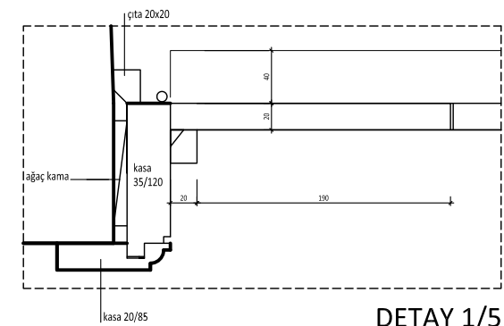
DETAY 1/5
