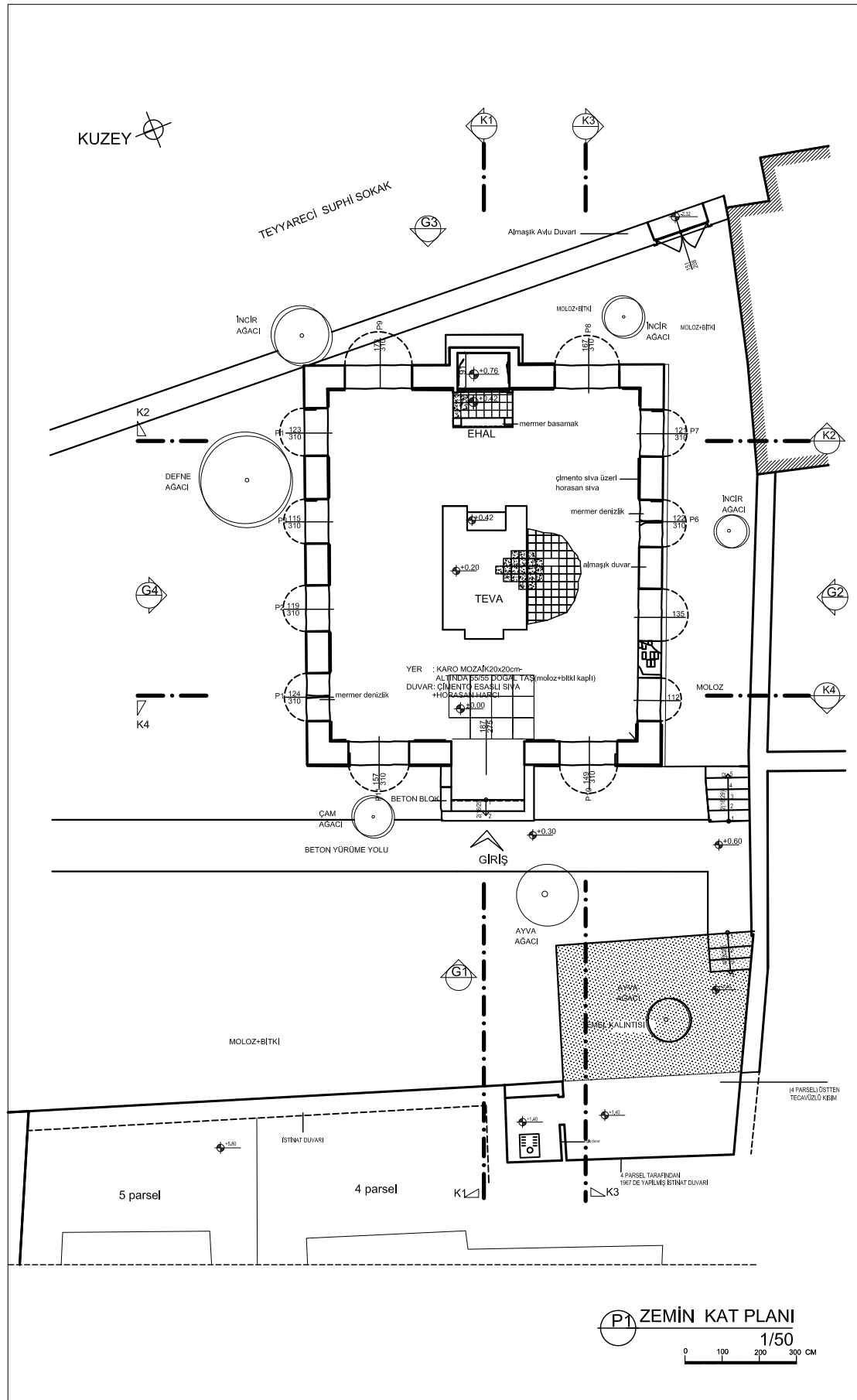
Zemin Kat Planı (Rölöve)
