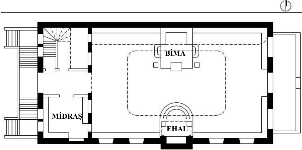
Şekil 1.7.Çift Odaklı Sinagog Plan Şeması örneği, Hemdat İsrail Sinagogu-Haydarpaşa (Tuna,S., 2006, s.138)
