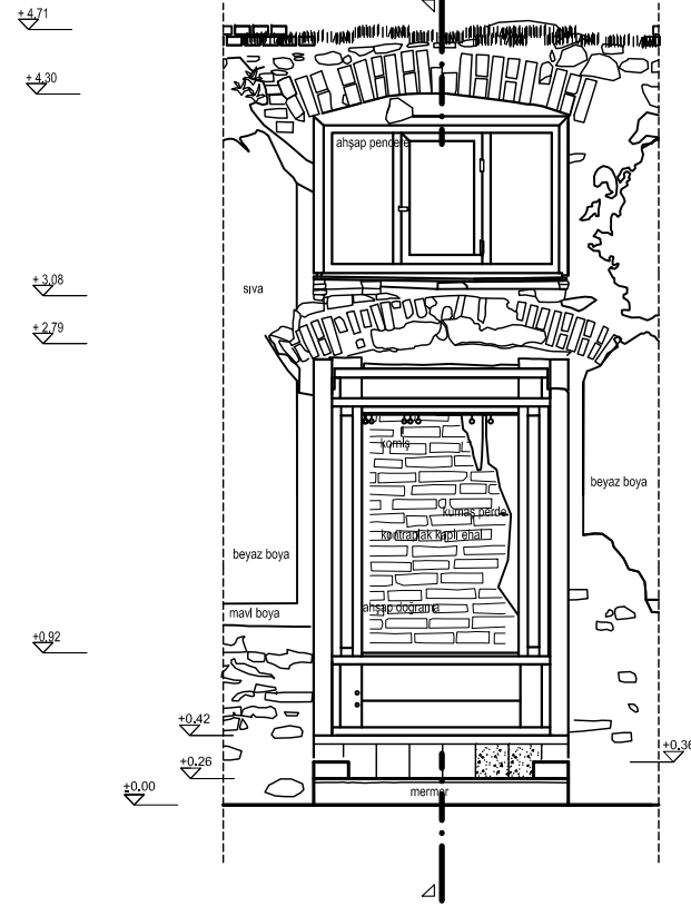
İÇ GÖRÜNÜŞ
