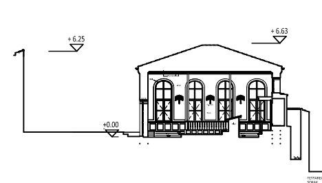
K1 KESİTİ ÖLÇEK:1/200
