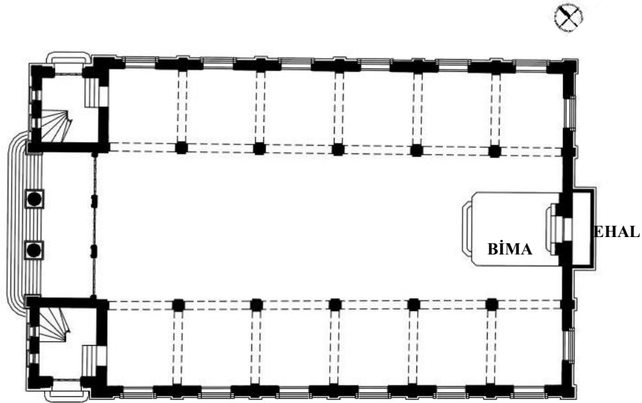
Şekil 1.6. Bazilikal Planlı Sinagog Plan Şeması Örneği, Edirne Büyük Sinagogu (Tuna,S.,2006, s.125)
