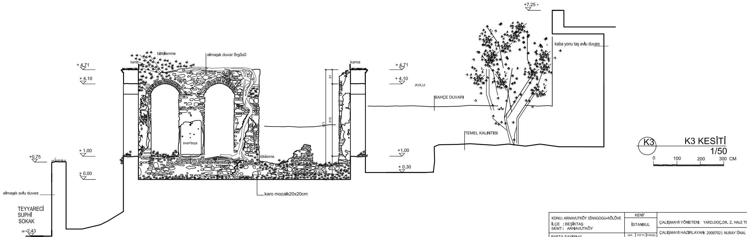
Çizim C.4. K1 ve K3 Kesitleri (Rölöve) 225
