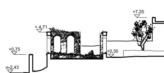
K1 KESIT| 1/200
