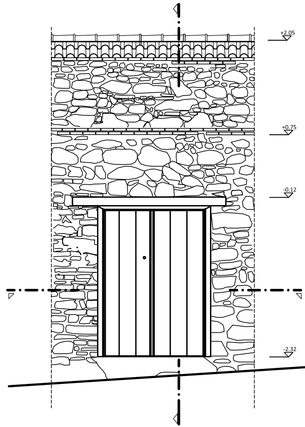
DIŞ GÖRÜNÜŞ
