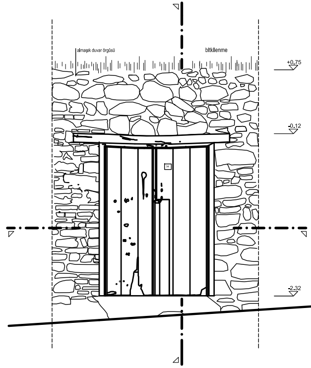
DIŞ GÖRÜNÜŞ
