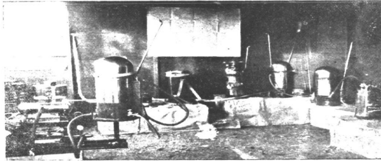
Macar pavnyonunda haseerat illâfina aile tulumbalar
