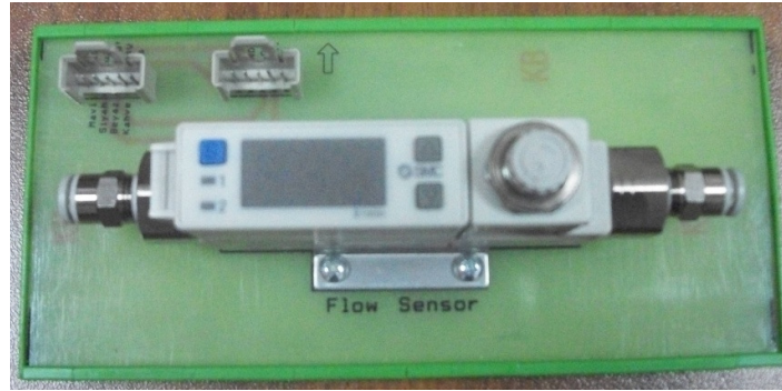
Şekil 5.9. İnspirasyon akış sensörüne ait elektronik kart düzeneği
