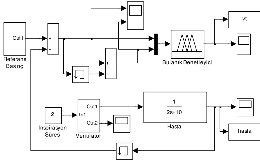
Şekil 4.21. Tidal volümün bulanık denetleyici ile kontrolü
