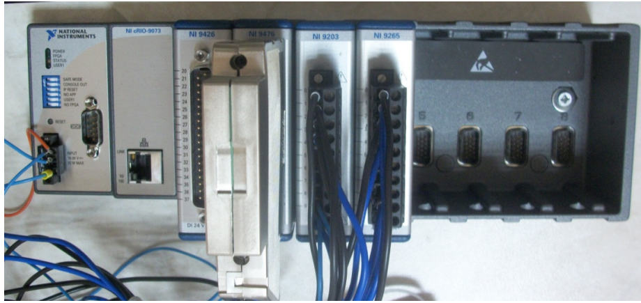
Şekil 5.3. c-RIO 9073 ve analog/dijital giriş/çıkış modülleri
