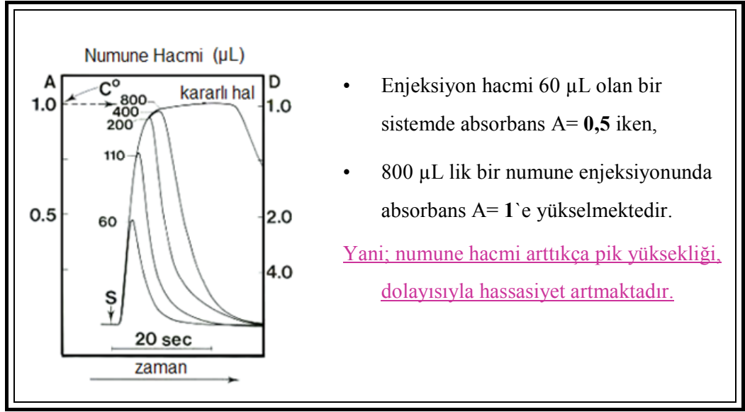
Şekil 4. 4. Akış enjeksiyon analizlerinde (FIA) numune hacminin etkisi
