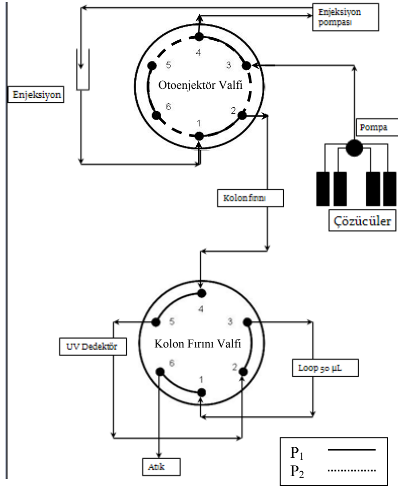
Şekil 6. 11. Hümik asitlerin tespiti için kullanılan akış enjeksiyon sisteminin şematik gösterimi:
