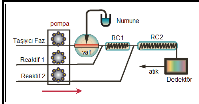
Şekil 4. 3. Akış enjeksiyon (FI) sistemlerinde türevlendirme reaktifinin kullanımı
