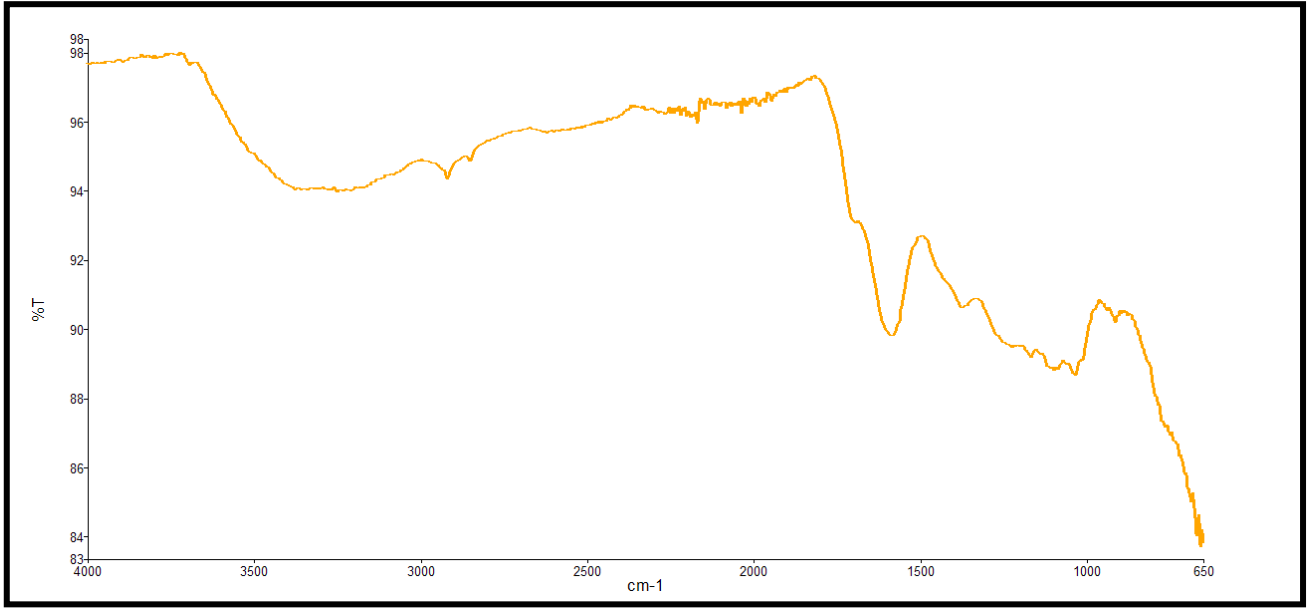
Şekil 2. 7. Hümik asit için örnek bir FTIR spektrumu
