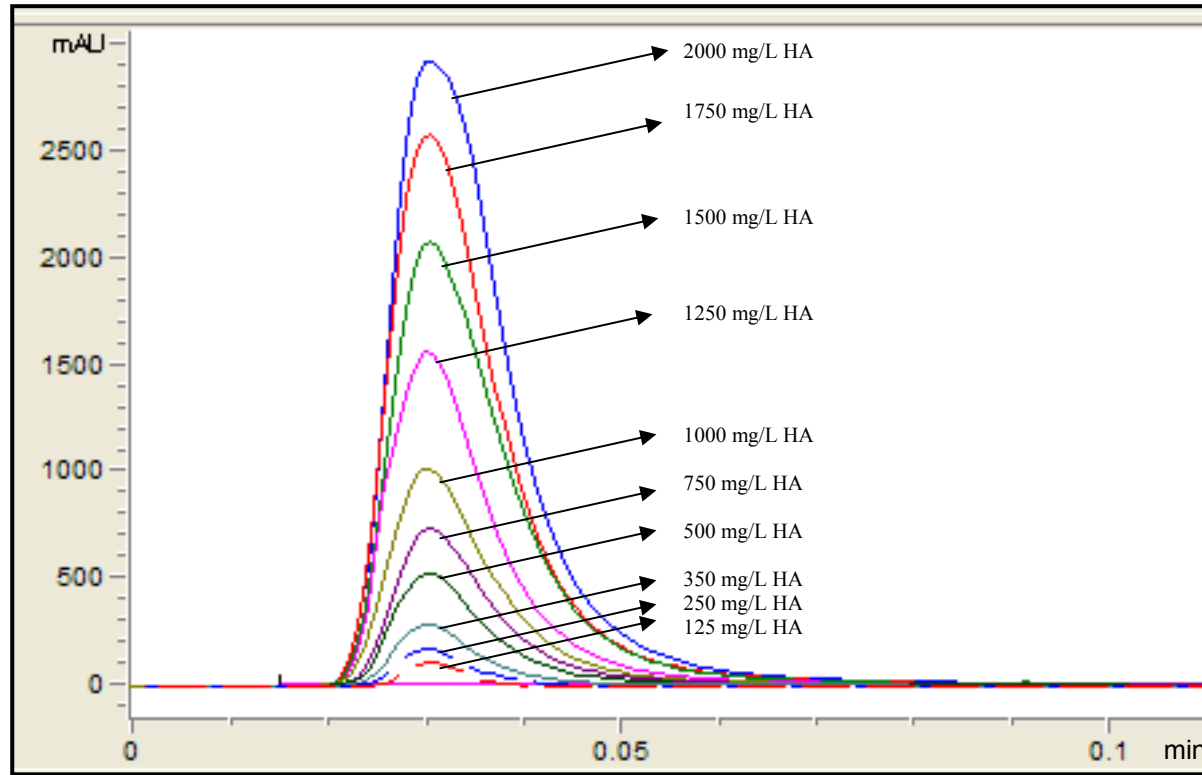
Şekil 7. 22. Parametreleri optimize edilmiş FIA sistemi ile enjeksiyonu yapılan 125 – 2000 mg/L aralığındaki hümik asit standartlarının sırasıyla küçükten büyüğe pikleri
