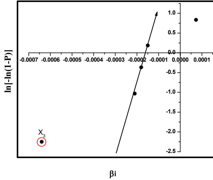
Şekil 7. 14. Sıcaklık ve numune hacmi faktörlerinin cevap değerine olan tesirlerini gösteren normal dağılım grafiği
