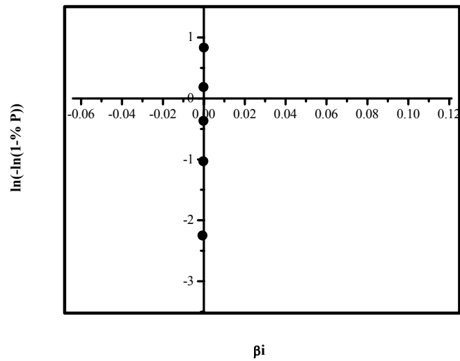
Şekil 7. 15. Şekil 7.10.'da verilmiş olan normal dağılım grafiğinin skalasında çizilen numune hacmi ve sıcaklık faktörlerinin normal dağılım grafiği
