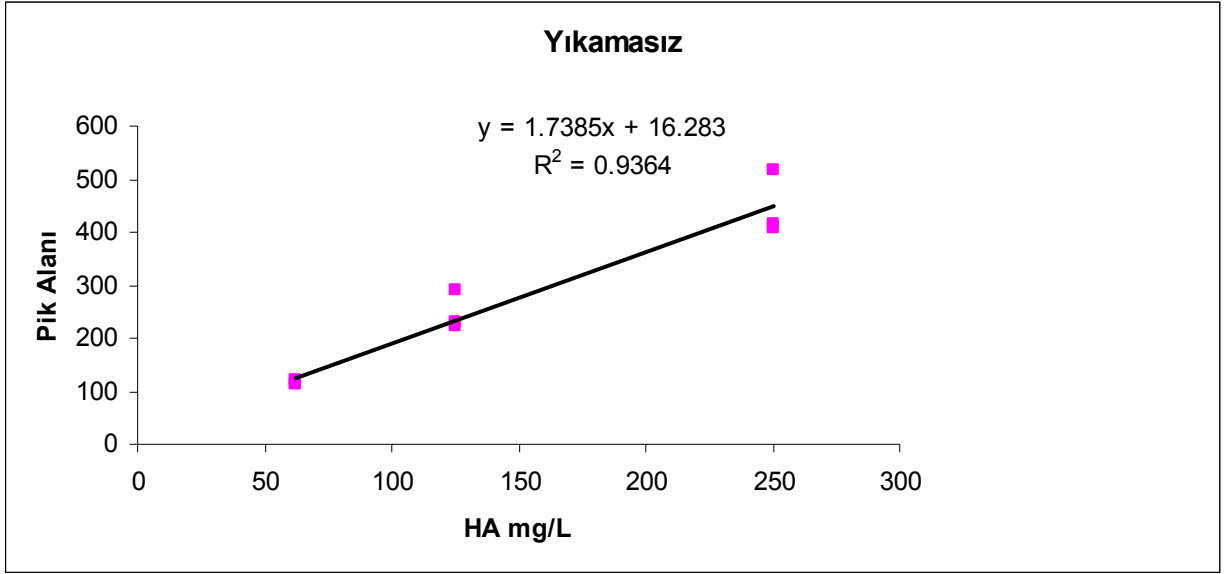
Şekil 7. 7. Enjektör yıkanmadan yapılan analizlerden elde edilen 3 HA standardın sisteme verilmesiyle elde edilen 9 pik alanının bir arada gösterimi
