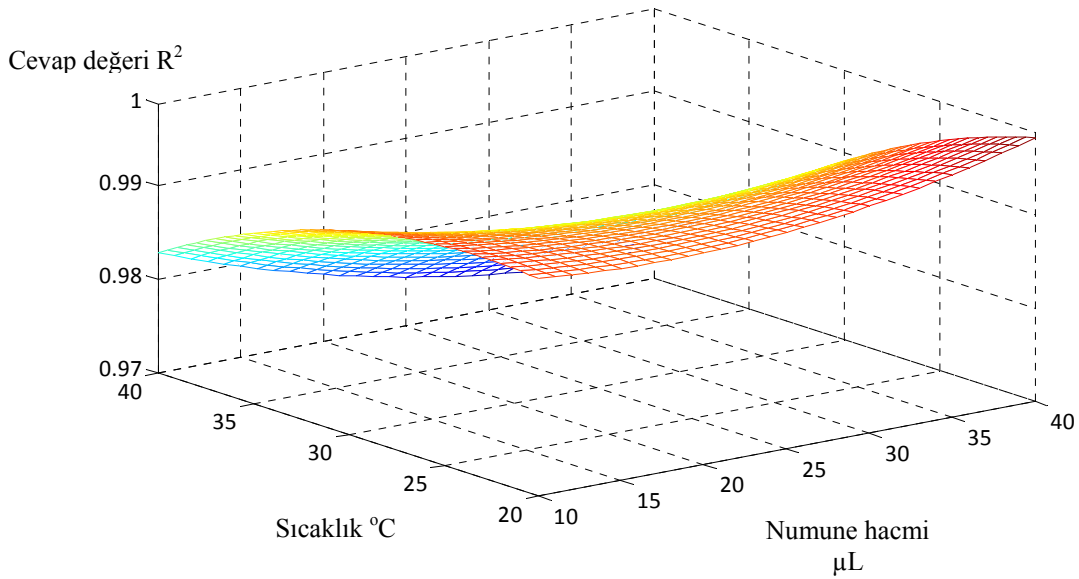
Şekil 7. 16. Değişen sıcaklık ve numune hacmi değerlerinde R^2 'de meydana gelen değişimi gösteren 3 boyutlu yüzey grafiği
