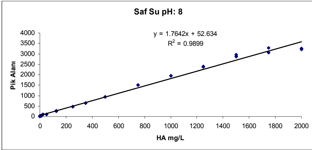
Şekil 7. 19. Saf su pH: 8 hareketli fazı ile FIA sistemine enjekte edilen 0-2000 mg/L'lik HA standartlarının kalibrasyon grafiği
