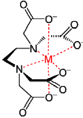
Şekil 2. 9. Hümik maddelerin kompleksleşmesine örnek olarak Metal-EDTA kompleksi
