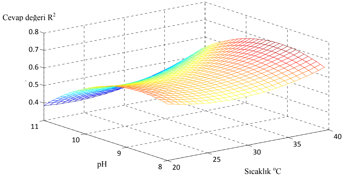
Şekil 7. 12. Değişen pH ve sıcaklık değerlerinde R^2 'de meydana gelen değişimi gösteren 3 boyutlu yüzey grafiği
