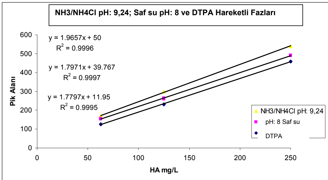
Şekil 7. 18. \text{NH}_3/\text{NH}_4\text{Cl} pH: 9,24; saf su pH: 8 ve DTPA hareketli fazları ile FIA sistemine enjekte edilen 62,5; 125 ve 250 mg/L'lik HA standartlarının pik alanlarının karşılaştırılması
