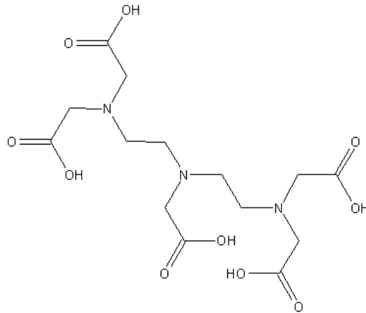
Şekil 7. 3. DTPA molekülü
