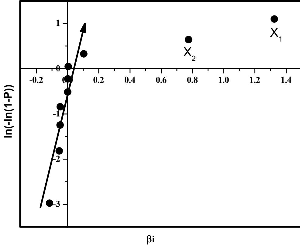
Şekil 5. 2. Etkilerin normal dağılım grafiği
