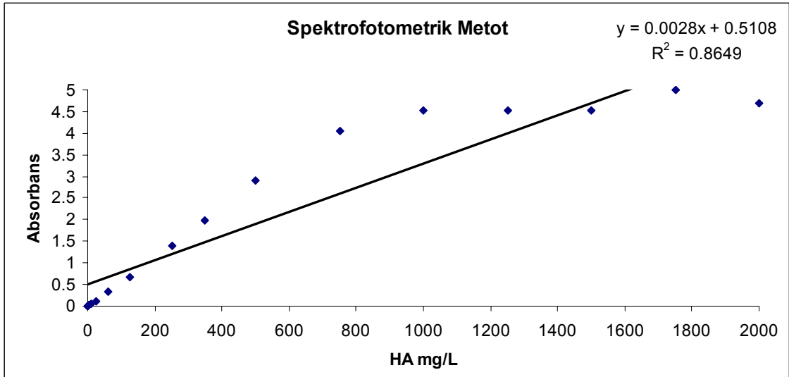
Şekil 7. 24. Spektrofotometrik metotla elde edilen kalibrasyon grafiği
