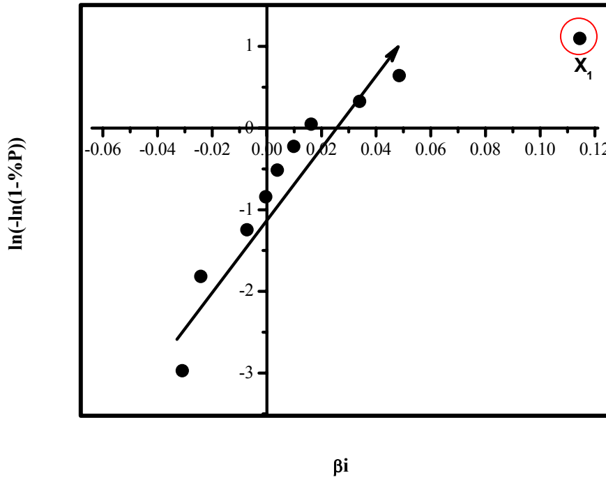
Şekil 7. 10. Akış hızı, pH ve sıcaklık faktörlerinin cevap değerine olan tesirlerini gösteren normal dağılım grafiği
