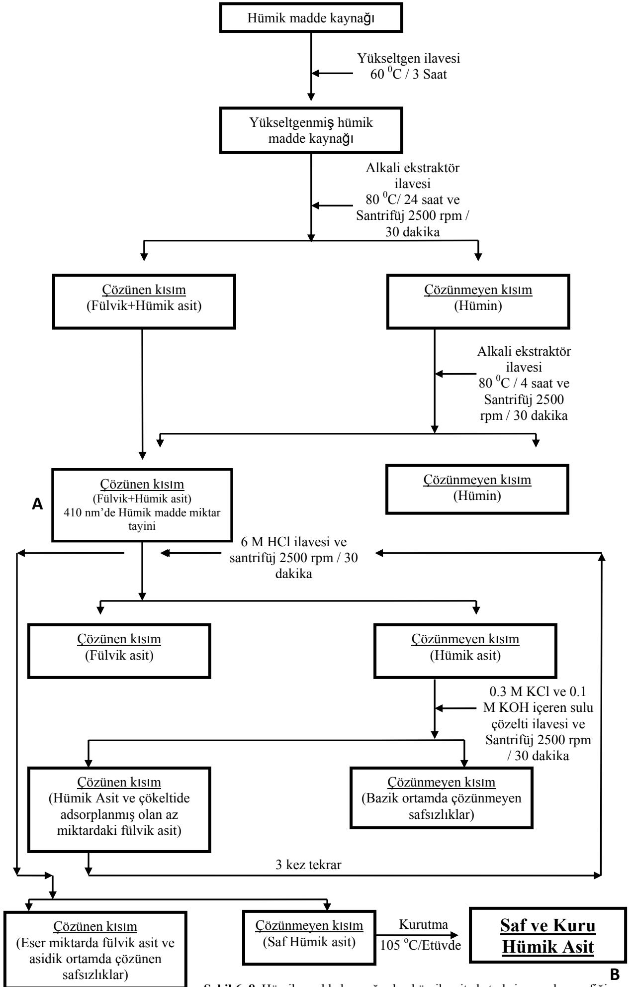
Şekil 6. 8. Hümik madde kaynağından hümik asit ekstraksiyonu akış grafiği
