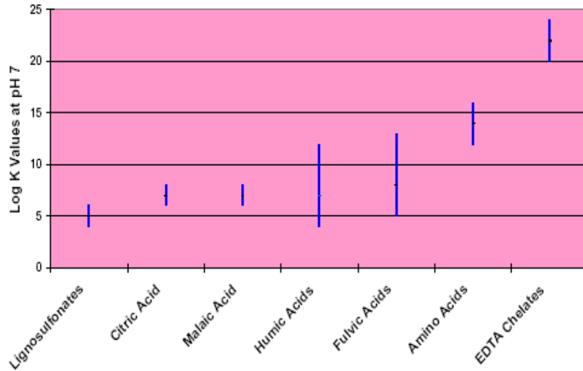
Şekil 2. 6. Cu (II) için pH=7'deki Log K Değerleri
