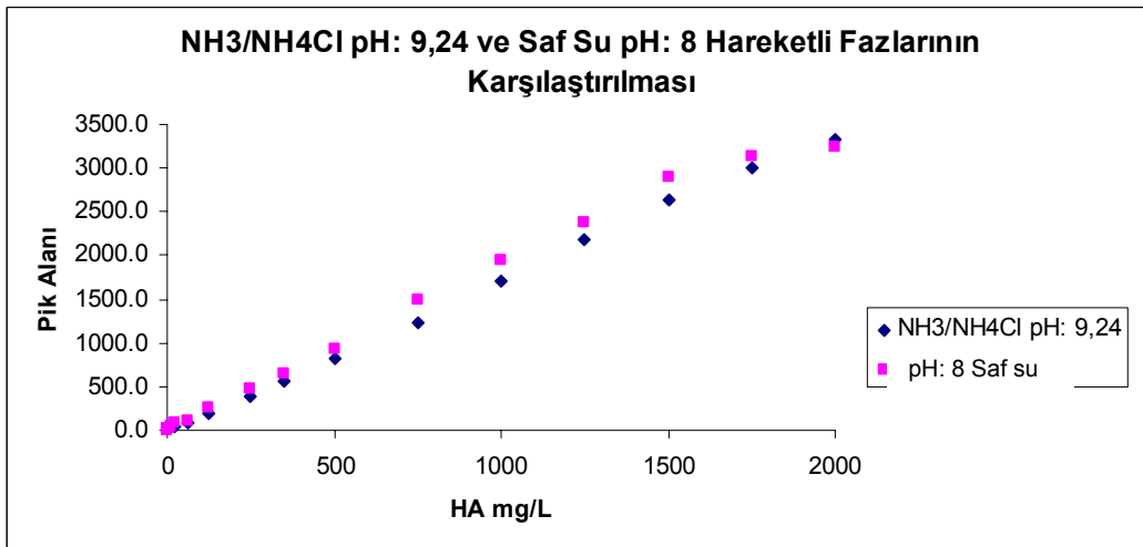
Şekil 7. 21. NH 3 /NH 4 Cl pH: 9,24 ve saf su pH: 8 hareketli fazları ile FIA sistemine enjekte edilen 0-2000 mg/L'lik HA standartlarının pik alanlarının karşılaştırılması
