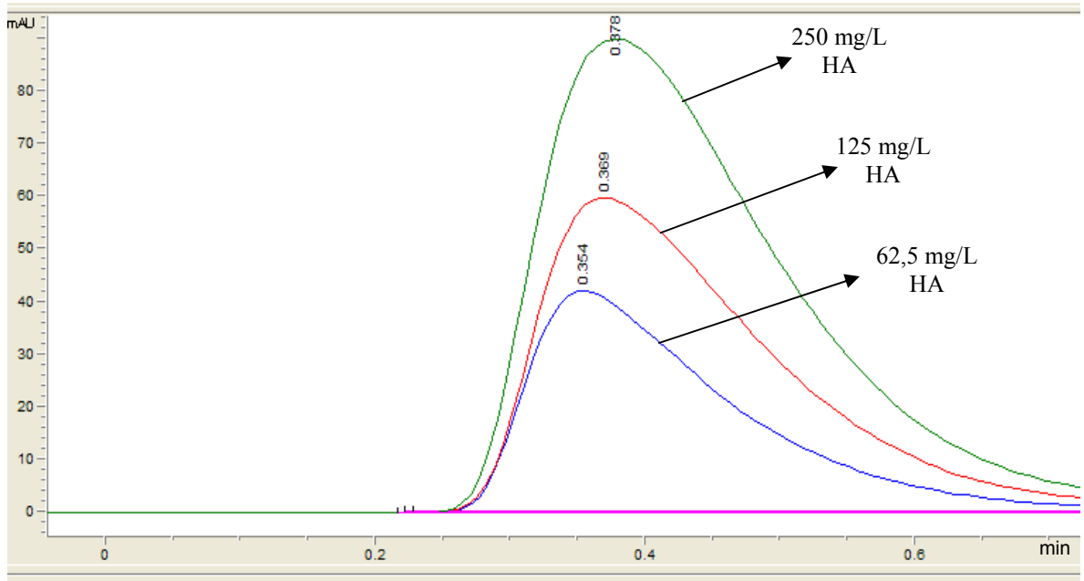
Şekil 7. 5. DTPA çözeltisi hareketli fazında sisteme enjekte edilen 3 HA standardı pikinin bir arada gösterilişi
