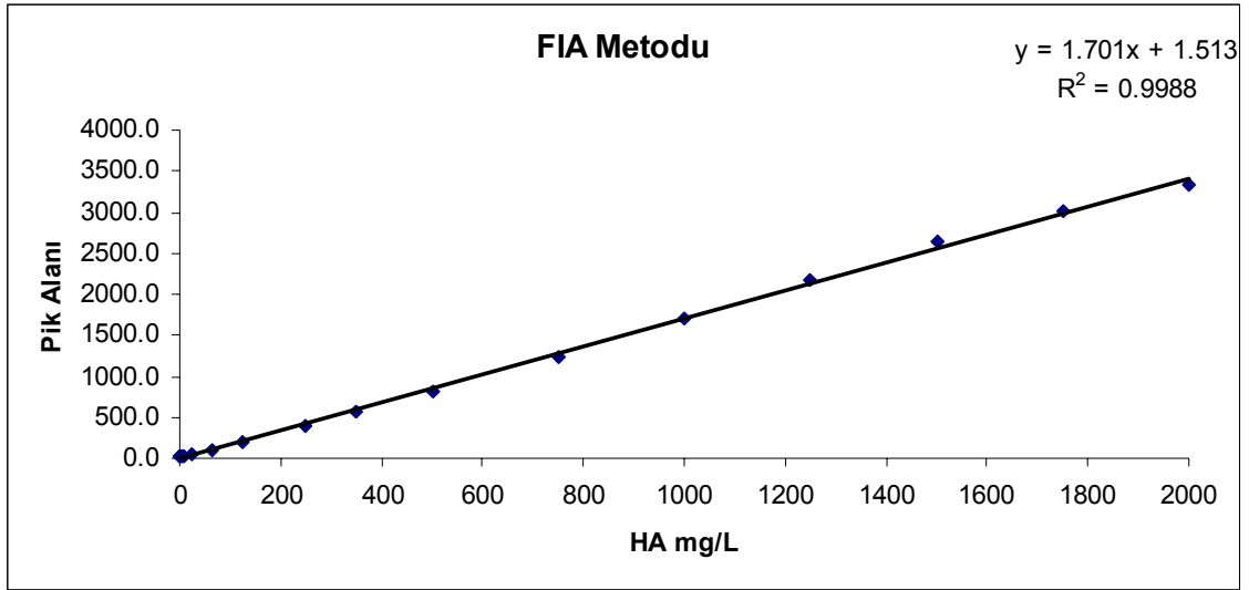
Şekil 7. 23. FIA metoduyla elde edilen kalibrasyon grafiği
