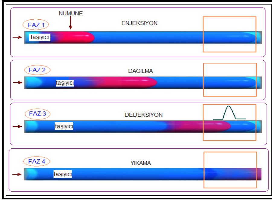
Şekil 4. 2. Akış enjeksiyon (FI) sistemlerinin çalışma prensibinin şematik gösterimi
