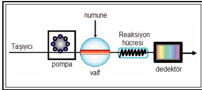
Şekil 4. 1. Akış enjeksiyon (FI) sistemi
