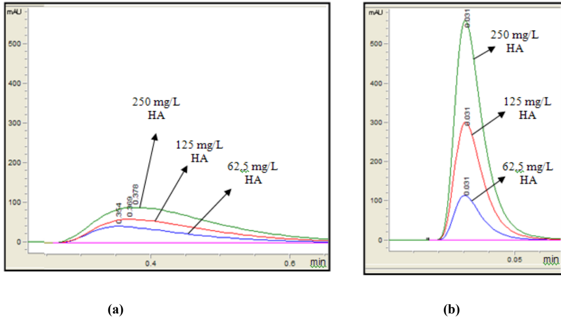
Şekil 7. 6. Sistem bağlantılarının değişiminin pikler üzerindeki etkisi: (a) Eski sistemle elde edilen HA pikleri (iç çapı: 0,50 mm), (b) yeni sistemle elde edilen HA pikleri (iç çapı: 0,18mm)
