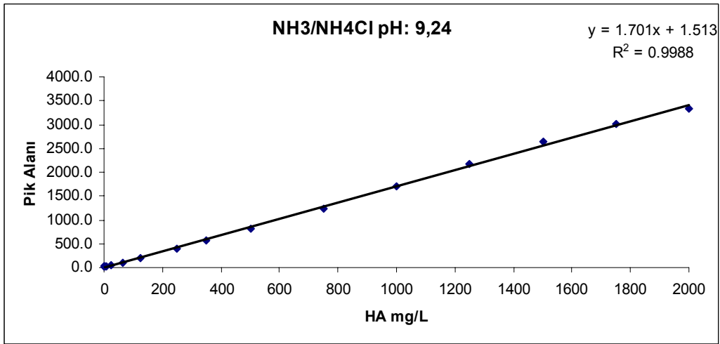
Şekil 7. 20. NH 3 /NH 4 Cl pH: 9,24 hareketli fazı ile FIA sistemine enjekte edilen 0-2000 mg/L'lik HA standartlarının kalibrasyon grafiği
