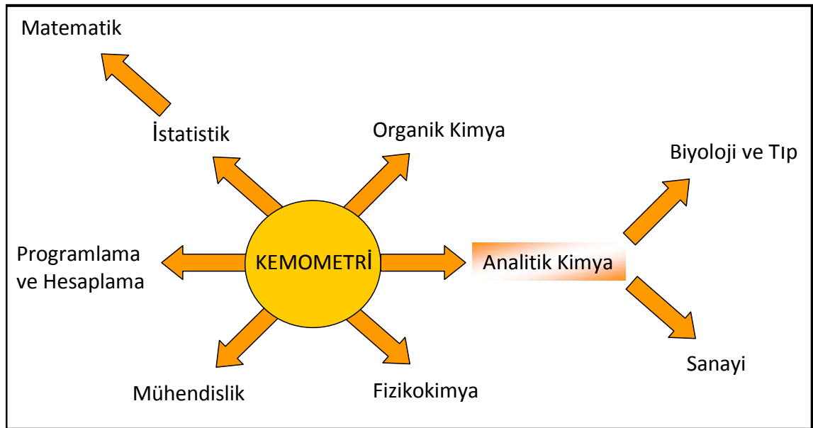
Şekil 5. 1 Kemometrinin ilişkili olduğu disiplinler (Dinç, 2007)
