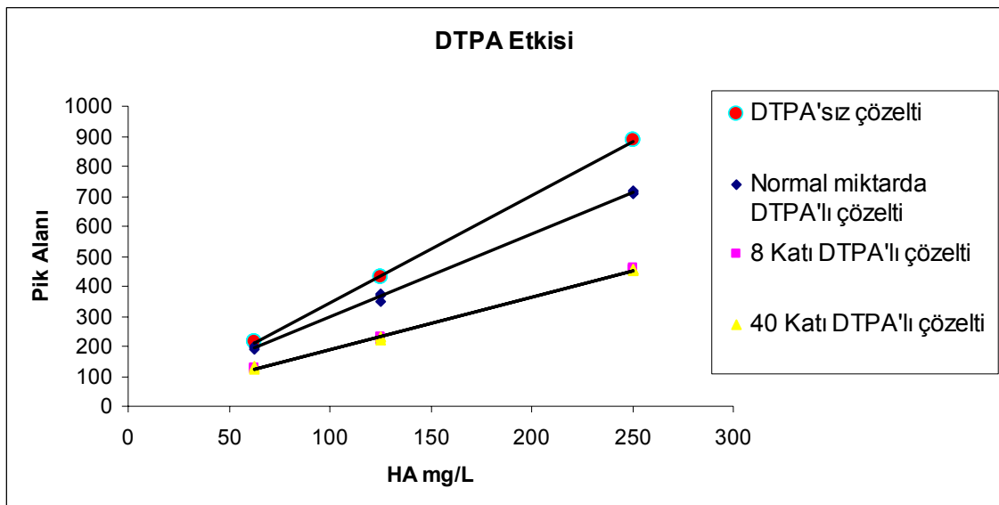
Şekil 7. 17. Farklı konsantrasyonlarda DTPA içeren DTPA çözeltileriyle yapılan analizlerin sonuçları
