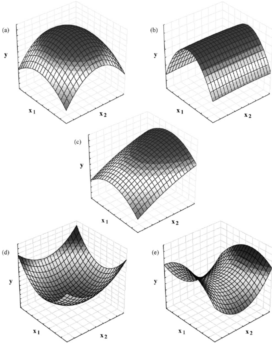
Şekil 5.3. İki değişkenli bir sistemin optimizasyonunda kullanılan kuadratik modelden elde edilen yüzey grafiklerinin bazı profilleri: (a) maksimum, (b) plato, (c) maksimum nokta deneysel alanın dışarısında, (d) minimum ve (e) eğri yüzey (Bezerra ve ark., 2008).
