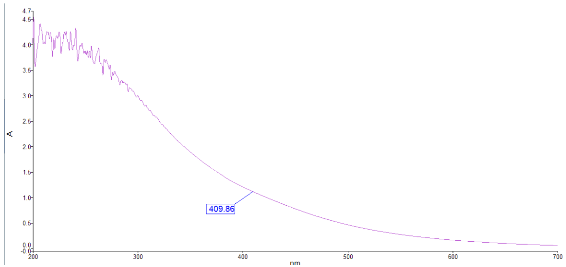
Şekil 6. 9. Örnek olarak verilmiş olan bir hümik asit çözeltisi UV spektrumu
