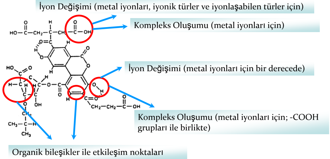
Şekil 2. 4. Hümik asitlerin başlıca etkileşim bölgeleri ve fonksiyonları
