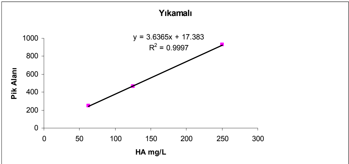
Şekil 7. 8. Enjektör yıkanarak yapılan analizlerden elde edilen 3 HA standardın sisteme verilmesiyle elde edilen 9 pik alanının bir arada gösterimi
