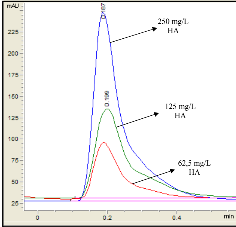
Şekil 7. 2. n-propanol hareketli fazında sisteme enjekte edilen 3 HA standardı pikinin bir arada gösterilişi
