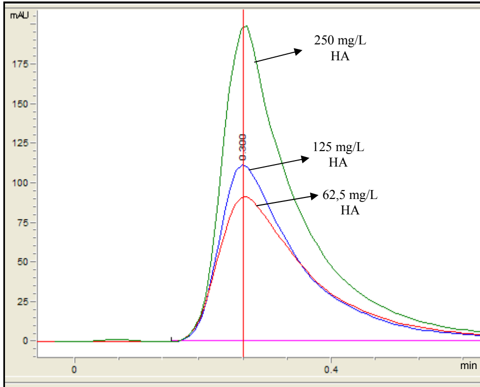
Şekil 7. 4 Sitrat/Fosfat tamponu hareketli fazında sisteme enjekte edilen 3 HA standardı pikinin bir arada gösterilişi
