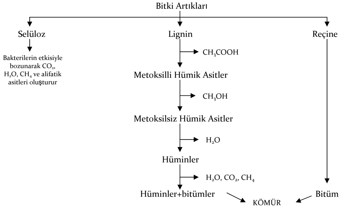
Şekil 2. 1. Lignin teorisine göre hümik maddelerin meydana gelişi
