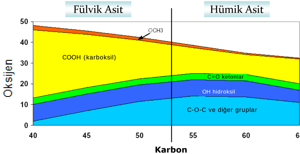
Şekil 2. 5. Fonksiyonel grup içeriği bakımından fülvik asit ve hümik asit
