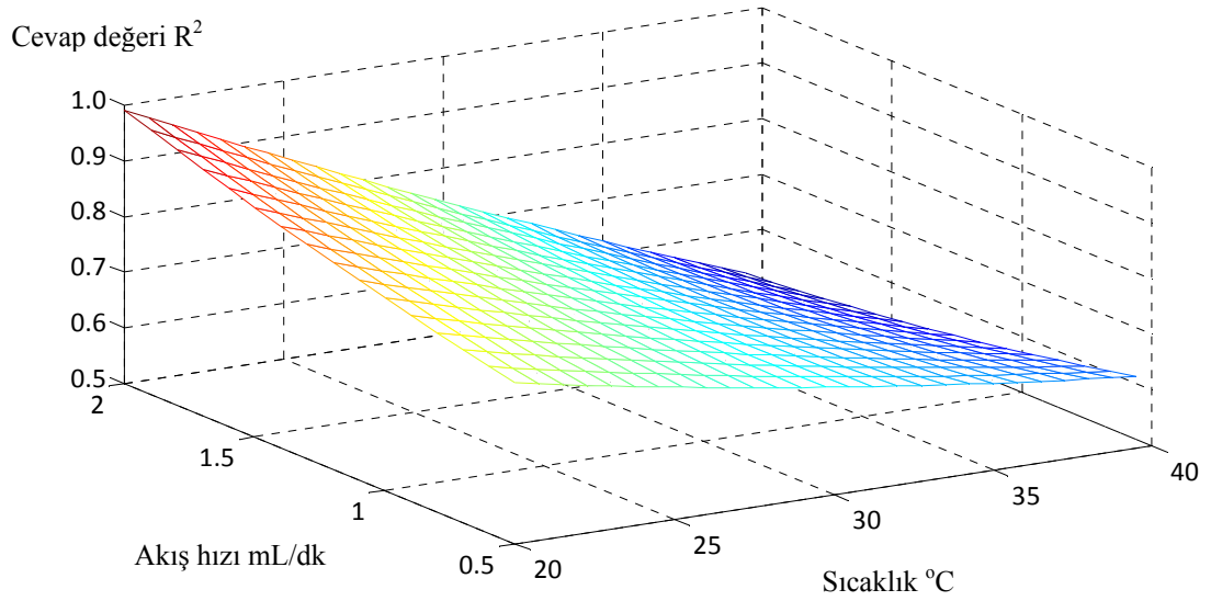
Şekil 7. 13. Değişen akış hızı ve sıcaklık değerlerinde R^2 'de meydana gelen değişimi gösteren 3 boyutlu yüzey grafiği
