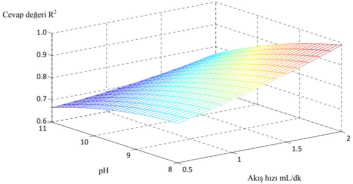
Şekil 7. 11. Değişen akış hızı ve pH değerlerinde R^2 'de meydana gelen değişimi gösteren 3 boyutlu yüzey grafiği
