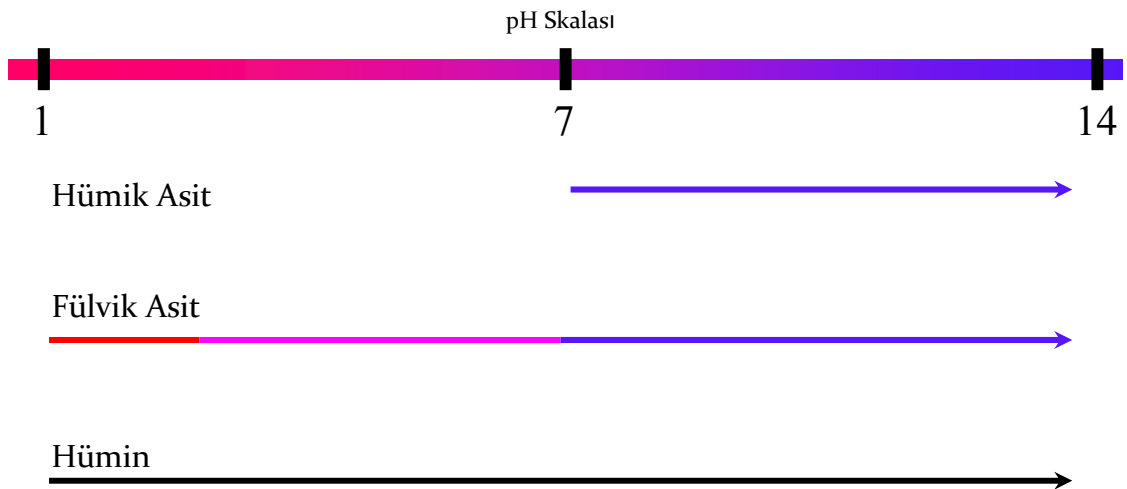
Şekil 2. 2. Hümik maddelerin farklı pH değerlerindeki çözünme kabiliyetlerine göre sınıflandırılması
