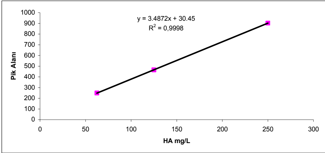
Şekil 6.12. Belirli bir deneysel koşula göre enjekte edilen 3 hümik asit standardının (62,5, 125 ve 250 mg/L) ardı ardına 3 tekrarlı analizden elde edilen 9 pik alanının bir grafikte gösterimi ve regresyon katsayısı
