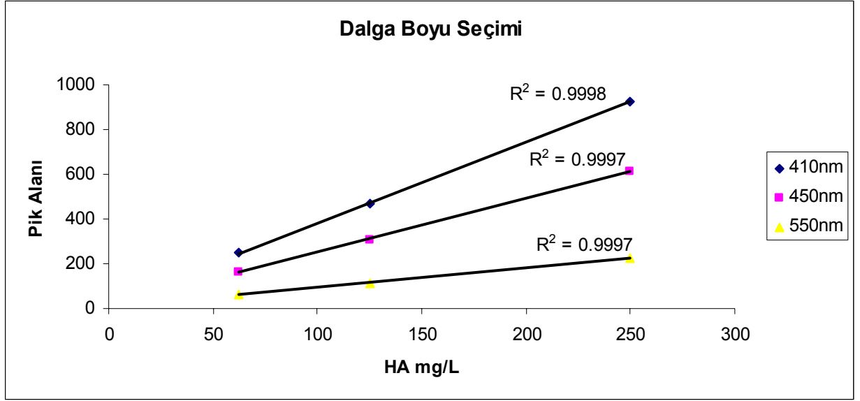
Şekil 7. 9. 410, 450 ve 550 nm dalga boylarında HA standartlarının verdiği pik alanları
