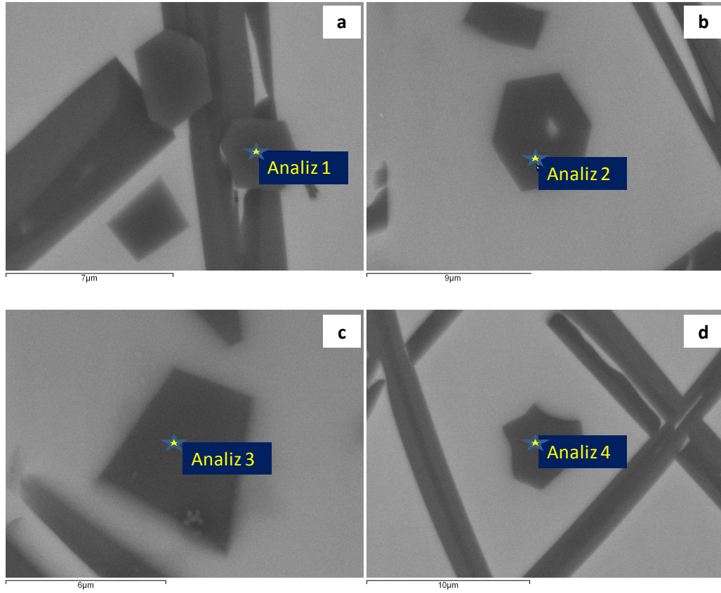
Şekil 4.76. K35 kodlu numunede sırtın içerisinde oluşmuş kristaller ve nokta analizlerinin yapıldığı noktalar a) analiz 1, b) analiz 2, c) analiz 3, d) analiz 4
