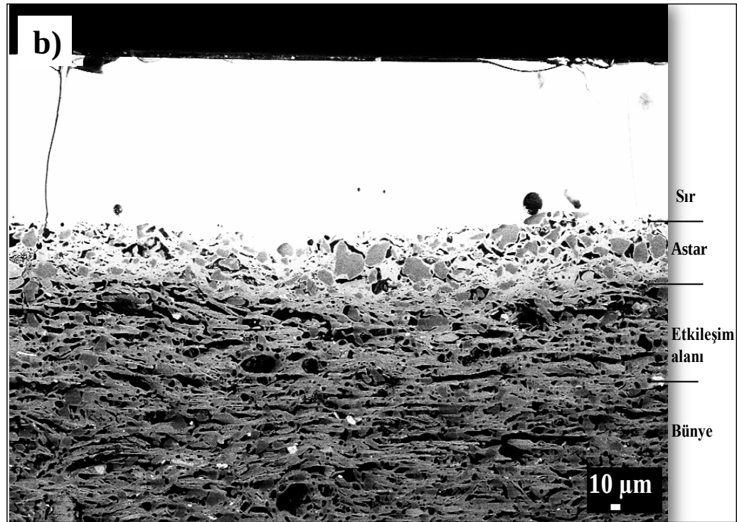
Şekil 4.13. K60 (graffito) kodlu numuneye ait temsili SEM (BSE) görüntüleri; a) bünye b) sır-bünye kesiti
