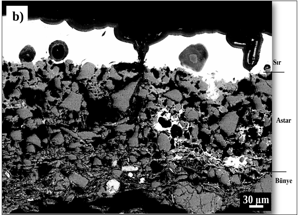
 ekil 4.22. G9 kodlu numuneye ait temsili SEM (BSE) g r nt leri; a) b nye b) sır-b nye kesiti
