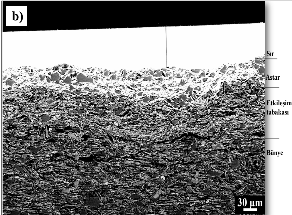
 ekil 4.20. G6 kodlu numuneye ait temsili SEM (BSE) g r nt leri; a) b nye b) sır-b nye kesiti
