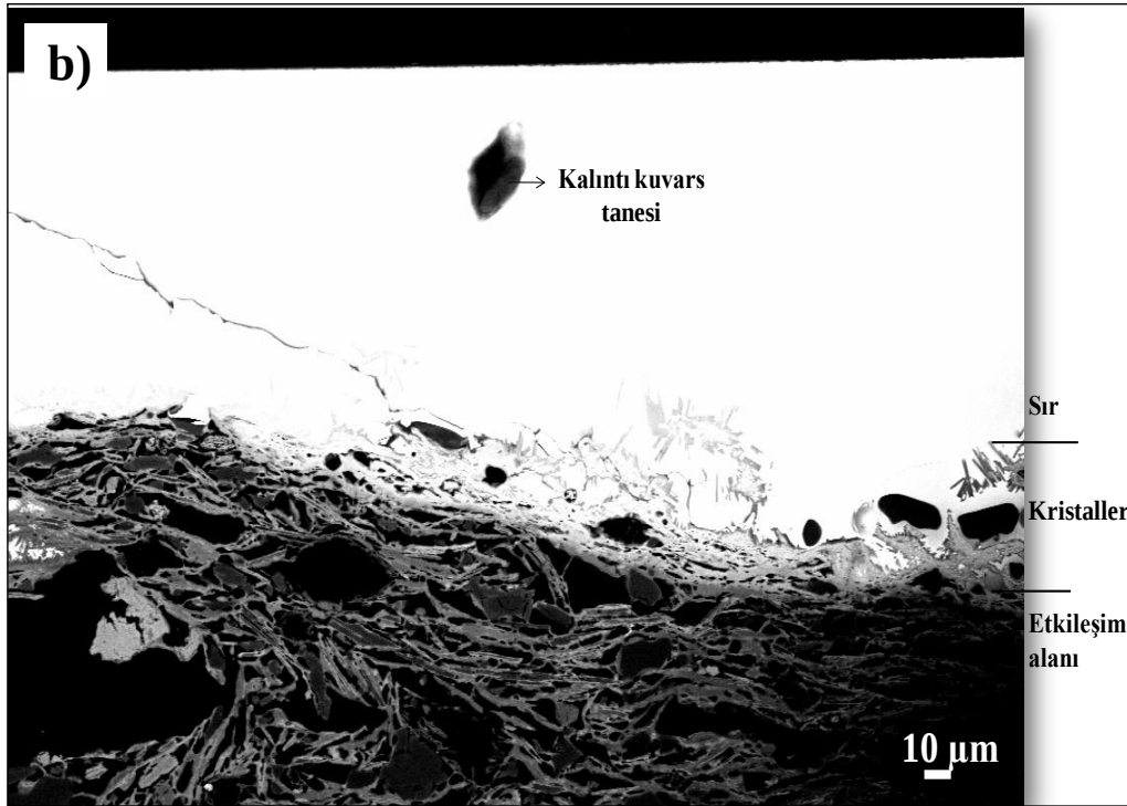
Şekil 4.10. K50 kodlu numuneye ait temsili SEM (BSE) görüntüleri; a) bünye b) sır-bünye kesiti
