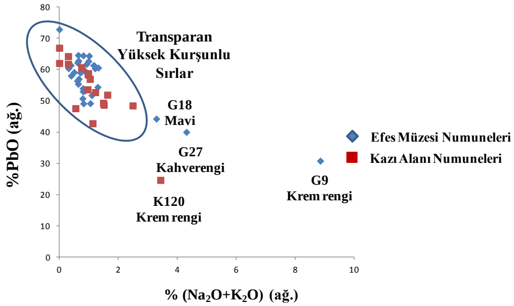
Şekil 4.35. Ayasuluk ve İsa Bey Hamamı Numunelerinin sırlarının SEM-EDX analizi sonuçlarına göre \%(\text{Na}_2\text{O}+\text{K}_2\text{O}) ve \% \text{PbO} oranları
