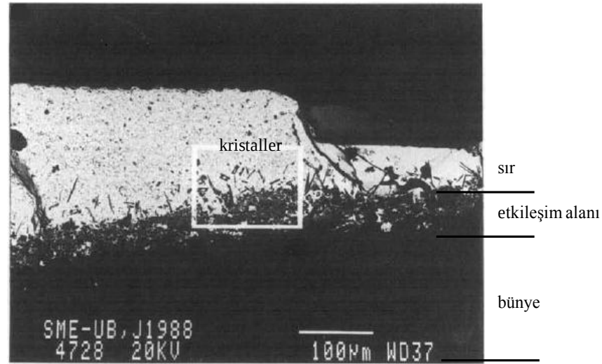
Şekil 2.4. İspanyada 14.yy Hispano-Moresque seramiğin yüksek kurşunlu sırası, sır-bünye ara yüzeyinde oluşan etkileşim alanı ve bu etkileşim alanındaki kristallerin SEM görüntüsü [45]
