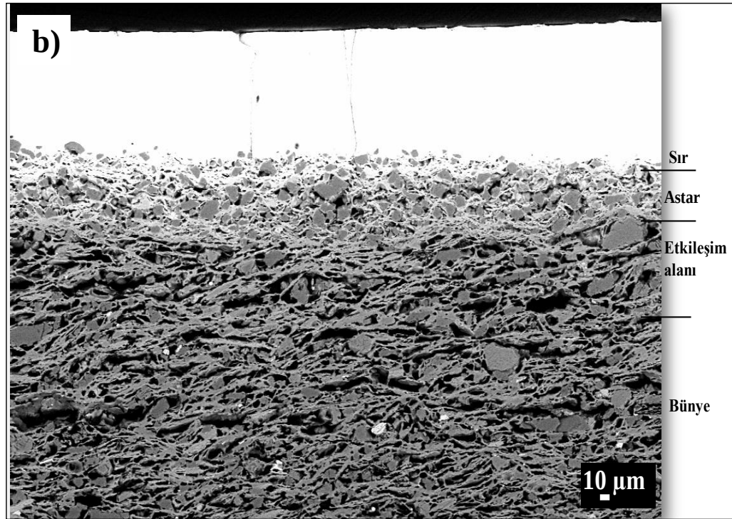
Şekil 4.11. K55 kodlu numuneye ait temsili SEM (BSE) görüntüleri; a) bünye b) sır-bünye kesiti
