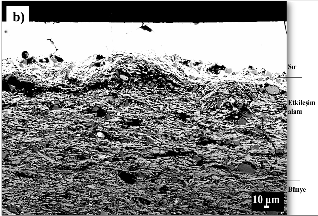
Şekil 4.9. K46 kodlu numuneye ait temsili SEM (BSE) görüntüleri; a) bünye b) sır-bünye kesiti
