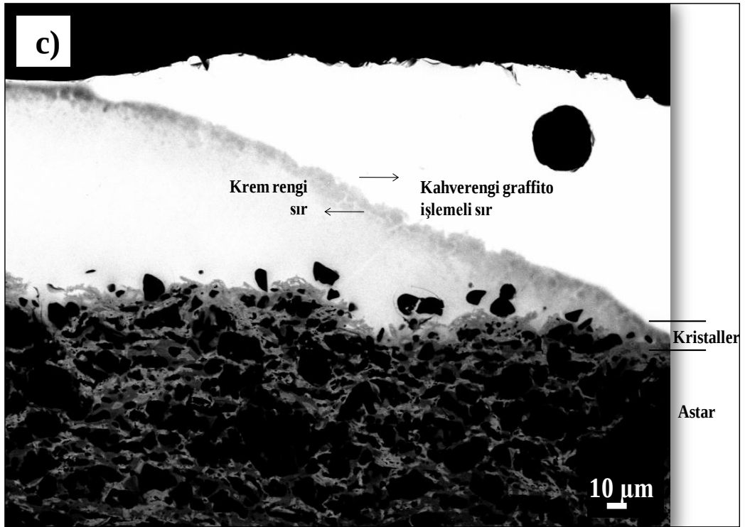
Şekil 4.16. K120 (graffito) kodlu numuneye ait temsili SEM (BSE) görüntüleri; a) bünye b) sır-bünye kesiti c) iki renkli sır bünye kesiti (Devam)
