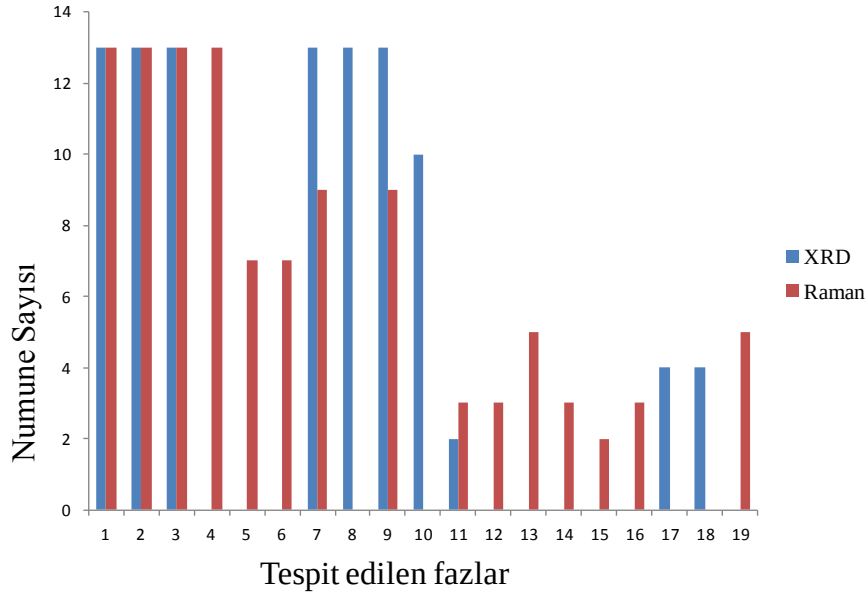
Şekil 4.64. Raman ve XRD analizi ile numunenlerin bünyelerinde bulunan fazların kümülatif sonuçlarının grafiği
