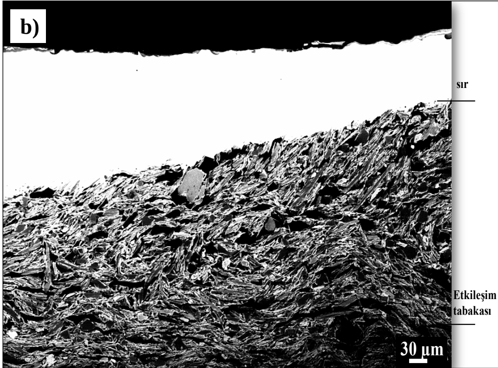
Şekil 4.17. G1 kodlu numuneye ait temsili SEM (BSE) görüntüleri; a) bünye b) sır-bünye kesiti
