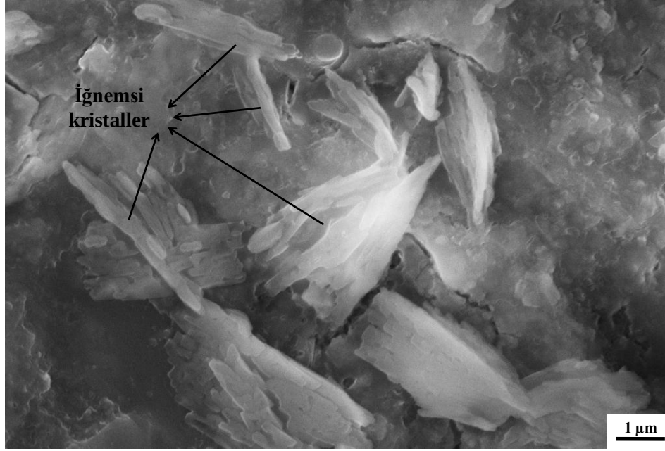
Şekil 4.74. Aşındırılmış ve dağlanmış sır tabakasının üst yüzeyinden alınan SEM-SE görüntüsü
