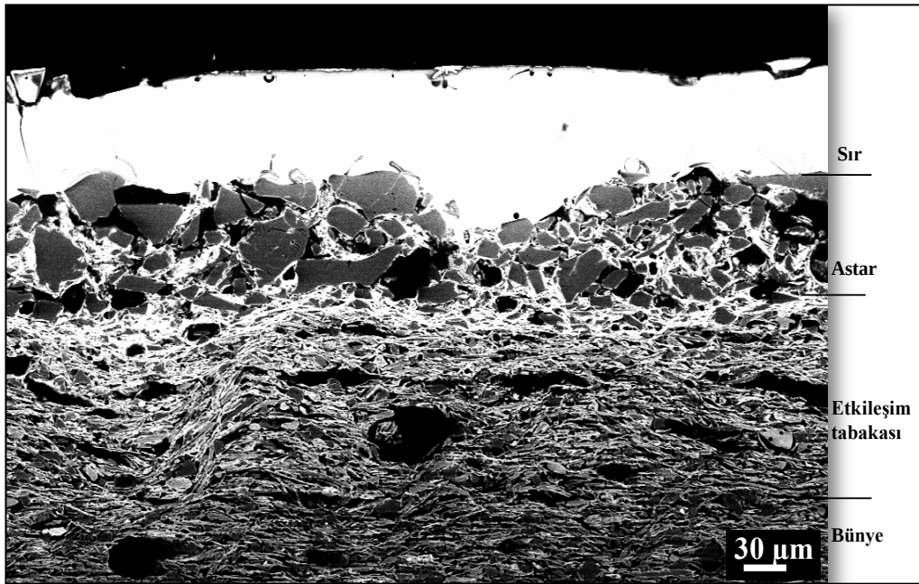
Şekil 4.31. G35 kodlu numuneye ait temsili SEM (BSE) görüntüleri; a) bünye b) sır-bünye kesiti
