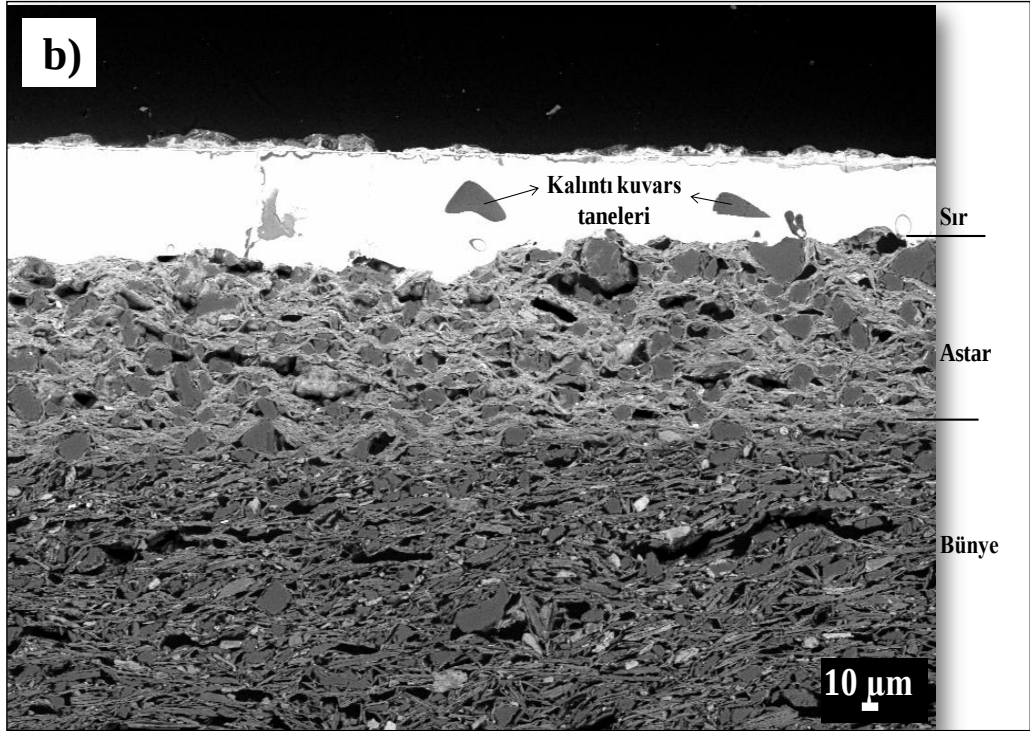
Şekil 4.8. K42 kodlu numuneye ait temsili SEM (BSE) görüntüleri; a) bünye b) sır-bünye kesiti
