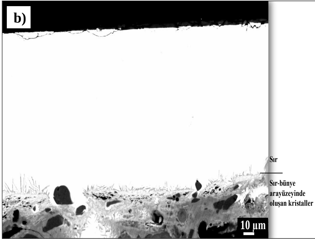
Şekil 4.6. K36 kodlu numuneye ait temsili SEM (BSE) görüntüleri; a) bünye b) sır-bünye kesiti
