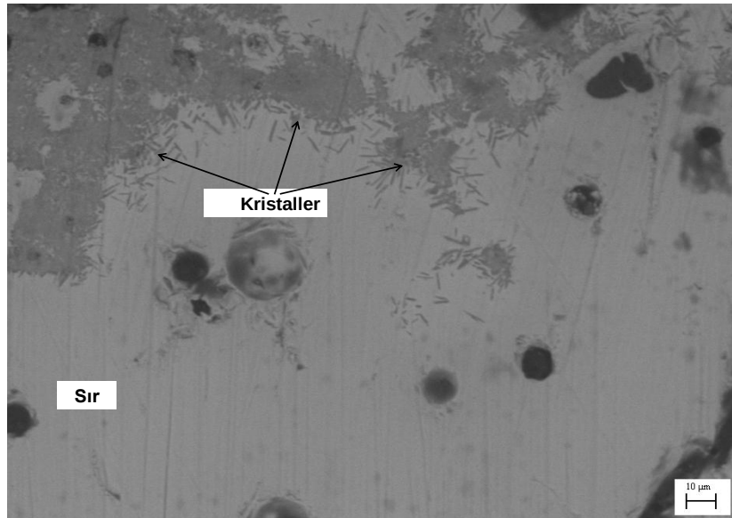
řekil 4.73. Ařındırılmıř sır tabakasının st yzeyinden alınan SEM-BSE grnts
