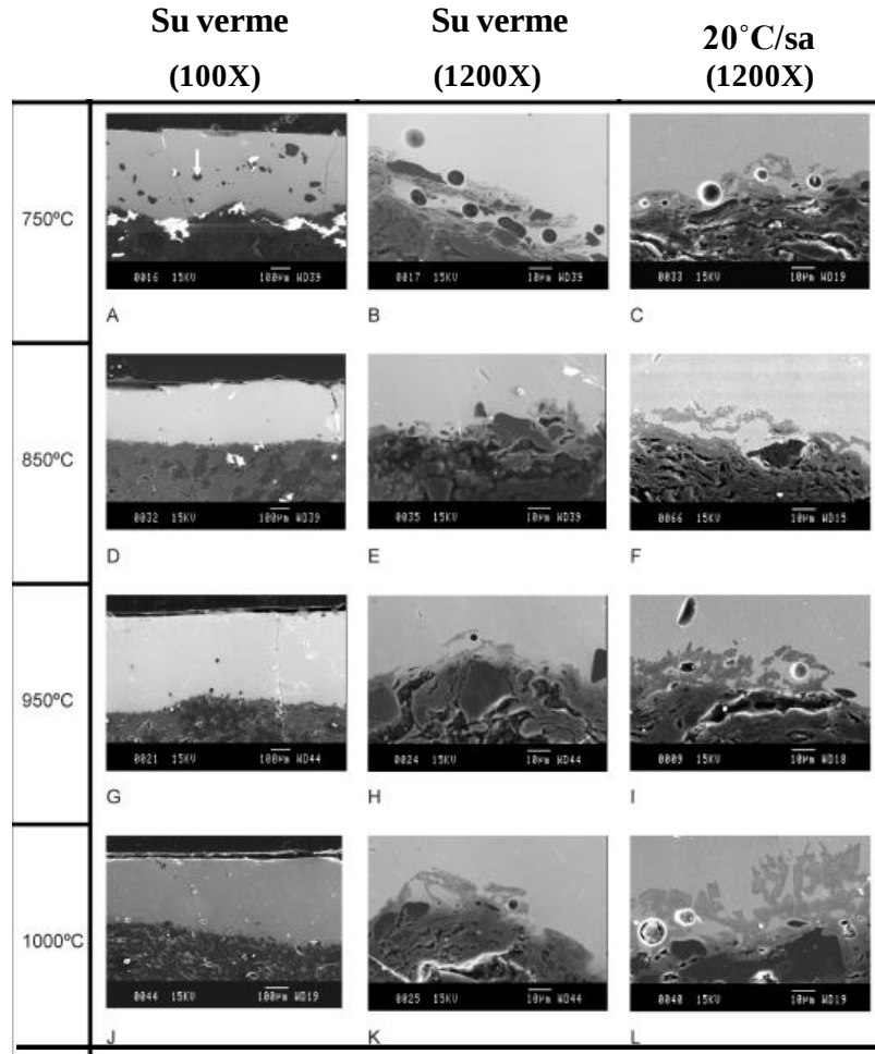
Şekil 2.7. 75/25 PbO/SiO 2 sınırının kaolinitik killi bünyeye farklı sıcaklıklarda uygulanması ardından numunelerin sır-bünye arayüzeylerinin 100X ve 1200X büyütme SEM görüntüleri, A) 750°C’de pişirilmiş ve su verme işlemi uygulanmış numune, numunenin sırında beyaz ok ile işaretlenmiş reaksiyona girmemiş kuvars taneleri [44]
