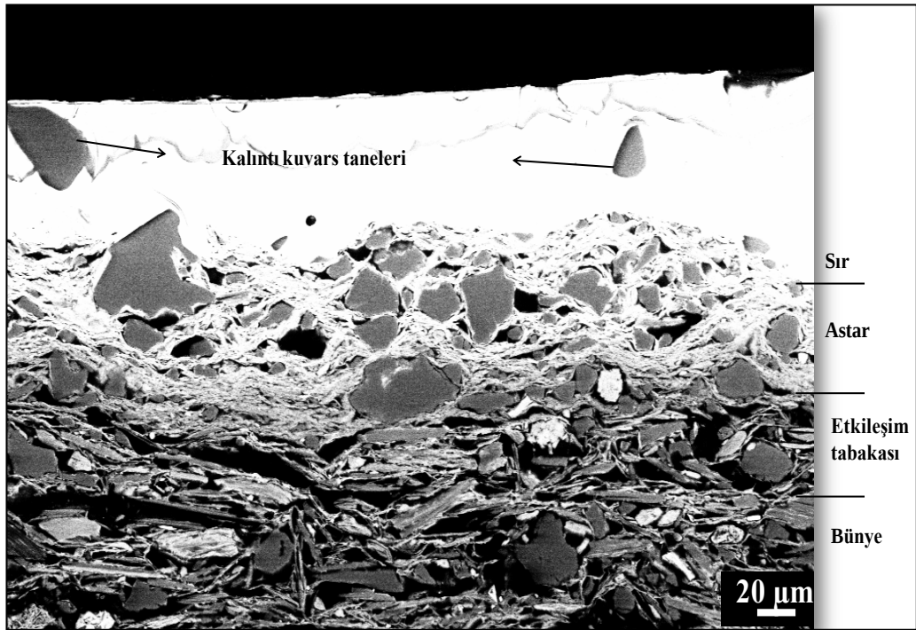
Şekil 4.27. G28 kodlu numuneyle ilgili SEM (BSE) görüntüleri; a) bünye b) sır-bünye kesiti
