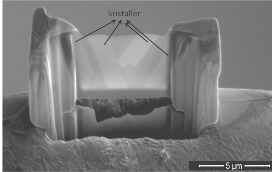
Şekil 4.70. FIB yöntemi ile numuneden çıkarılan iğnemsı kristallerin FIB cihazı ile alınmış görüntüsü
