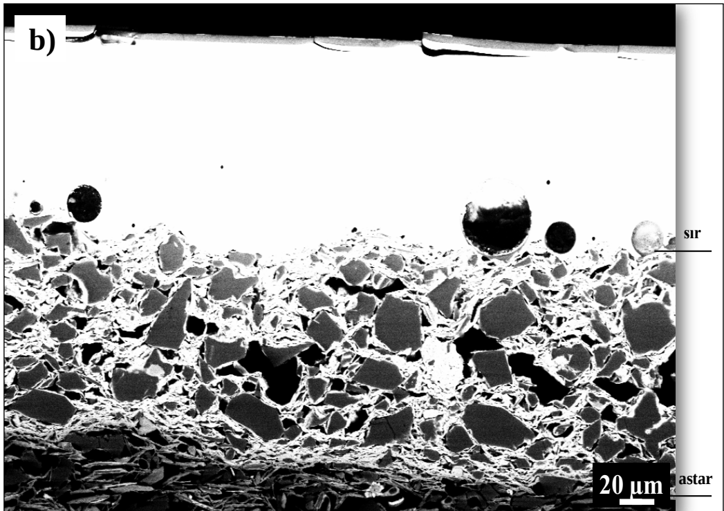
Şekil 4.21. G7 kodlu numuneye ait temsili SEM (BSE) görüntüleri; a) bünye b) sır-bünye kesiti
