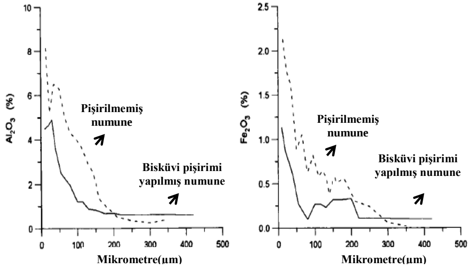
Şekil 2.6. Pişirilmemiş ve bisküvi pişirimi yapılmış numunelere uygulanan kurşunlu sırın pişirimi sonrası bünyeden sıra doğru (orjin=0 mikron) Al_2O_3 ve Fe_2O_3 oksitlerinin konsantrasyonlarının değişimi [42]
