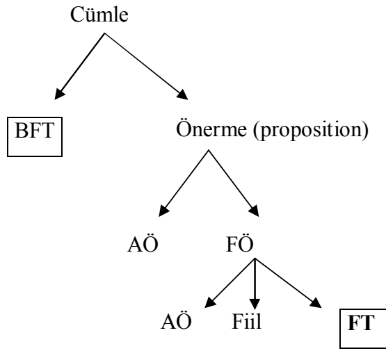
Şekil 8: Helbig ve Schenkel (1991)'in Derin Yapı Analizi
