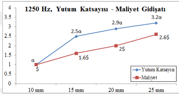
Şekil 6.5 : Poliüretan (PU) malzemenin kalınlığına bağlı olarak yutum katsayısı ve maliyet arasındaki ilişki
