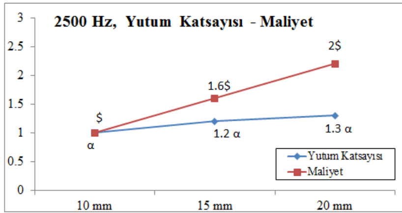
Şekil 6.9 : Koton keçe malzemenin kalınlığına bağlı olarak yutum katsayısı ve maliyet arasındaki ilişki
