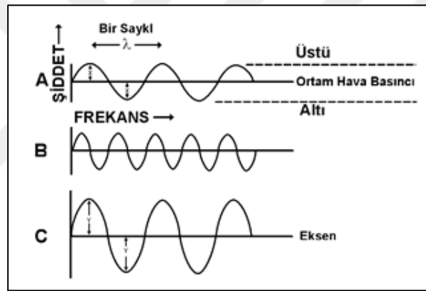
Şekil 2.2 : Ses Dalgası [1]
