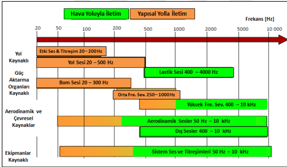
Şekil 4.2 : Araç ses ve titreşim kaynağı frekans analizi
