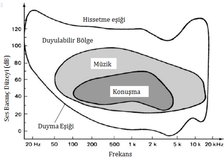
Şekil 2.1 : İşitme sınır eğrisi
