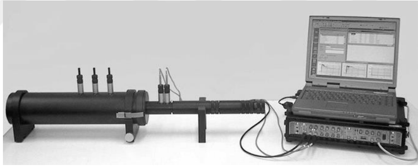
Şekil 3.1 : Empedans tüp ölçüm yöntemi test düzeneği [2].
