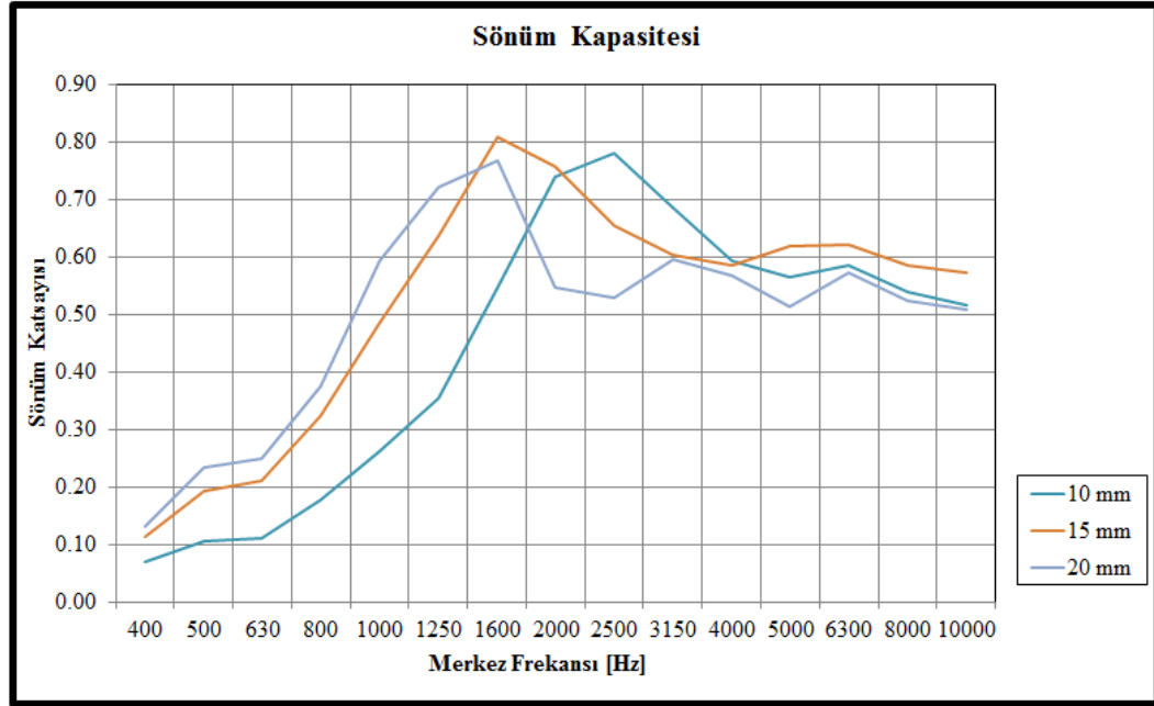
Şekil 6.6 : Polipropilen ses sönüm katsayısı – kalınlık değişimi
