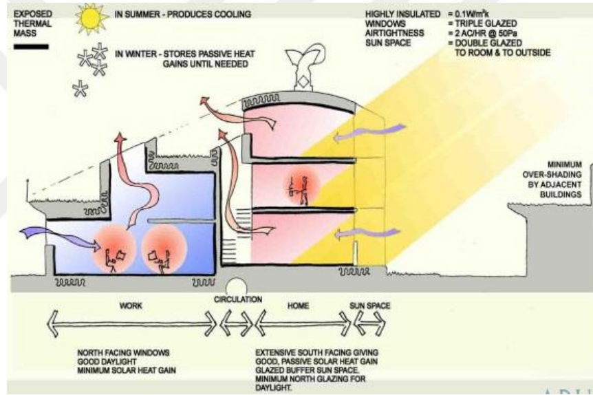
Şekil 3.4. Fiziksel çevre verilerinin bina kabuğunda değerlendirilmesi [38].
