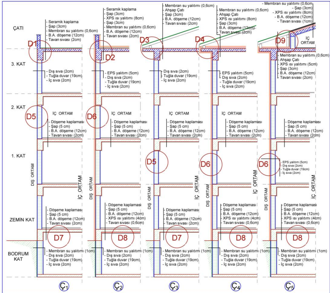
Şekil 4.25. Dört Katlı (B+Z+3K) örnek bina kısmi kesit
