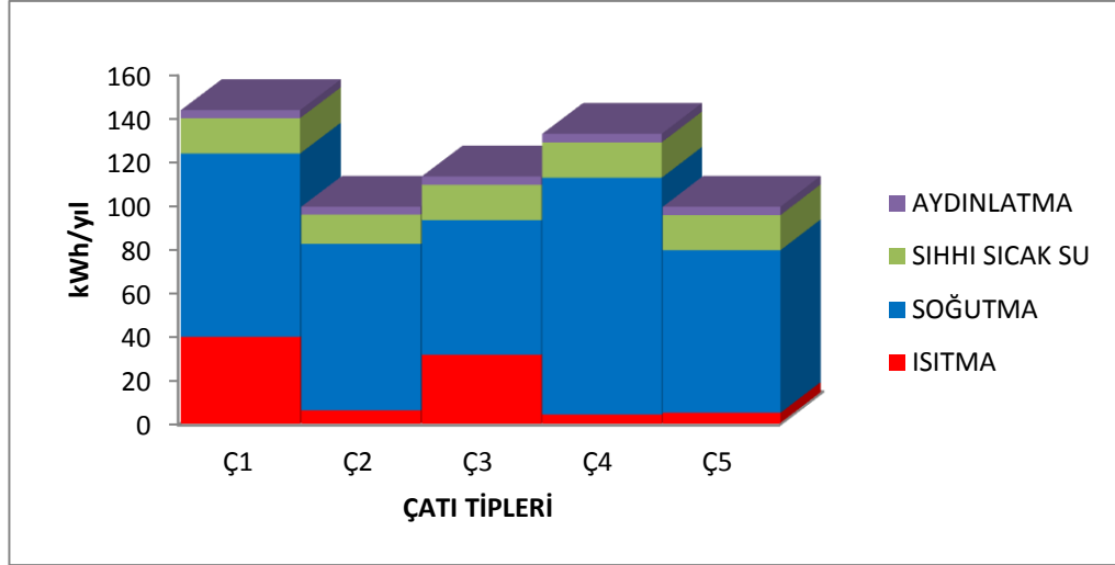
Şekil 4.33. 1.D.G. Bölgesi (Adana) (B+Z+5 / Altı Katlı) sonuçları (URL, Ocak 2017)
