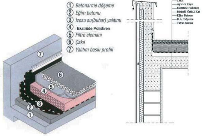
b. Teras çatı yalıtımı
