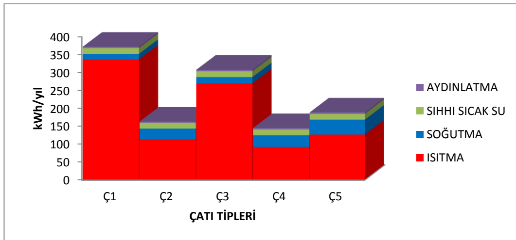
Şekil 4.44. 4.D.G.Bölgesi (Erzurum) (B+Z+3 / Dört Katlı) sonuçları (URL, Ocak 2017)
