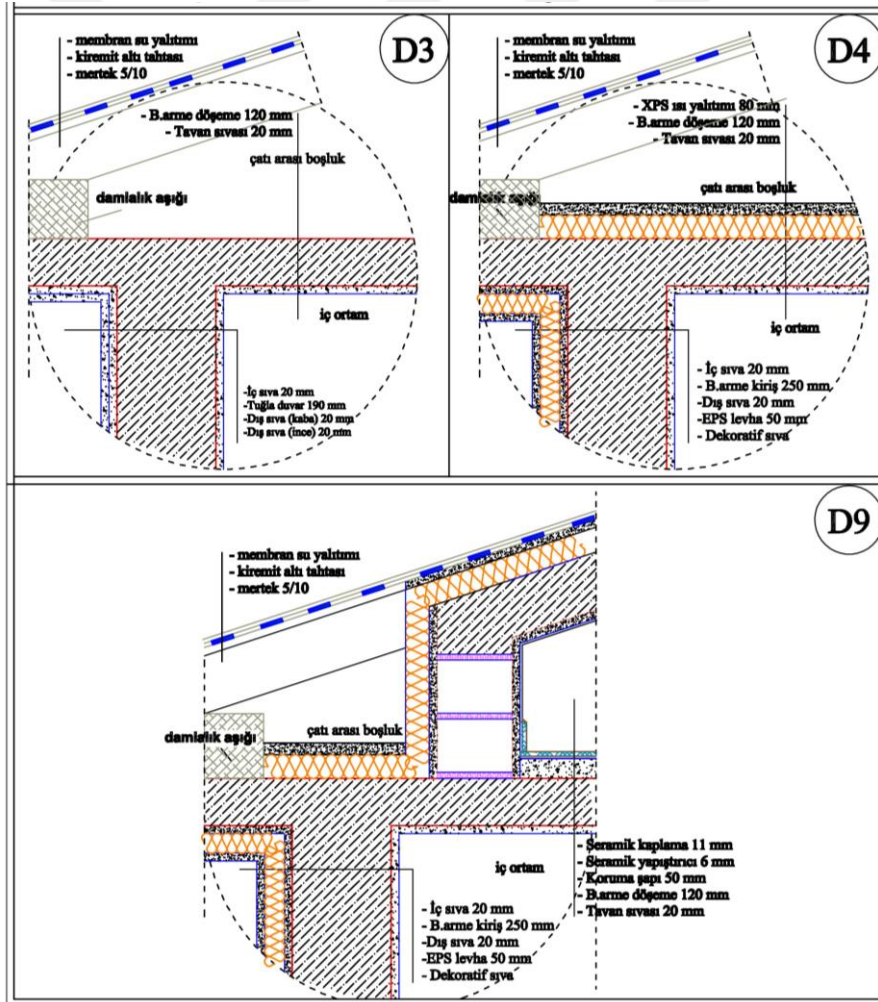
Şekil 4.28. Eğimli çatı tipleri (Ç3,Ç4,Ç5) nokta detayları
