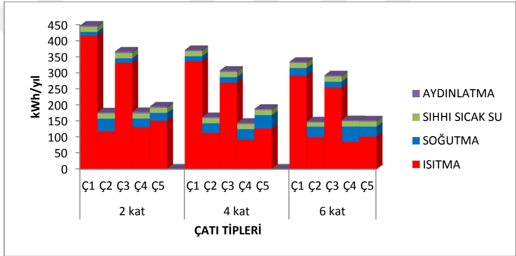
Şekil 4.46. 4.D.G.Bölgesi (Erzurum) iki, dört, altı katlı sonuçları (URL, Ocak 2017)
