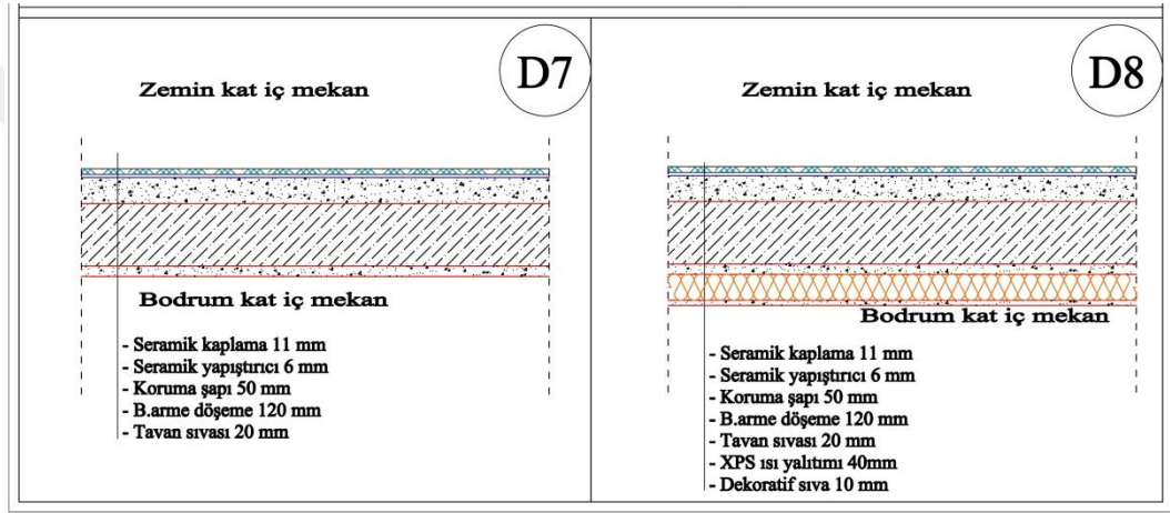
Şekil 4.30. Isıtılan ve ısıtılmayan döşeme nokta detayları
