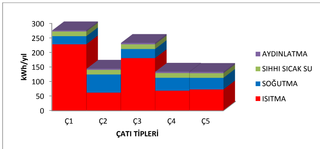
Şekil 4.39. 3.D.G. Bölgesi (Ankara)(B+Z+1 / İki Katlı) sonuçları (URL, Ocak 2017)
