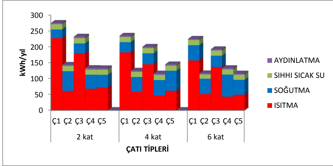
Şekil 4.42. 3.D.G. Bölgesi (Ankara) iki, dört, altı katlı sonuçları (URL, Ocak 2017)
