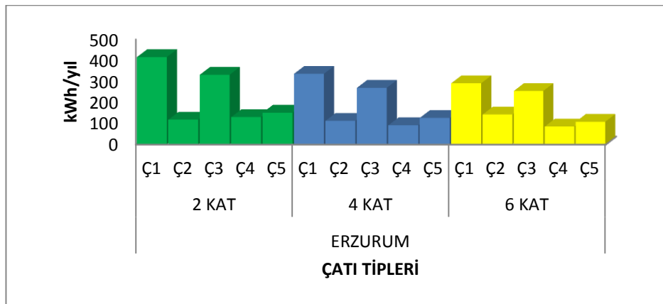
Şekil 5.8. Erzurum ilindeki beş farklı çatı tipinin iki, dört ve altı katlı binalardaki ısıtma enerji ihtiyaçları
