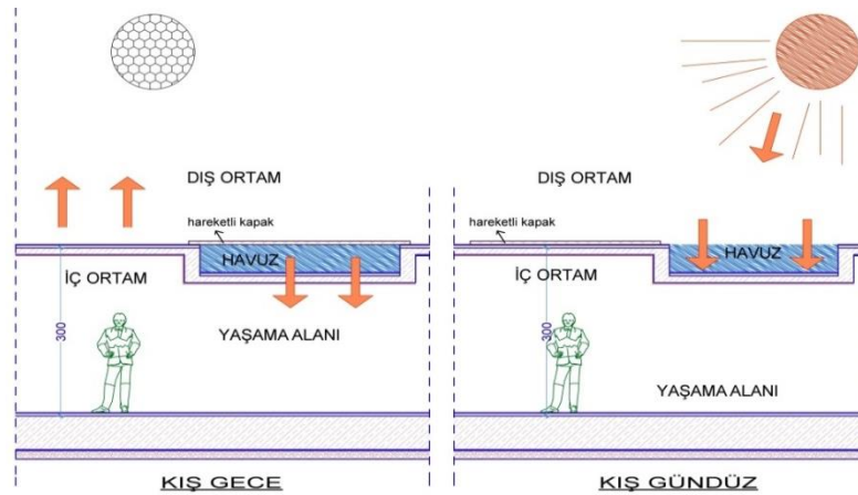
Şekil 3.16. Çatı havuzlarının kış dönemi çalışma prensibi [48]
