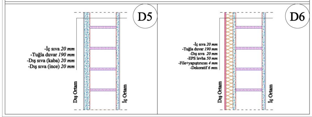
Şekil 4.29. Dış duvar nokta detayları
