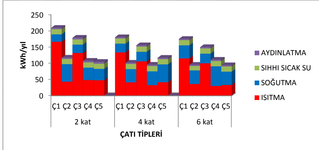
Şekil 4.38. 2.D.G. Bölgesi (İstanbul) iki, dört, altı katlı sonuçları (URL, Ocak 2017)
