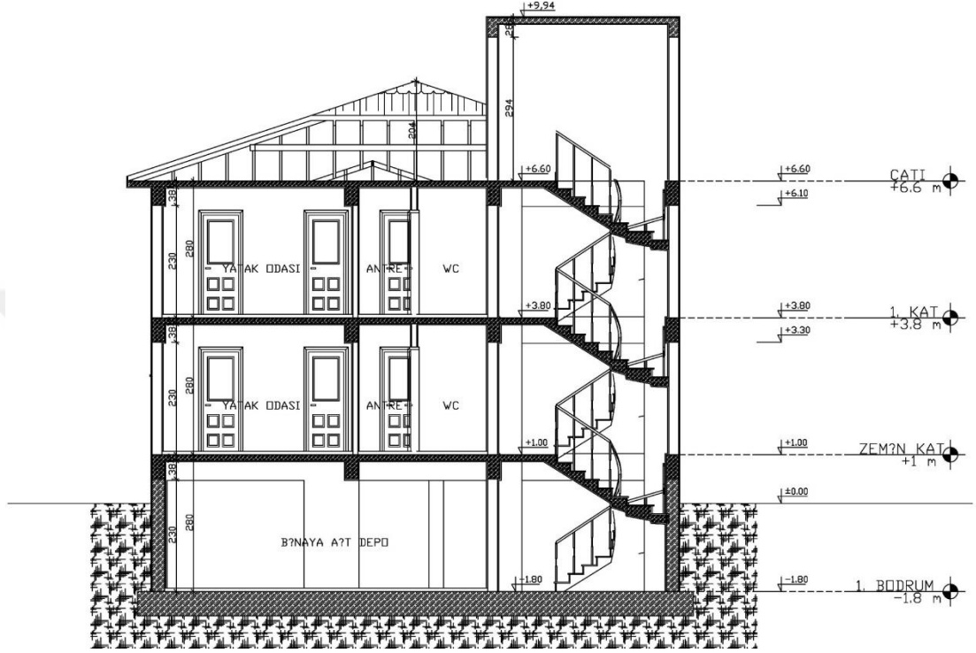
Şekil B.1. İncelenen örnek proje A-A kesiti (B+Z+1K / İki Katlı)
