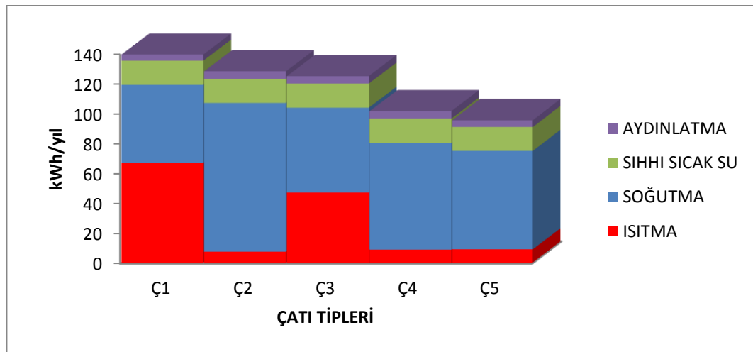
Şekil 4.31. 1.D.G. Bölgesi (Adana) (B+Z+1/ İki Katlı) sonuçları (URL, Ocak 2017)
