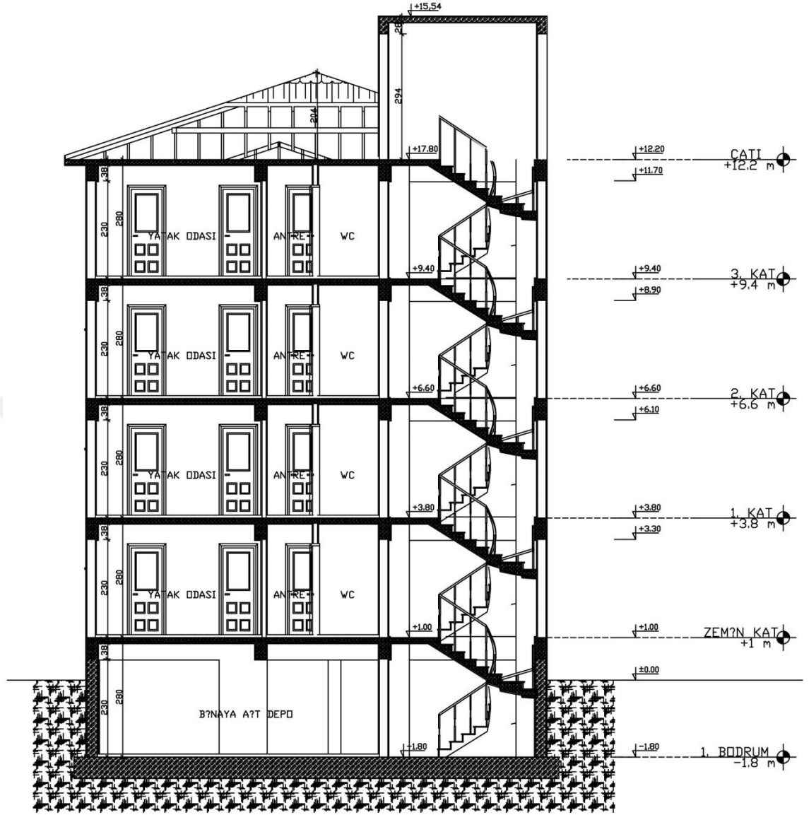
Şekil B.2. İncelenen örnek proje A-A kesiti (B+Z+3K / Dört Katlı)
