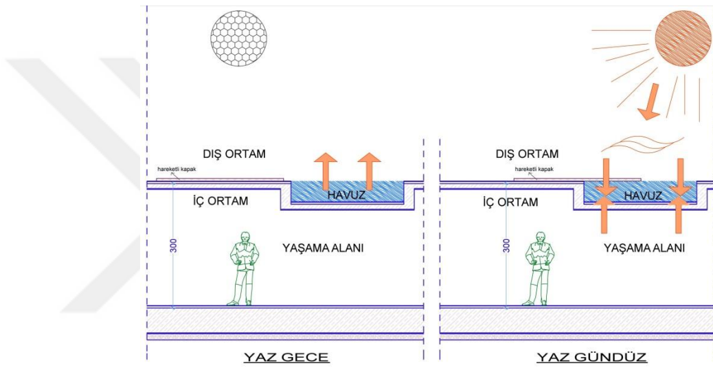
Şekil 3.17. Çatı havuzlarının yaz dönemi çalışma prensibi
