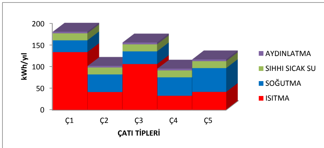
Şekil 4.36. 2.D.G. Bölgesi (İstanbul) (B+Z+3 / Dört Katlı) sonuçları (URL, Ocak 2017)
