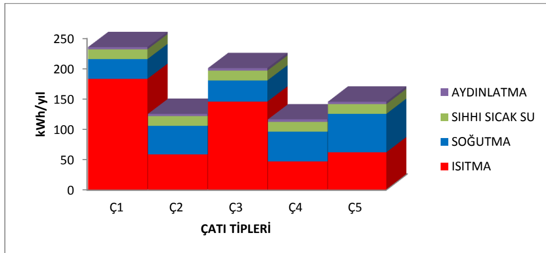
Şekil 4.40. 3.D.G.Bölgesi (Ankara) (B+Z+3 / Dört Katlı) sonuçları (URL, Ocak 2017)
