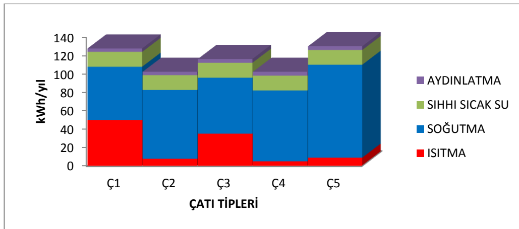
Şekil 4.32. 1.D.G. Bölgesi (Adana)(B+Z+3 / Dört Katlı) sonuçları (URL, Ocak 2017)
