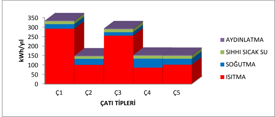
Şekil 4.45. 4.D.G.Bölgesi (Erzurum) (B+Z+5 / Altı Katlı) sonuçları (URL, Ocak 2017)
