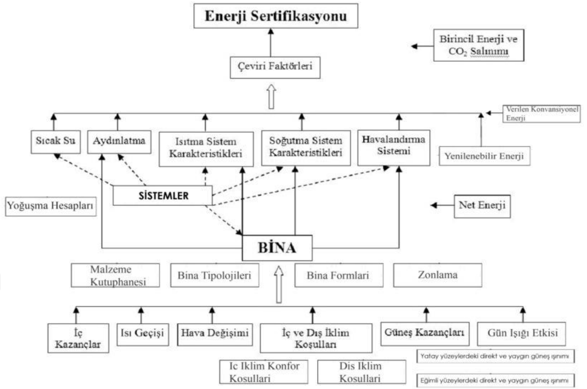
Şekil 4.1. BEP-TR hesaplama yöntemi esasları [58].
