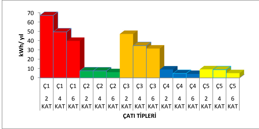
Şekil 5.1. Adana ilindeki beş farklı çatı tipinin iki, dört ve altı katlı binalardaki ısıtma enerji ihtiyaçları
