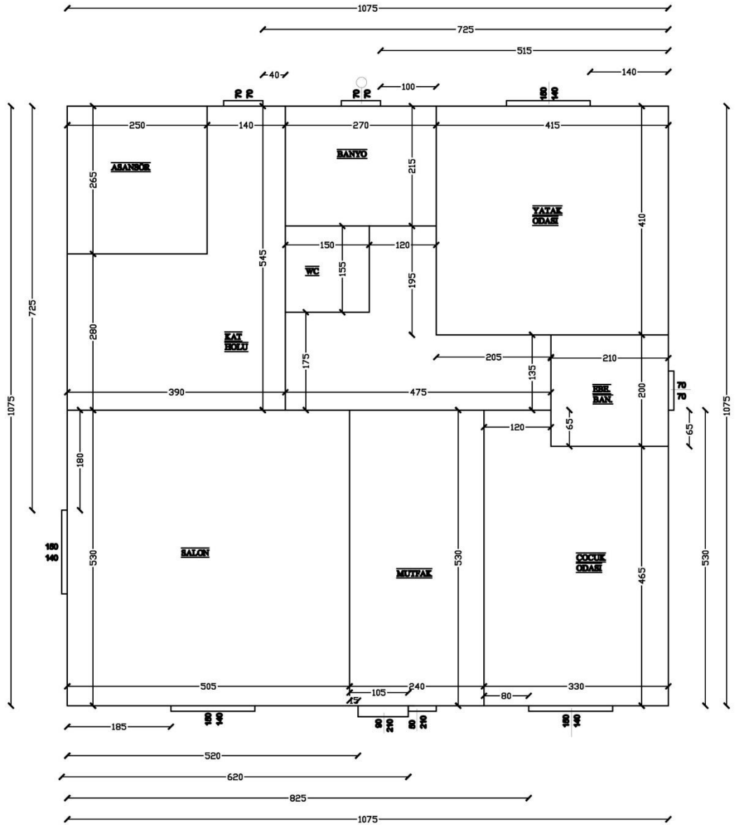
Şekil 4.3. Örnek projenin tel çerçeve çizimi
