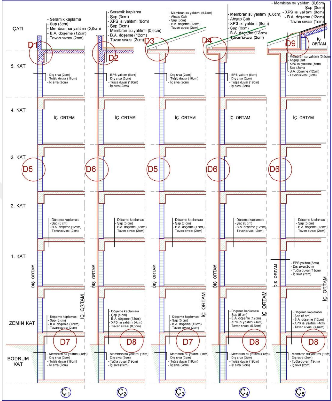
Şekil 4.26. Altı Katlı (B+Z+5K) örnek bina kısmi kesit
