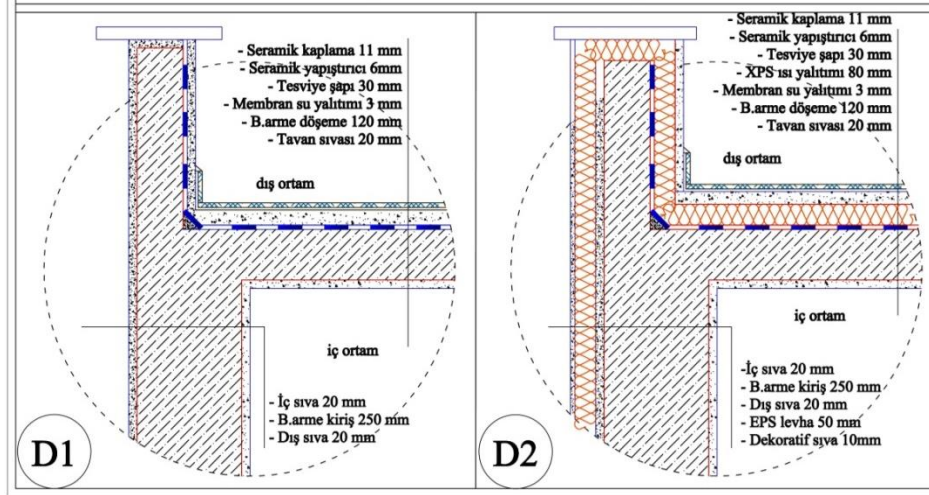
Şekil 4.27. Teras çatı tipleri (Ç1,Ç2) nokta detayları
