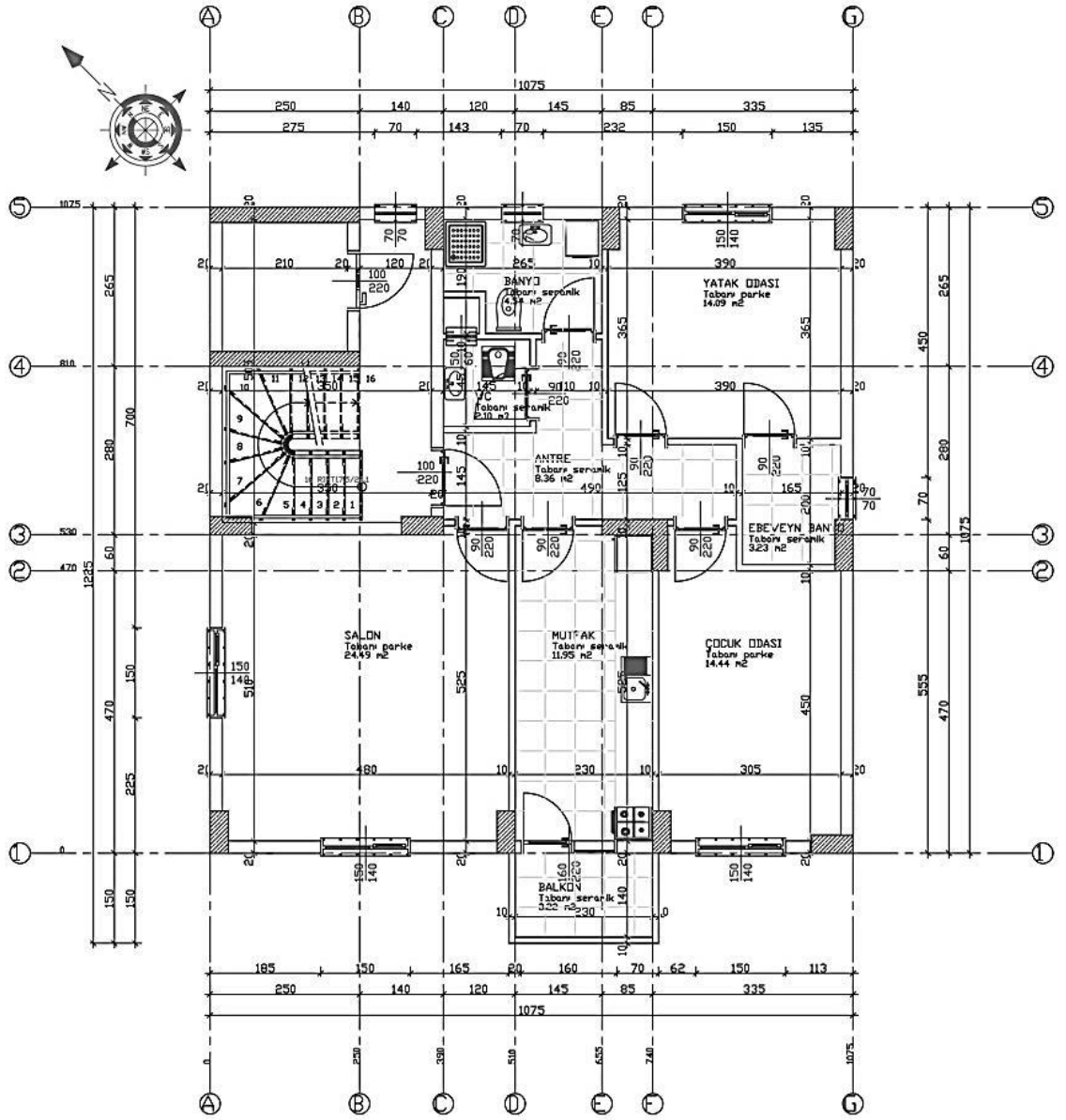
Şekil A.3. İncelenen örnek proje normal kat planı
