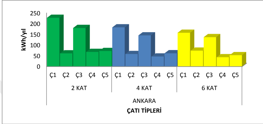
Şekil 5.7. Ankara ilindeki beş farklı çatı tipinin iki, dört ve altı katlı binalardaki ısıtma enerji ihtiyaçları
