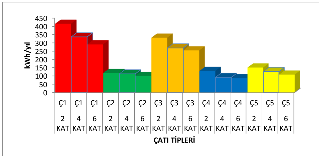
Şekil 5.4. Erzurum ilindeki beş farklı çatı tipinin iki, dört ve altı katlı binalardaki ısıtma enerji ihtiyaçları
