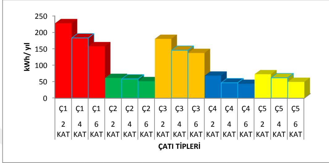
Şekil 5.3. Ankara ilindeki beş farklı çatı tipinin iki, dört ve altı katlı binalardaki ısıtma enerji ihtiyaçları
