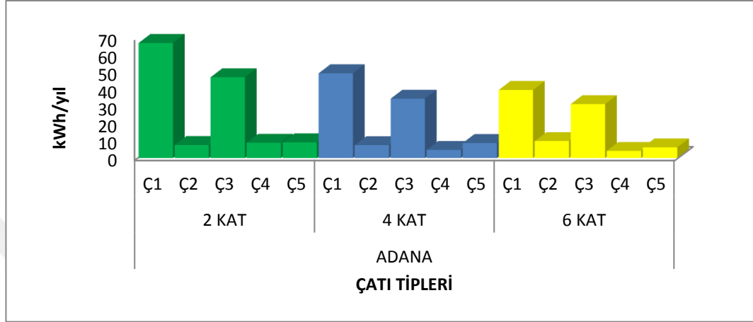
Şekil 5.5. Adana ilindeki beş farklı çatı tipinin iki, dört ve altı katlı binalardaki ısıtma enerji ihtiyaçları
