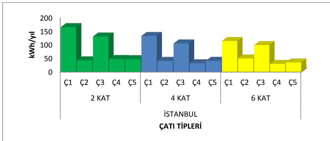
Şekil 5.6. İstanbul ilindeki beş farklı çatı tipinin iki, dört ve altı katlı binalardaki ısıtma enerji ihtiyaçları
