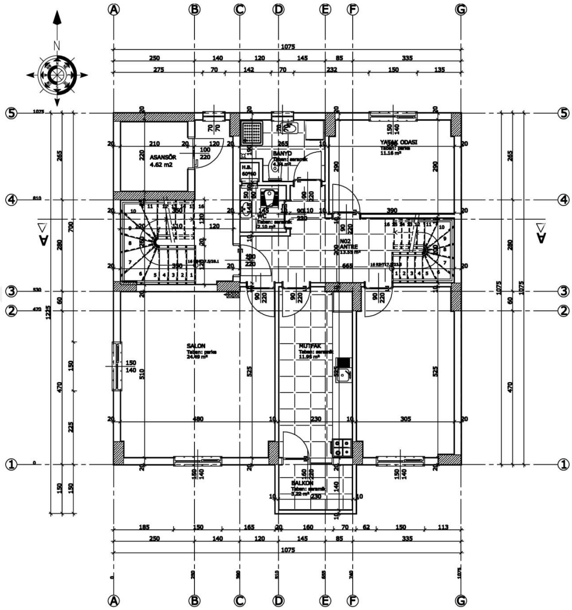
Şekil A.4. İncelenen örnek proje son kat planı
