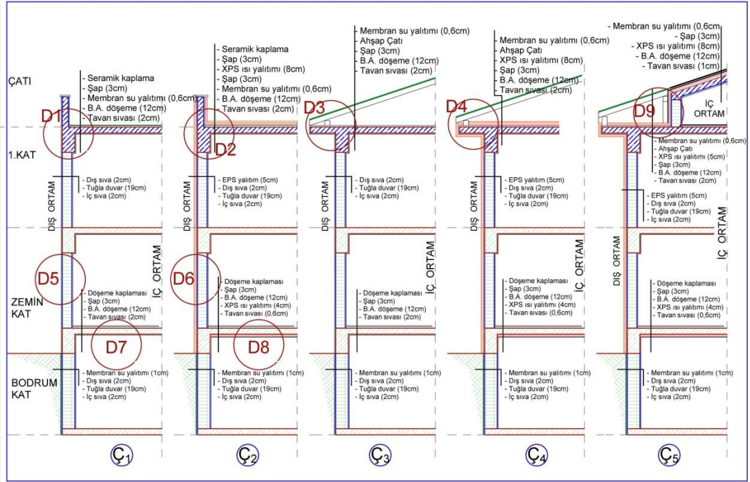
Şekil 4.24. İki Katlı (B+Z+1K) örnek bina kısmi kesit
