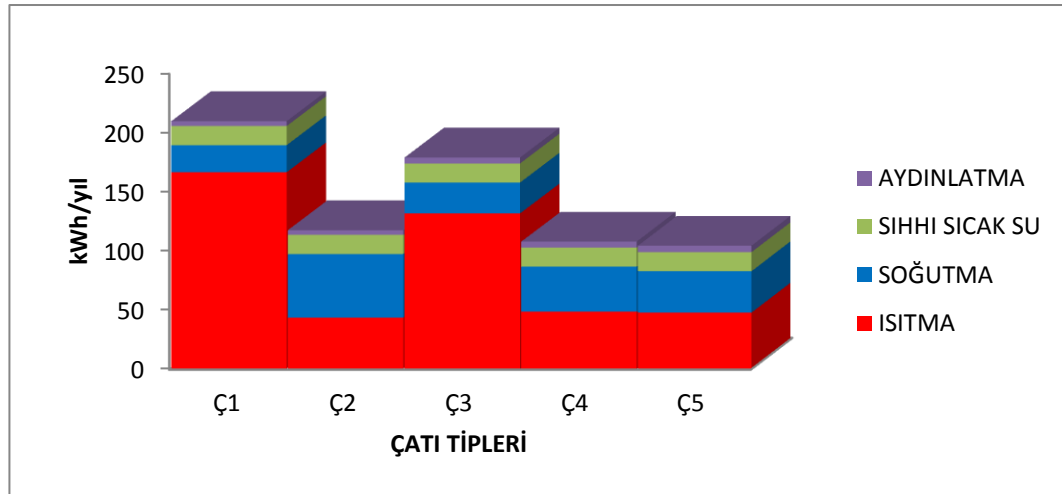
Şekil 4.35. 2.D.G. Bölgesi (İstanbul) (B+Z+1 / İki Katlı) sonuçları (URL, Ocak 2017)
