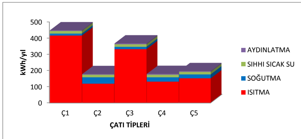
Şekil 4.43. 4.D.G. Bölgesi (Erzurum) (B+Z+1 / İki Katlı) sonuçları (URL, Ocak 2017)
