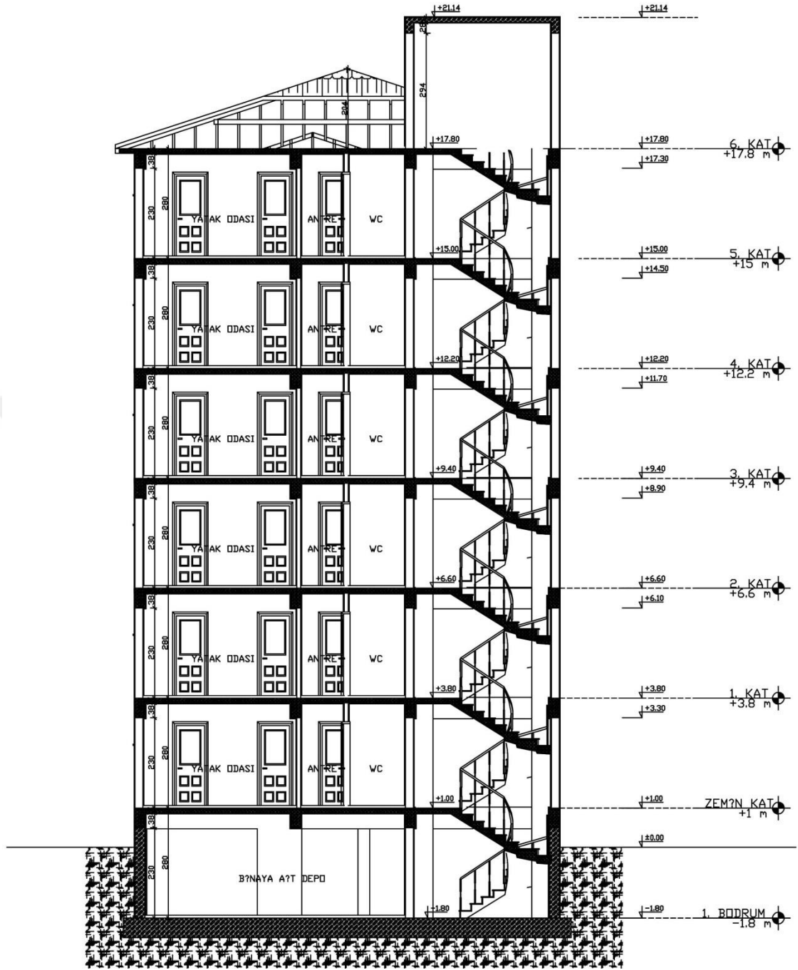
Şekil B.3. İncelenen örnek proje A-A kesiti (B+Z+5K / Altı Katlı)
