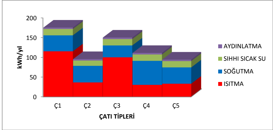
Şekil 4.37. 2.D.G. Bölgesi (İstanbul) (B+Z+5 / Altı Katlı) sonuçları (URL, Ocak 2017)
