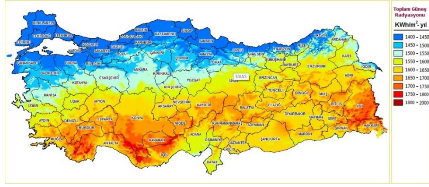
Şekil 2.3. Türkiye'nin güneş enerjisi potansiyel haritası [24].
