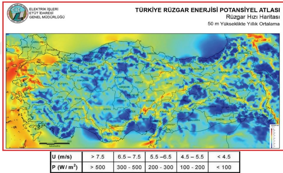
Şekil 2.4. Türkiye'nin rüzgar enerjisi potansiyel haritası [26].
