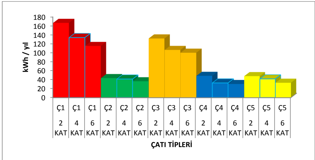
Şekil 5.2. İstanbul ilindeki beş farklı çatı tipinin iki, dört ve altı katlı binalardaki ısıtma enerji ihtiyaçları
