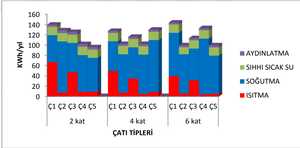
Şekil 4.34. 1.D.G. Bölgesi (Adana) iki, dört, altı katlı sonuçları (URL, Ocak 2017)
