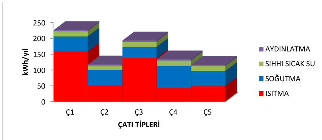
Şekil 4.41. 3.D.G. Bölgesi (Ankara) (B+Z+5 / Altı Katlı) sonuçları (URL, Ocak 2017)
